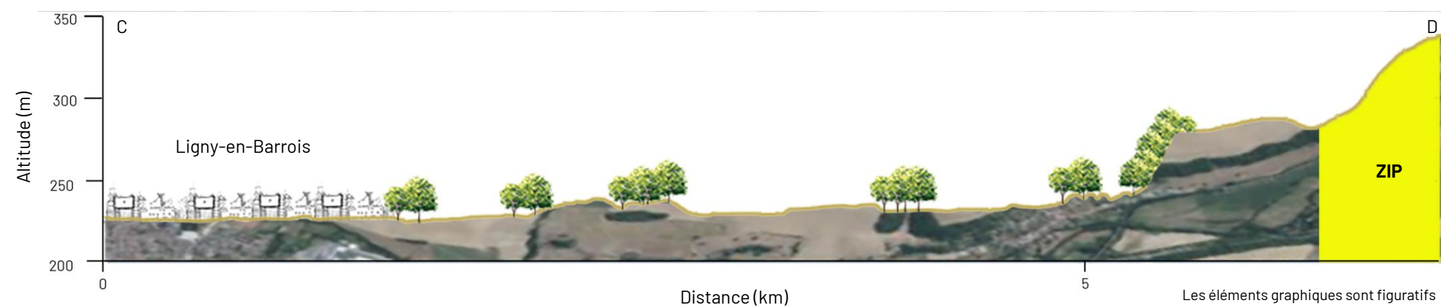
Illustration 1 : Coupe CD © Ora environnement
