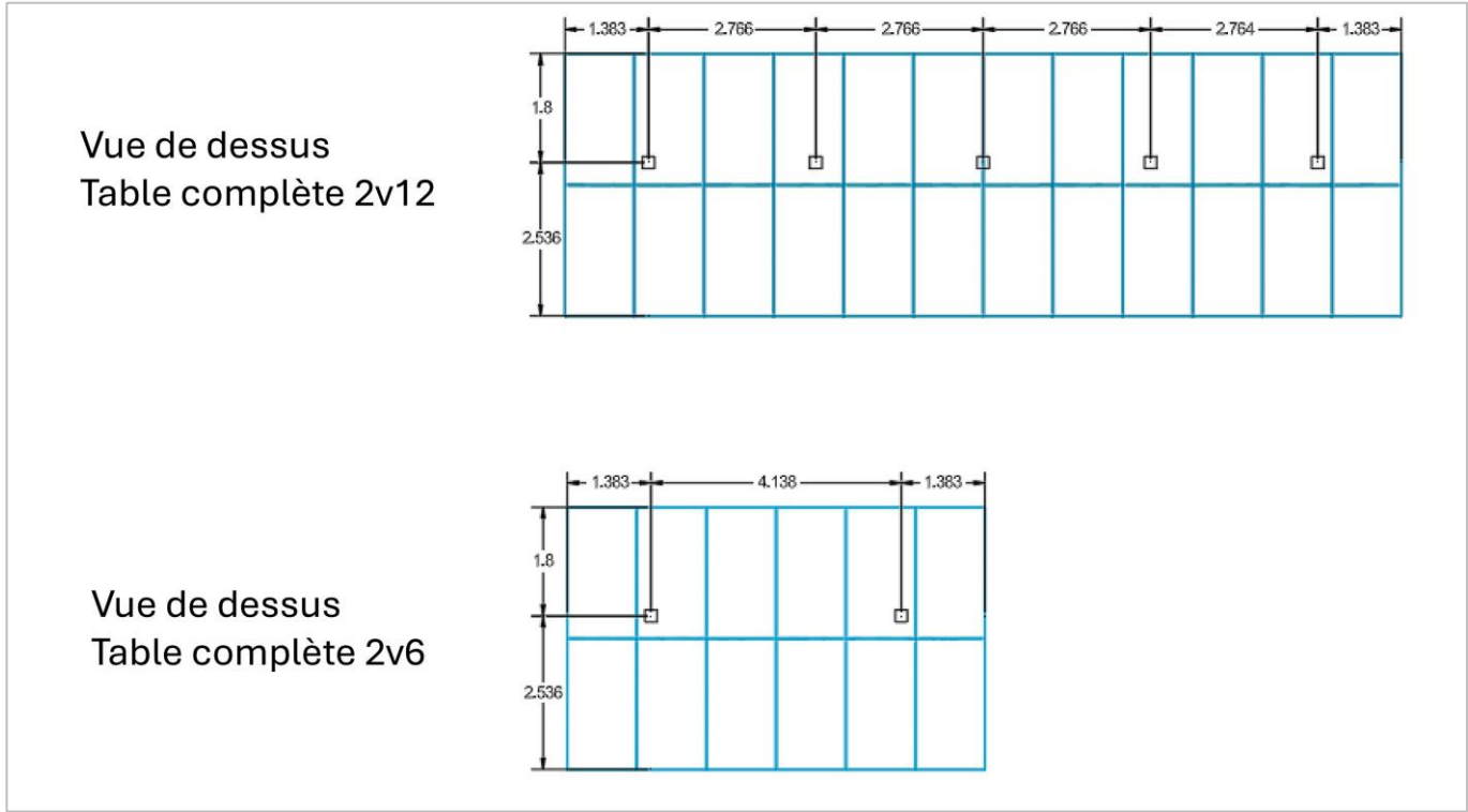
Figure 41 : Plan des structures photovoltaïques vues de haut (Source : ESCOFI)
