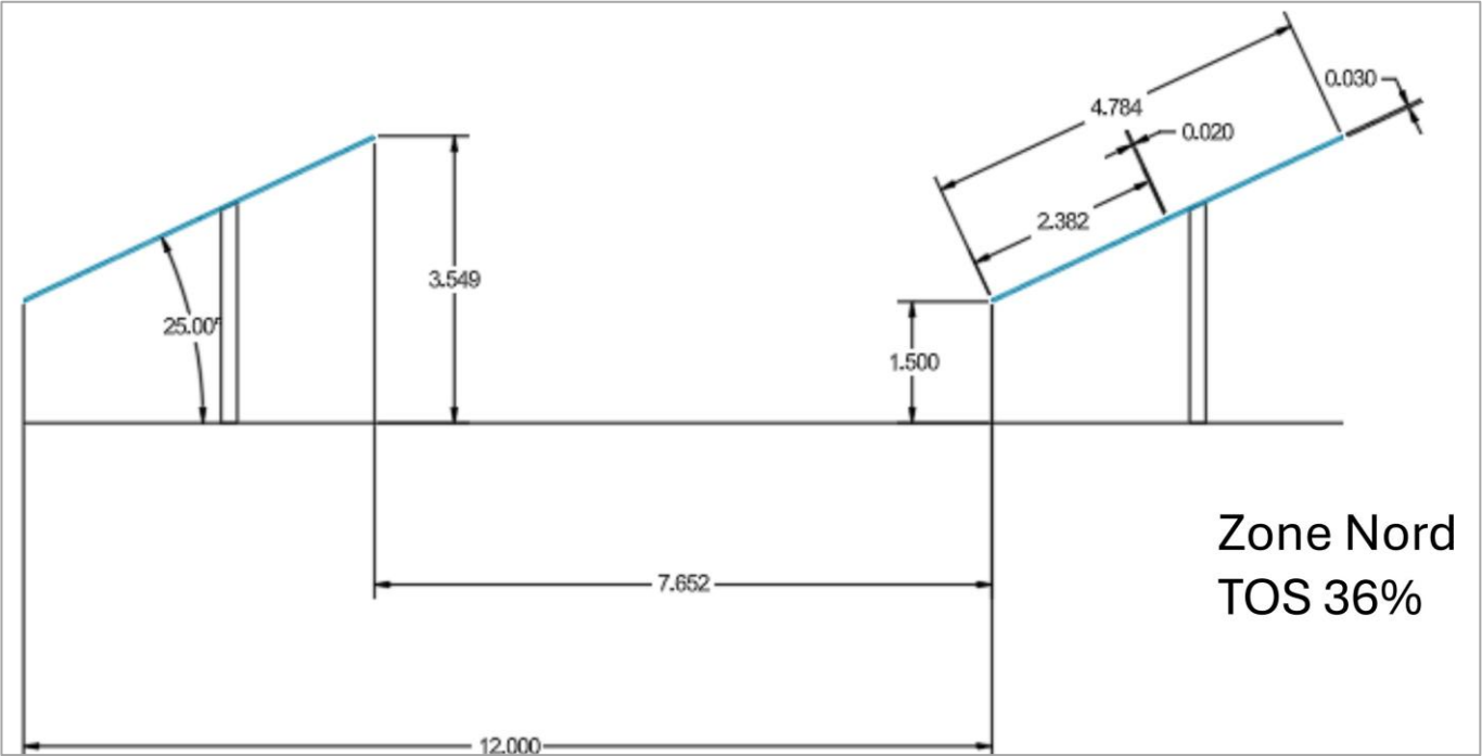
Figure 42 : Plan de façade d'une table photovoltaïque de profil en zone nord (Source : ESCOFI)
