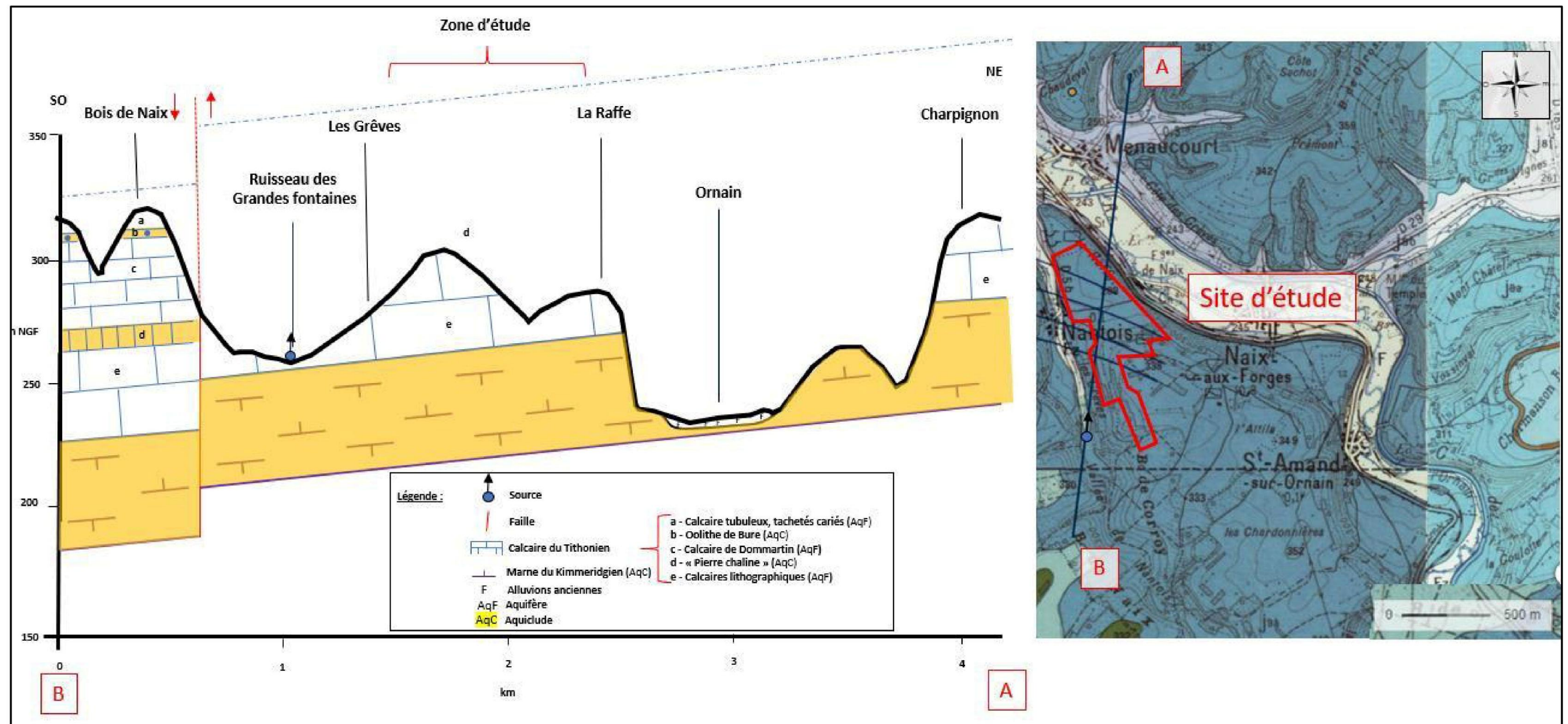
Figure 20 : Coupe géologique au droit du site d'étude (Source : BURGEAP)
