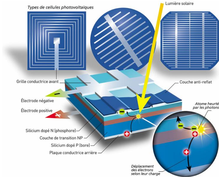
Figure 46 : Fonctionnement d'une cellule photovoltaïque (Source : Direct Energie)
