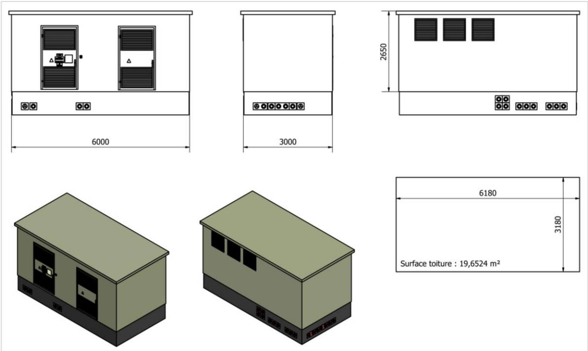
Figure 48 : Plan de façade d'un poste de transformation (Source : ESCOFI)
