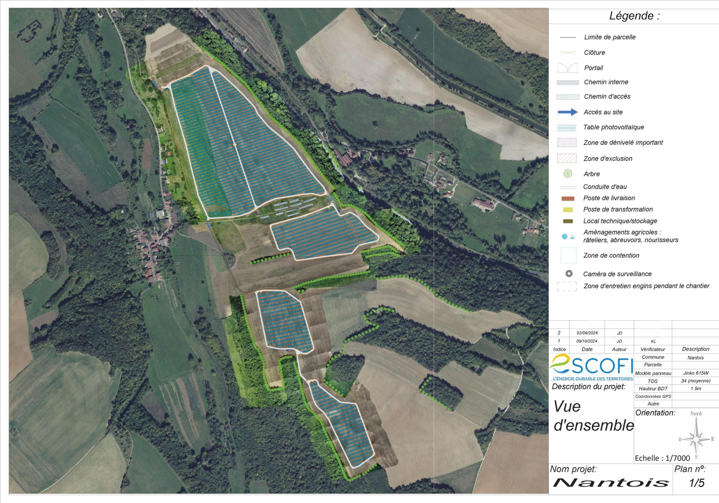
Figure 44 : Plan de masse du projet (Source : ESCOFI)
