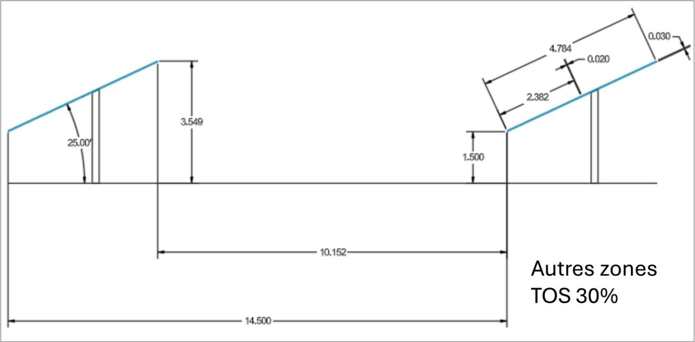
Figure 43 : Plan de façade d'une table photovoltaïque de profil dans les autres zones (Source : ESCOFI)
