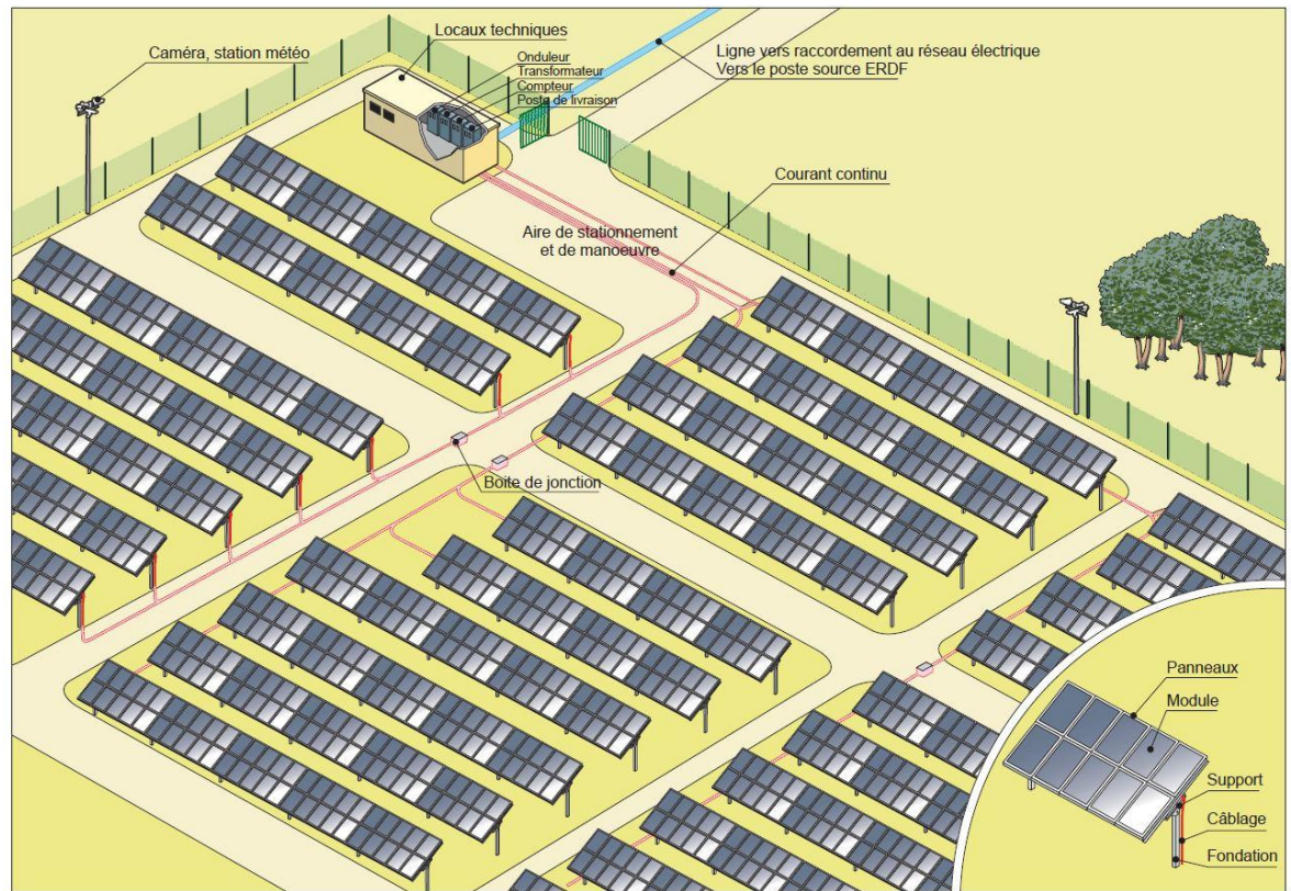
Figure 47 : Schéma d'une centrale photovoltaïque (Source : MEDDTL)
