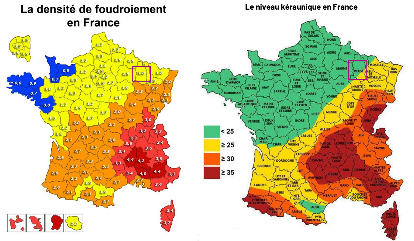
Carte 52 : Densité de foudroiement et niveau kéraunique en France
