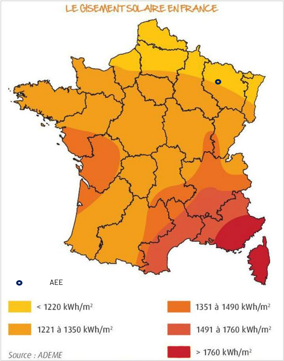
Carte 43 : Gisement solaire en France (Source : MEDDTL et ADEME)
