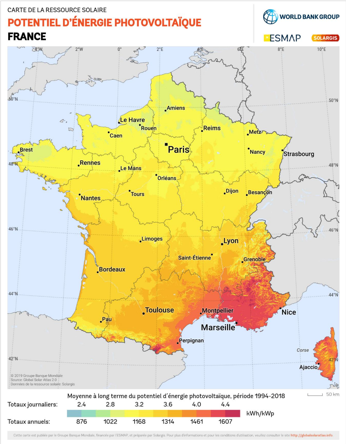
Carte 110 : Ensoleillement en France (Source : ESCOFI)
