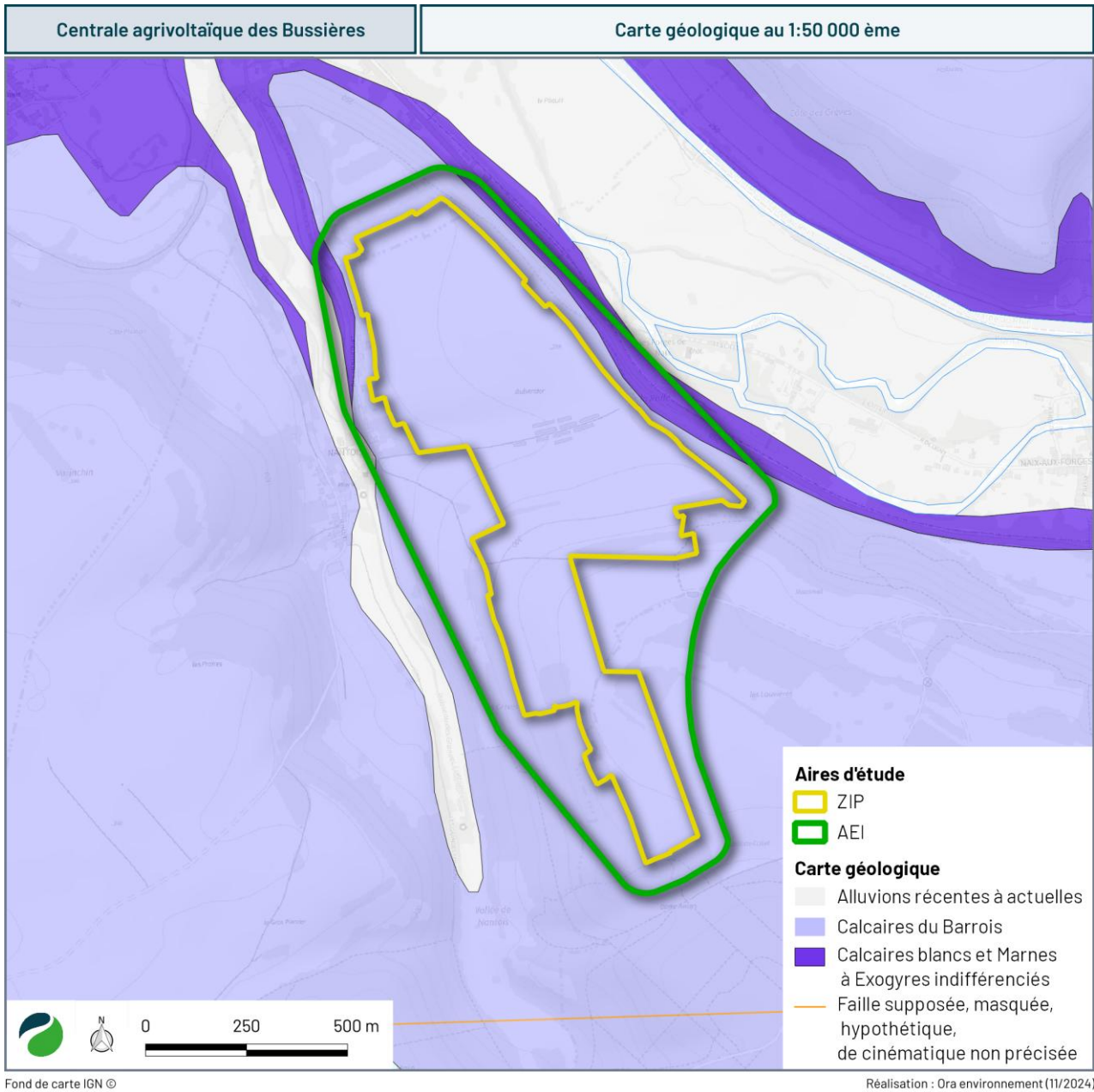
Carte 29 : Extrait de la carte géologique au 1 : 50 000 sur l’aire d’étude immédiate (Données : BRGM)
