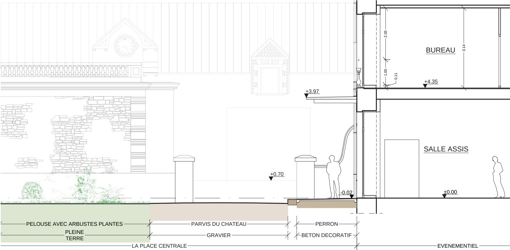
Coupe-profil sur le perron
