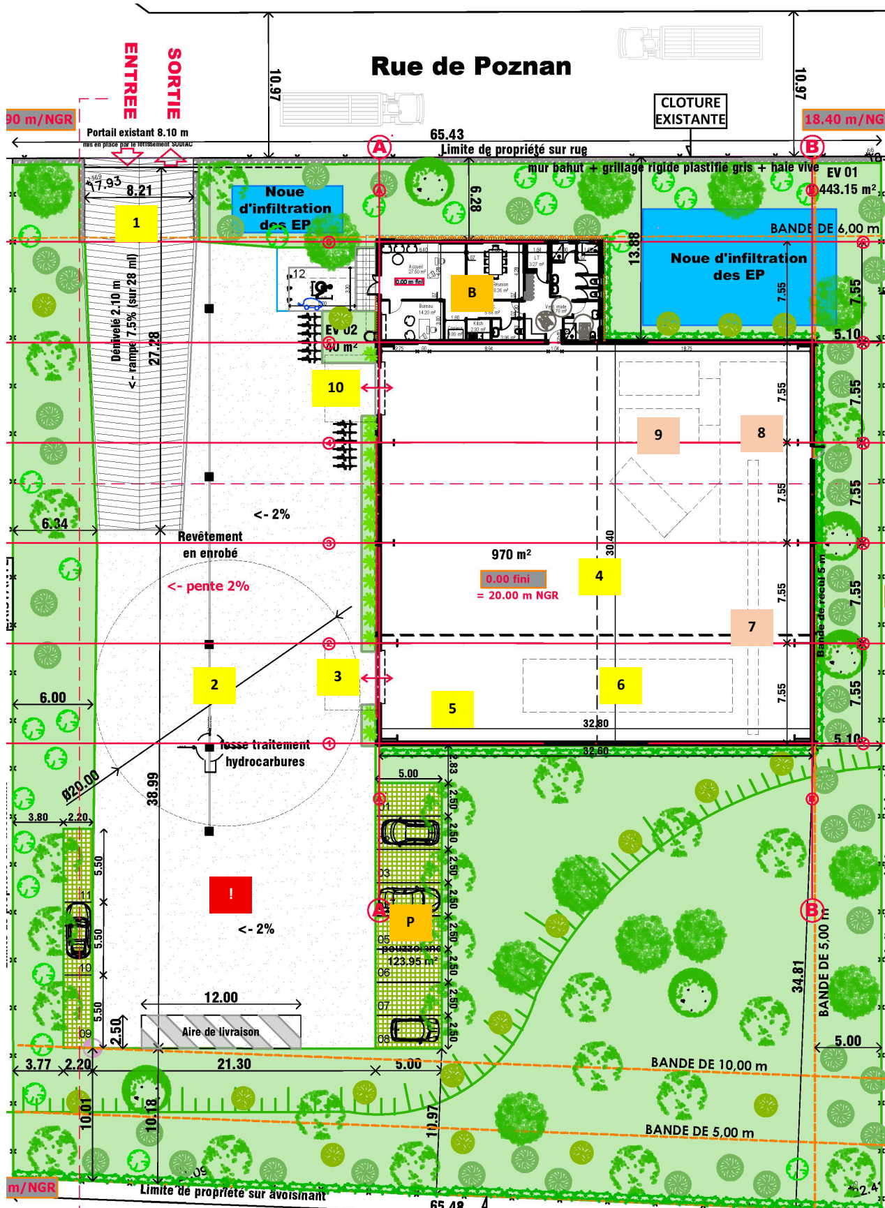
Figure 5 : Plan de masse de l'installation et zonages
