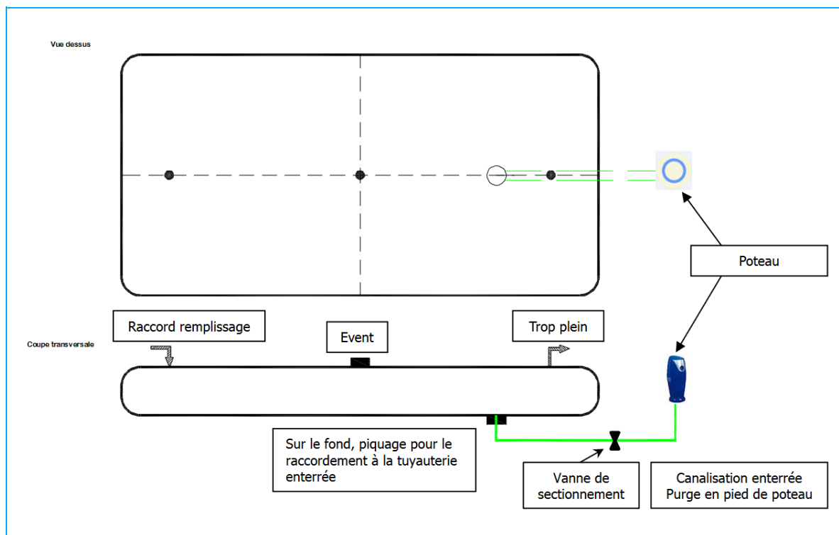
Figure 12 : Equipements du P.E.I interne bache souple rétention
