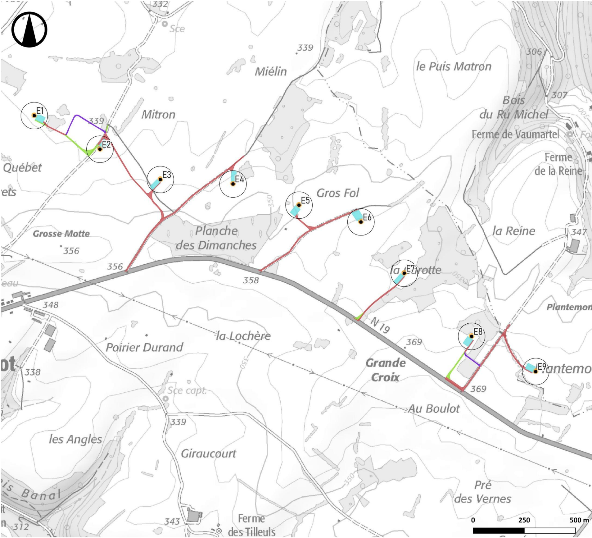
Carte 10 : Présentation de l'installation (éoliennes E1 à E9)
