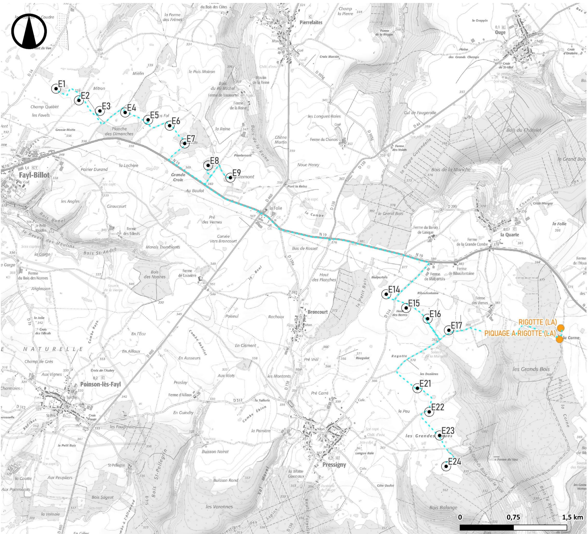
Carte 12 : Raccordement inter-éolien
