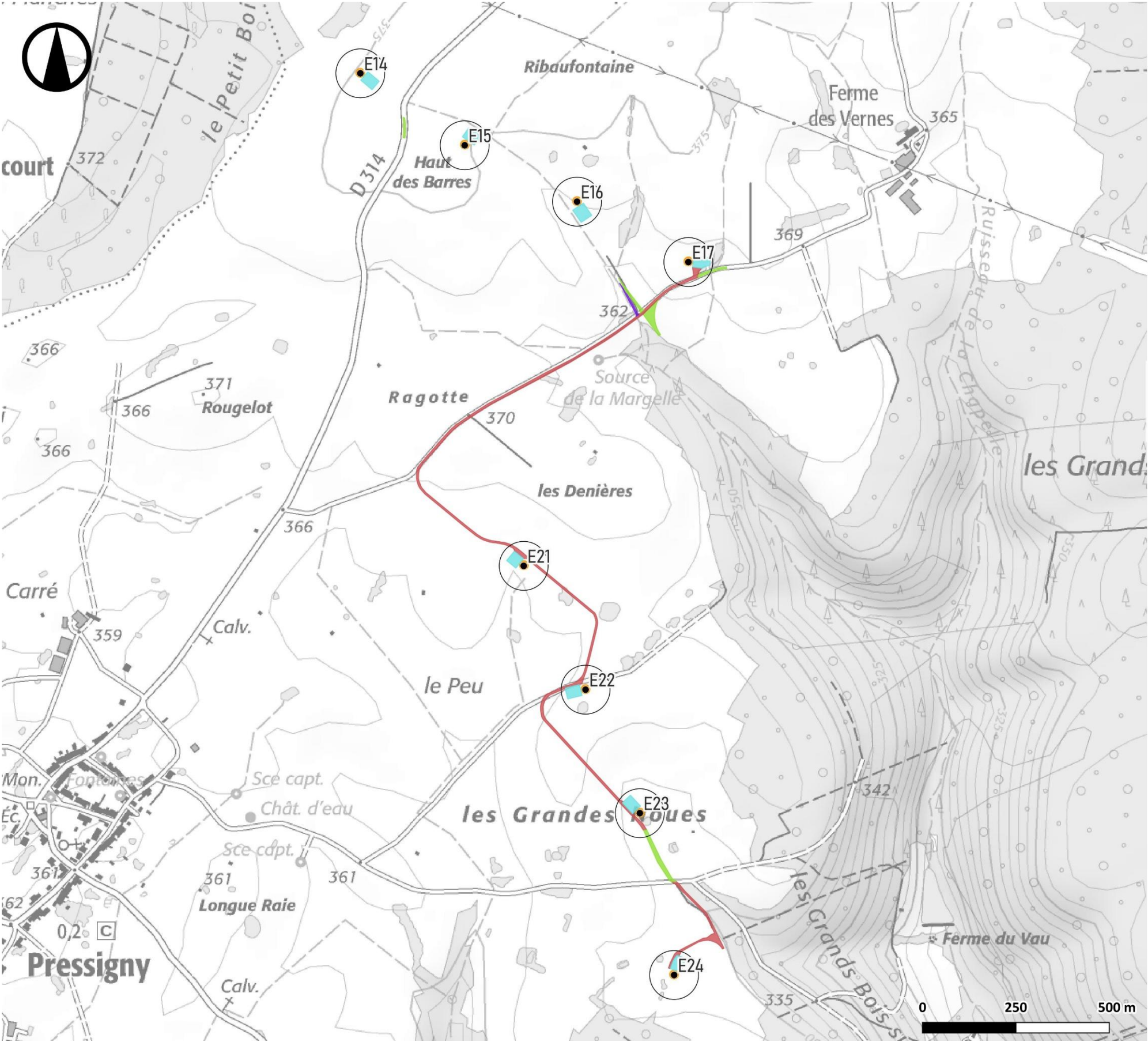
Carte 11 : Présentation de l'installation (éoliennes E14 à E24)
