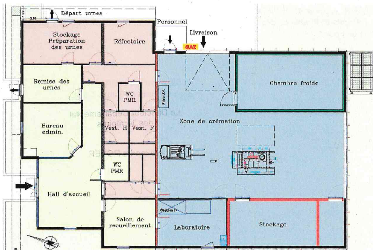
Figure 4 – Extrait du plan de masse bâtiment
