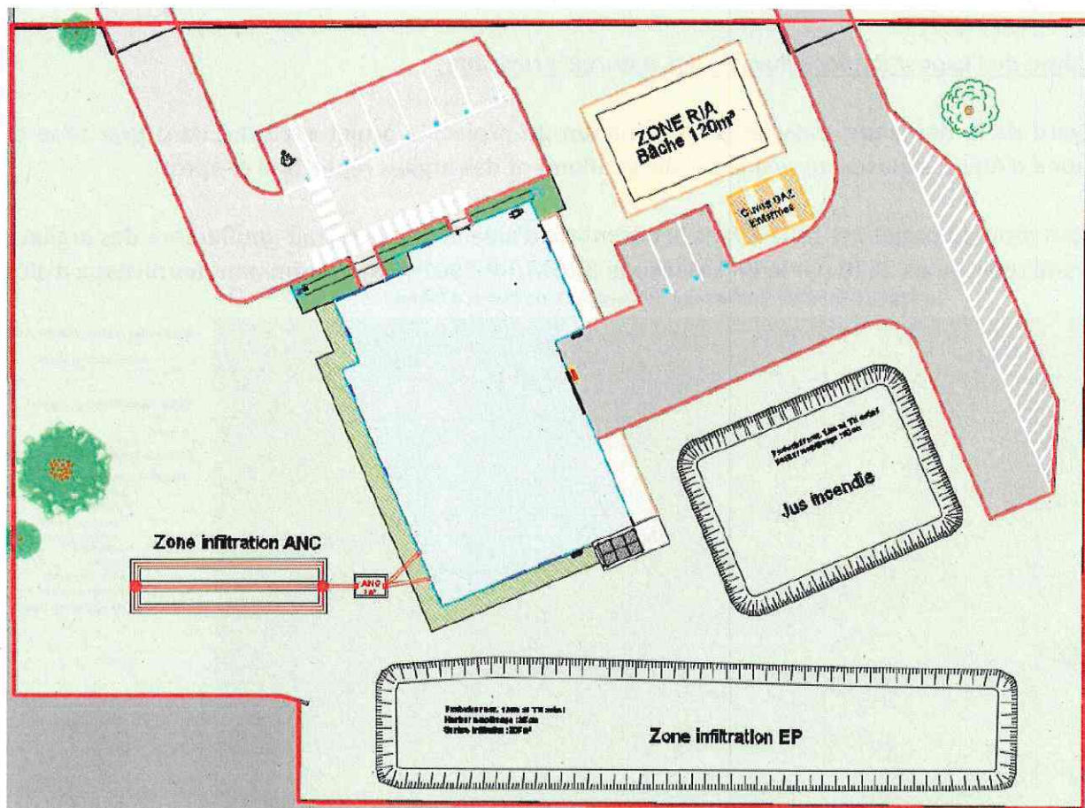
Figure 3 – Extrait du plan de masse AVP
