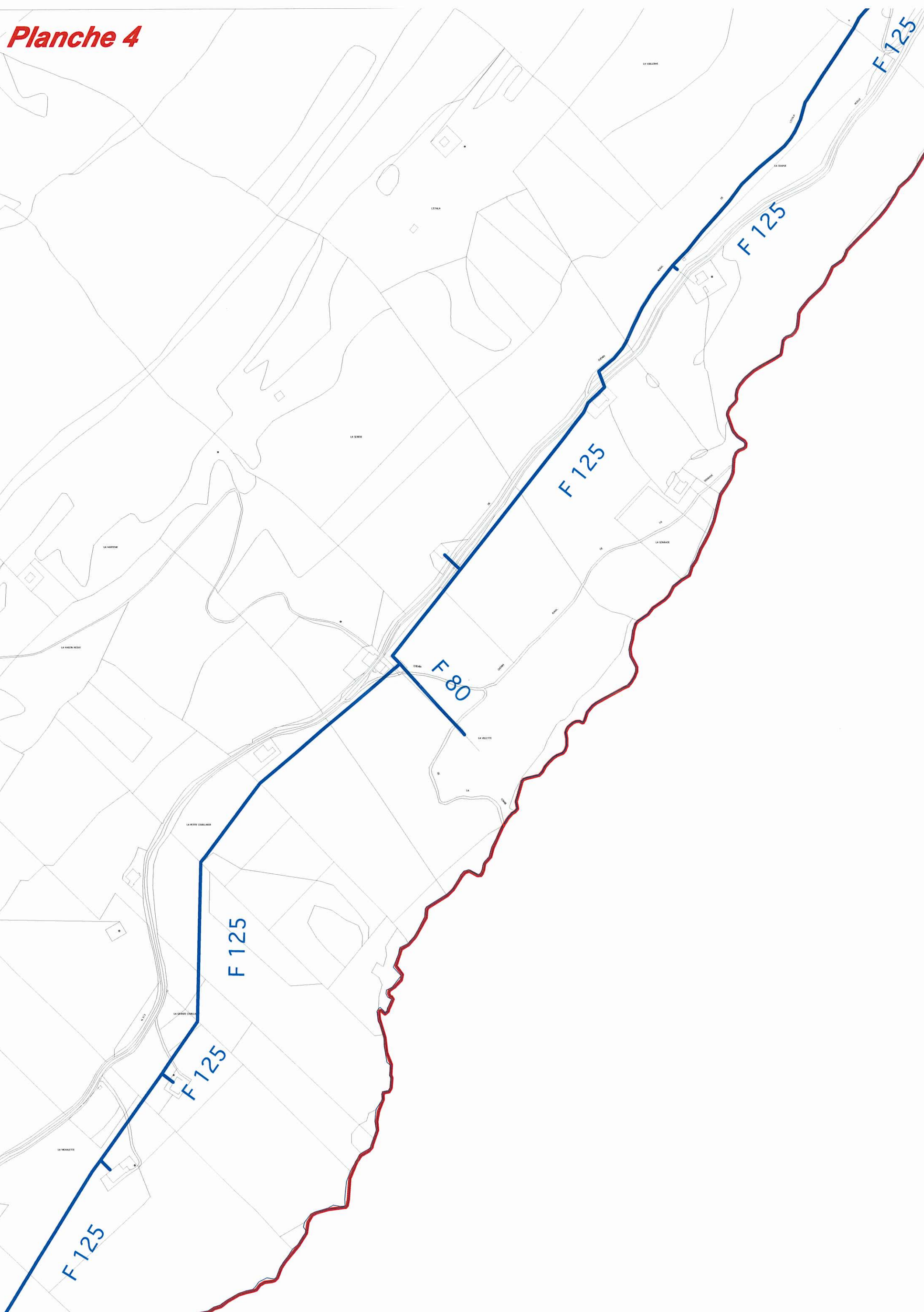
Commune de Lajoux - Réseaux d'eau potable d'après les plans dessinés par le Cabinet d'Etudes Marc Merlin en 1993 - Planche 4 - 1/5000°
