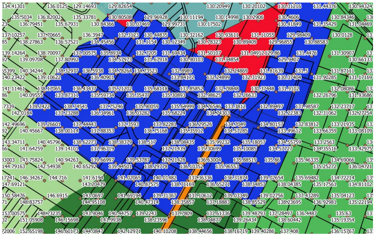
Relevé topographique de la zone
