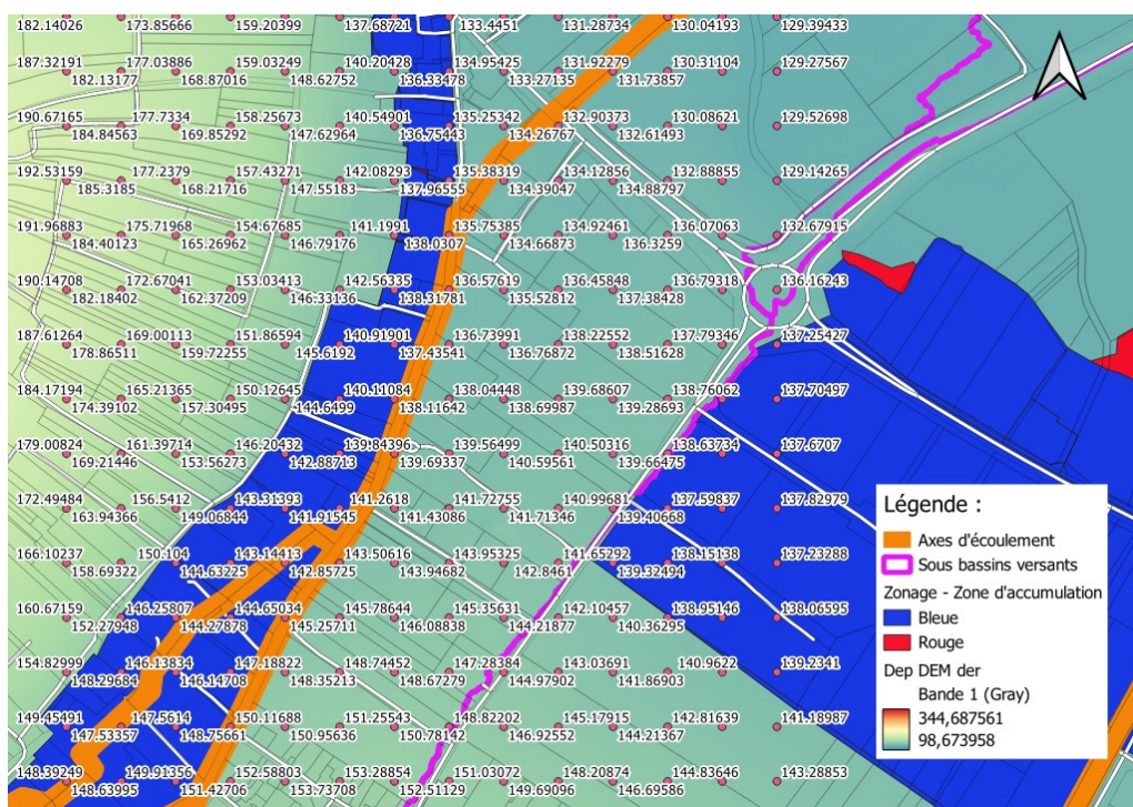
Relevé topographique de la zone
