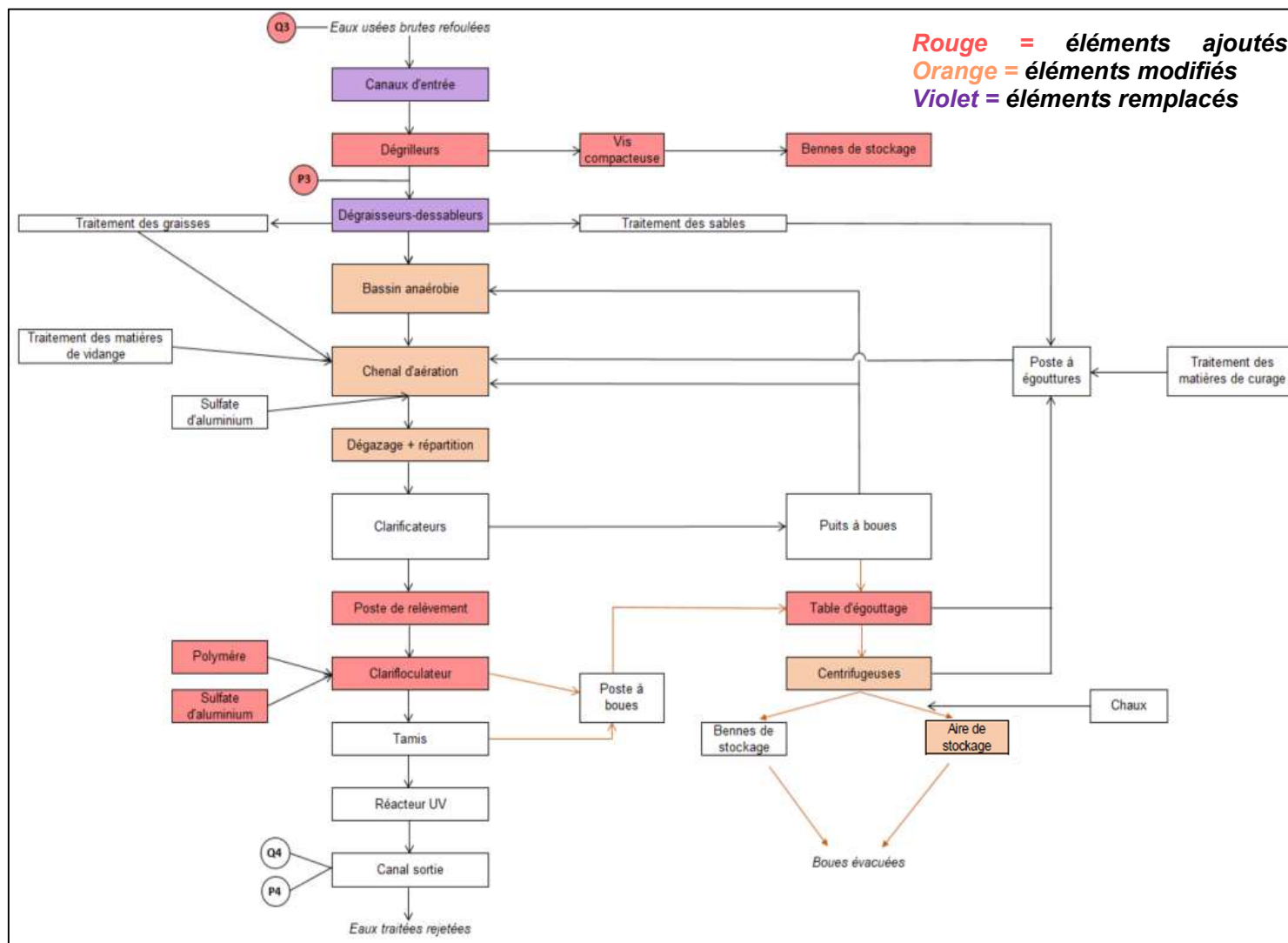
Figure 8 : Nouvelle filière de traitement de Lann Pont Houar
