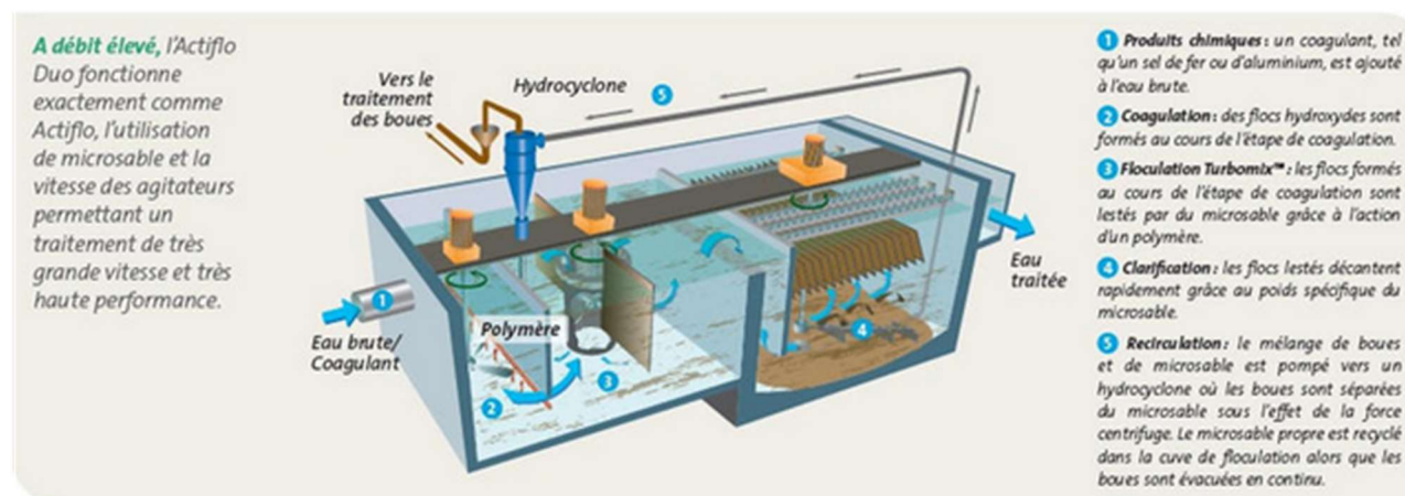
Figure 89 : Principe de fonctionnement de l' Actiflo Duo , développé par Veolia Water technologies
