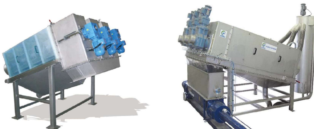
Figure 90 : Exemples de presses à vis
