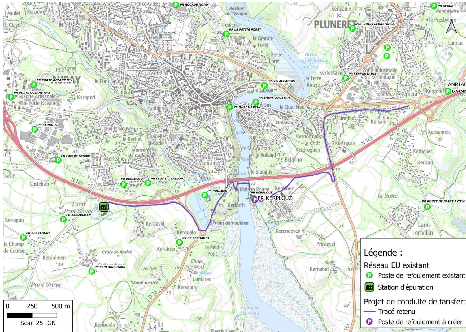
Figure 4 : Plan de situation générale du projet de sécurisation de la chaîne de transfert des eaux usées au 1/16 000ème
