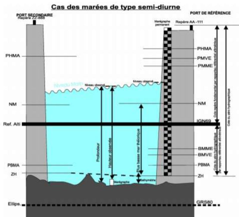
Figure 34 : Schéma récapitulatif des niveaux de marées
