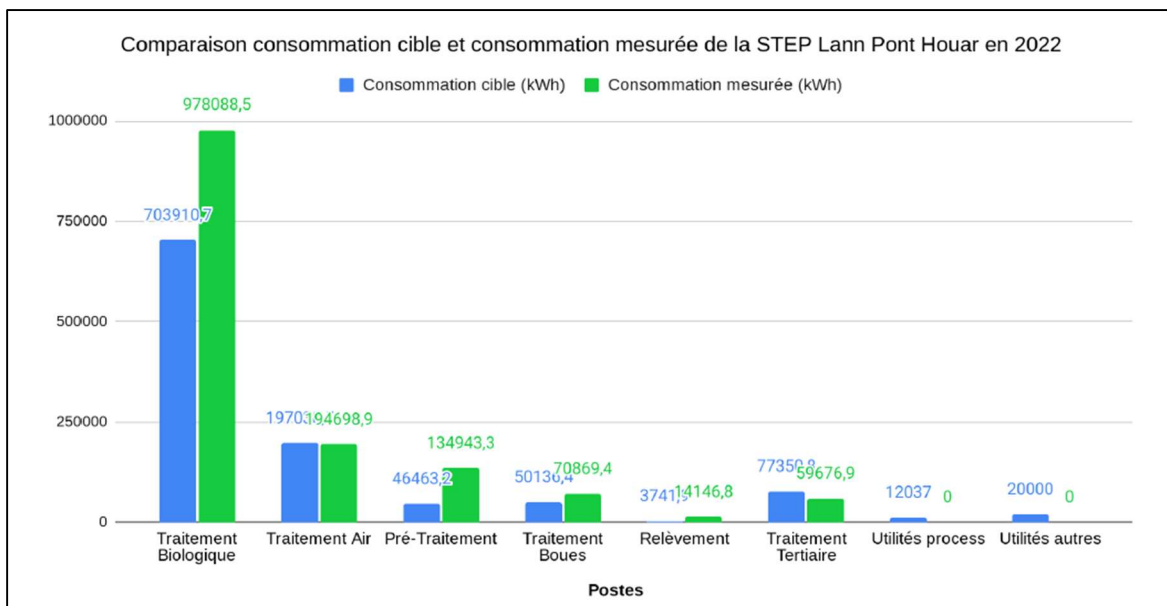
Figure 12 : Comparaison consommation cible et consommation mesurée de la STEP de Lann Pont Houar en 2022
