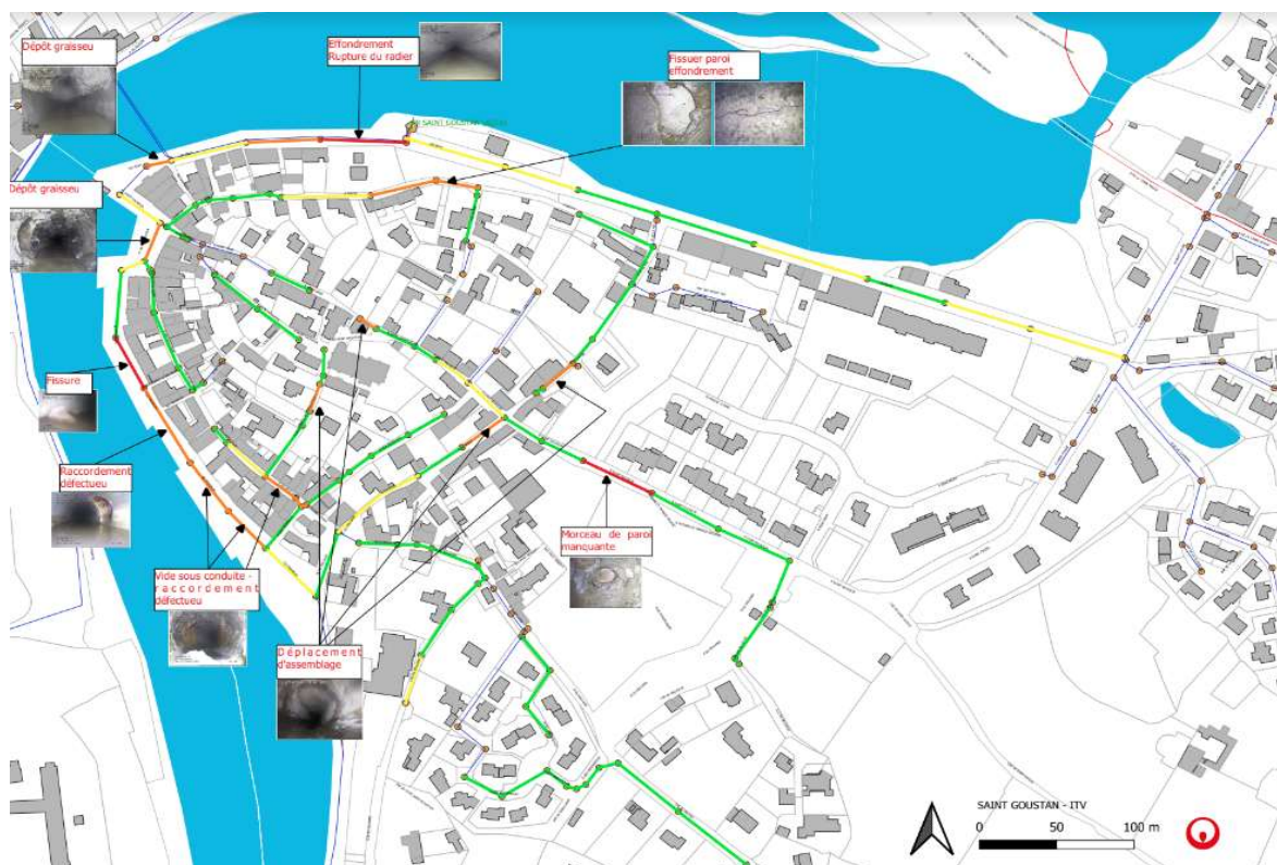
Figure 6 : Secteurs de Saint-Goustan ayant fait l'objet d'inspections caméra
