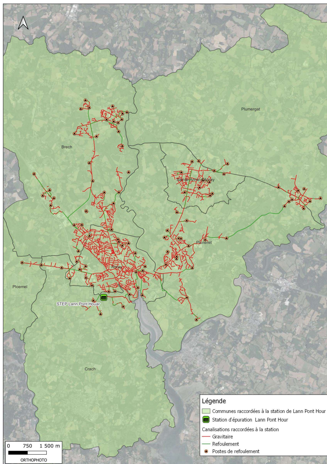
Figure 7 : Localisation du réseau de collecte à travers les communes raccordées à la STEP de Lann Pont Houar
