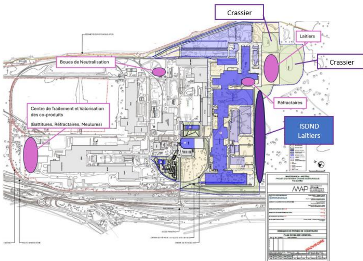
Figure 317: Plan de stockage des co-produits du site
