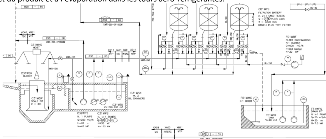
Figure 307: Extrait du PID du système de récupération des filtrations des hydrocarbures, filtration et clarification du circuit XB11
