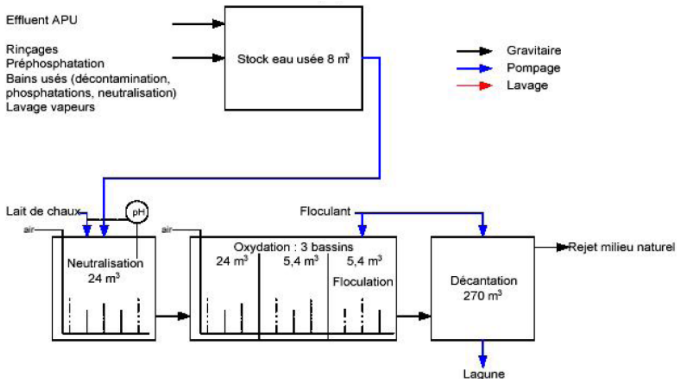
Figure 22 : Schéma de principe de la station de neutralisation
