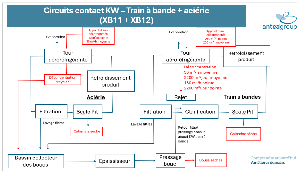
Figure 305: Schéma simplifié du circuit contact (KW)
