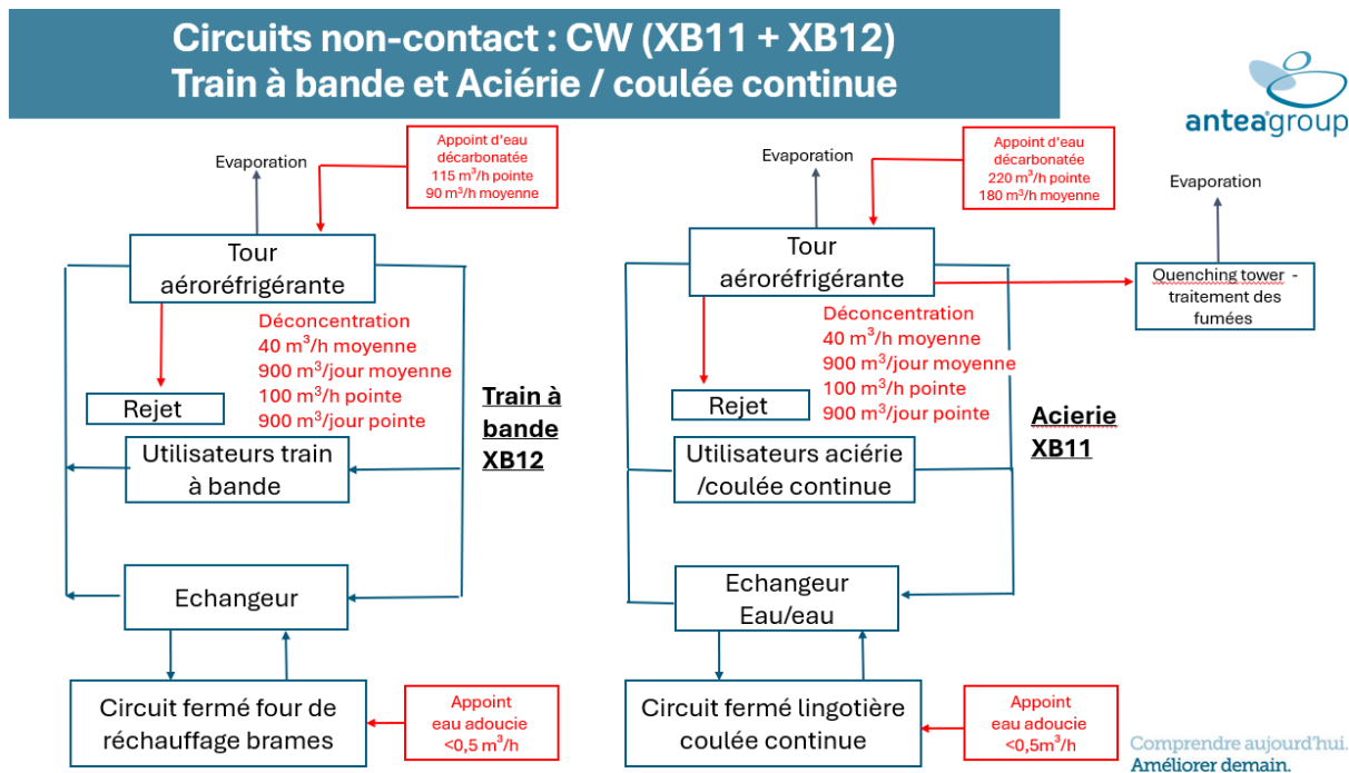
Figure 304: Schéma simplifié du circuit non-contact (CW)
