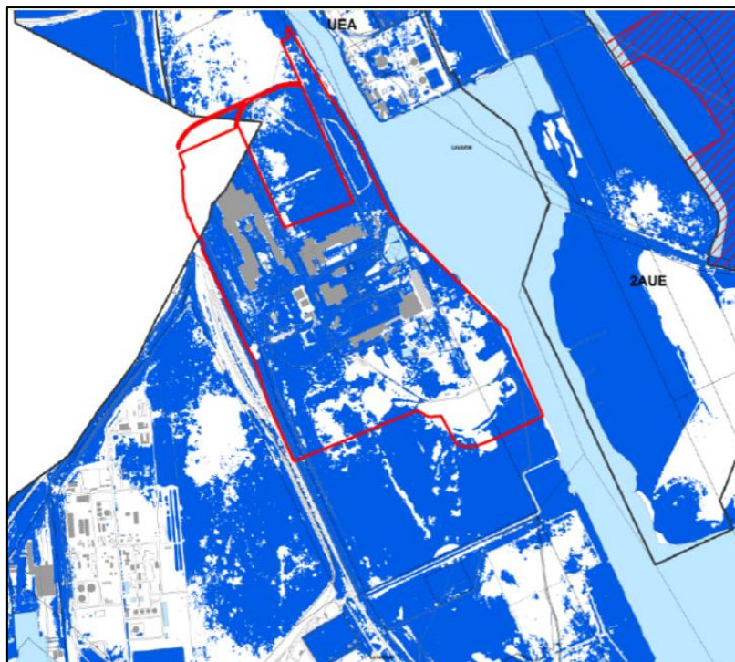
Figure 344: Cartographie indicative des espaces situés sous la cote 2,40 m NGF concernés par la prise en compte du risque submersion marine
