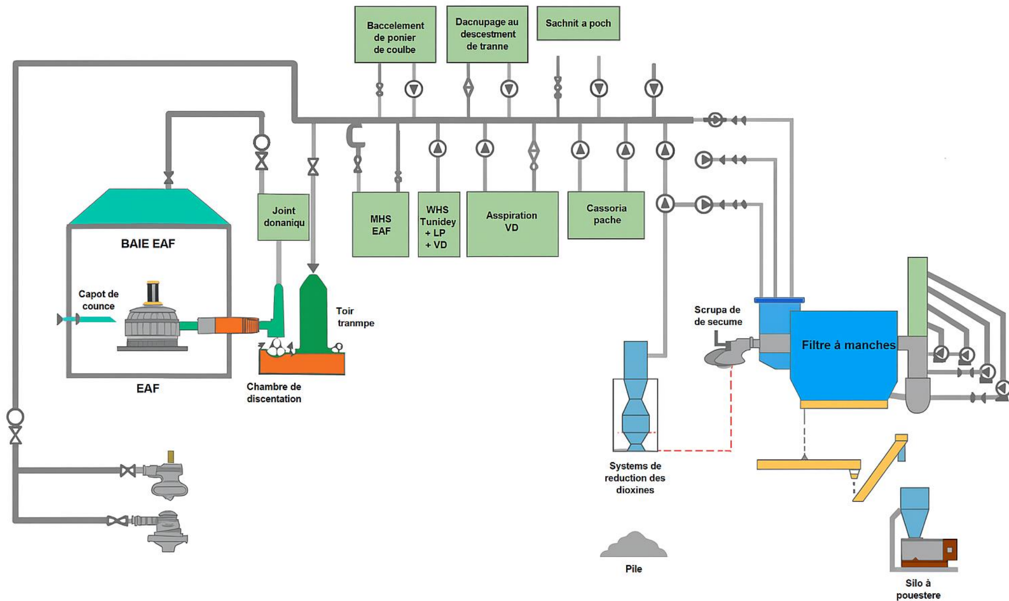
Figure 33: Schéma du procédé de traitement des fumées
