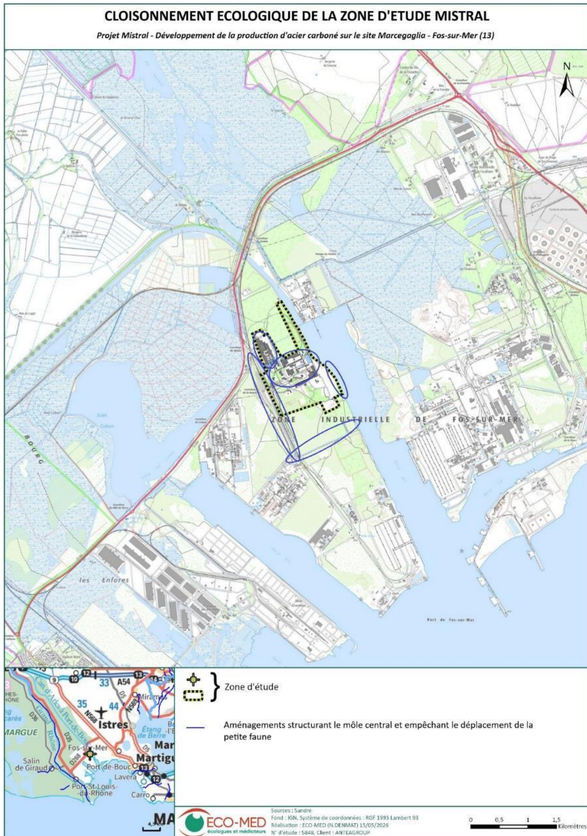
Figure 254 : Localisation des secteurs aménagés rendant le déplacement de la petite faune impossible
