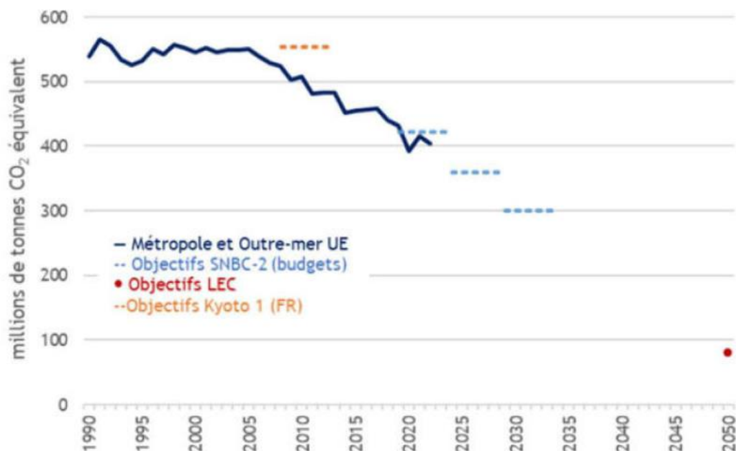
Figure 144: Graphique de l'évolution des émissions dans l'air de CO 2 , depuis 1990 en France (Métropole et outre-mer UE)
