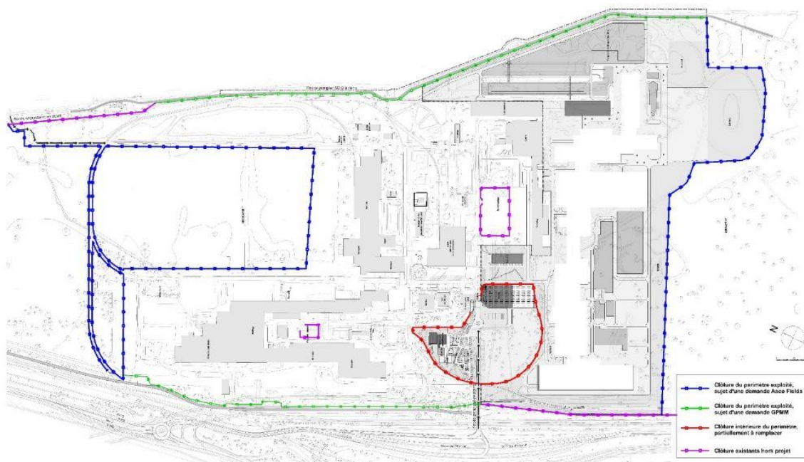
Figure 268: Clôtures du projet Mistral
