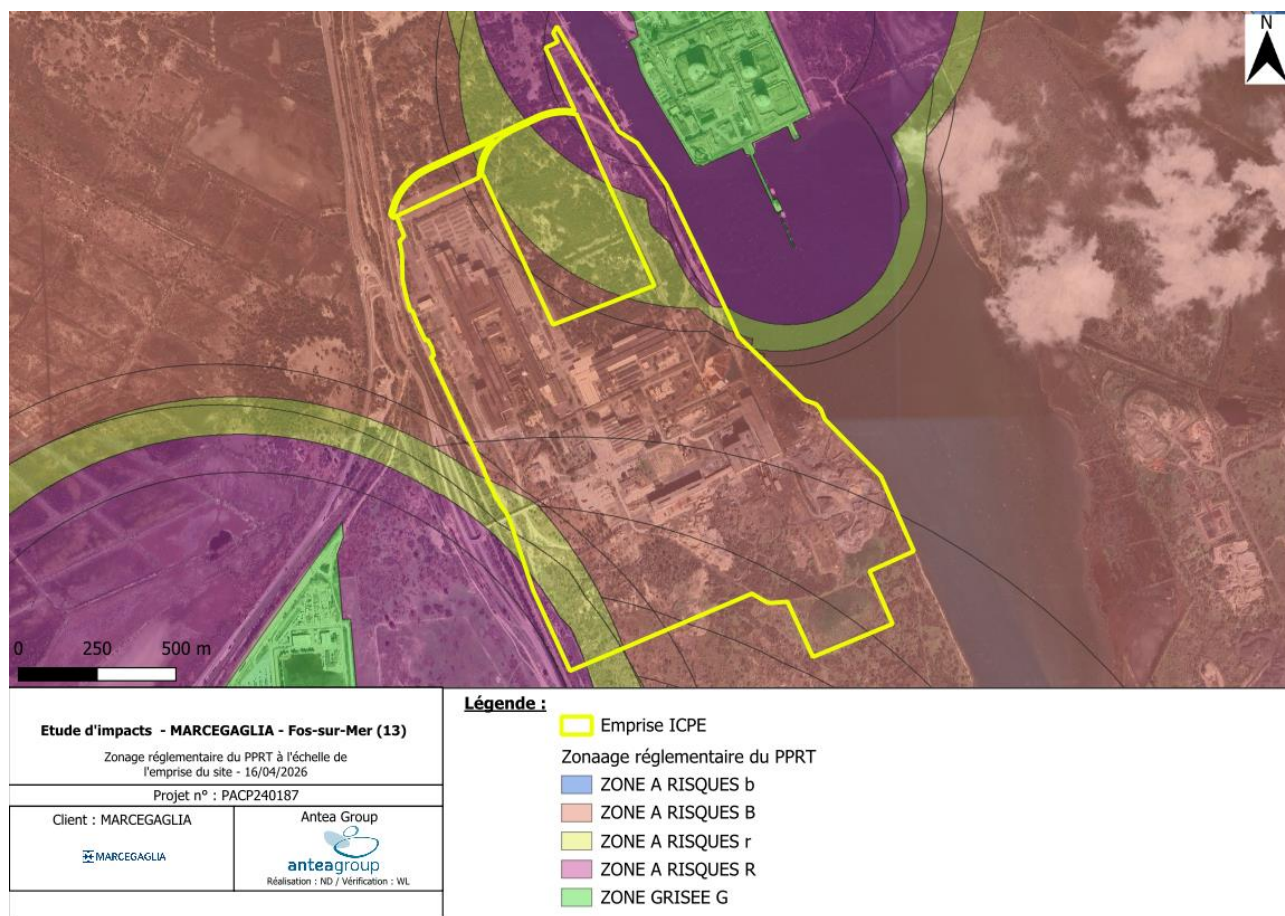
Figure 163 : Zonage du PPRT FOS-OUEST (échelle site MARCEGAGLIA)
