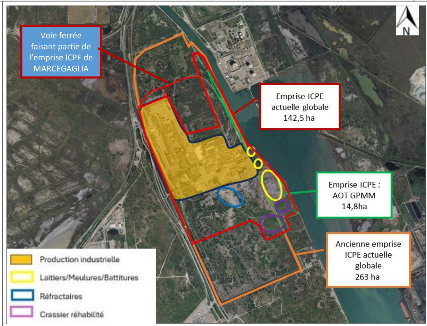
Figure 12 : Installations actuelles du site autorisé
