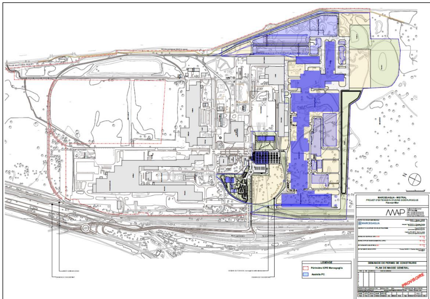
Figure 29 : Plan de masse du site projeté
