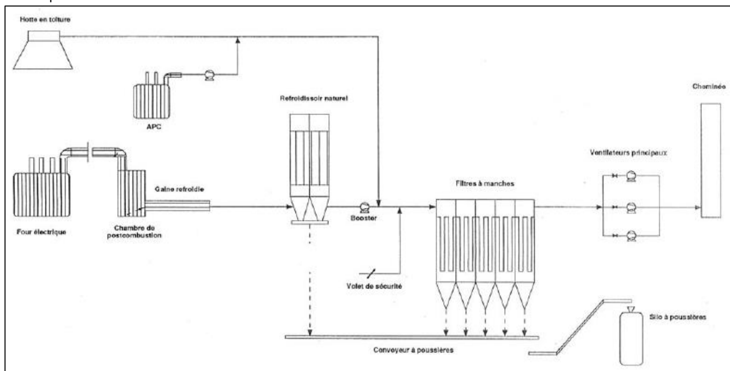
Figure 138 : Unité de dépoussiérage de l'aciérie
