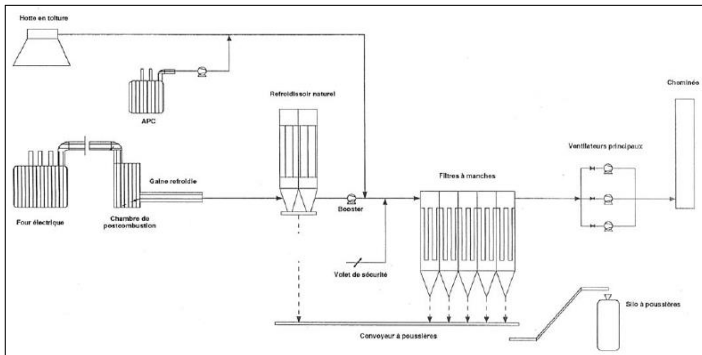
Figure 16 : Unité de dépoussiérage de l'aciérie
