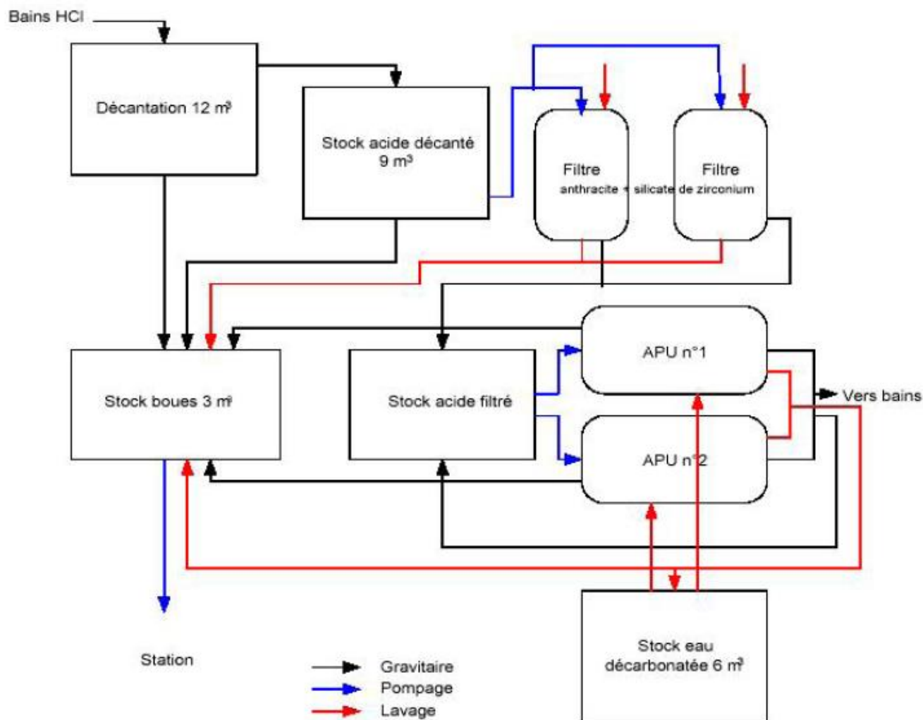
Figure 21 : Unité de régénération HCl
