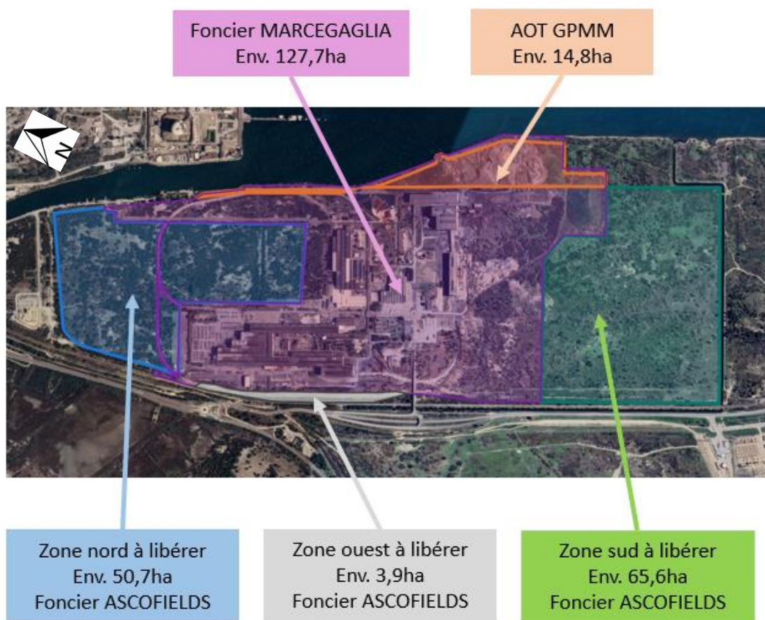
Figure 5: Nouvelle emprise ICPE du site MARCEGAGLIA
