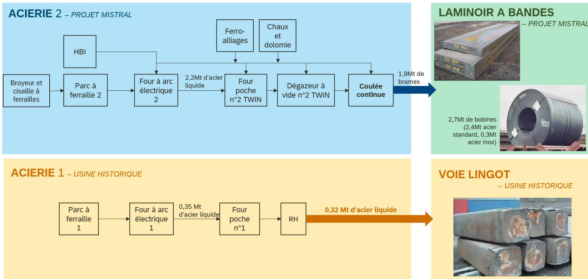
Figure 31: Processus général de la future usine
