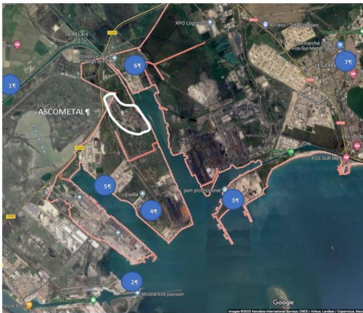
Figure 325: Localisation des points de mesures des retombées atmosphériques
