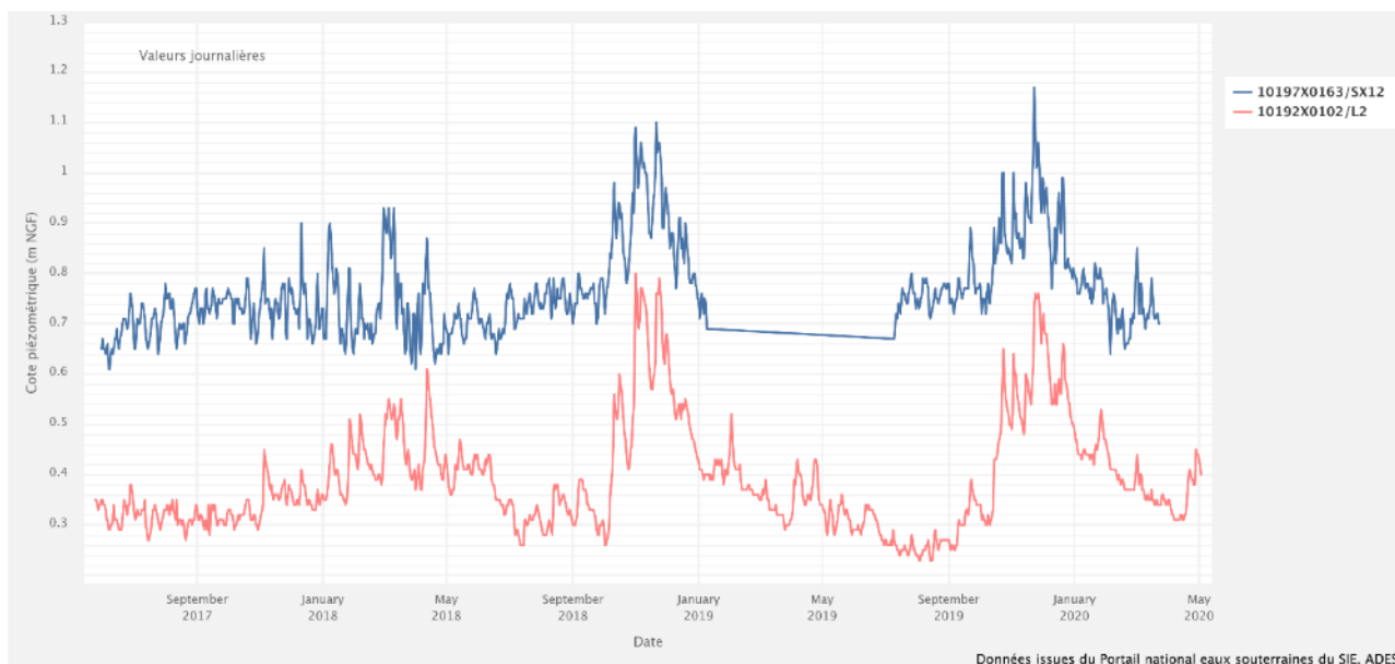
Figure 70 : Suivi piézométrique de SX12 et L2 entre le 25/05/2017 et le 03/05/2020
