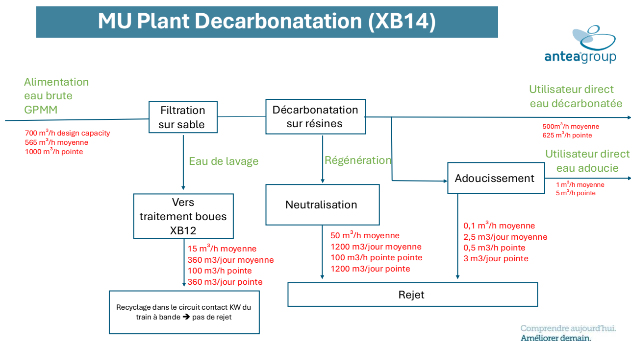
Figure 303: Schéma simplifié du traitement de l'eau brute
