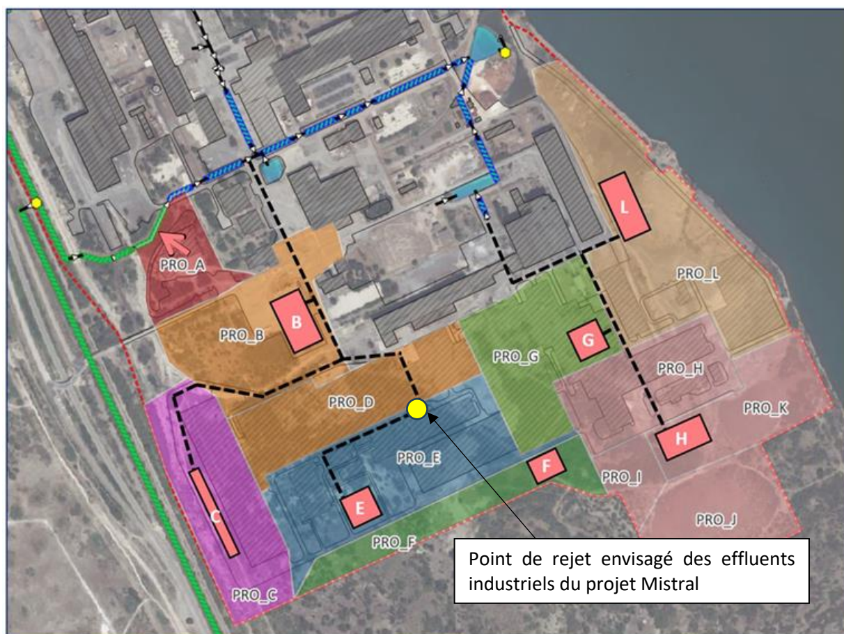
Figure 306: Point de rejet envisagé du rejet commun des eaux de refroidissement contact et non contact du projet Mistral
