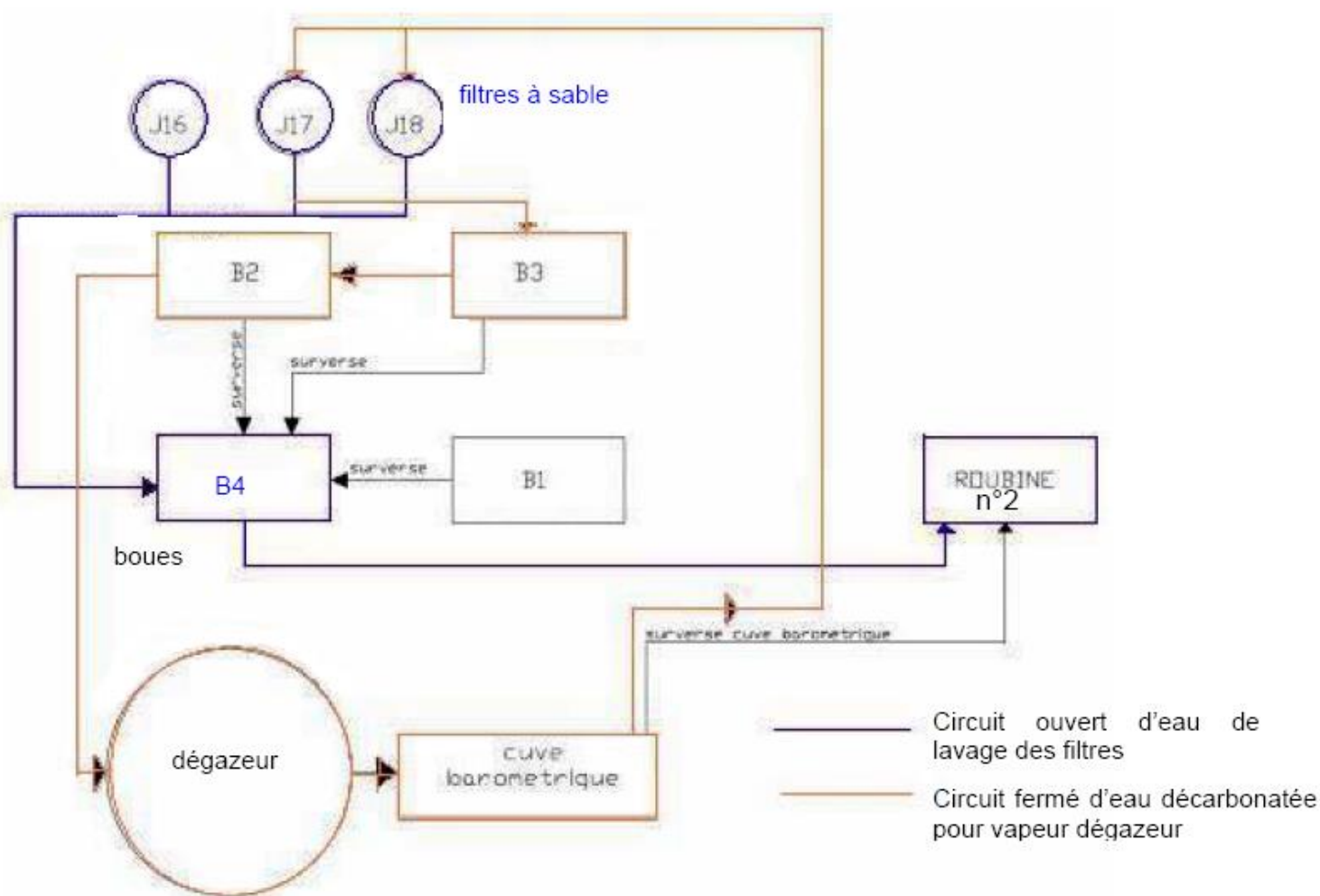
Figure 19 : Circuit de mise sous vide du dégazeur RH
