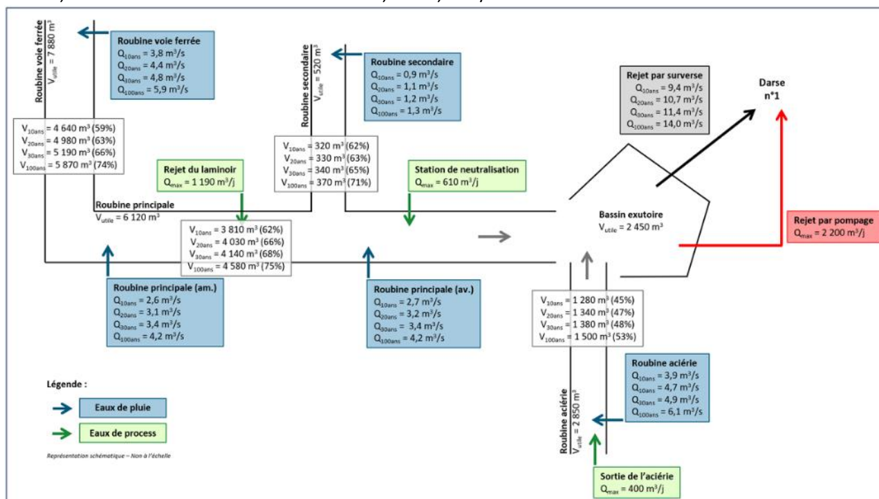
Figure 294: Schéma synoptique du diagnostic hydraulique en situation actuelle du réseau structurant d'eau de l'usine de Fos-sur-Mer
