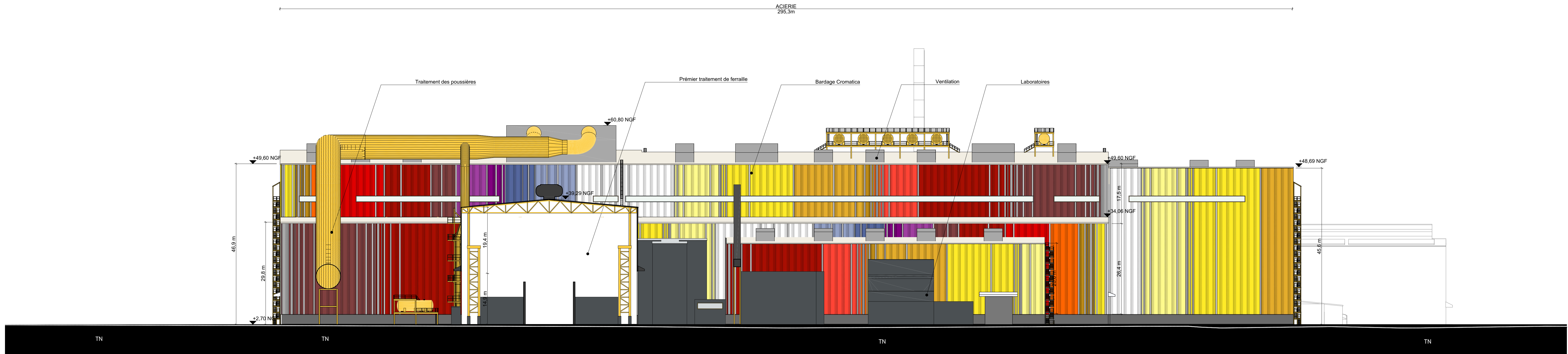
FAÇADE EST 2 - 1/500
