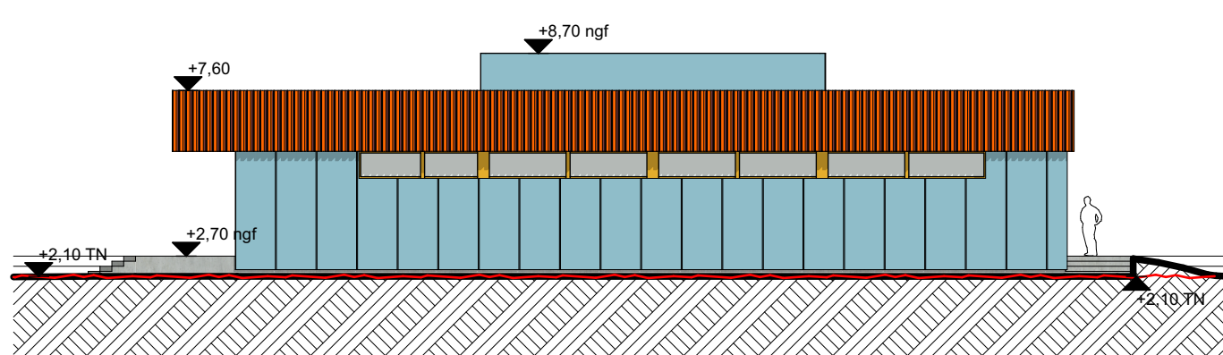
FAÇADE SUD - 1/200
