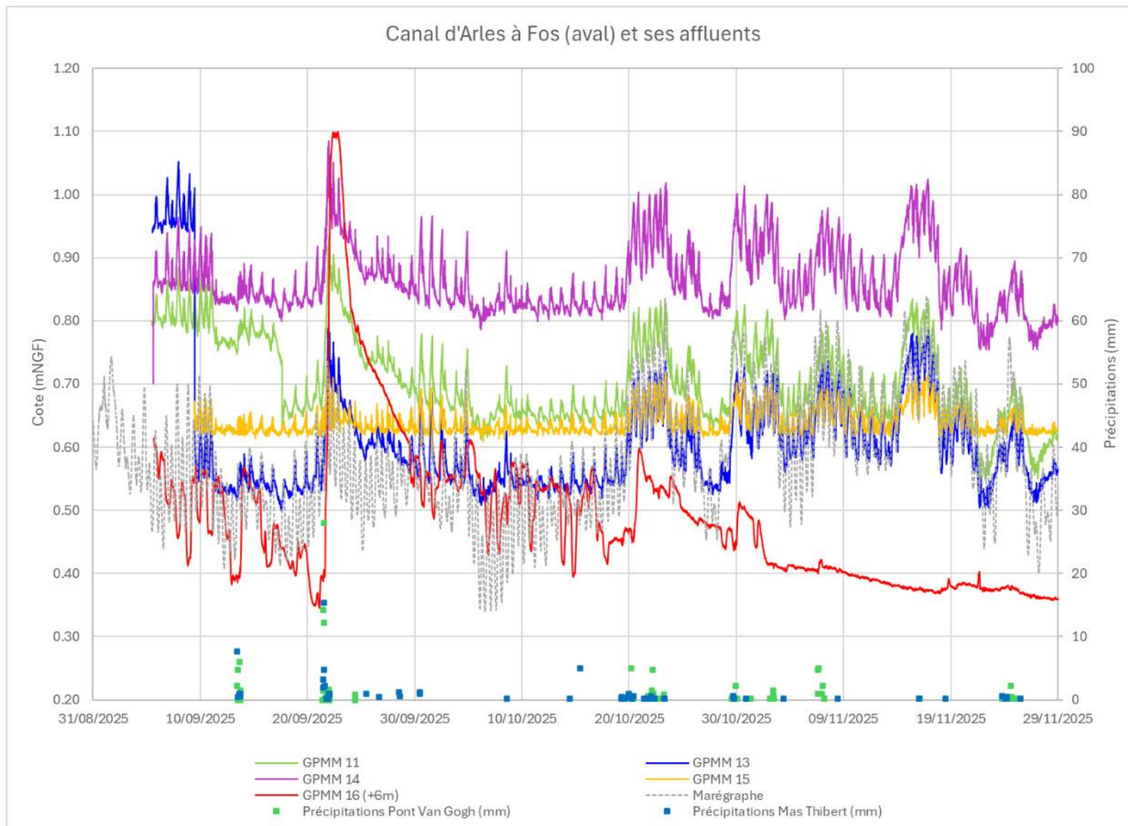
Figure 13 : Hauteurs du Canal d'Arles à Fos et de ses affluents en aval de Mas Thibert
