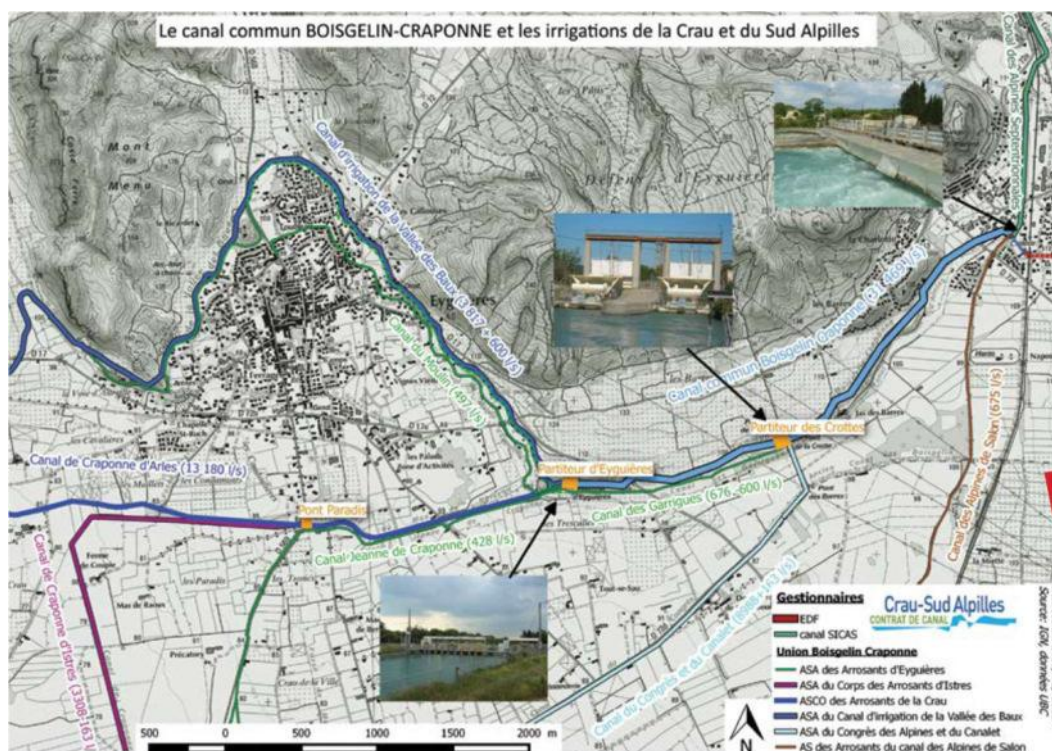
Figure III-3 : Prise d'eau des canaux de la plaine de Crau dans la via le canal Commun Boisgeline-Craponne (source : Guide pratique de l'arrosant, 2015).
