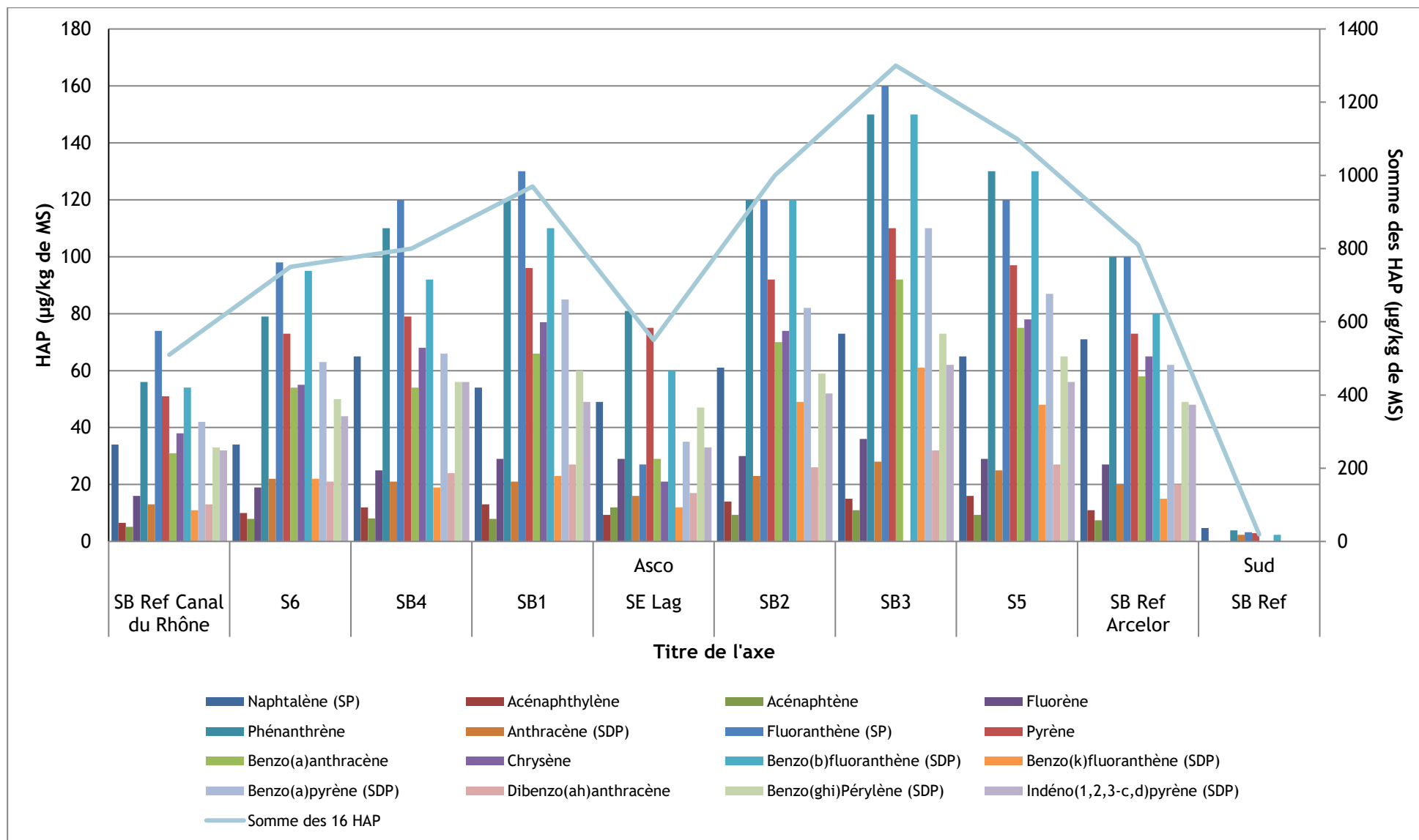
Figure 61. Profils de contaminations des sédiments par les hydrocarbures aromatiques polycycliques en 2018
