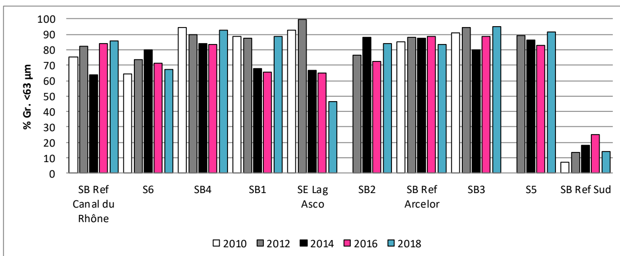
Figure 27. Pourcentage de fraction fine au niveau des stations de suivi de 2010 à 2018 (Safege, In Vivo, Setec)
