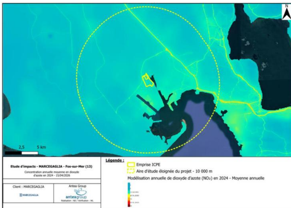
Figure 26 : NO 2 – Moyenne annuelle 2024 en µg/m³
