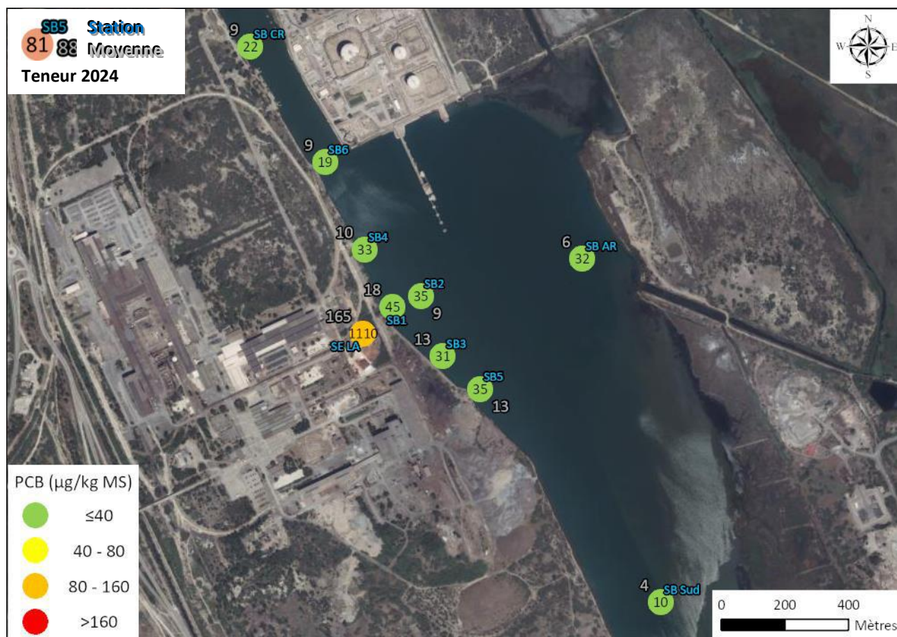
Figure 83 : Localisation des stations, teneurs des PCB mesurées en 2024 et moyennes
