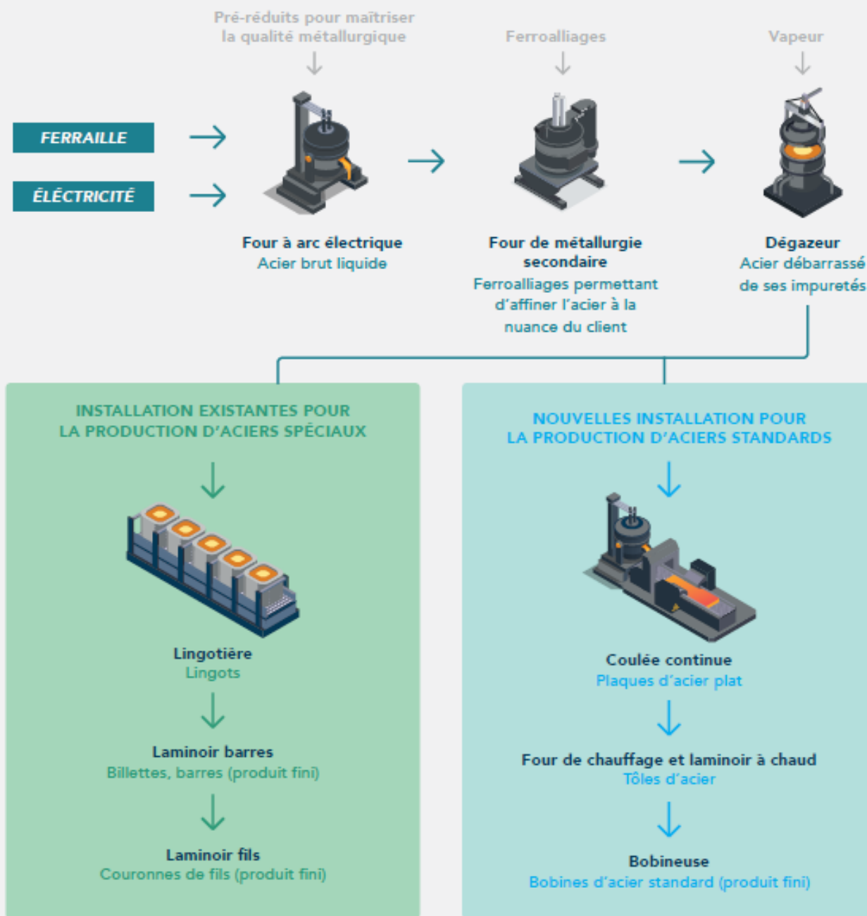
Figure 21: Les étapes de fabrication
