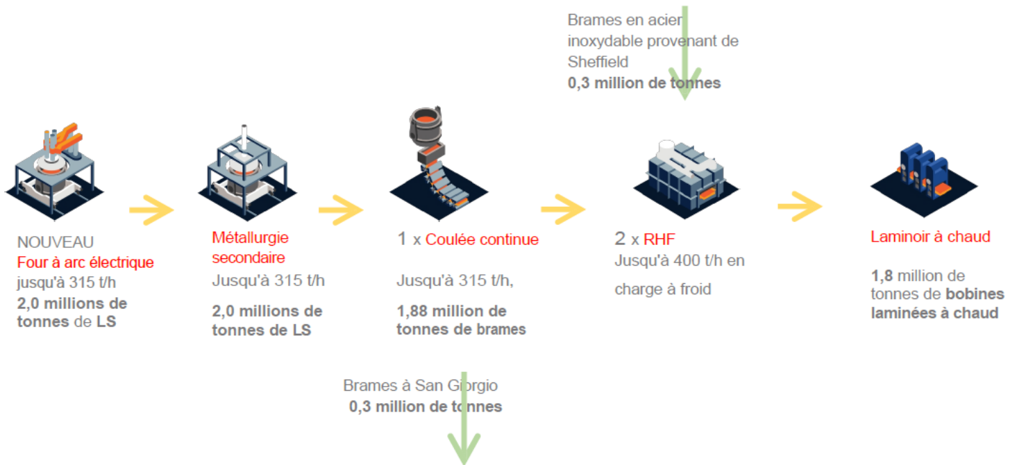
Figure 20: Schéma des flux de matériaux
