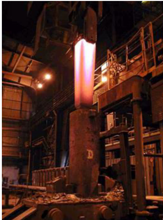
Photo 3 : Démoulage d'un lingot
