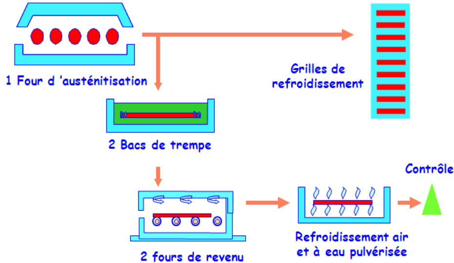
Figure 26 : Ligne de traitement thermique avec four d'austénitisation
