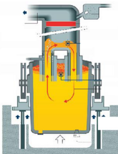
Figure 17 : Dégazeur RH
