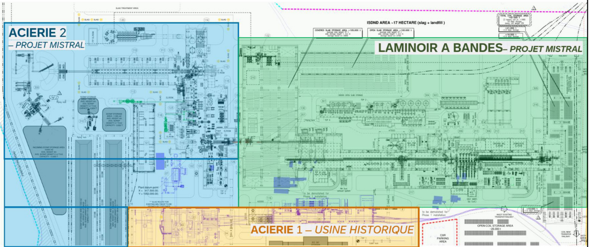
Figure 42: Agencement général de la nouvelle usine
