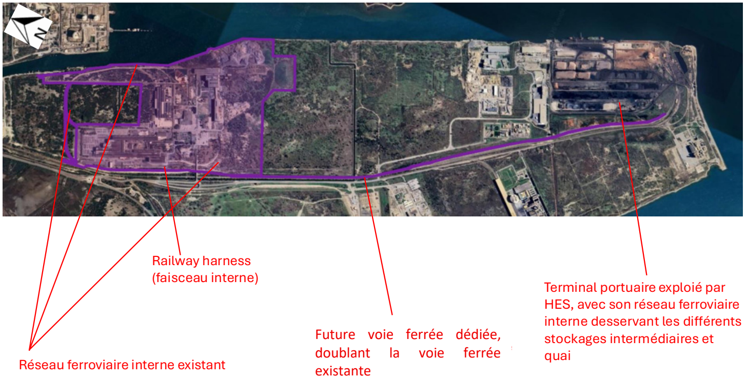
Figure 10: Tracé de la voie ferrée vers le terminal HES
