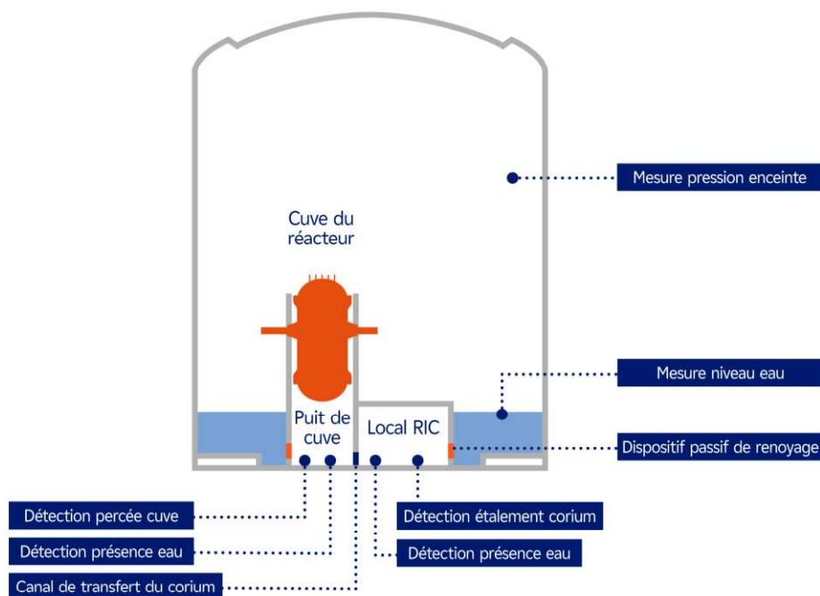
Figure 11. Illustration de la mesure de niveau d'eau dans les puitsards du bâtiment réacteur et de la détection de l'étalement du corium dans le local d'instrumentation du cœur (RIC)
