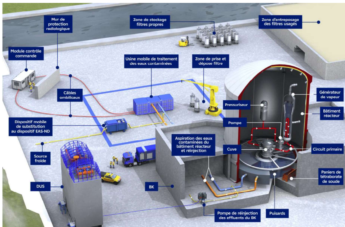
Figure 10. Illustration des dispositions « Lignes fixes pour le traitement des eaux contaminées dans le bâtiment réacteur et modules mobiles de traitement des eaux contaminées », « Mise en œuvre d'une ligne d'injection et d'un dispositif mobile de substitution au dispositif EAS-ND », « Réinjection des effluents du bâtiment combustible dans le bâtiment réacteur », « Mise en place de paniers de tétraborate de diSodium décahydraté dans les puisards du bâtiment réacteur »
