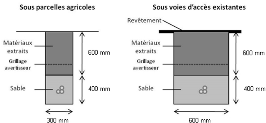
Figure 24 : Coupes générales des tranchées destinées à l'enfouissement des lignes électriques
