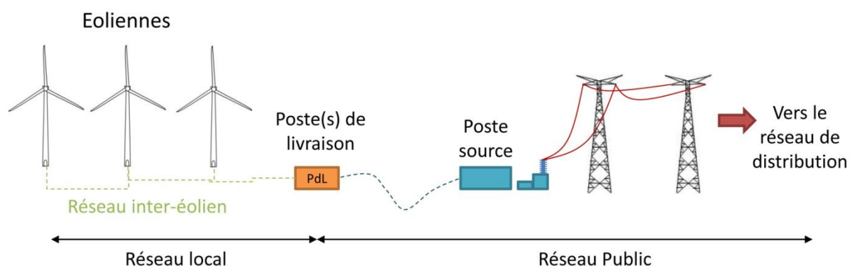
Figure 23 : Schéma de raccordement électrique d'un parc éolien
