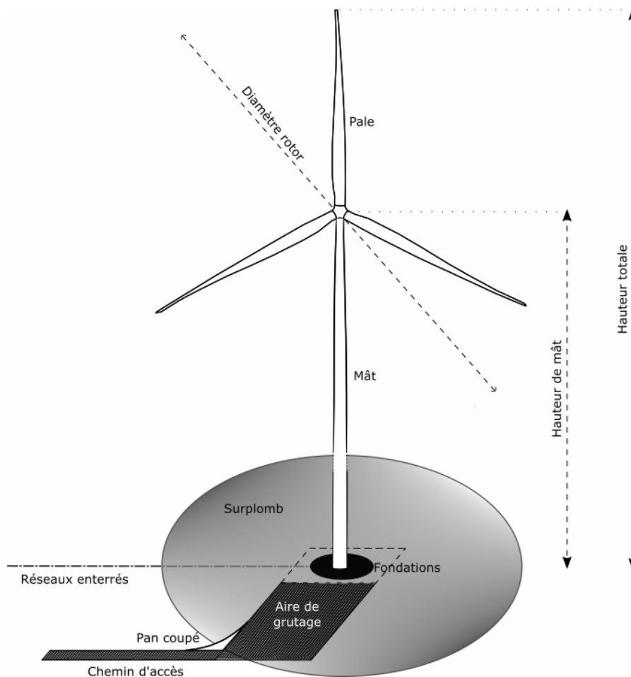
Figure 21 : Illustration des emprises au sol d'une éolienne (source : Eolise)
