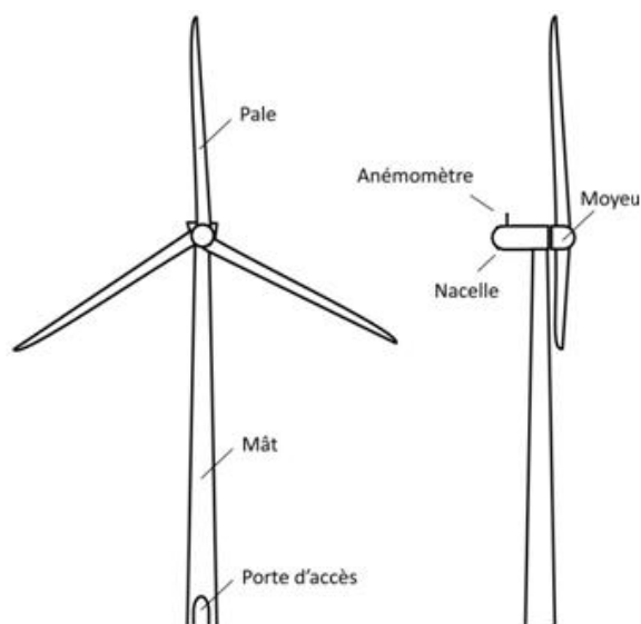
Figure 19 : Schéma simplifié d'un aérogénérateur
