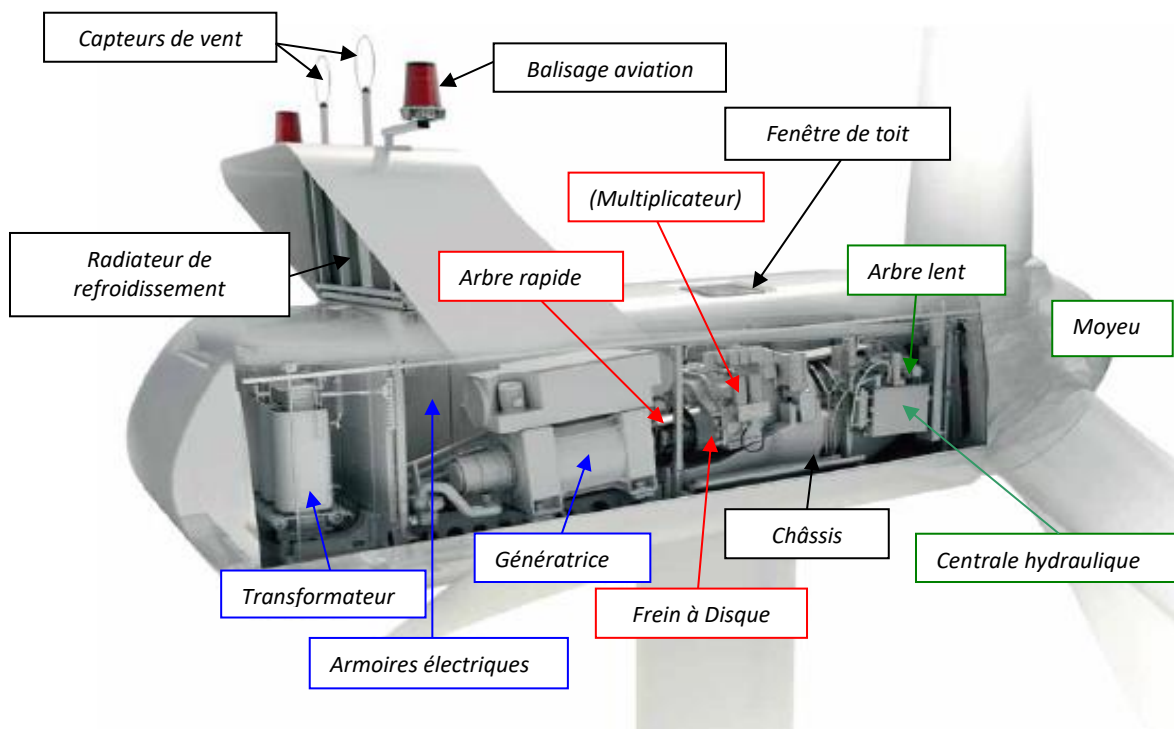
Figure 20 : Composants d'une nacelle (Source : Vestas)
