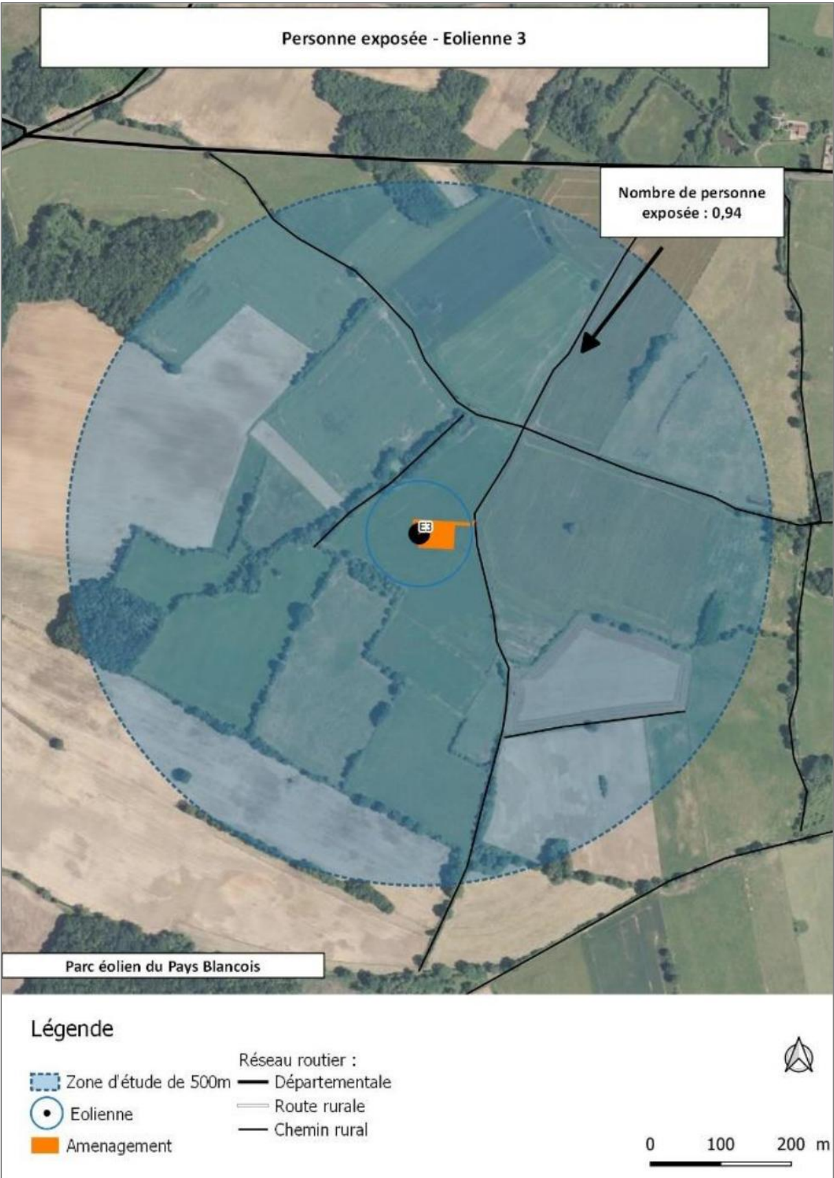
Carte 159 : Personnes exposées au niveau de l'éolienne E3 (Source : EOLISE)
