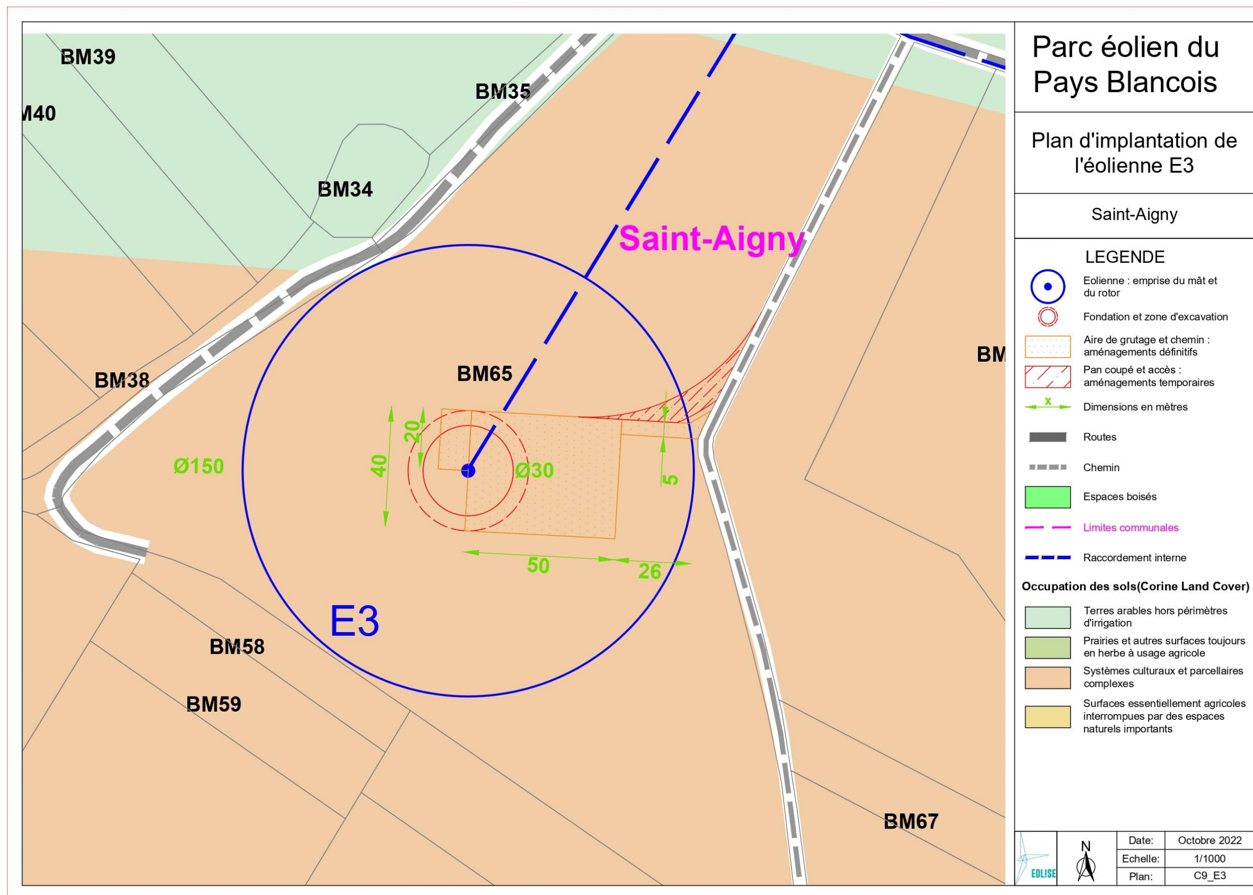
Carte 124 : Plan de masse de l'éolienne E3 (Source : EOLISE)
