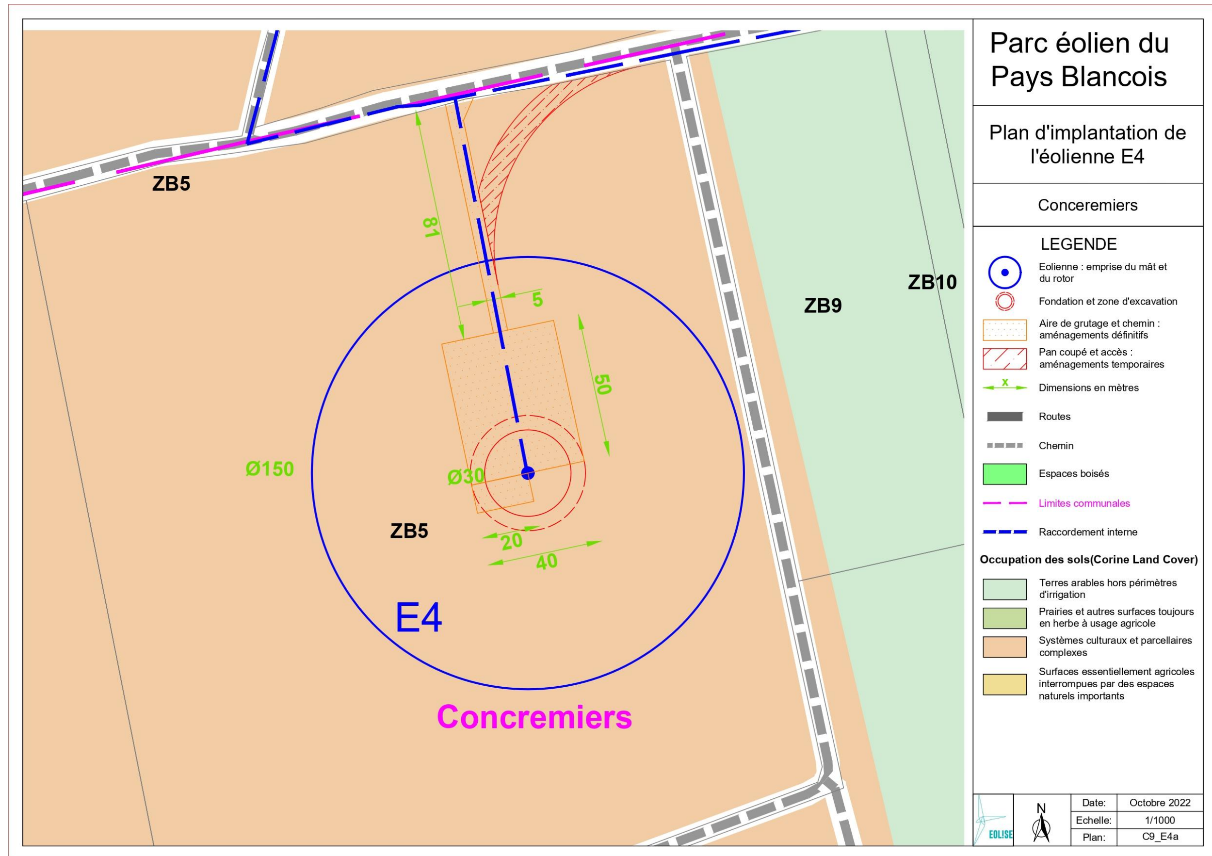
Carte 125 : Plan de masse de l'éolienne E4 (Source : EOLISE)
