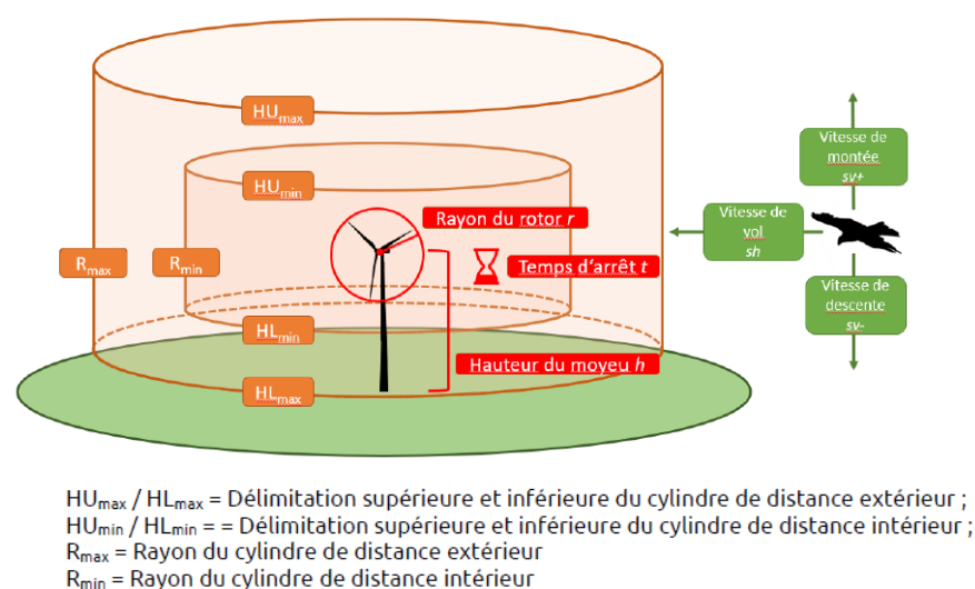
Figure 62 : Schéma de dimensionnement des cylindres intérieurs et extérieurs (Source : THEMA Environnement)
