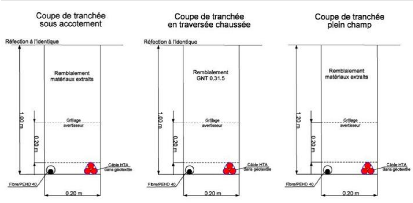
Figure 42 : Types de travaux de raccordement selon la nature du sol (Source : Enedis)
