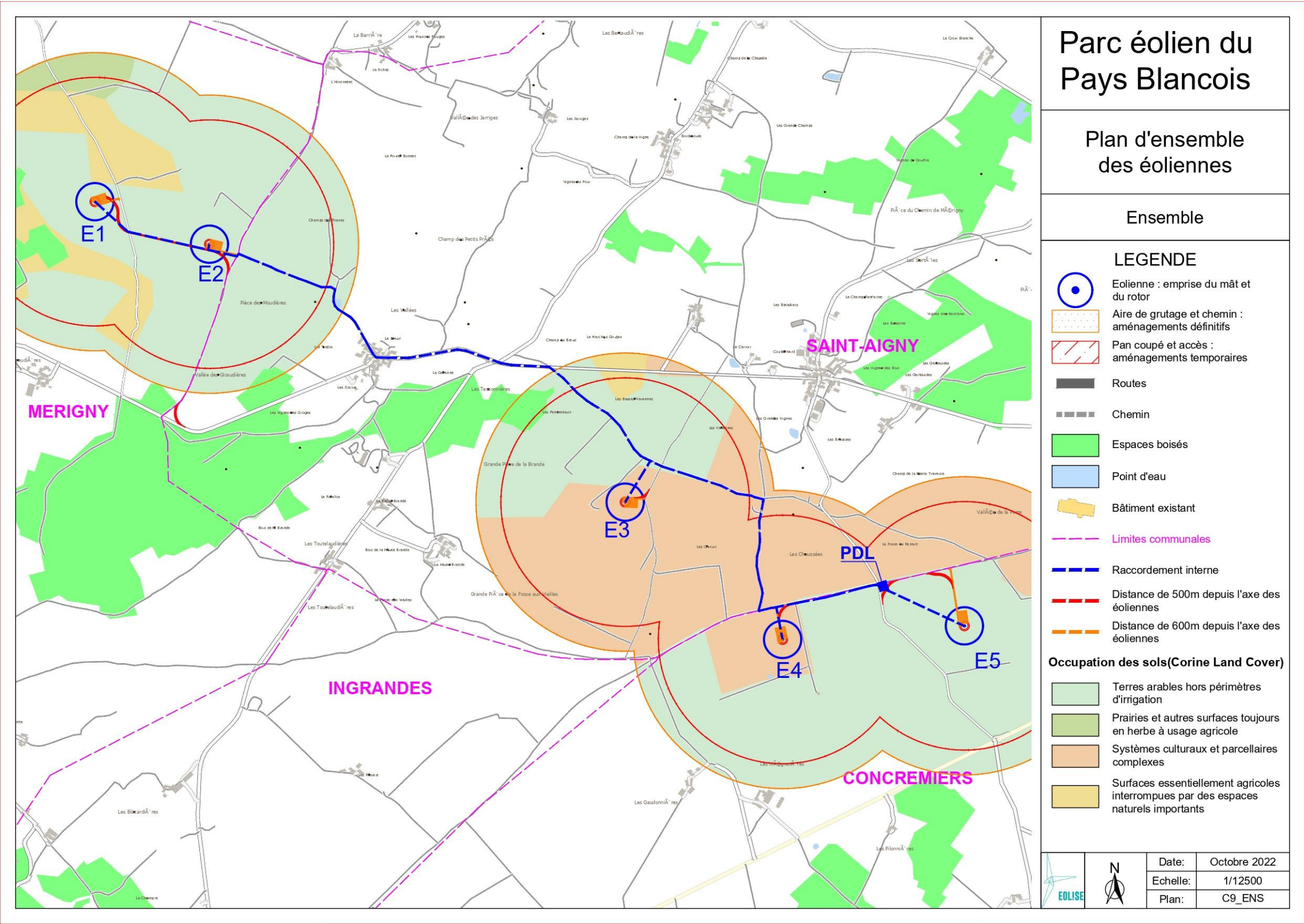
Carte 121 : Plan de masse général du parc éolien du Pays Blancois (Source : EOLISE)
