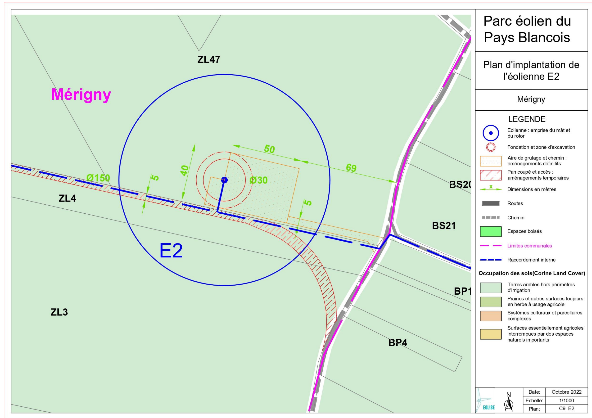
Carte 123 : Plan de masse de l'éolienne E2 (Source : EOLISE)
