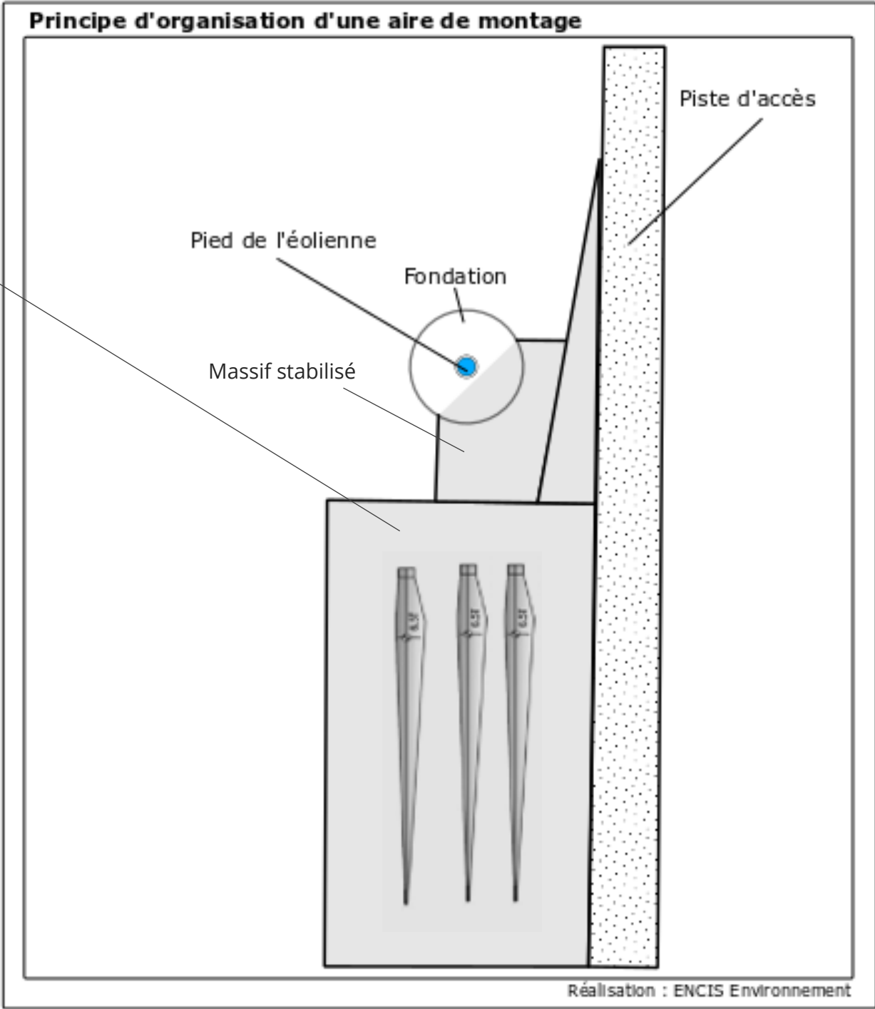
Figure 38 : Exemple d'aire de montage d'une éolienne
