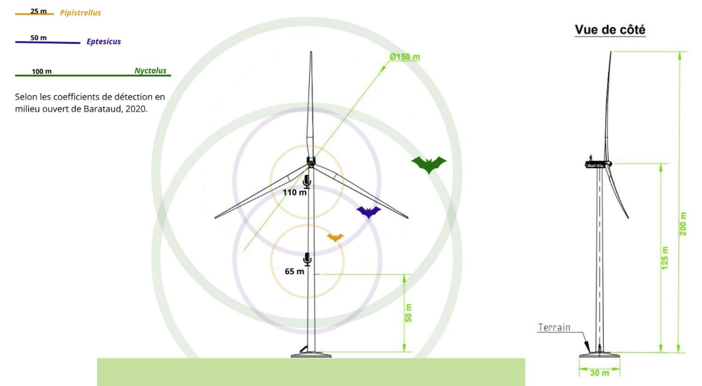
Figure 9 : Localisation des hauteurs de micros et distances de détection des chiroptères de haut vol projetées sur le modèle d'éolienne retenu (Source : ECHOCHIROS)
