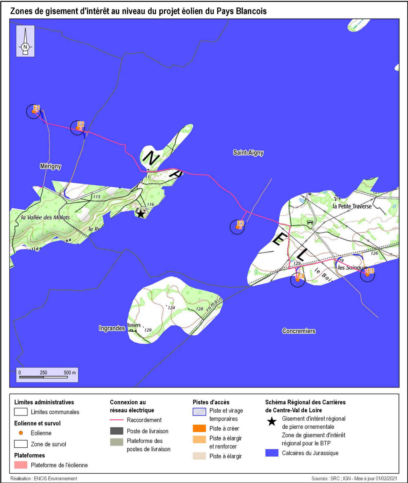
Carte 133 : Zones de gisement d'intérêt au niveau du projet éolien du Pays Blancs
