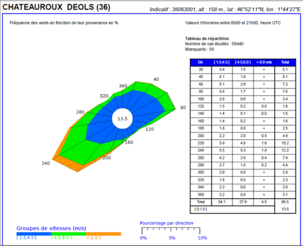
Figure 10 : Distribution des vents à 10 m à la station de Châteauroux-Déols (36) (Source : Météo France)
