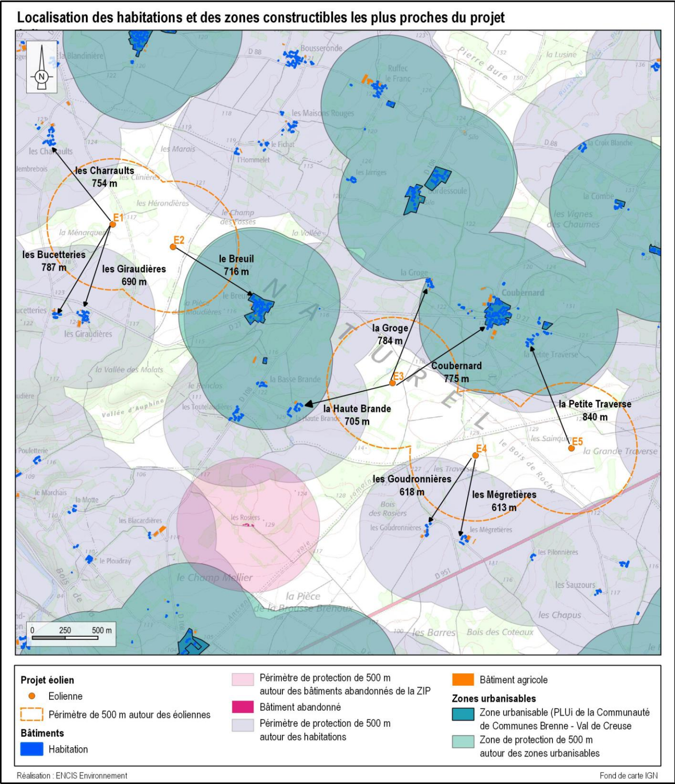
Carte 147 : Localisation des habitations par rapport au projet
