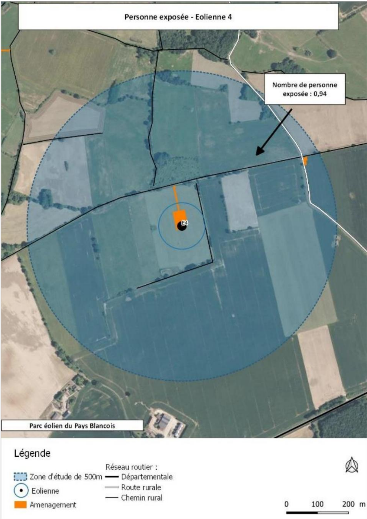
Carte 160 : Personnes exposées au niveau de l'éolienne E4 (Source : EOLISE)
