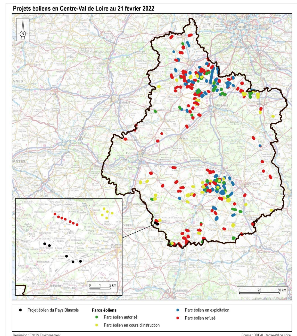
Carte 50 : Projets éoliens en Centre-Val de Loire au 21 février 2022 (source : DREAL Centre-Val de Loire)
