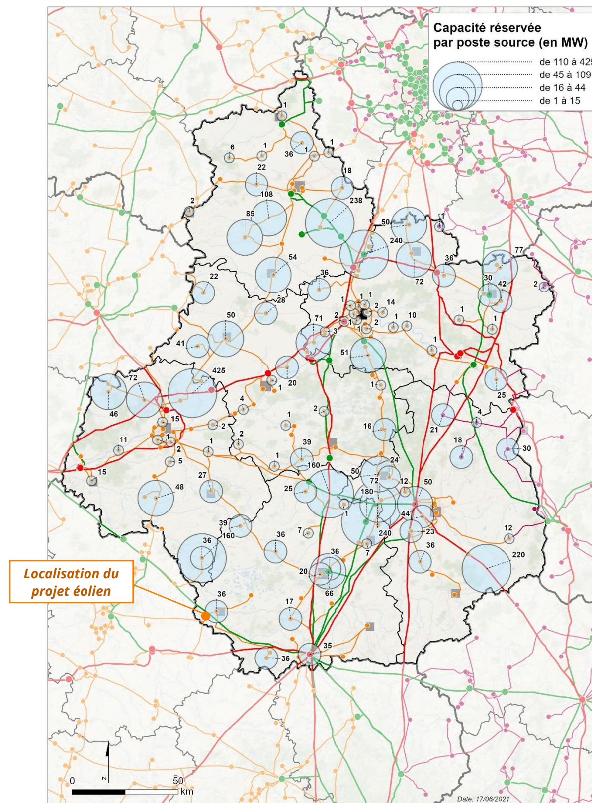
Carte 129 : Capacités d'accueil réservées dans le S3REnR (source : RTE)
