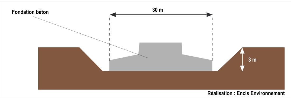
Figure 34 : Schéma type d'une fondation d'éolienne dans le cadre du projet du Pays Blancois (Source : ENCIS Environnement)
