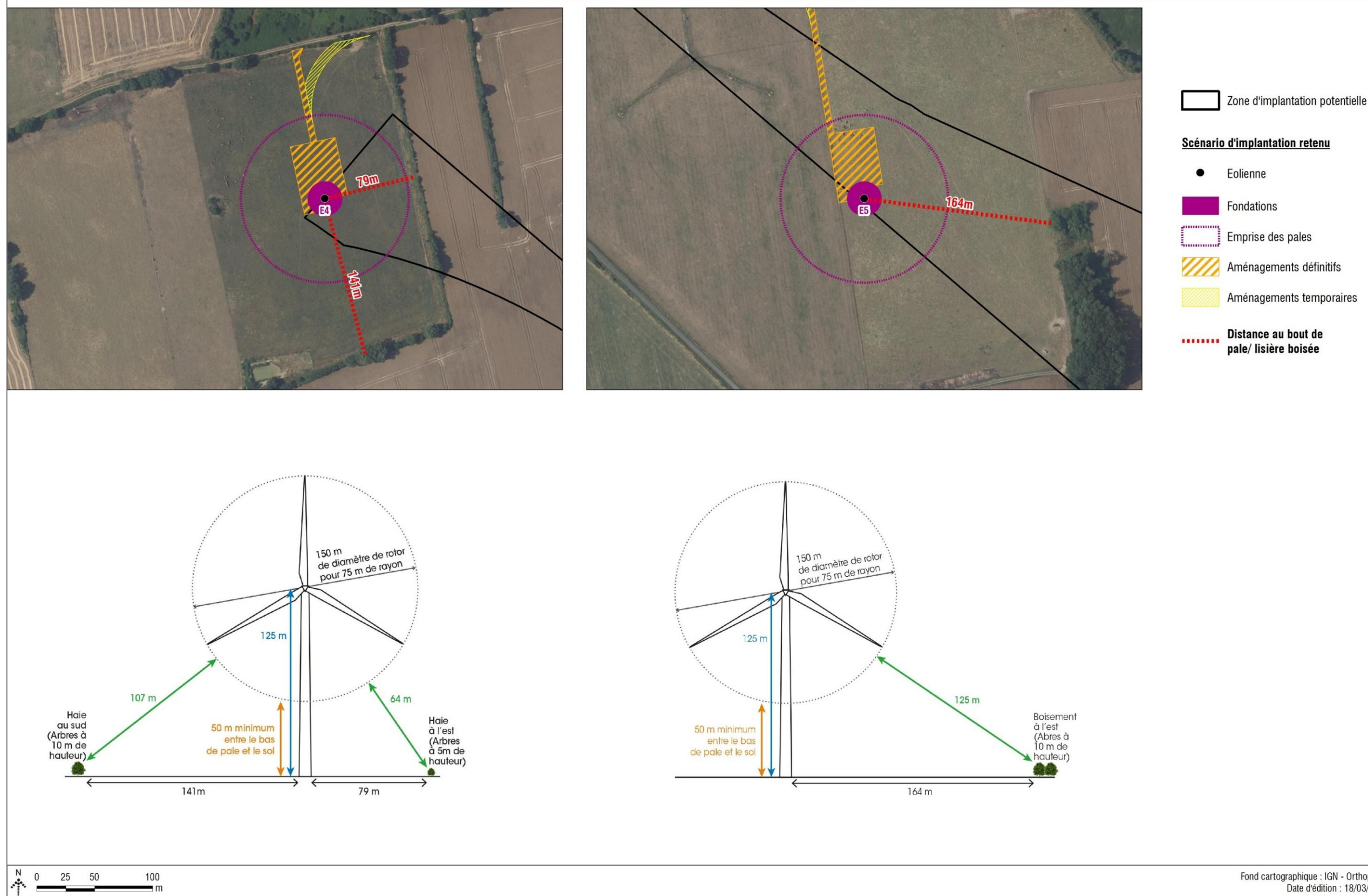
Carte 167 : Distances entre les éoliennes E4 et E5 et les lisières boisées les plus proches (Source : THEMA Environnement)
