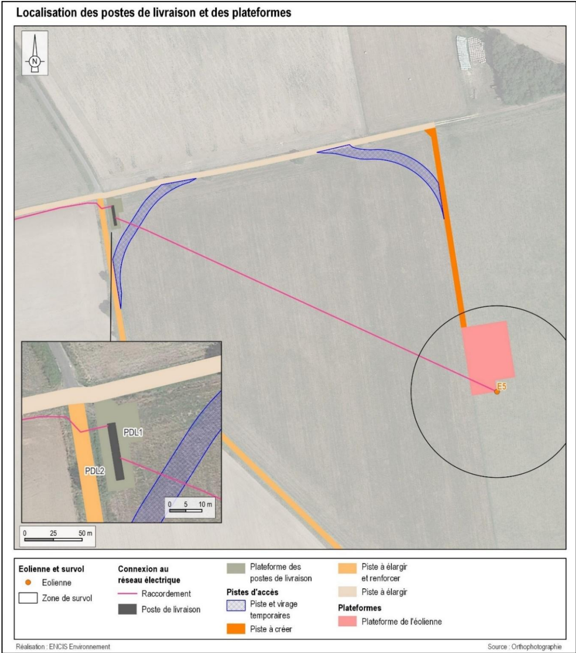
Carte 119 : Plan de masse des postes de livraison
