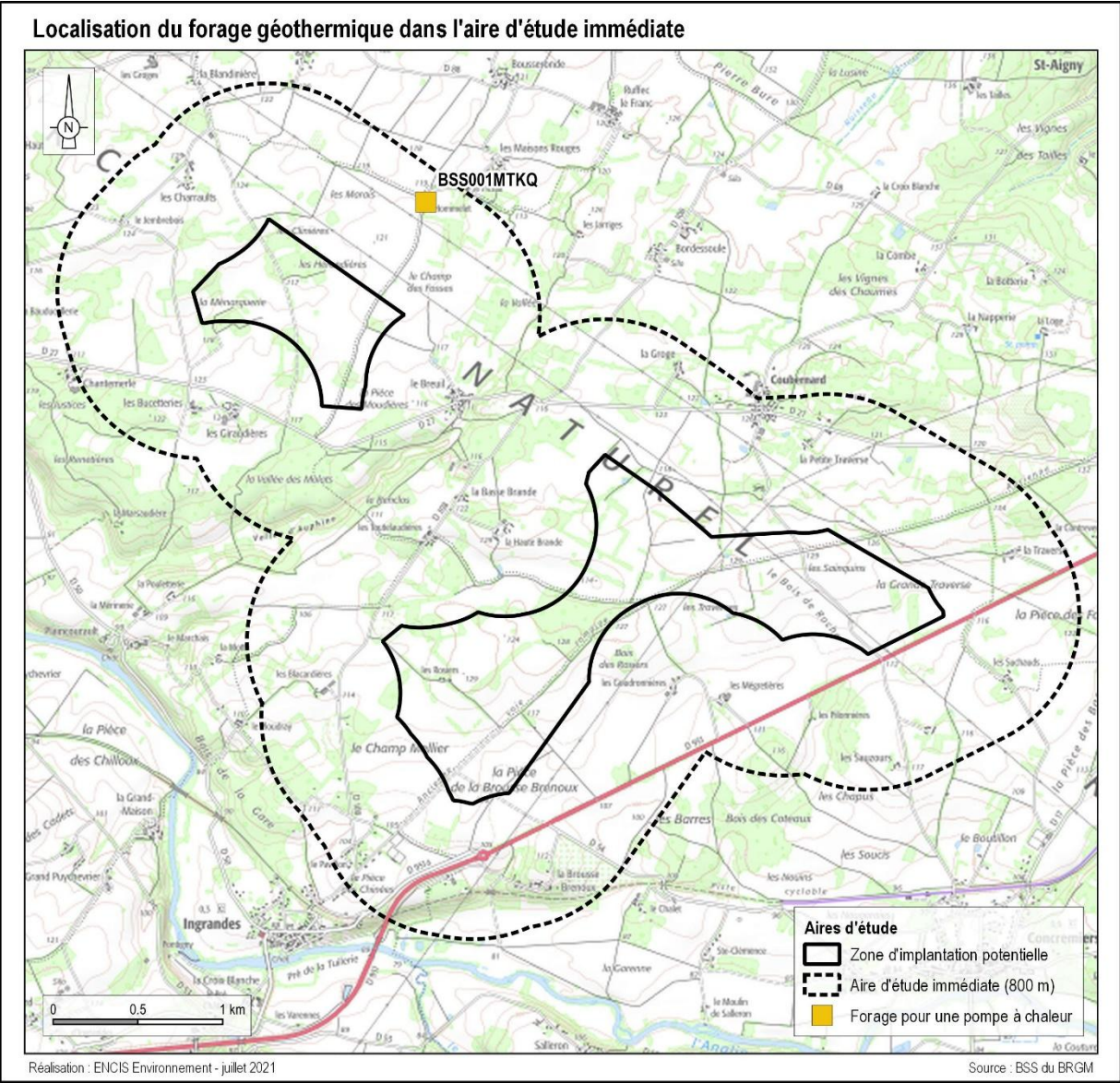
Carte 22 : Localisation du forage pour l'utilisation d'une pompe à chaleur dans l'aire d'étude immédiate
