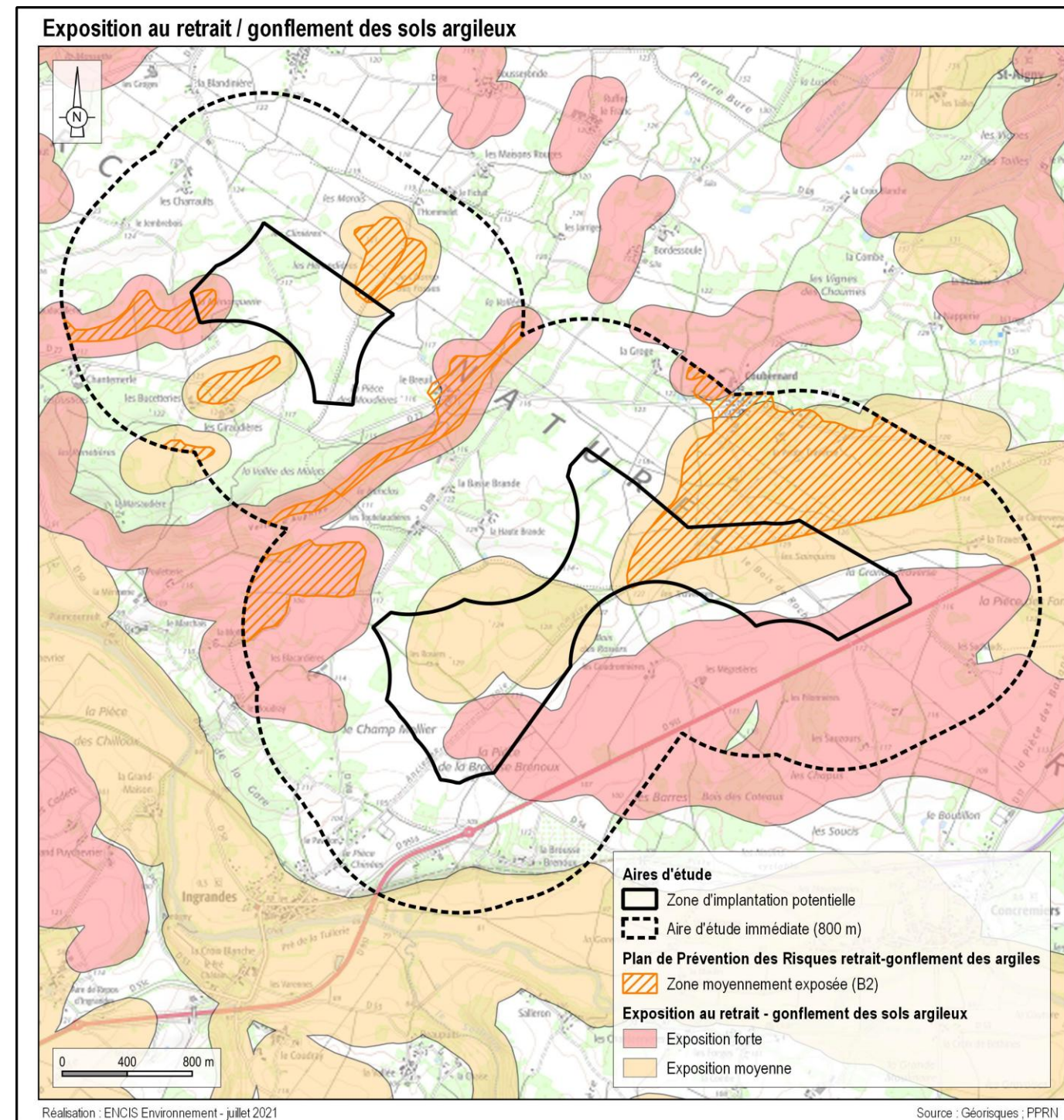
Carte 32 : Exposition au retrait-gonflement des sols argileux à proximité de la zone d'implantation potentielle
