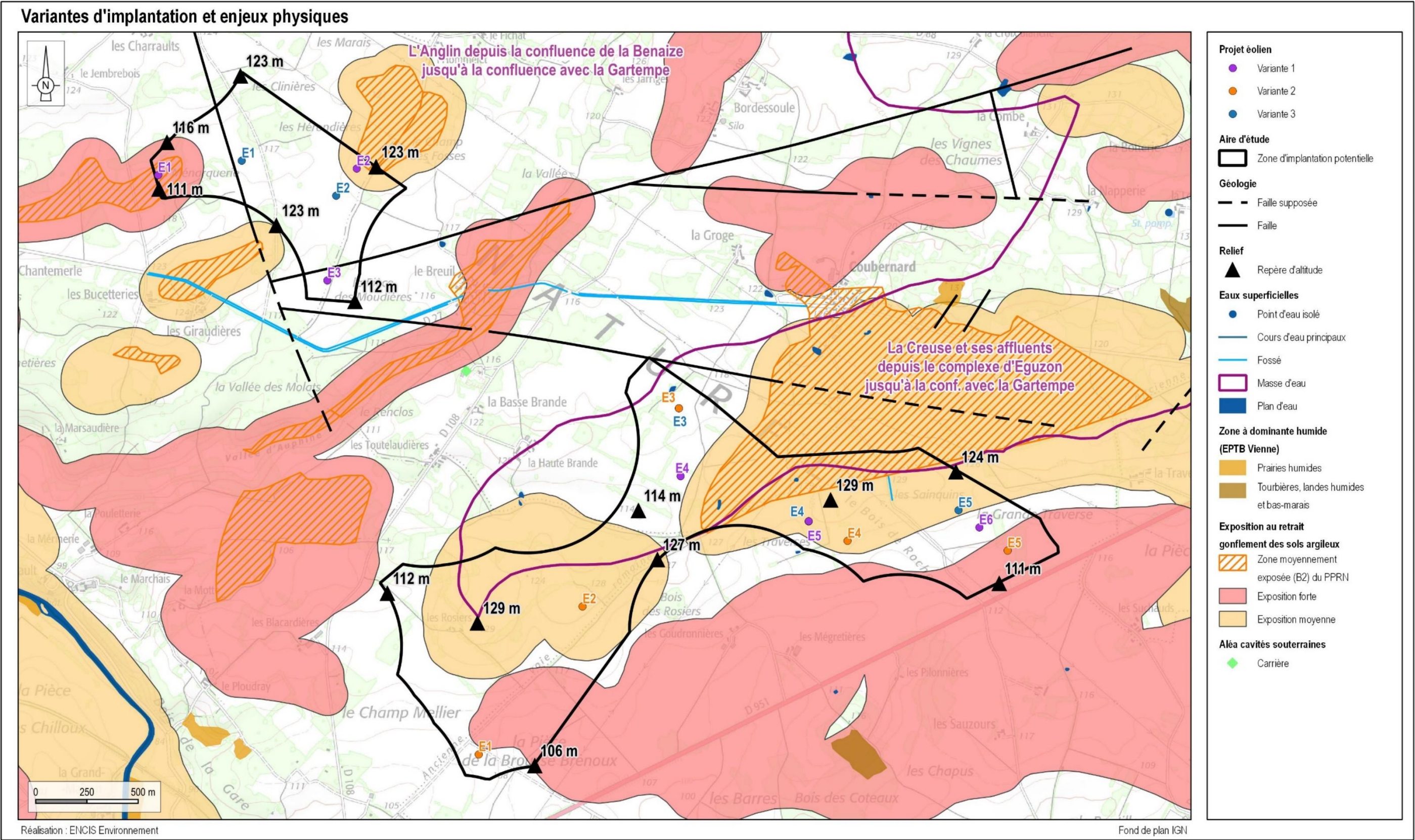
Carte 110 : Comparaison des variantes du point de vue physique
