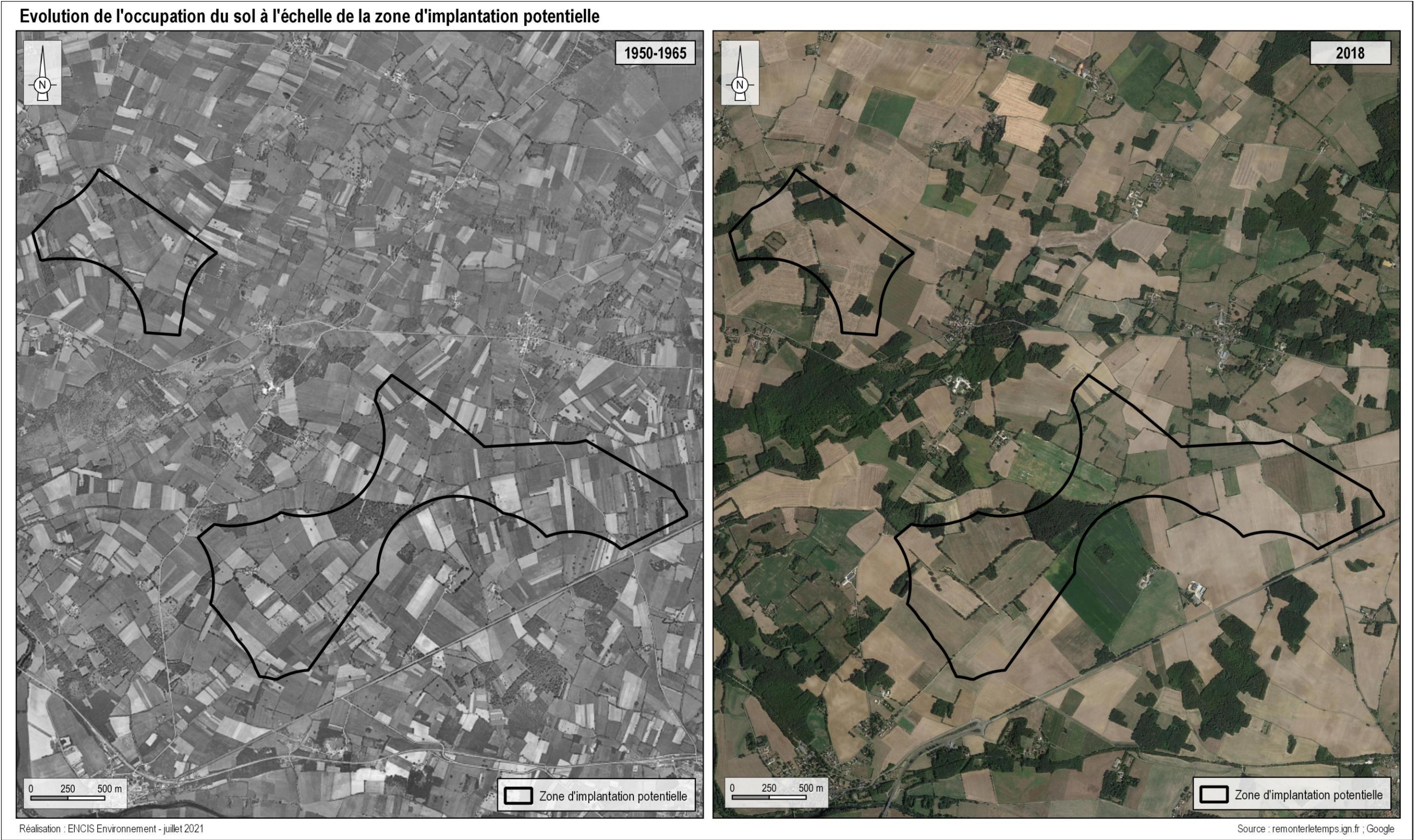
Figure 25 : Photos aériennes du site de 1950-1965 - à gauche - et 2018 - à droite (Source : remonterletemps.ign.fr)
