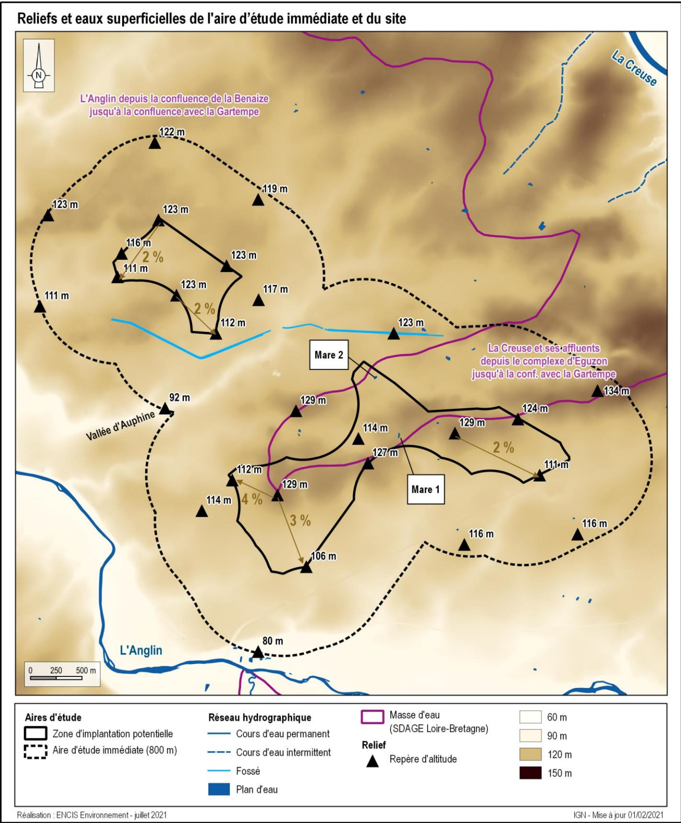
Carte 25 : Relief et eaux superficielles de l'aire d'étude immédiate et de la zone d'implantation potentielle
