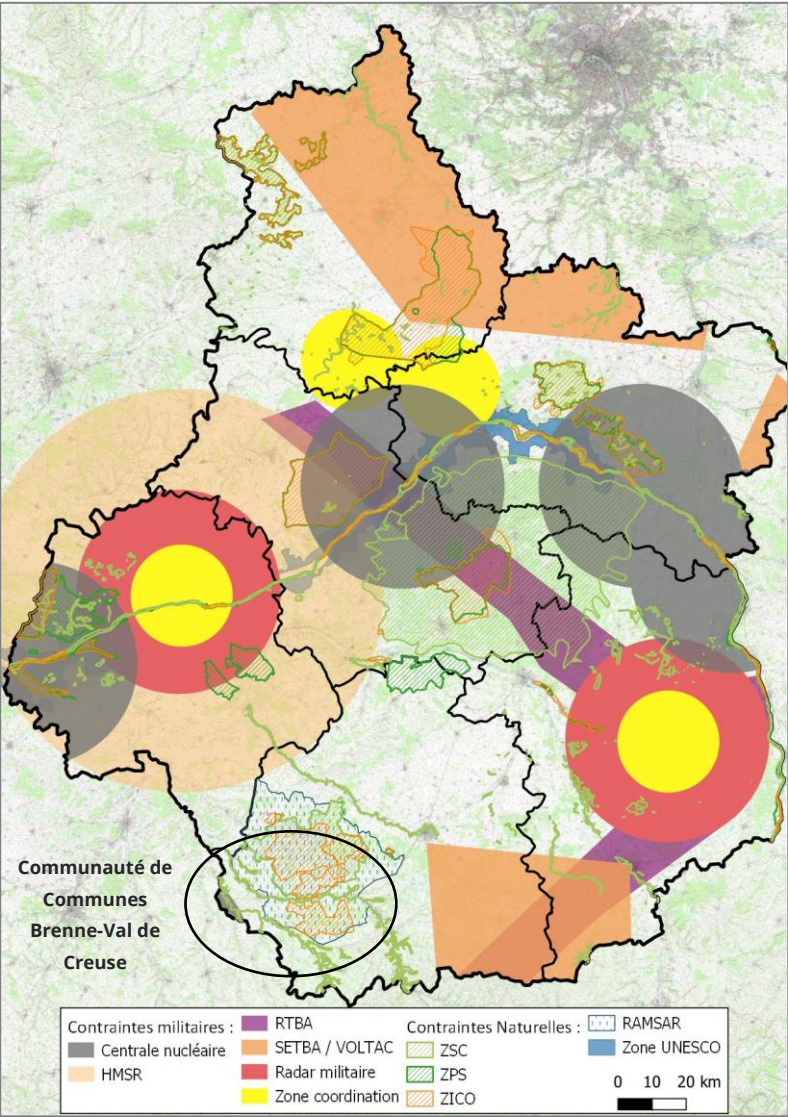
Carte 89 : Carte des contraintes au développement éolien en région Centre-Val de Loire (Source : EOLISE)
