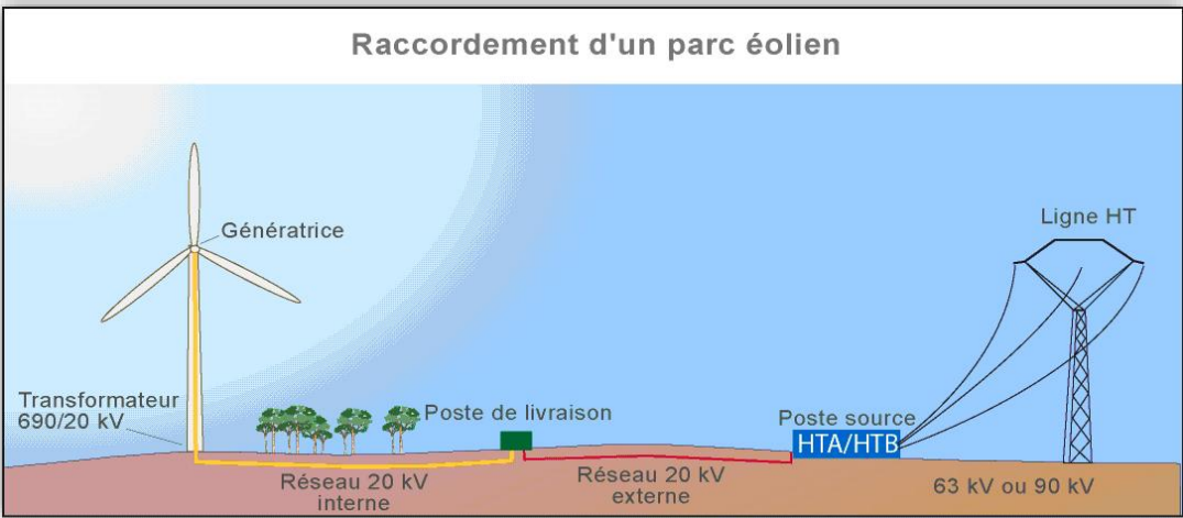
Figure 35 : Organisation générale du raccordement électrique au réseau de distribution (Source : ENCIS Environnement)
