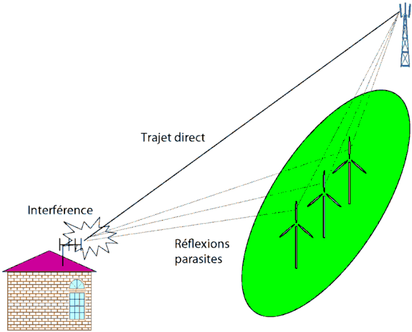
Figure 53 : Principe de la perturbation du signal TV par un parc éolien (Source : ANFR)
