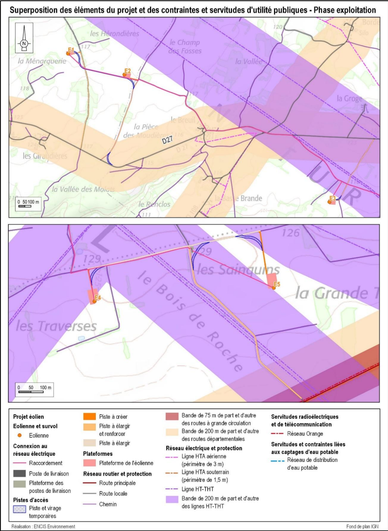
Carte 150 : Localisation du projet vis-à-vis des servitudes et contraintes
