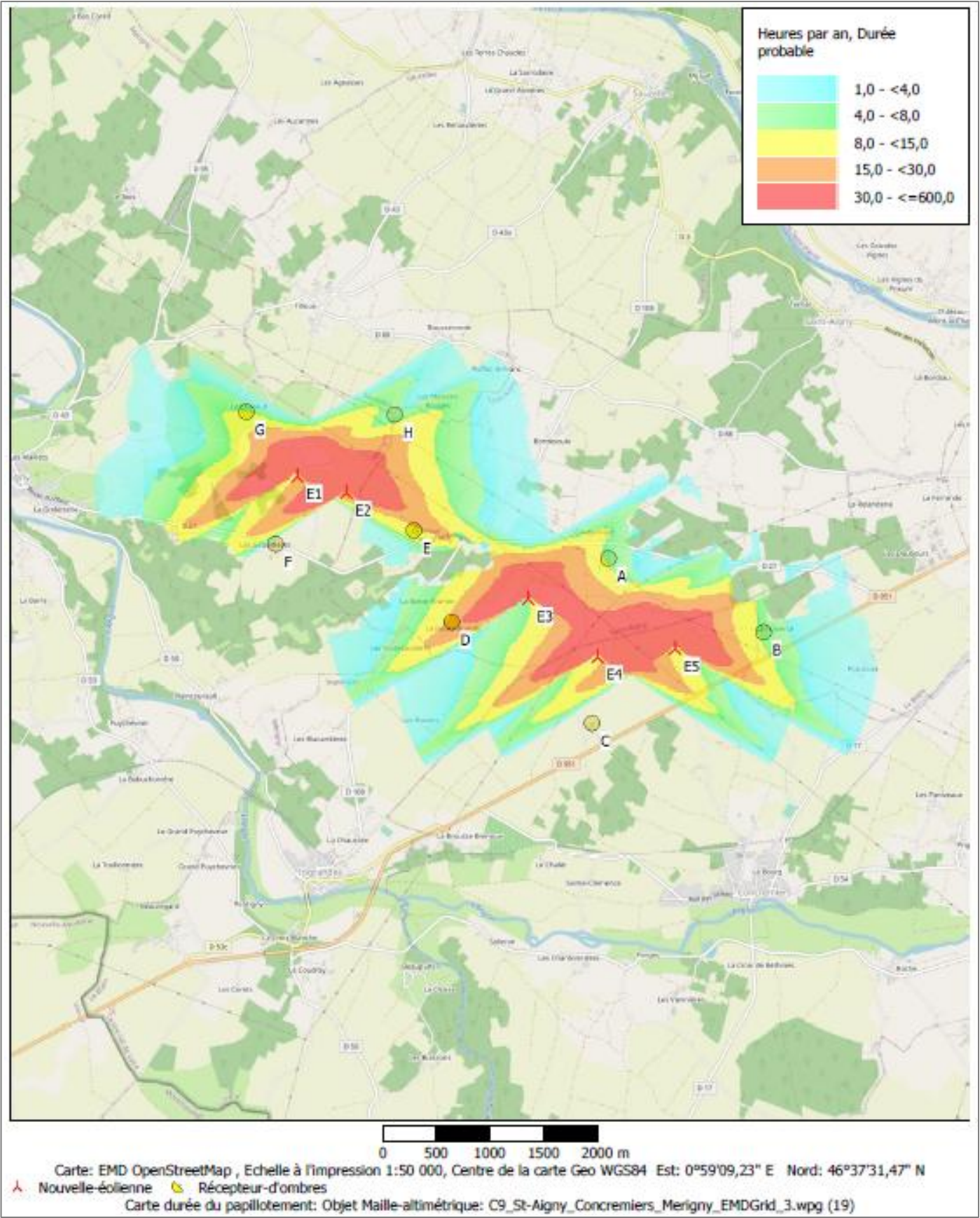
Carte 155 : Répartition de la durée probable d'ombre, sur terrain nu sans végétation (Source : EOLISE)
