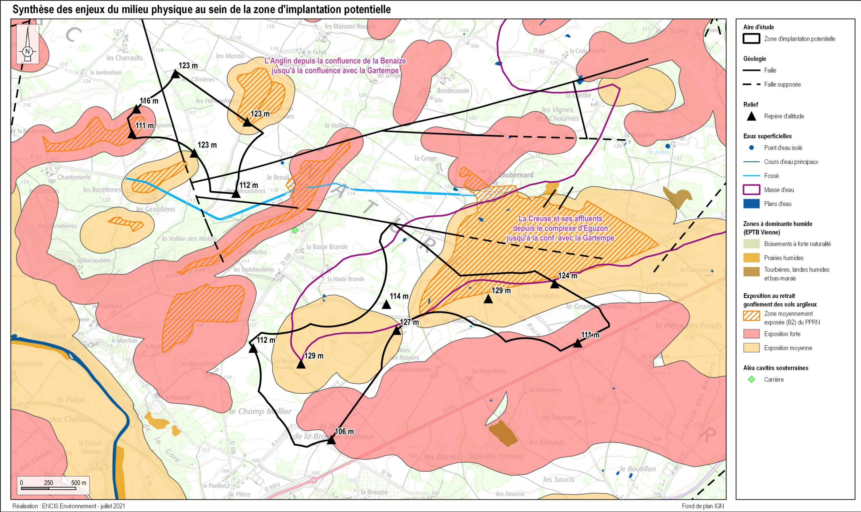
Carte 78 : Synthèse des enjeux du milieu physique de la zone d'implantation potentielle
