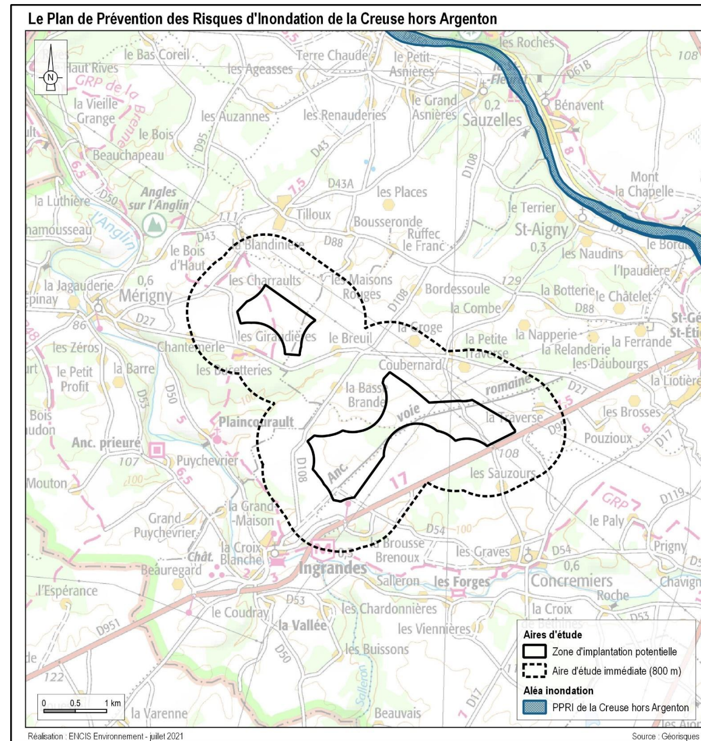
Carte 29 : Aléa inondation dans l'aire d'étude immédiate
