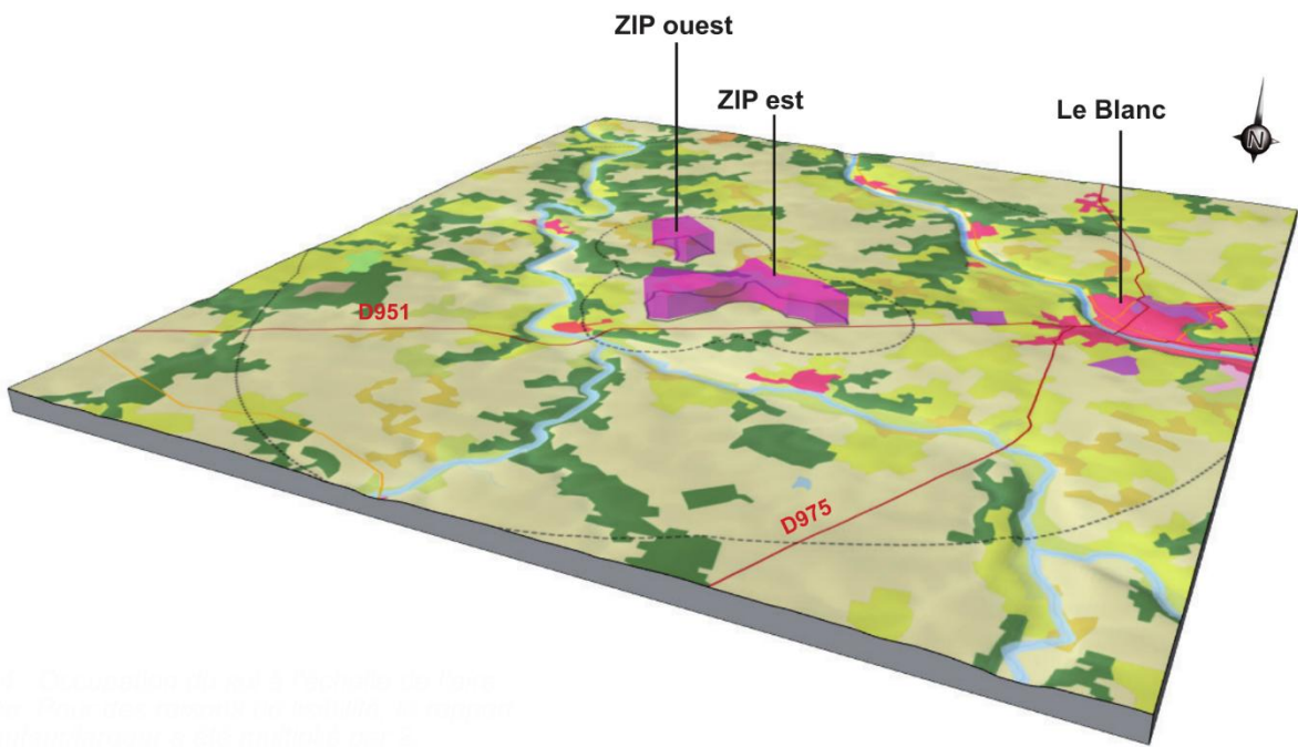
Figure 23 : Occupation du sol à l'échelle de l'aire rapprochée. Pour des raisons de lisibilité, le rapport hauteur/largeur a été multiplié par 2
