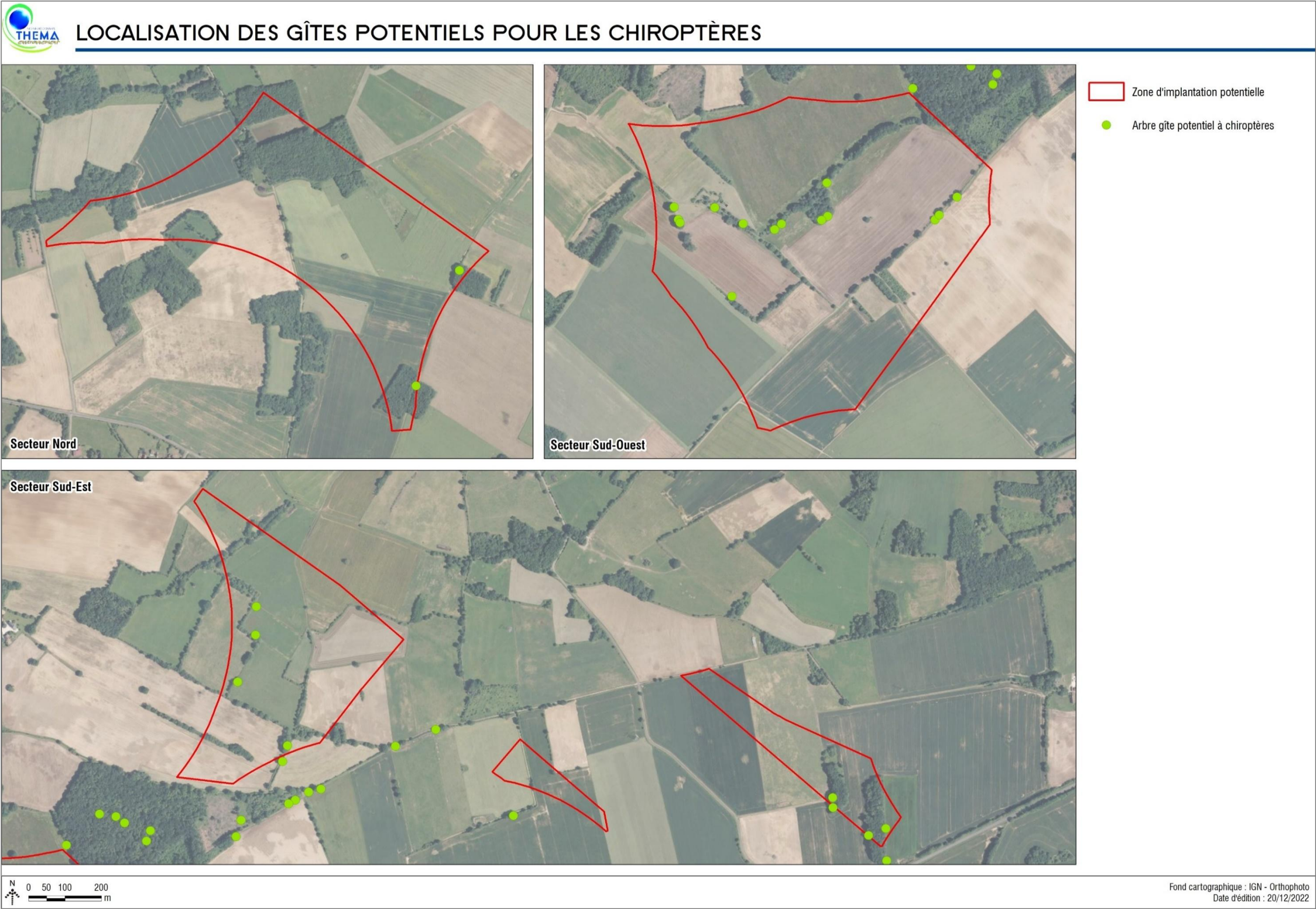
Carte 75 : Localisation des arbres gîtes potentiels pour les chiroptères (Source : THEMA Environnement)
