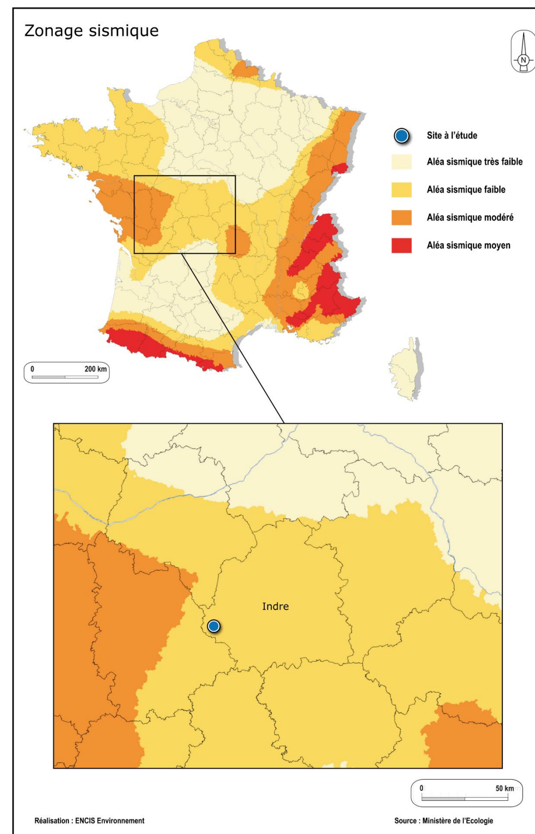
Carte 34 : Zonage sismique dans l'Indre
