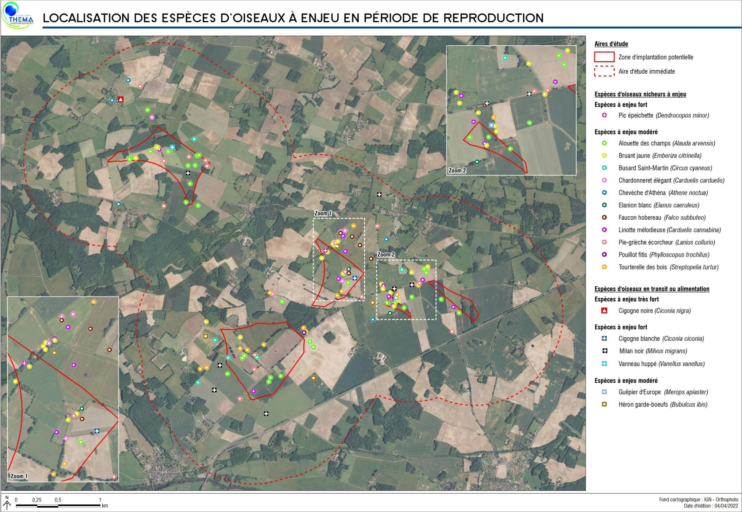
Carte 71 : Localisation des observations d'oiseaux nicheurs à enjeu dans l'aire d'étude immédiate (Source : THEMA Environnement)
