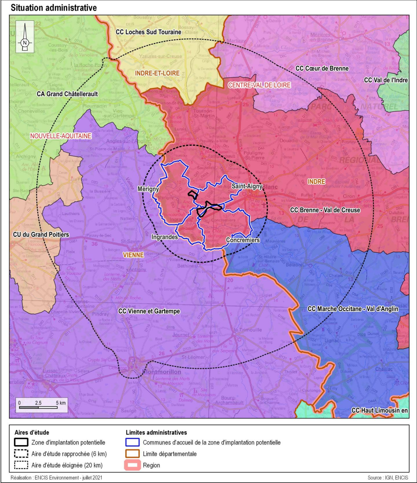
Carte 2 : Localisation du site d'implantation dans l'Indre et au sein de la Communauté de Communes
