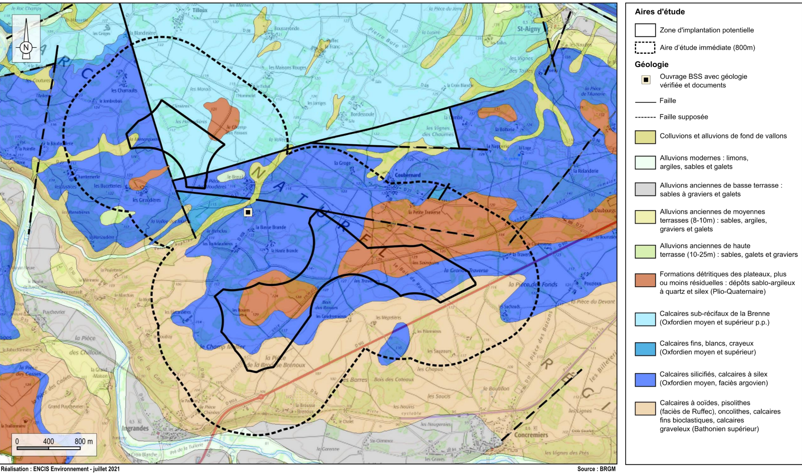
Carte 20 : Extrait des cartes géologiques au 1/50 000 (Sources : BRGM, IGN)
