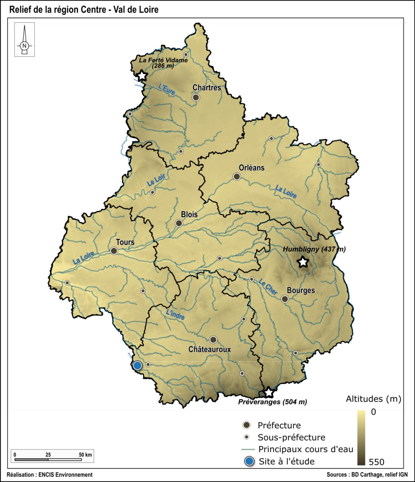
Carte 23 : Relief et eaux superficielles du Limousin
