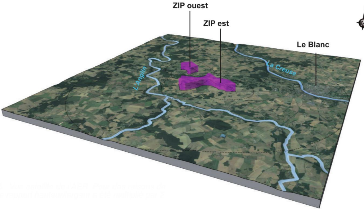
Figure 22 : Vue satellite de l'AER. Pour des raisons de lisibilité, le rapport hauteur/largeur a été multiplié par 2
