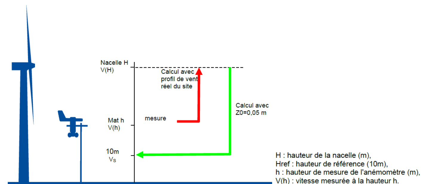
Figure 7 : Principe du calcul de la vitesse standardisée V_s (Source : EREA INGENIERIE)
