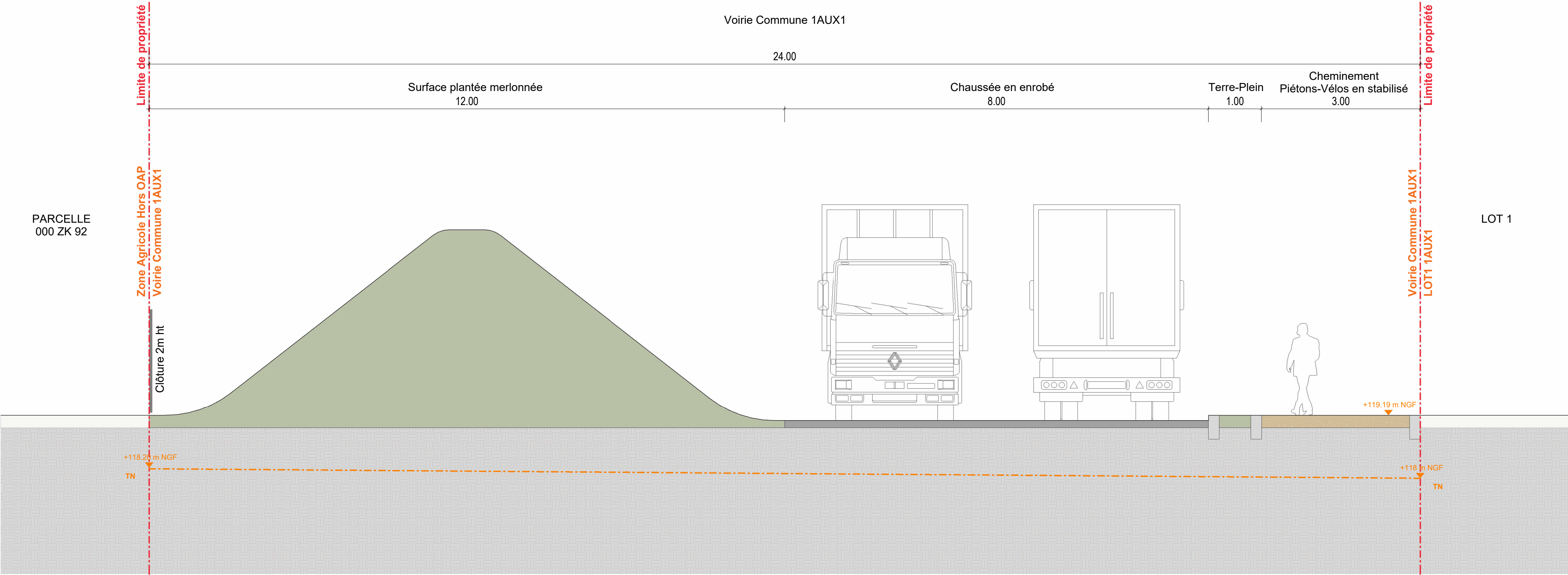
COUPE PRINCIPE VOIRIE COMMUNE Echelle 1:50
