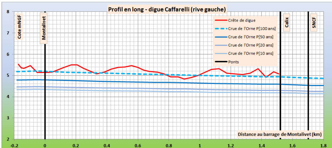
Figure 4-6 : lignes d'eau pour les crues de référence – Caffarelli.
