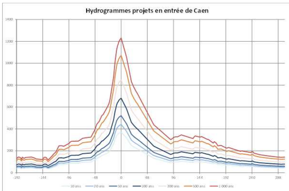
Figure 4-1 : hydrogrammes de crues de l'Orne à Caen.
