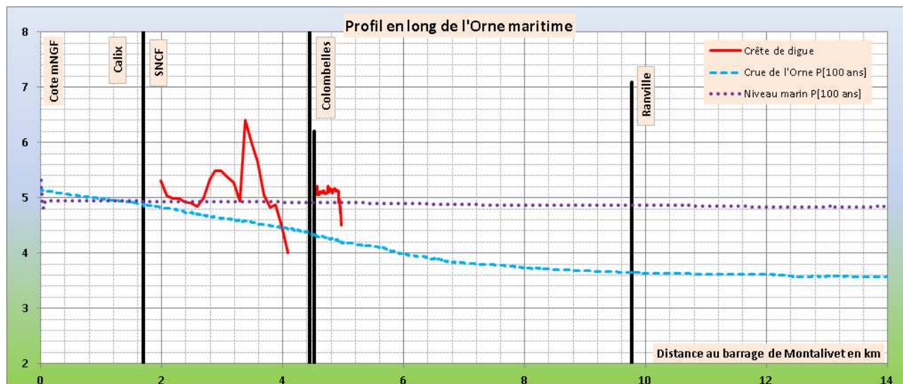
Figure 6-1 : profil en long des deux évènements centennaux le long de l'Orne maritime.
