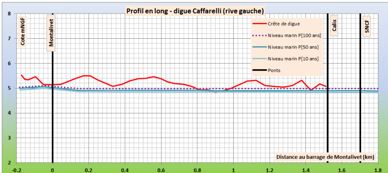
Figure 5-4 : lignes d'eau pour les évènements marins de référence – Caffarelli.
