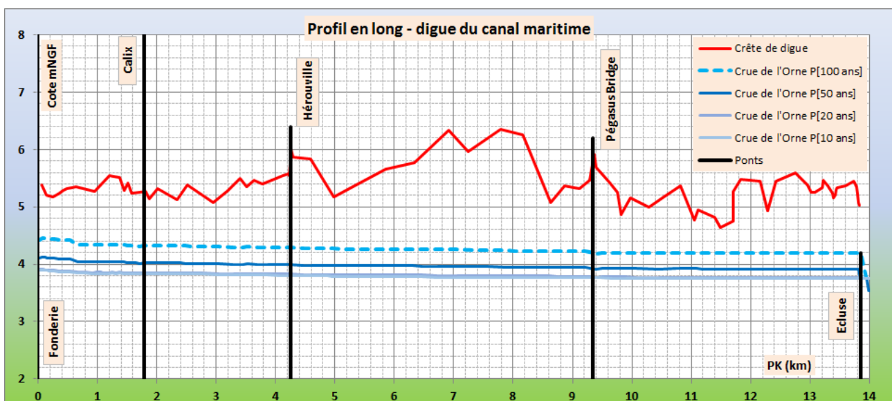
Figure 4-9 : lignes d'eau pour les crues de référence – Canal maritime.
