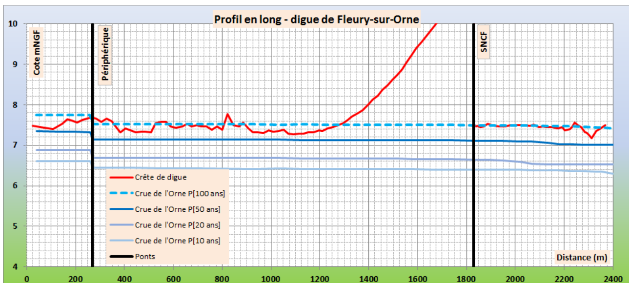
Figure 4-3 : lignes d'eau pour les crues de référence – Fleury-sur-Orne.
