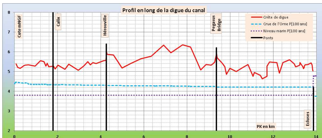
Figure 6-2 : profil en long des deux évènements centennaux le long du canal.
