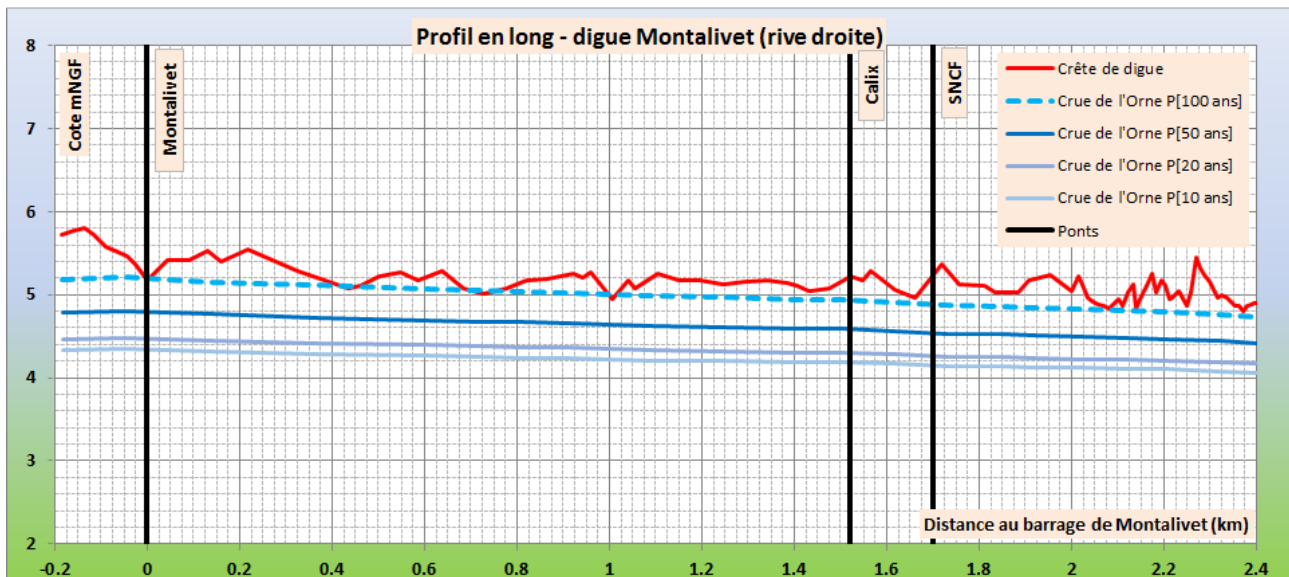
Figure 4-7 : lignes d'eau pour les crues de référence – Montalivet.
