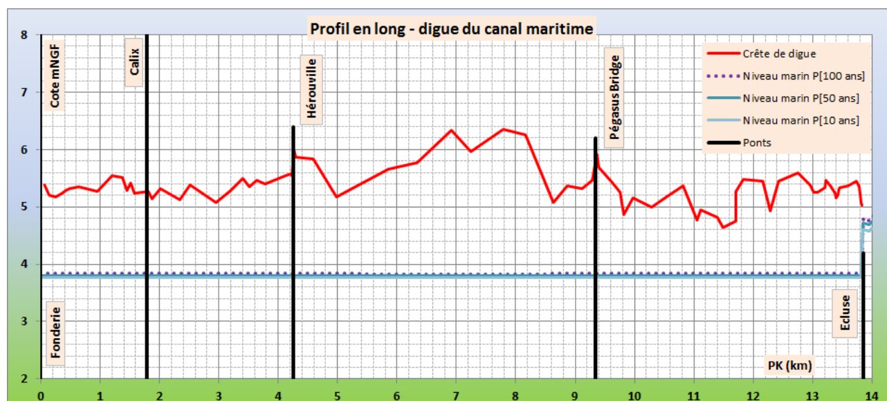
Figure 5-7 : lignes d'eau pour les événements marins de référence – Canal maritime.
