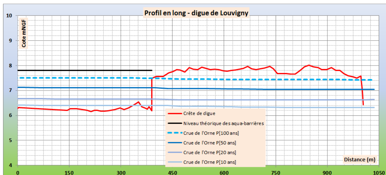
Figure 4-4 : lignes d'eau pour les crues de référence – Louvigny.
