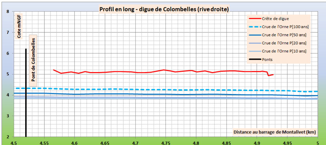
Figure 4-8 : lignes d'eau pour les crues de référence – Colombelles.
