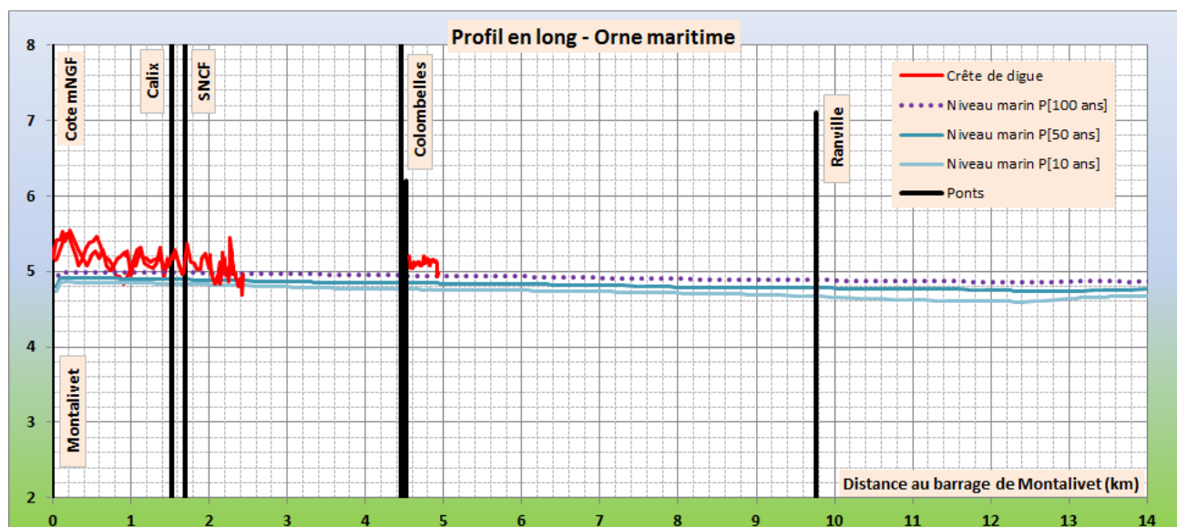
Figure 5-3 : lignes d'eau le long de l'Orne maritime.
