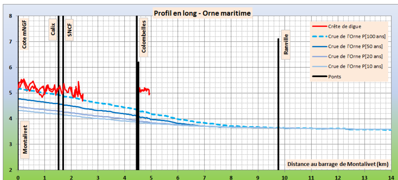
Figure 4-5 : lignes d'eau le long de l'Orne maritime.
