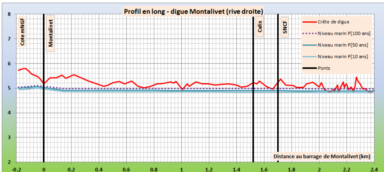
Figure 5-5 : lignes d'eau pour les évènements marins de référence – Montalivet.
