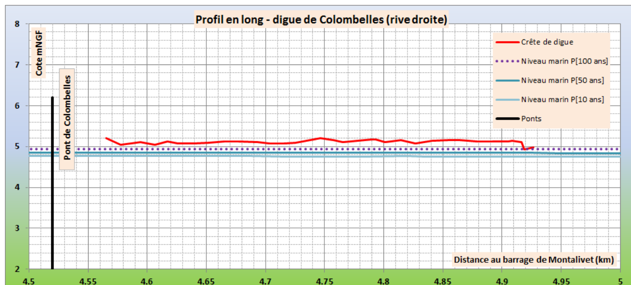
Figure 5-6 : lignes d'eau pour les événements marins de référence – Colombelles.
