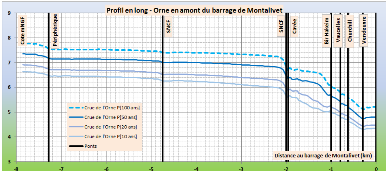
Figure 4-2 : lignes d'eau le long de l'Orne fluviale.
