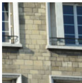
Finition rugueuse, lits de différentes épaisseurs, pierres de longueurs variées, joints légèrement creux.
