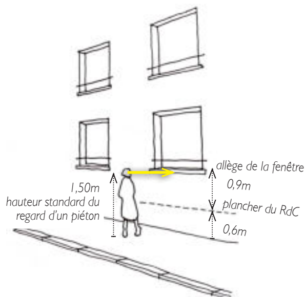
Exemple de hauteur du plancher de rez-de-chaussée par rapport au trottoir qui permet de préserver l'intimité des logements.
