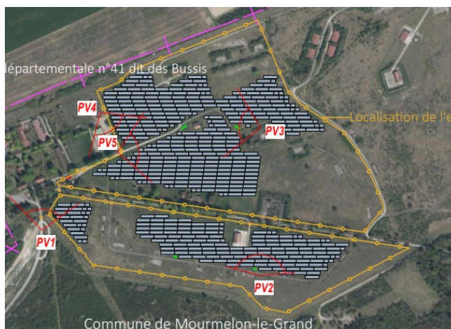
Figure 64 : Projet photovoltaïque final
