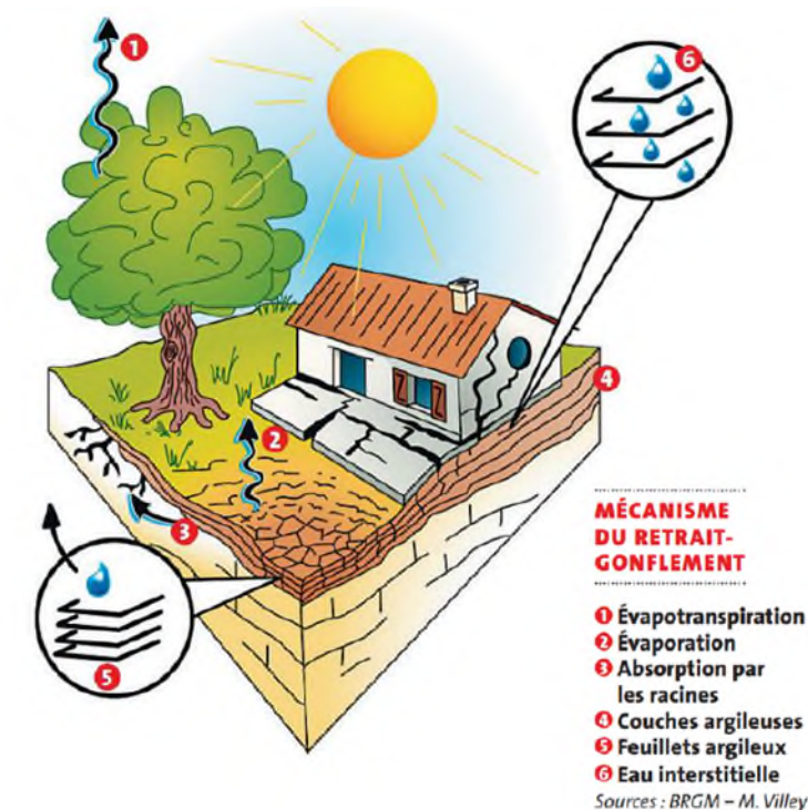
Figure 109 - Schéma du phénomène de retrait-gonflement des argiles (source : BRGM)
