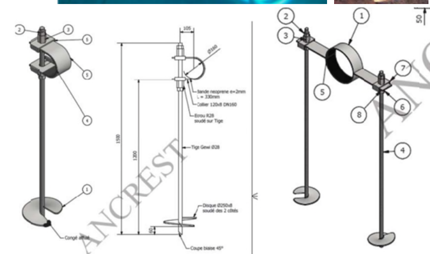
Figure 102 - Exemple d'ancre à sable type hélicoïdale (Harmony) de 1,5m de long pour assurer la stabilité de la conduite avec colliers de cerclage
