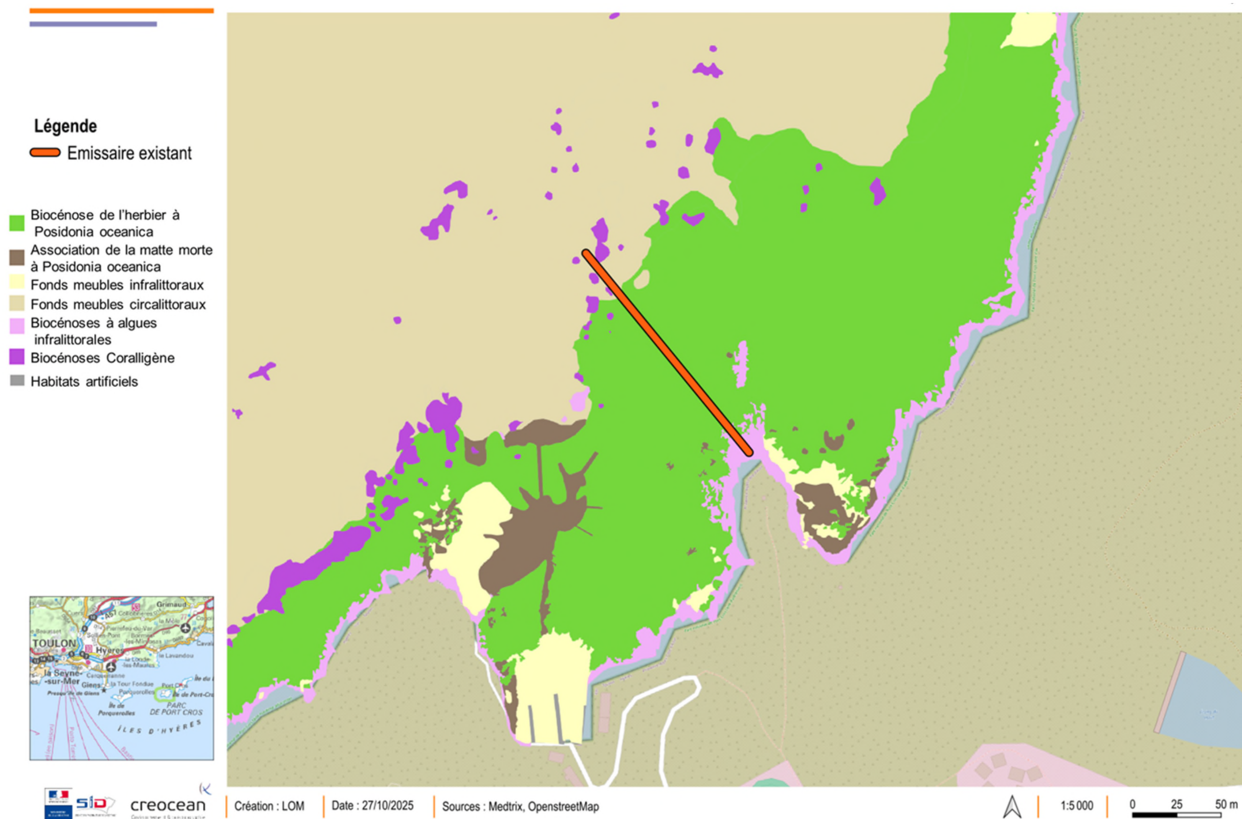
Figure 90 - Cartographie des biocénoses marines au niveau de la zone d'étude (source : MEDTRIX, 2022)
