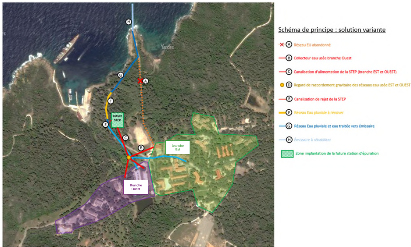
Figure 100 - Plan de principe du scénario n°2
