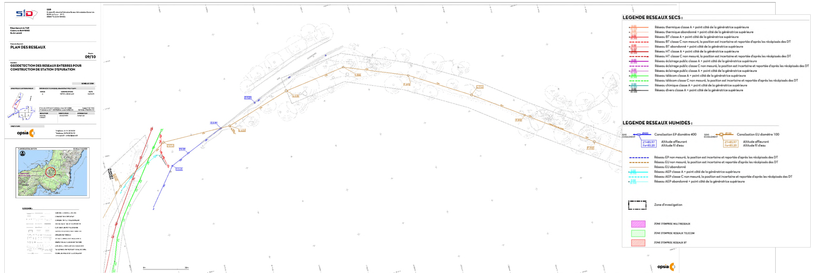
Figure 67 - Plan des réseaux, secteur nord de la zone d'étude (source : Opsia)
