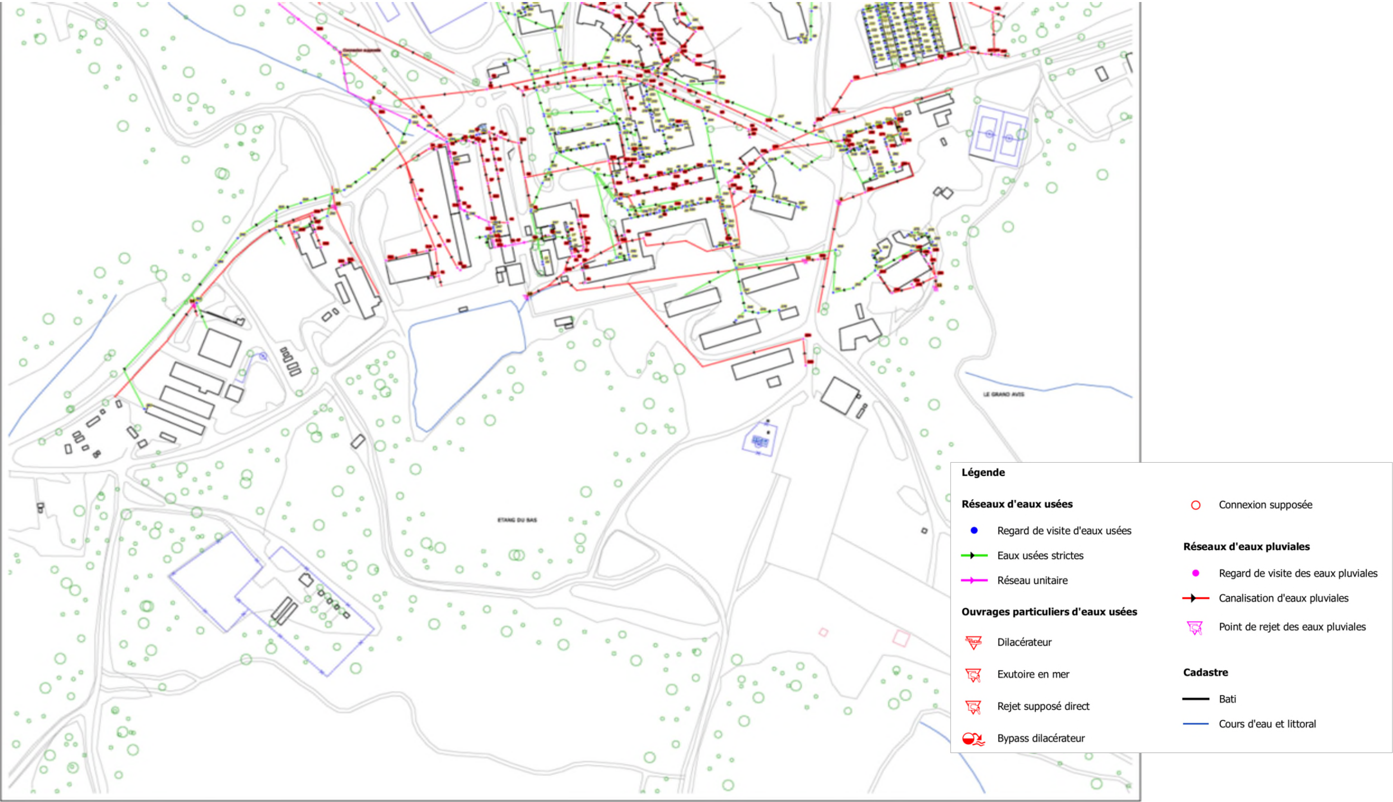
Figure 64 - Cartographie (2/2) de l'architecture des réseaux d'eaux usées et pluviales de la Base vie du Levant (source : Cereg)
