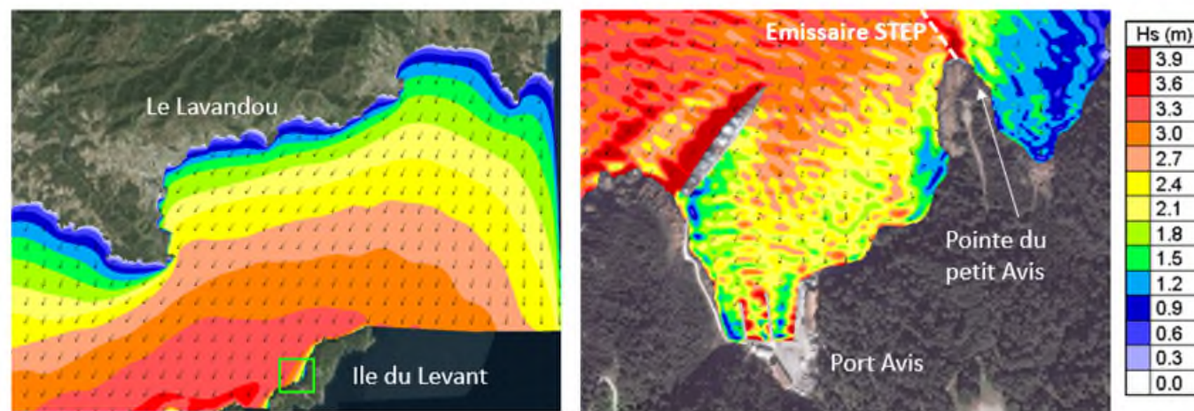
Figure 44 - Planche de génération de mer de vent de secteur NNE (conditions de vent T50) à gauche et planche d'agitation au droit de Port Avis (source : BONNA TP, 2020)
