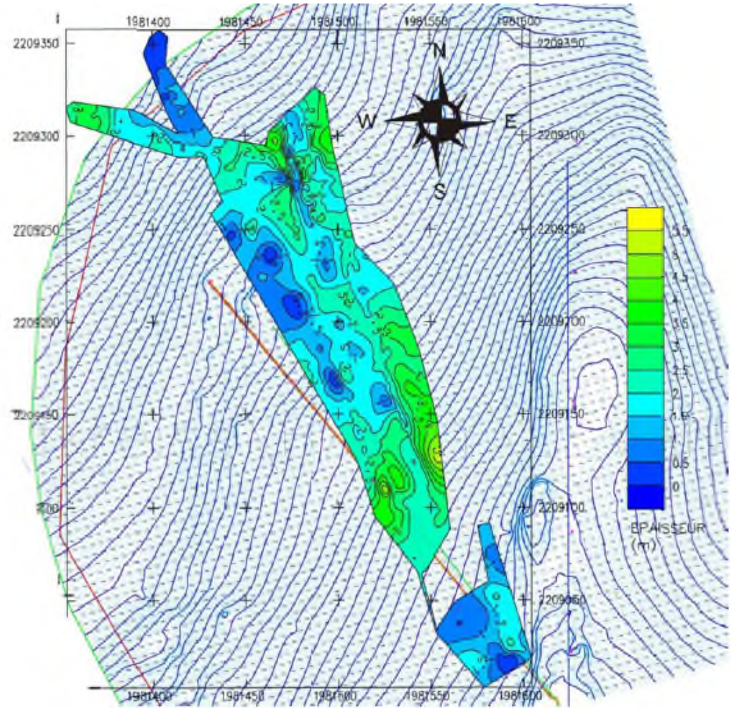
Figure 37 - Épaisseur de sédiments (source : Sixense, 2019) – Émissaire en rouge sur la figure
