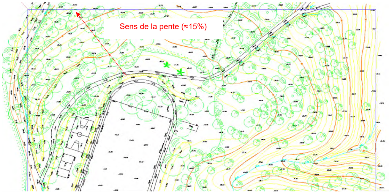
Figure 32 - Extrait des levés topographiques effectués sur site (source : OPSIA)
