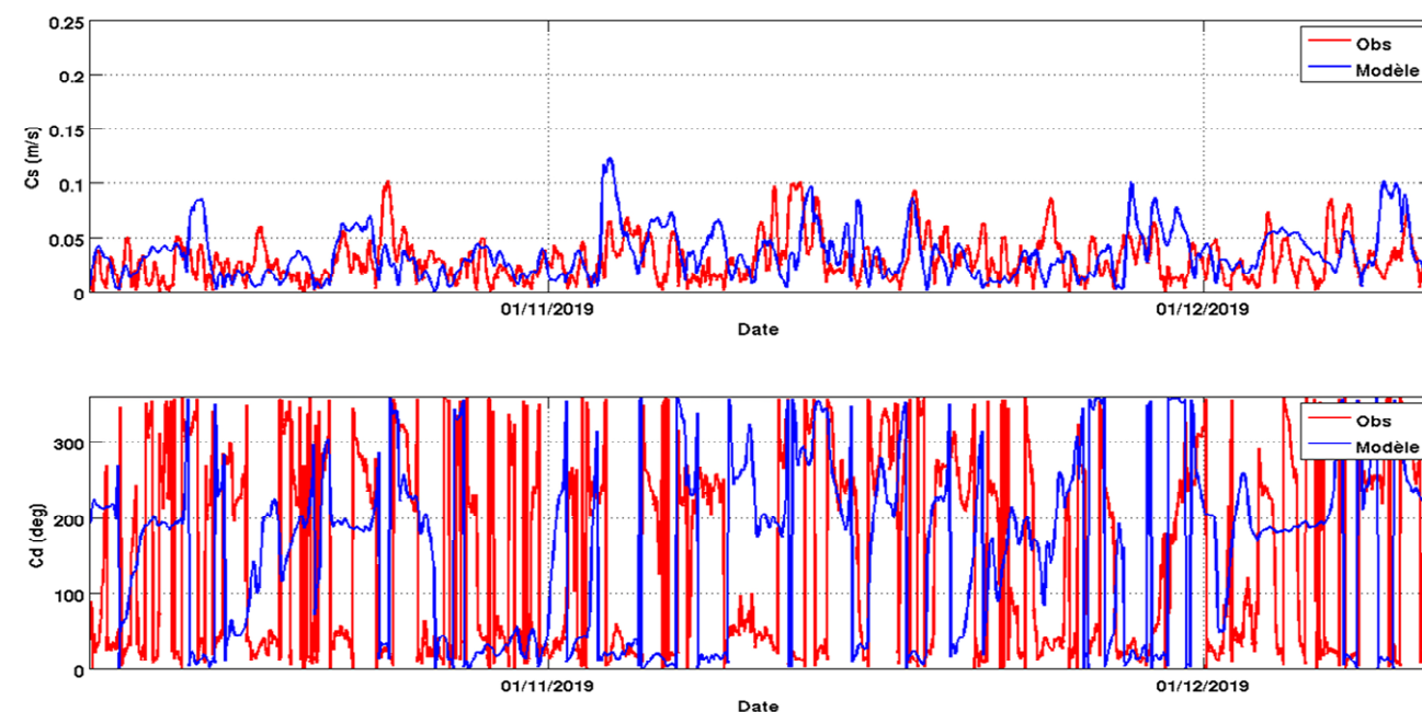
Figure 47 - Série temporelle de vitesse et direction de courant (mesures en rouge et modèle en bleu)
