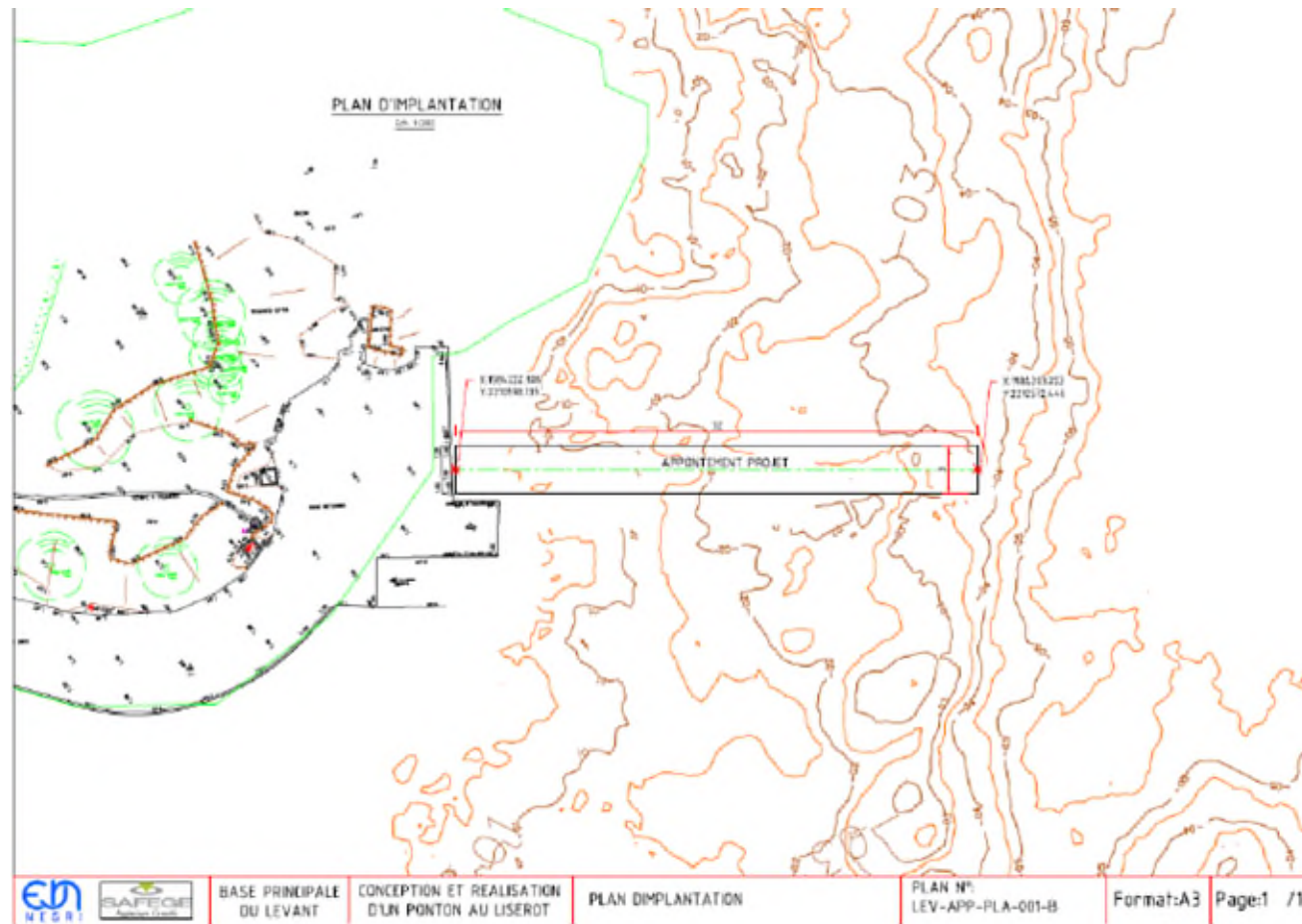
Figure 125 - Plan masse du projet (source : dossier loi sur l'eau réfection du ponton de Liserot)
