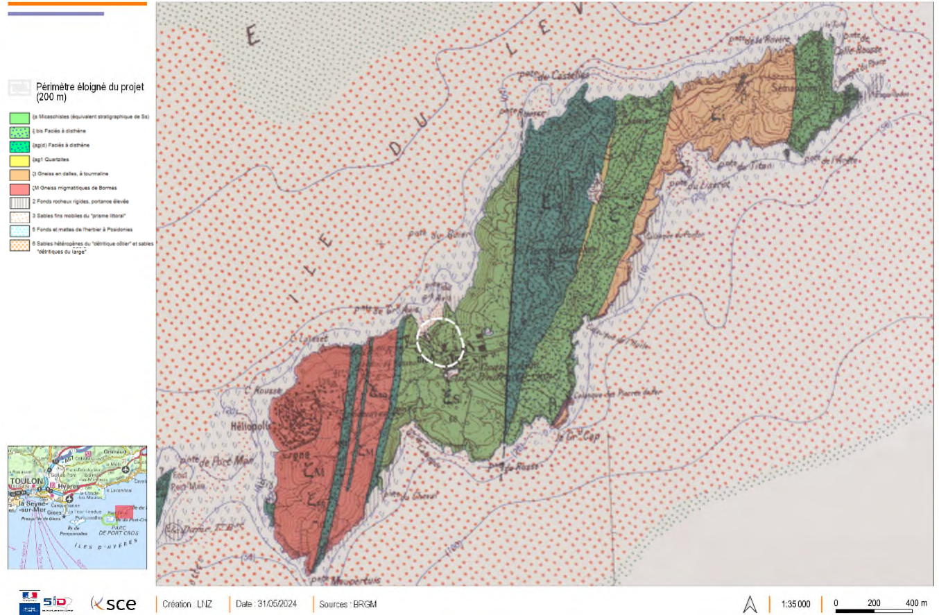
Figure 35 - Formations géologiques présentes sur l'île du Levant
