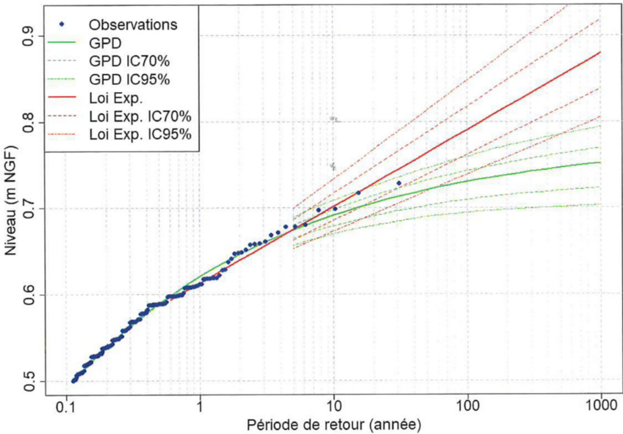
Figure 45 - Niveau d'eau extrême au port de Toulon (source : CEREMA, 2018)
