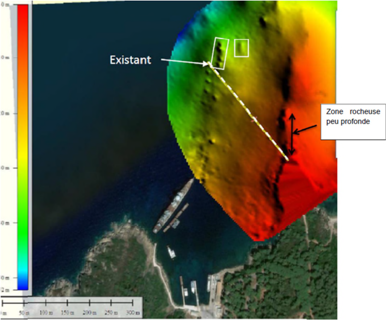
Figure 34 - Couverture du levé bathymétriques fourni dans le cadre de l'étude (source : OPSIA, 2019)
