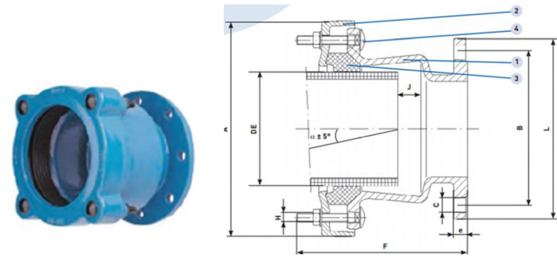
Figure 101 - Exemple d'adaptateur à bride très grande tolérance
