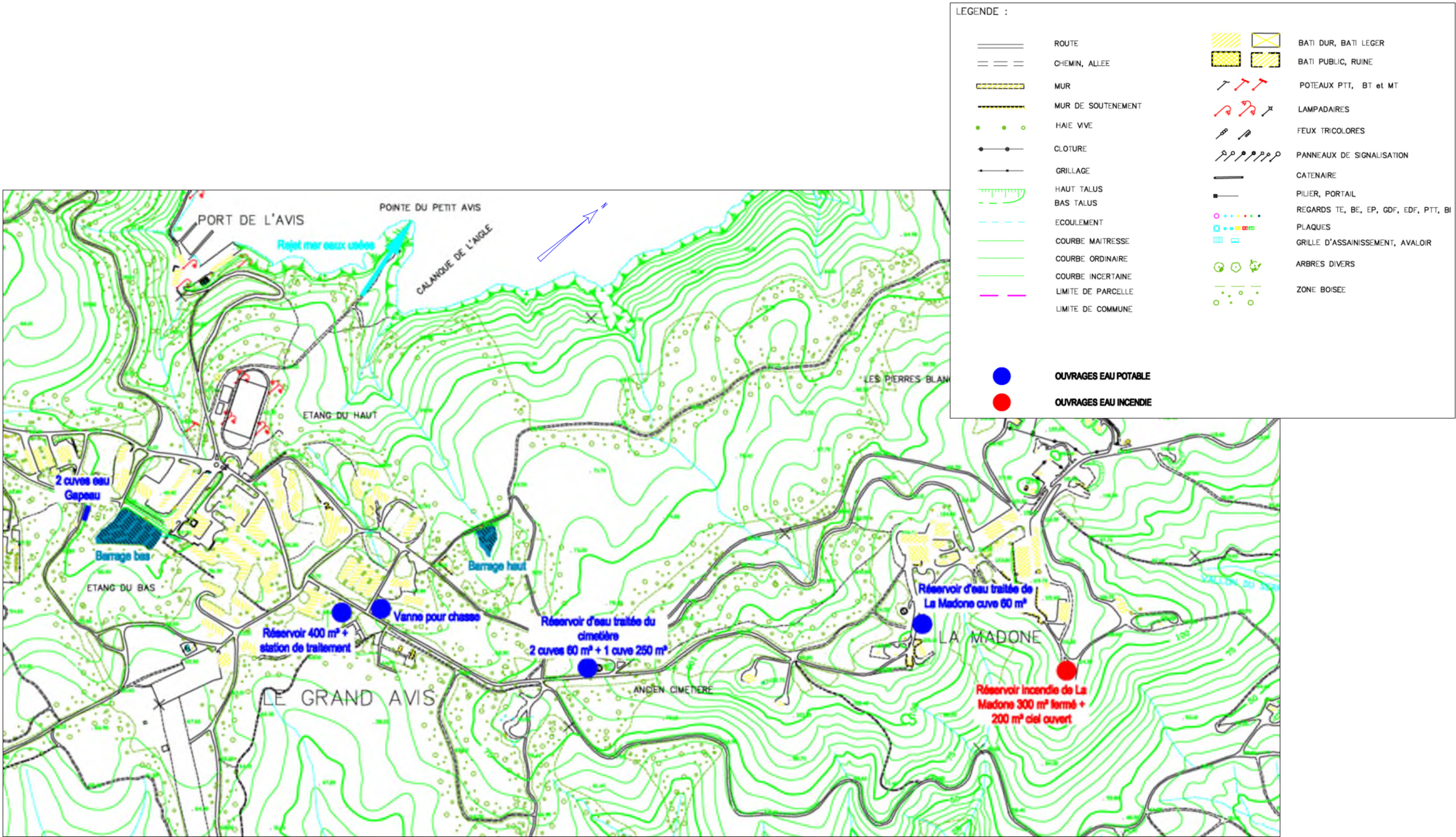
Figure 62 - Extrait du plan des installations du réseau d'adduction en eau potable et incendie (source : ERG Environnement)
