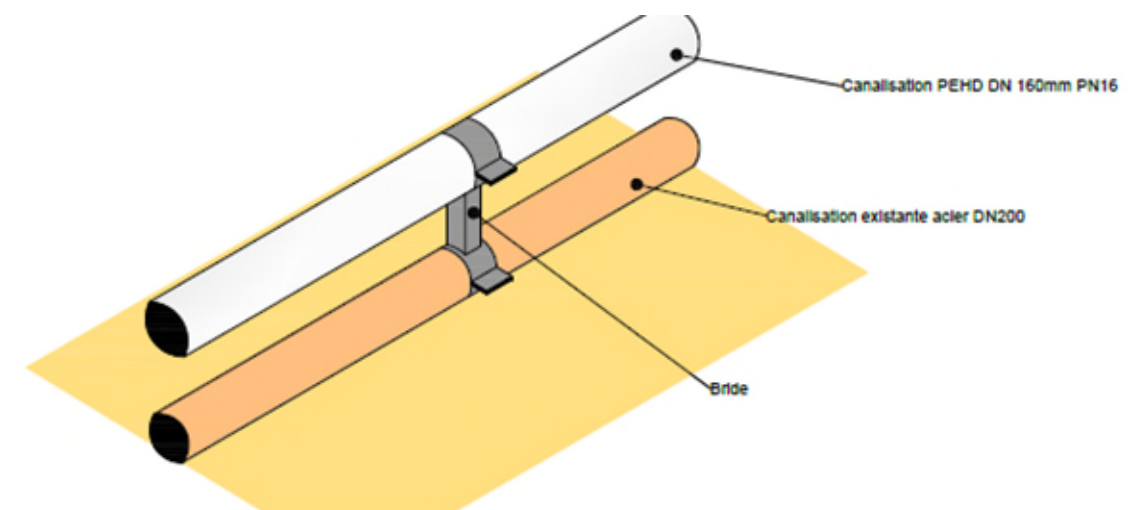
Figure 105 - Schéma du principe de fixation sur conduite existante
