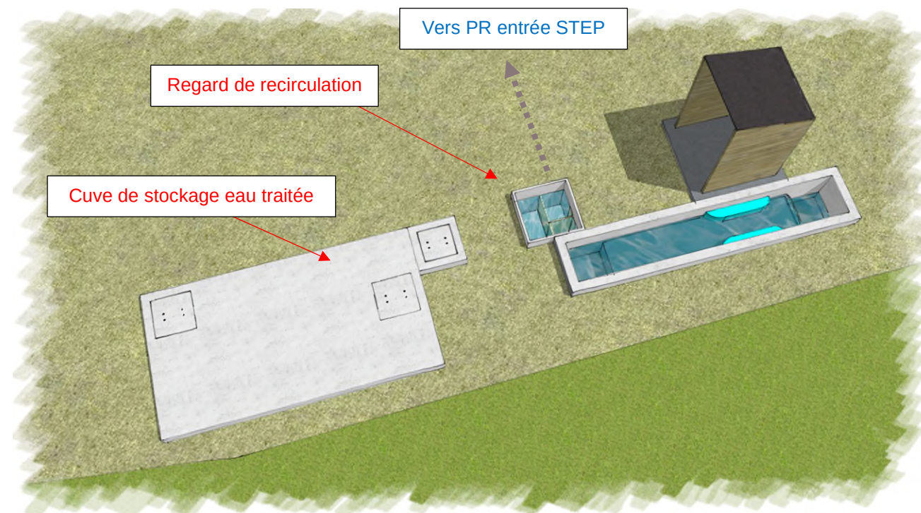
Figure 11 - Plans « Deuxième étage de filtration »
