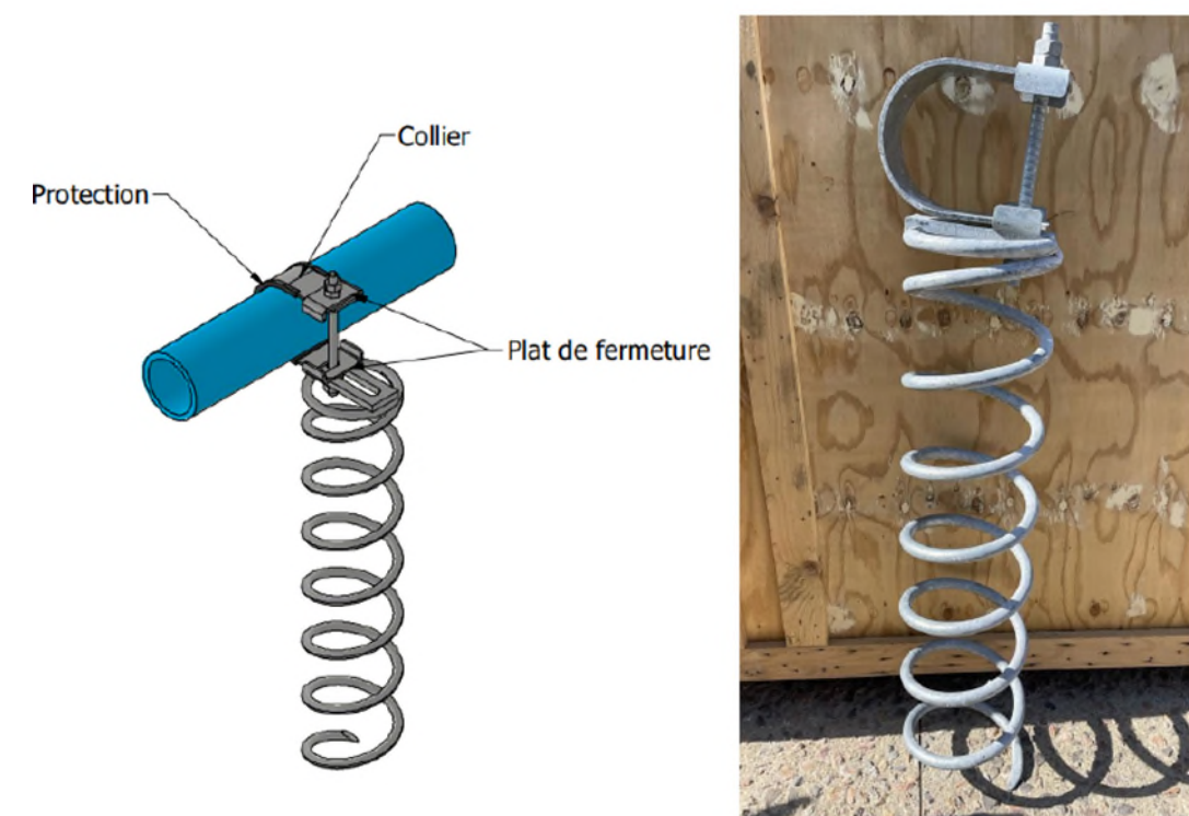
Système de fixation de l'émissaire
