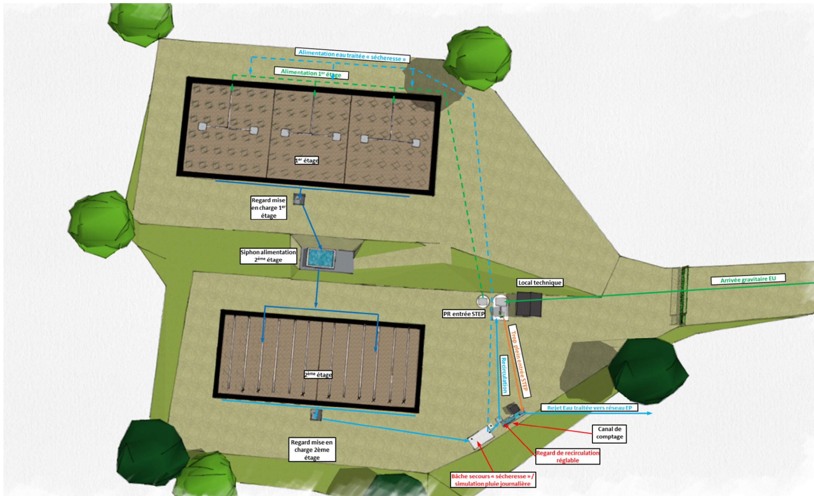
Figure 14 - Vue de dessus de la future STEP
