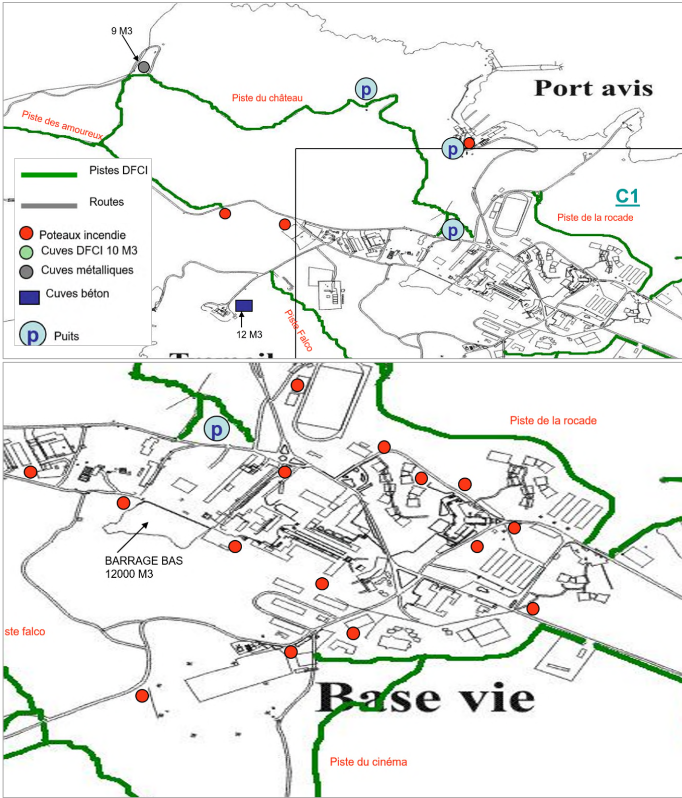
Figure 66 - Plan incendie du Levant (source : DGA)
