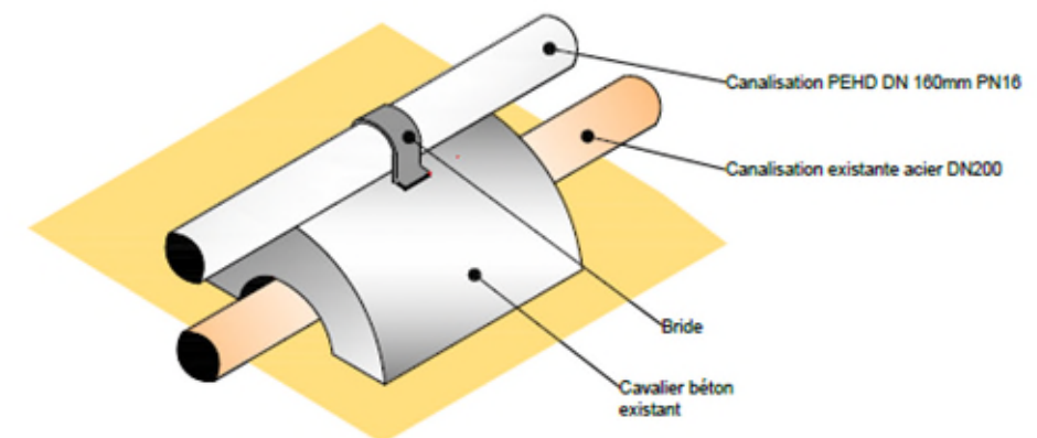
Figure 104 - Schéma du principe de pose et fixation conduite PEHD 160 sur cavalier béton existant
