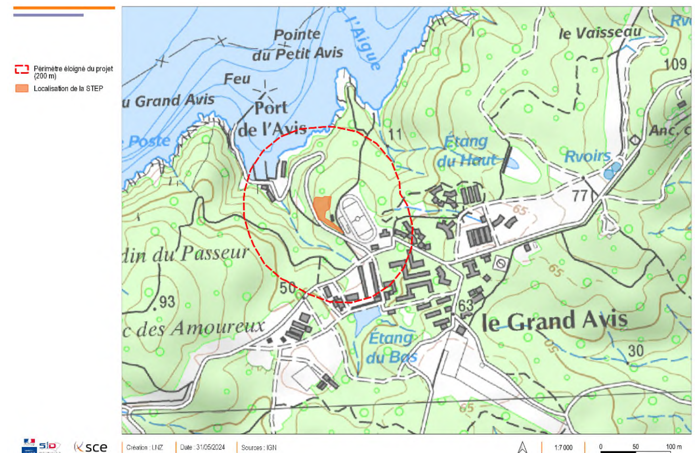
Figure 43 - Carte du réseau hydrographique
