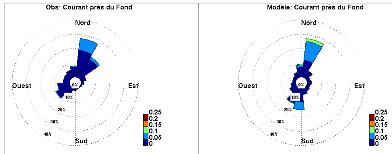
Figure 46 - Courants au fond (source : BONNA TP, 2020)
