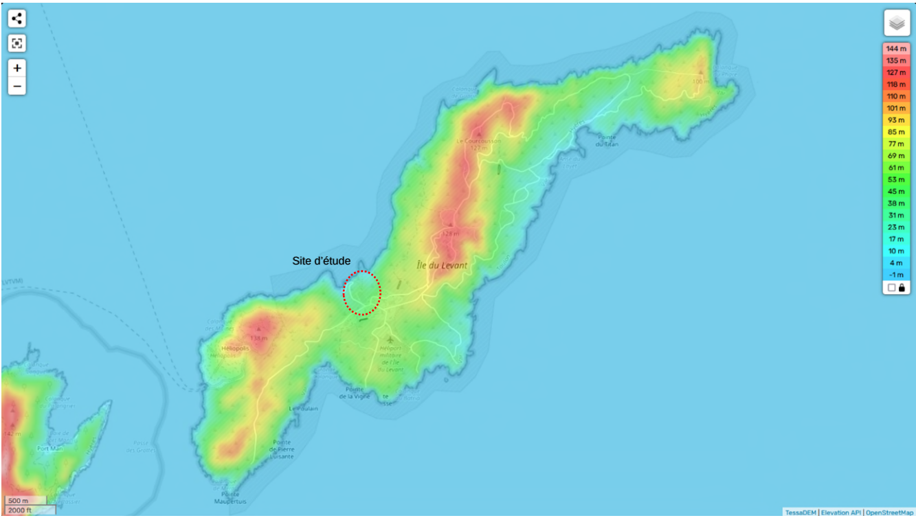
Figure 33 - Topographie du site d'étude (Source : Topographic-map.com)
