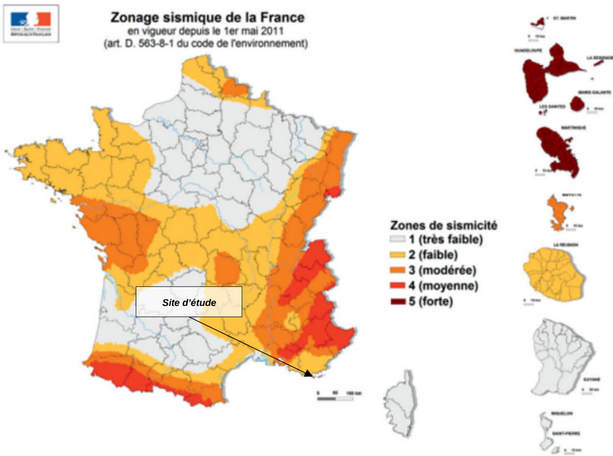
Figure 51 - Localisation du site d'étude sur la carte du zonage sismique de la France
