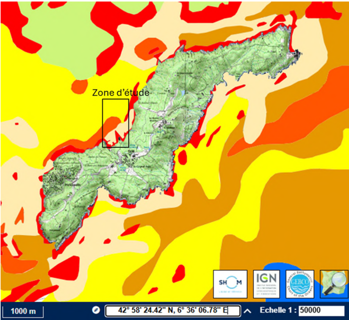
Figure 36 - Nature des fonds au 1/50 000e (source : SHOM)
