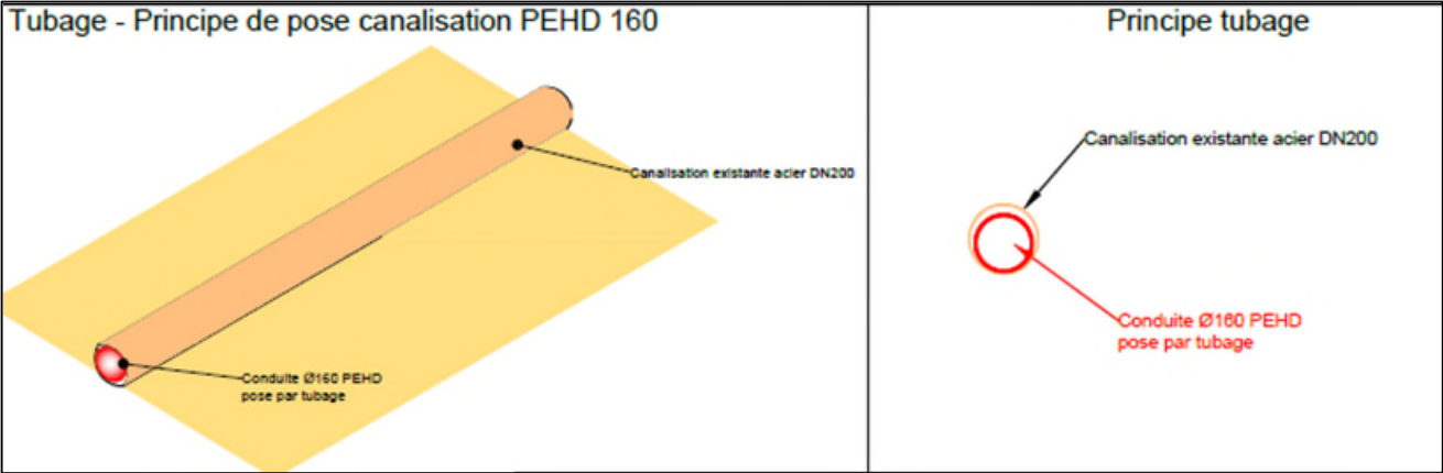
Figure 106 - Schéma du principe du tubage
