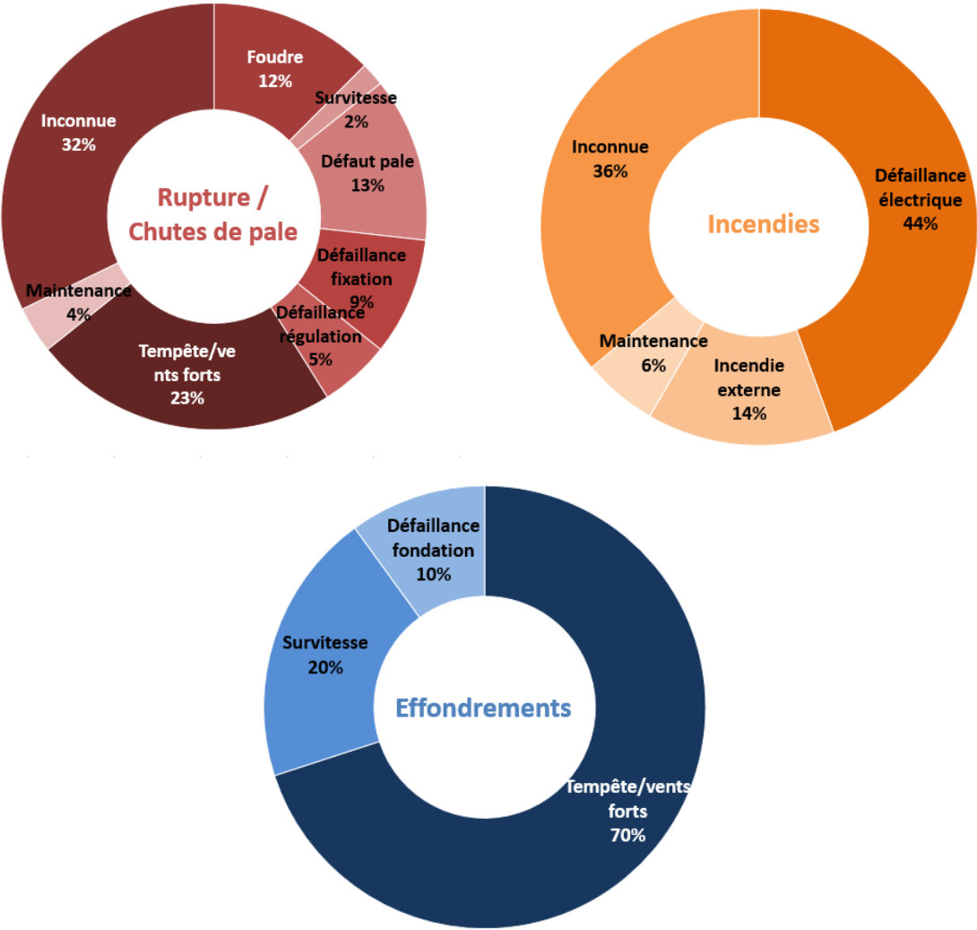
Figure 5 : Répartition par cause des principaux événements accidentels sur le parc éolien français entre 2000 et 2025 (Source : BEJC)
