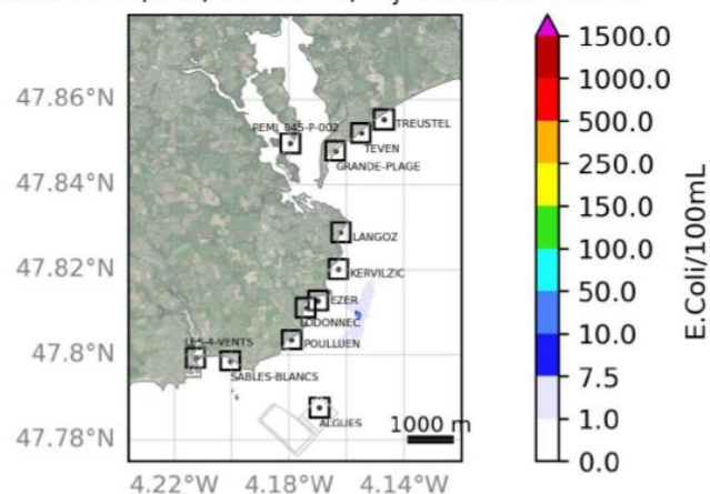
Figure 15 : Évolution de la concentration maximale en E. Coli dans le Scénario 7 (Rejet continu, VE, sans vent) – Impact du traitement bactériologique réduisant les rejets de 10^5 à 10^4 et 10^3 E. Coli/100 ml
