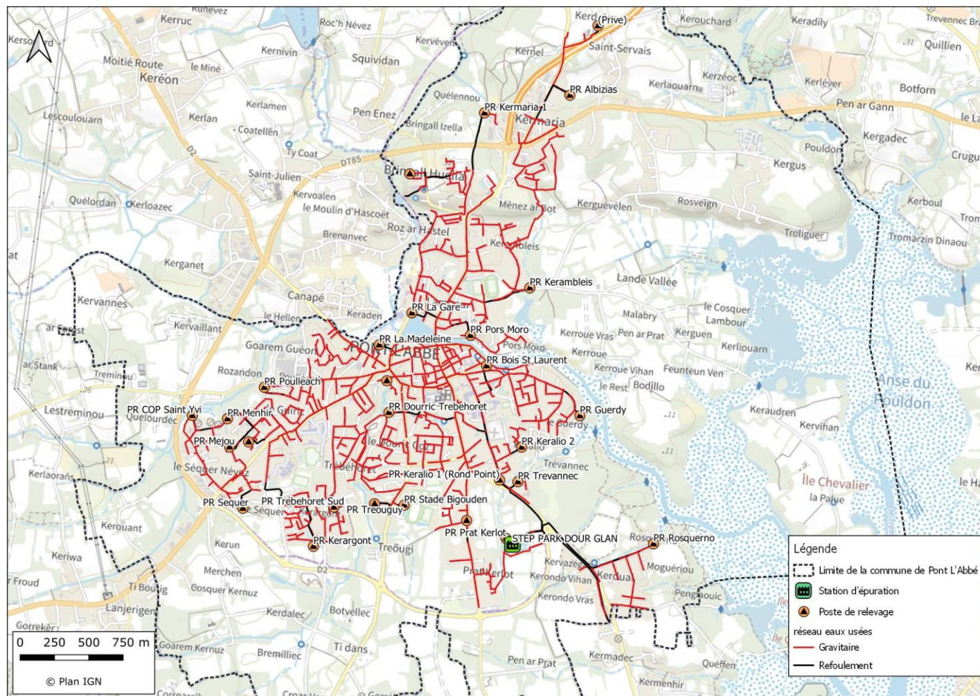
Figure 1 : Localisation du système d'assainissement et identification cadastrale de la station d'épuration de Pont l'Abbé
