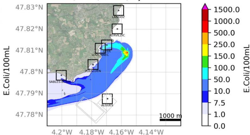
Concentrations maximales dans l'eau Scénario 5: VE, hiver, vent E, rejet continu à 10^4
