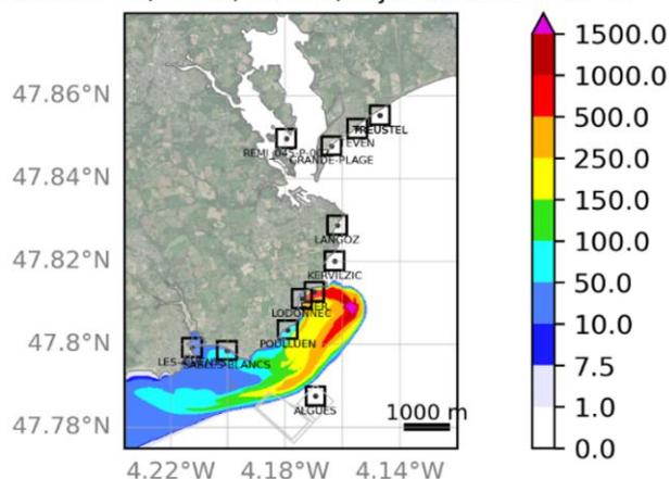
Concentrations maximales dans l'eau Scénario 5: VE, hiver, vent E, rejet continu à 10^5
