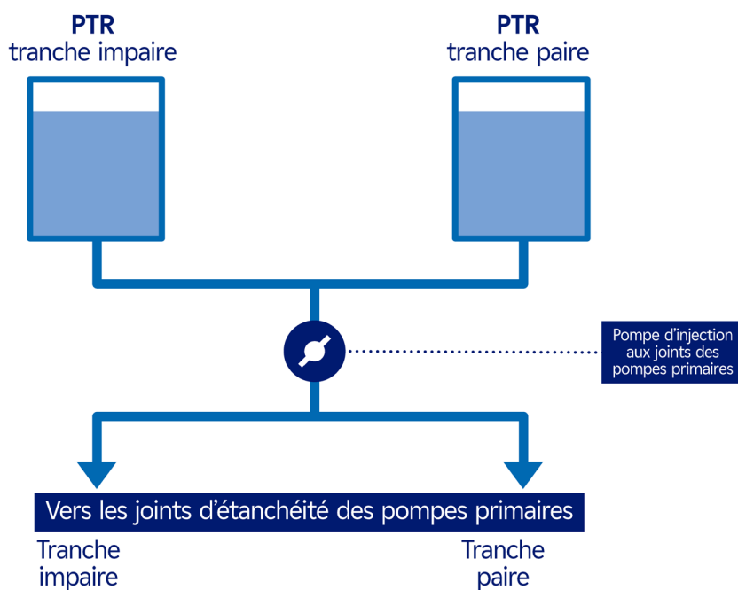
Figure 16. Configuration avant l'installation de la pompe d'injection aux joints «Noyau Dur» (PIJ-ND)
