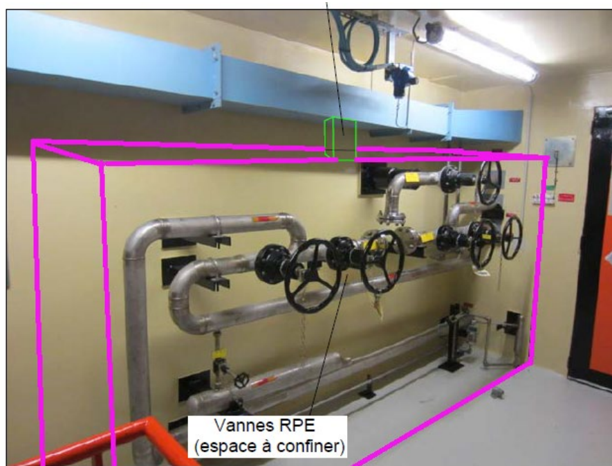
Figure 20. Création d'une enceinte ventilée raccordée à la filtration iode autour de certains équipements du système de collecte des effluents de l'îlot nucléaire (RPE) : photo du local et emplacement de la disposition
