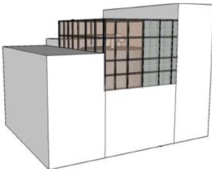
Figure 18. Protection contre la tornade «Noyau Dur» : photo de l'installation actuelle - exemple du réacteur n°1 de la centrale nucléaire du Tricastin et illustration de la disposition proposée, de type « grilles renforcées », autour de la bâche PTR cylindrique.
