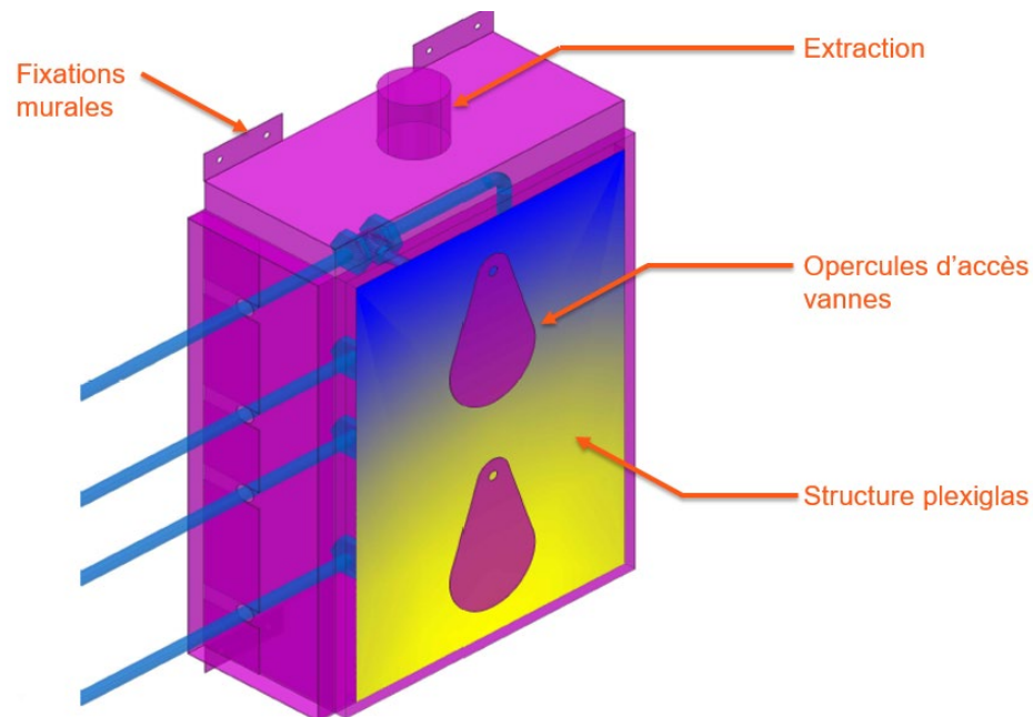
Figure 21. Création d'une enceinte ventilée raccordée à la filtration iode autour de certains équipements du système de collecte des effluents de l'îlot nucléaire (RPE) : illustration de la disposition
