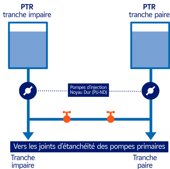
Figure 17. Configuration avec pompes d'injection aux joints «Noyau Dur» (PIJ-ND)
