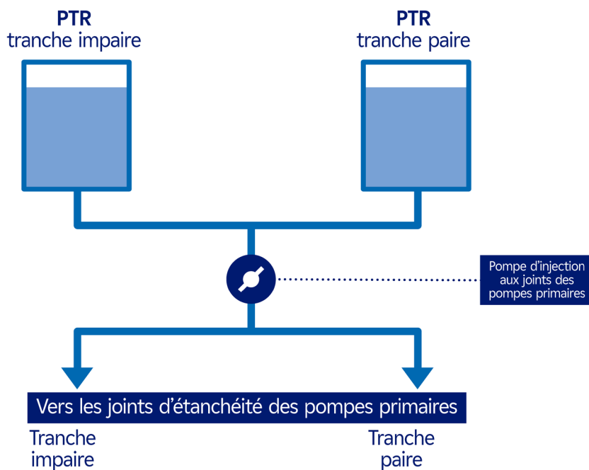
Figure 16. Configuration avant l'installation de la pompe d'injection aux joints «Noyau Dur» (PIJ-ND)
