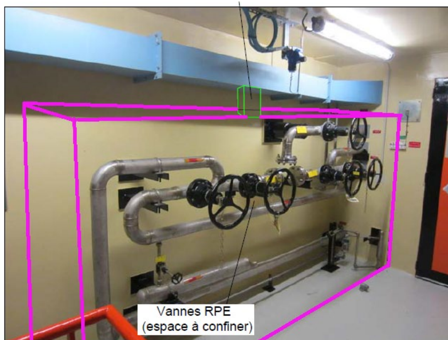
Figure 20. Création d'une enceinte ventilée raccordée à la filtration iode autour de certains équipements du système de collecte des effluents de l'îlot nucléaire (RPE) : photo du local et emplacement de la disposition
