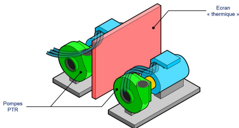
Figure 7. Installation d'un écran thermique entre les pompes du système de refroidissement de la piscine d'entreposage du combustible
