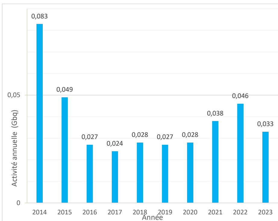
Figure 5 : Activité en iodes rejetée à l'atmosphère par le CNPE du Blayais sur la période 2014 – 2023 (GBq/an)
