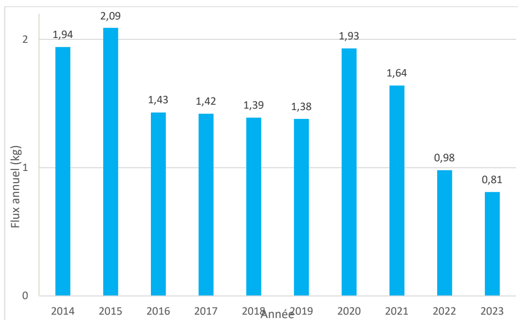
Figure 10 : Rejets annuels d'hydrazine sur la période 2014-2023 du CNPE du Blayais
