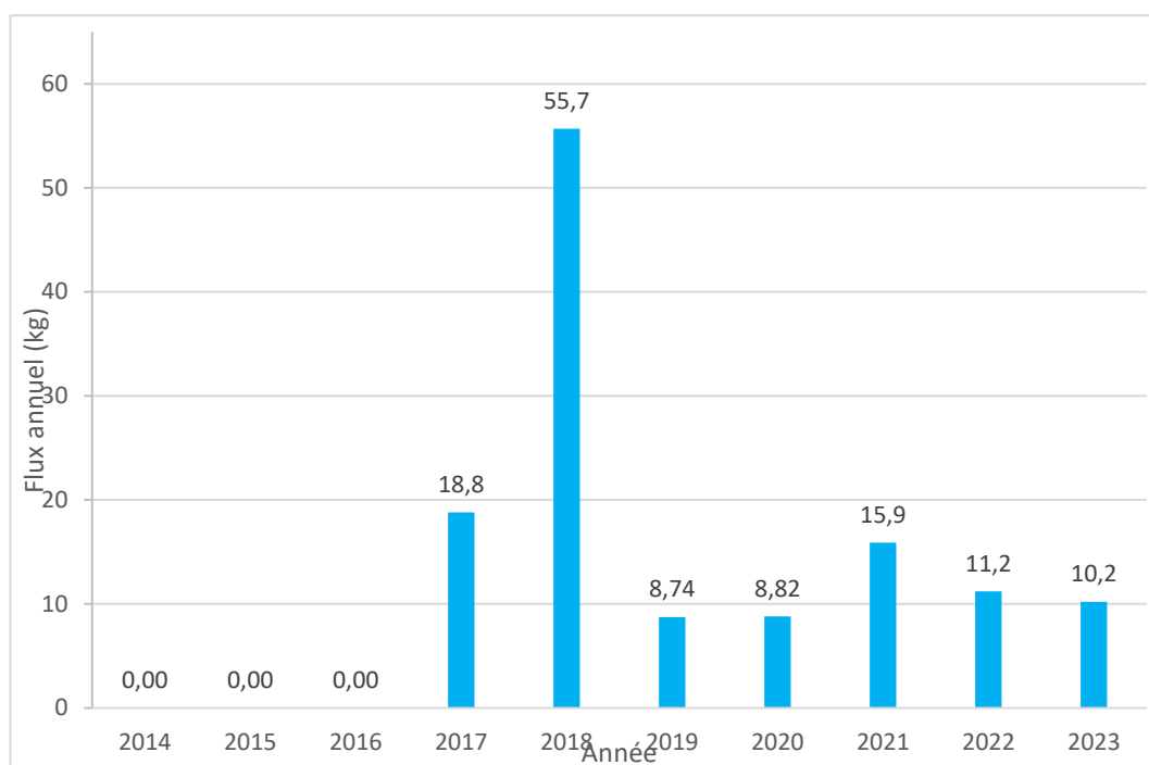
Figure 12 : Rejets annuels d'éthanolamine du CNPE du Blayais sur la période 2014- 2023
