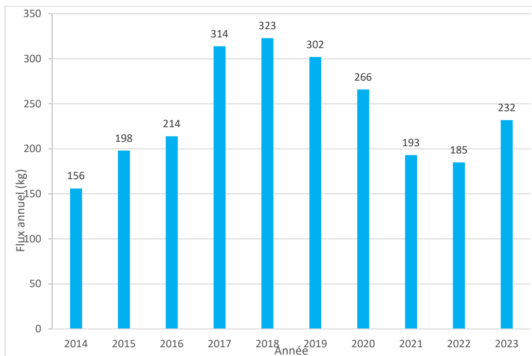
Figure 14 : Rejets annuels en phosphates du CNPE du Blayais sur la période 2014- 2023
