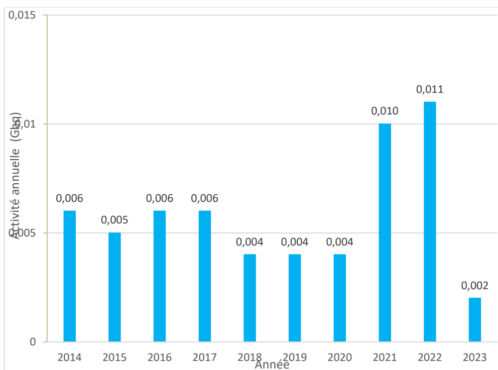
Figure 7 : Activité en autres PF/PA rejetée à l'atmosphère par le CNPE du Blayais sur la période 2014-2023 (GBq/an)
