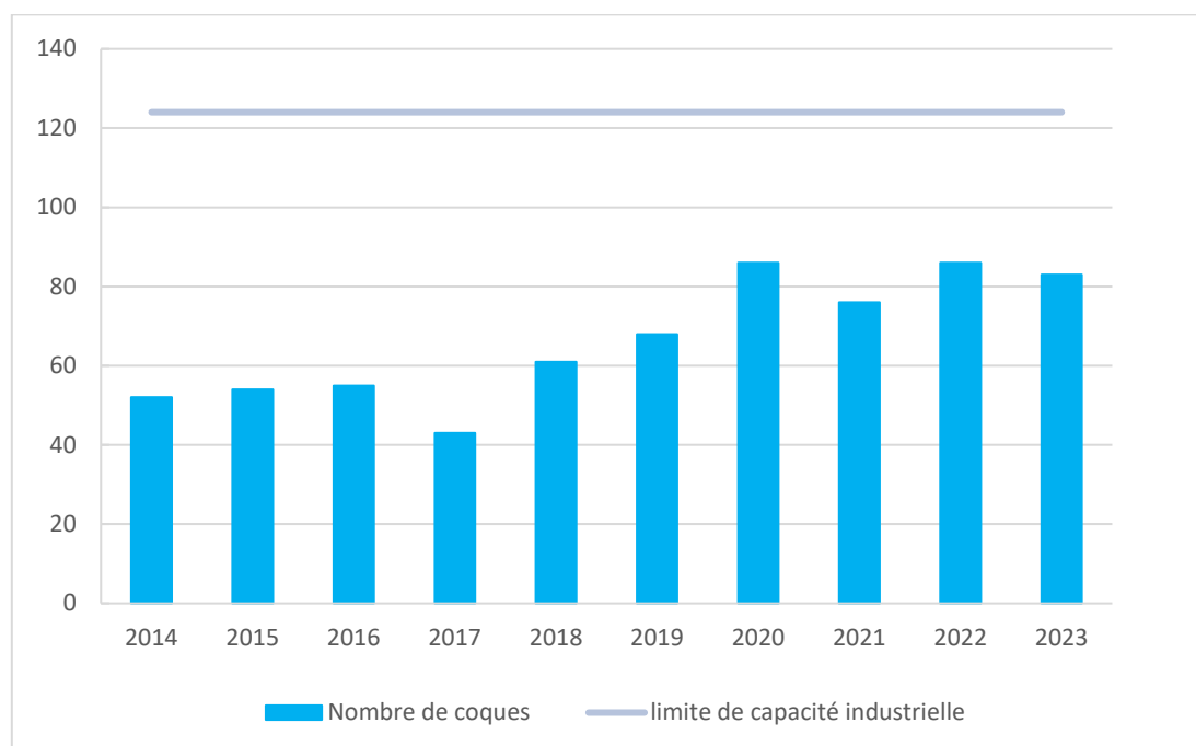
Figure 15 : Évolution du nombre de coques entreposées sur la période 2014 – 2023
