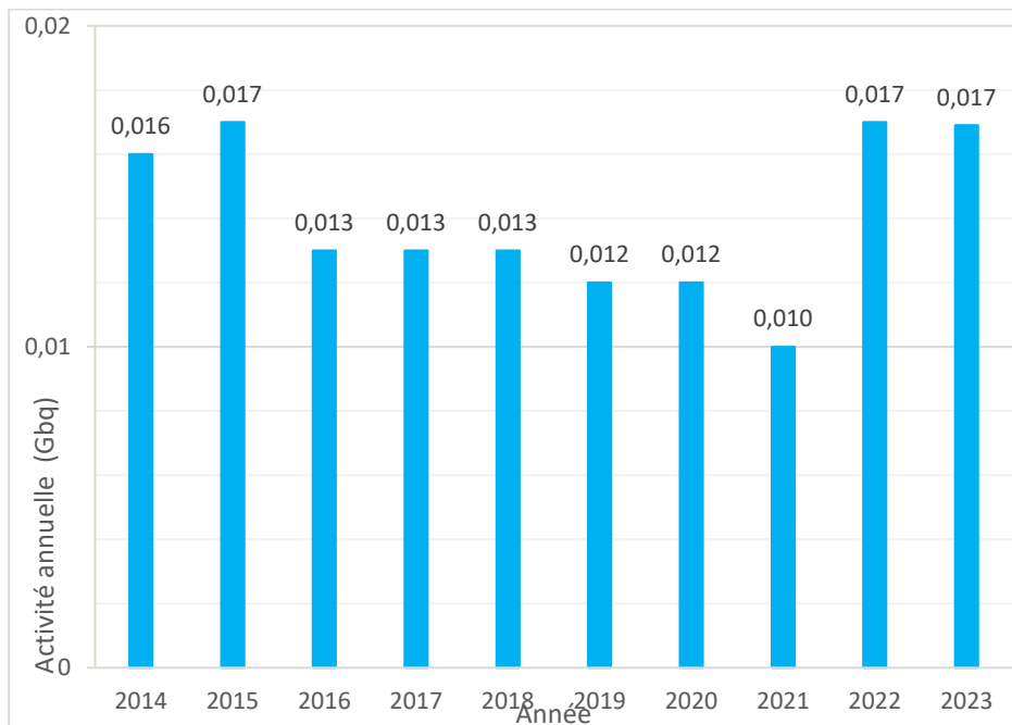
Figure 6 : Activité en iodes rejetée dans les effluents liquides du CNPE du Blayais sur la période 2014 – 2023 (GBq/an)
