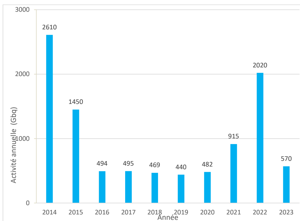
Figure 4 : Activité en gaz rares rejetée à l'atmosphère du CNPE du Blayais sur la période 2014 – 2023 (GBq/an)
