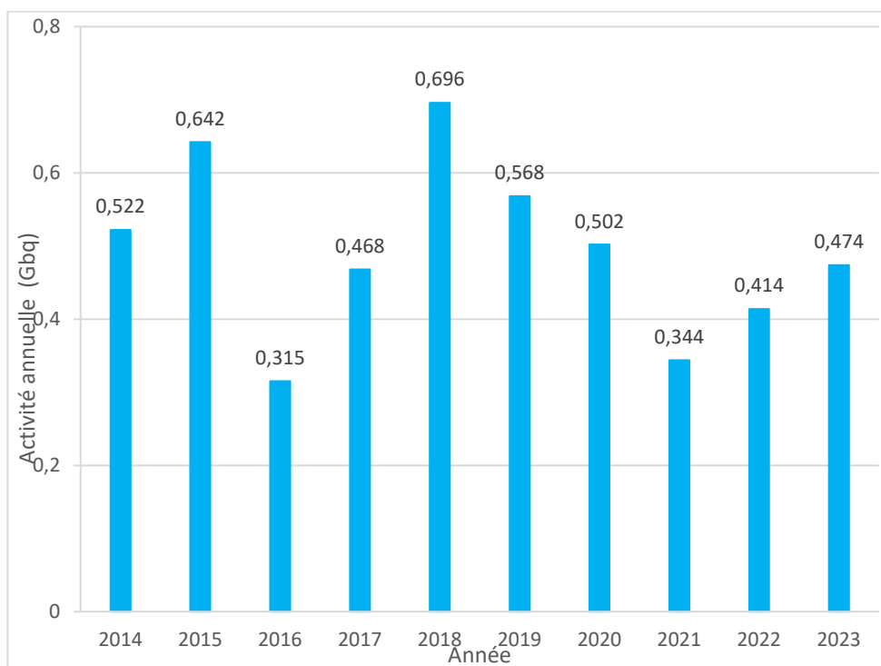
Figure 8 : Activité en autres PF/PA rejetée dans les effluents liquides du CNPE du Blayais sur la période 2014-2023 (GBq/an)
