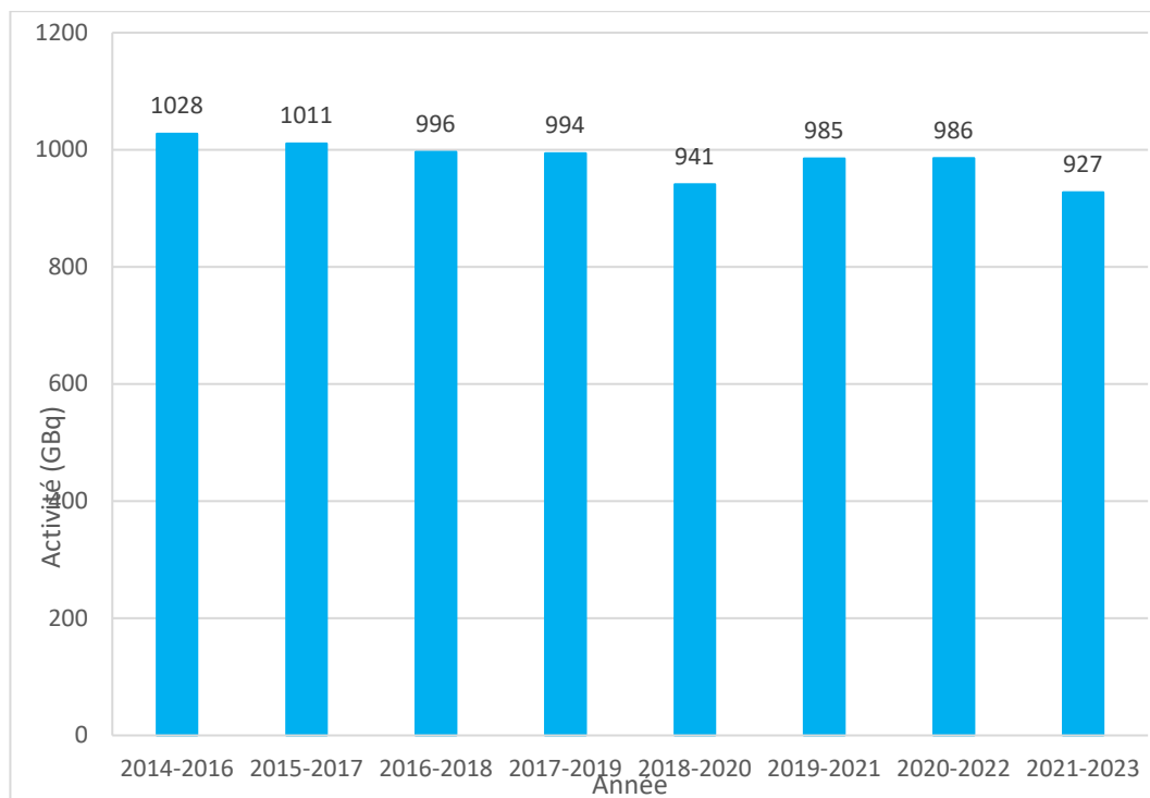
Figure 3 : Activité en tritium rejetée à l'atmosphère, moyenne sur 3 années glissantes sur la période 2014 – 2023, du CNPE du Blayais (GBq/an)
