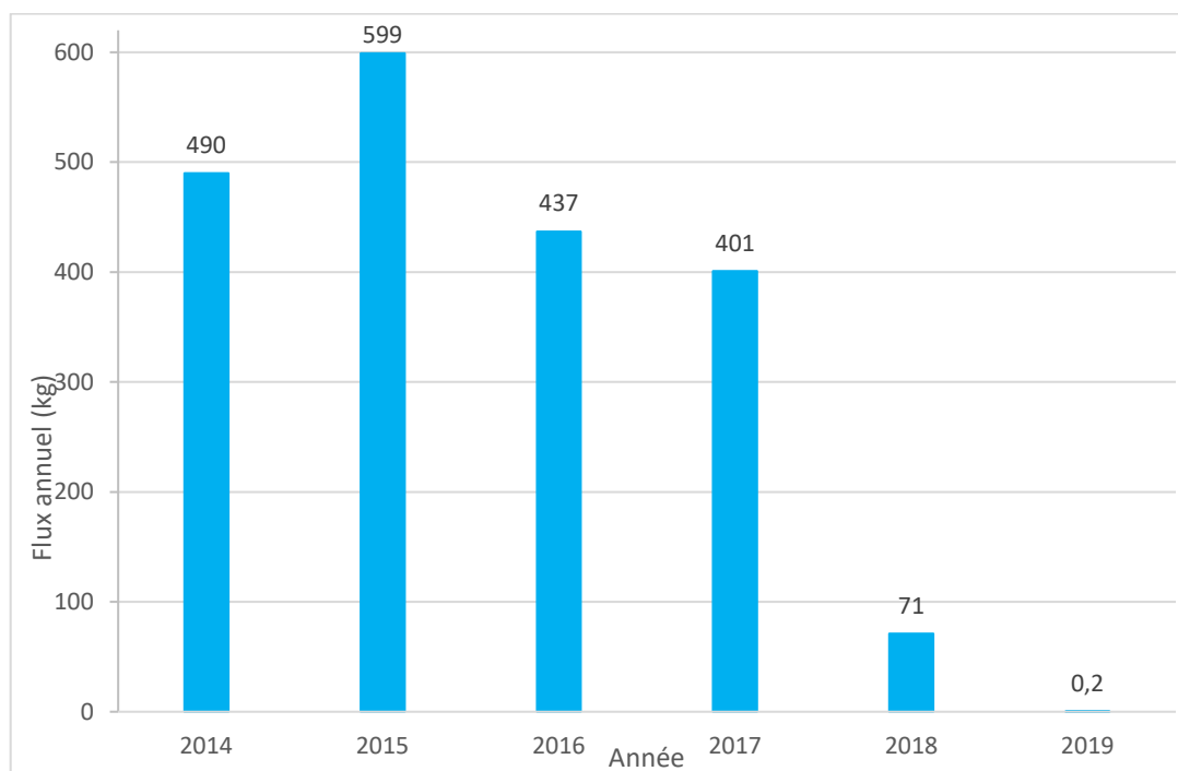
Figure 11 : Rejets annuels de morpholine sur la période 2014-2019 du CNPE du Blayais
