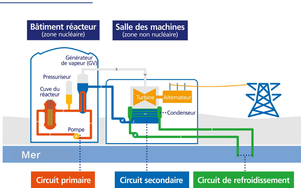
Figure 5. Schéma de principe de fonctionnement de la centrale nucléaire, sans aéroréfrigérant
