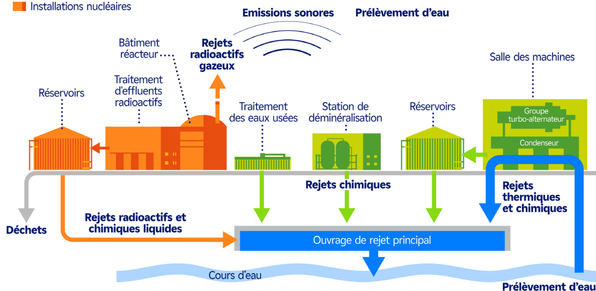
Figure 21. Représentation des inconvénients selon les parties de l'installation Source froide en circuit « ouvert »
