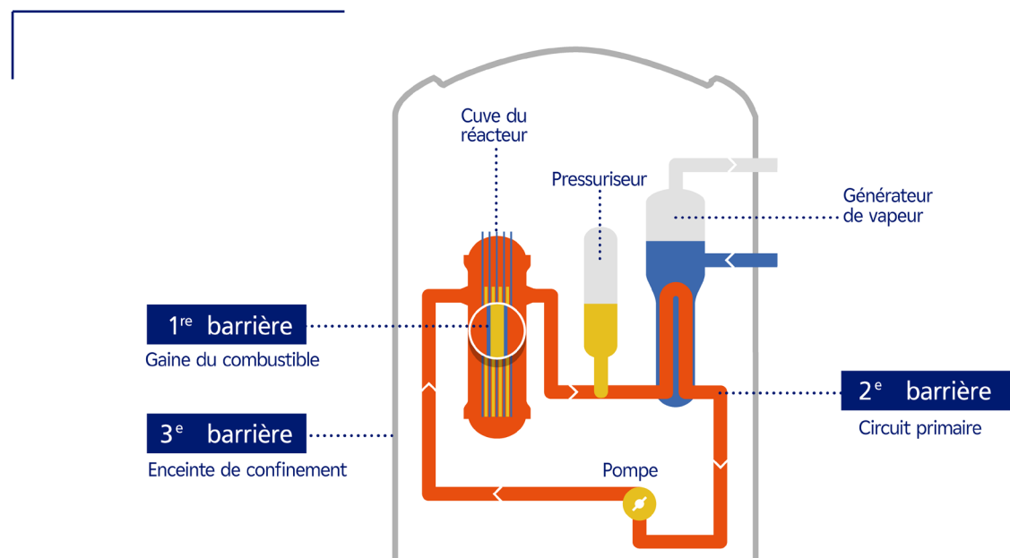
Figure 6. Schéma des trois barrières de confinement
