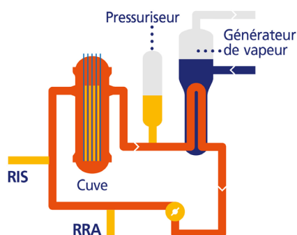
Figure 7. Schéma des trois fonctions de sûreté
