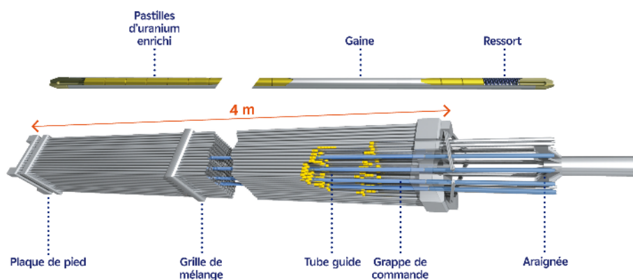
Figure 11. Schéma d'un assemblage combustible
