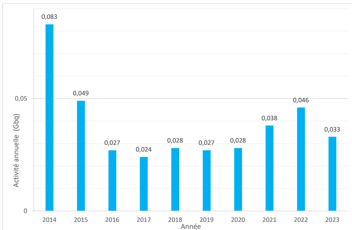
Figure 22. Activité en iodes rejetée à l'atmosphère sur la période 2014-2023 de la centrale nucléaire du Blayais
