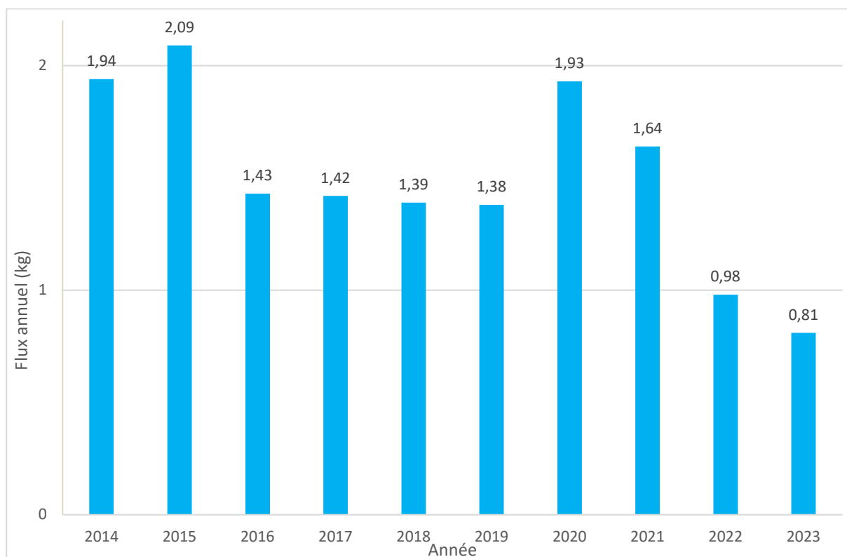
Figure 23. Rejets annuels d'hydrazine sur la période 2014 - 2023 de la centrale nucléaire du Blayais
