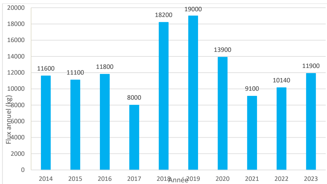
Figure 9 : Rejets annuels d'acide borique sur la période 2014-2023 du CNPE du Blayais
