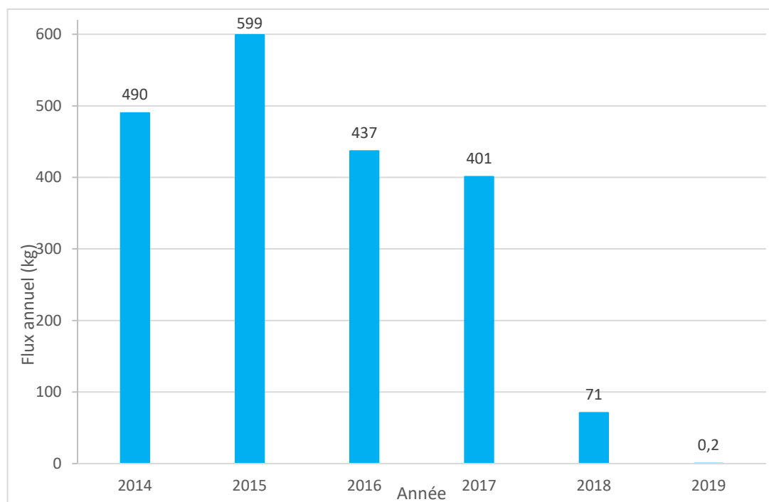
Figure 11 : Rejets annuels de morpholine sur la période 2014-2019 du CNPE du Blayais
