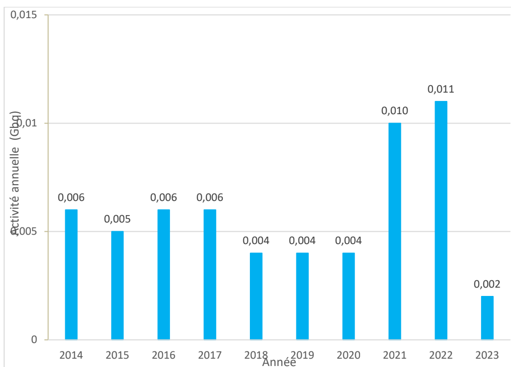
Figure 7 : Activité en autres PF/PA rejetée à l'atmosphère par le CNPE du Blayais sur la période 2014-2023 (GBq/an)
