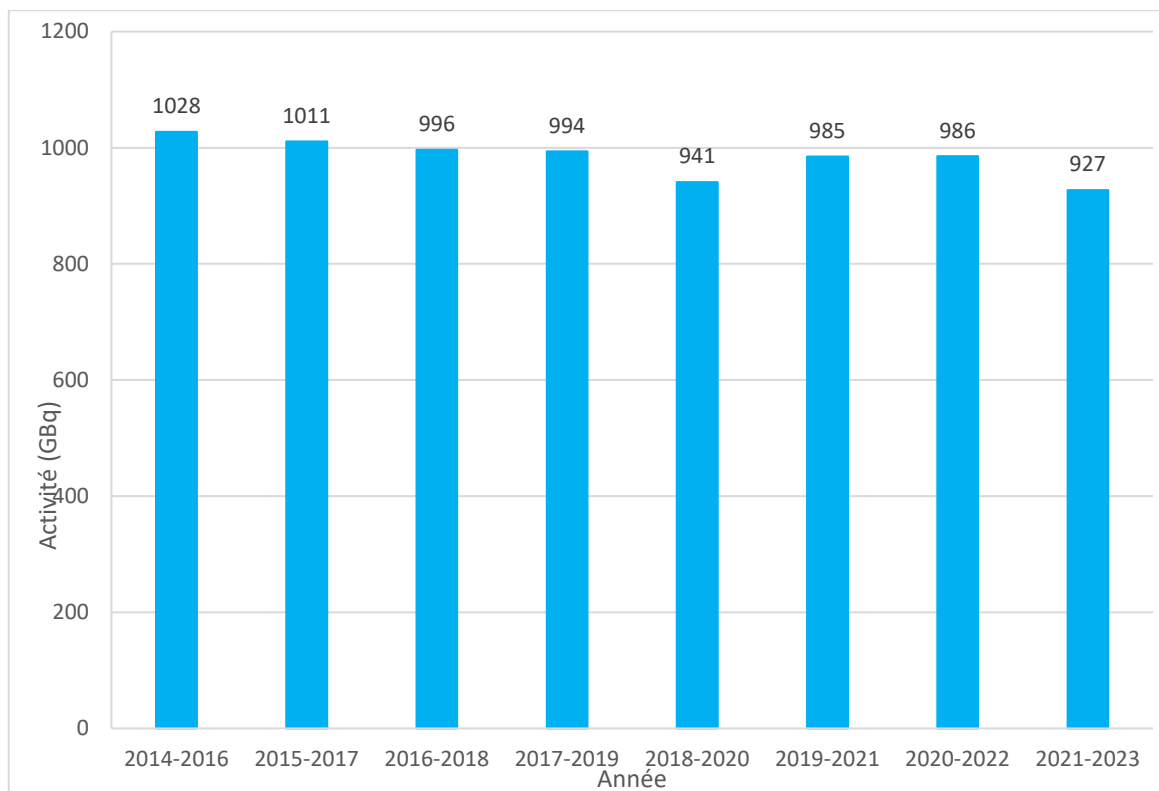
Figure 3 : Activité en tritium rejetée à l'atmosphère, moyenne sur 3 années glissantes sur la période 2014 – 2023, du CNPE du Blayais (GBq/an)
