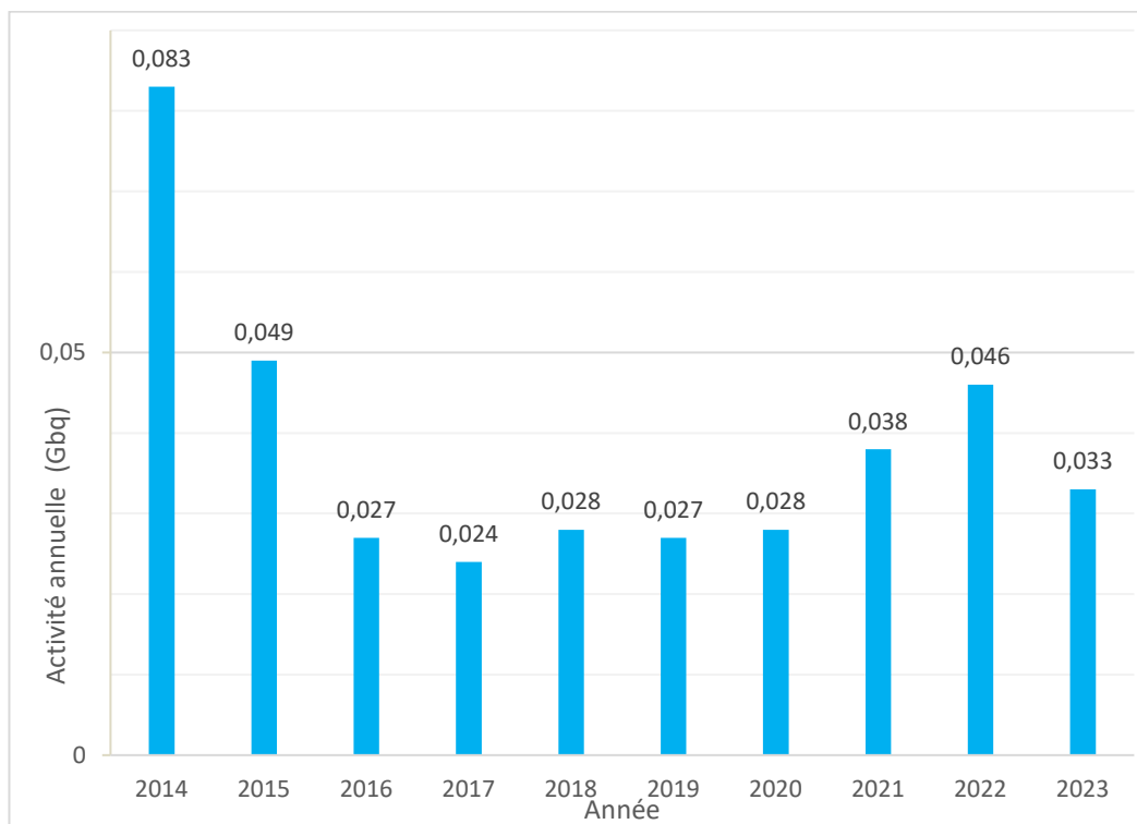
Figure 5 : Activité en iodes rejetée à l'atmosphère par le CNPE du Blayais sur la période 2014 – 2023 (GBq/an)
