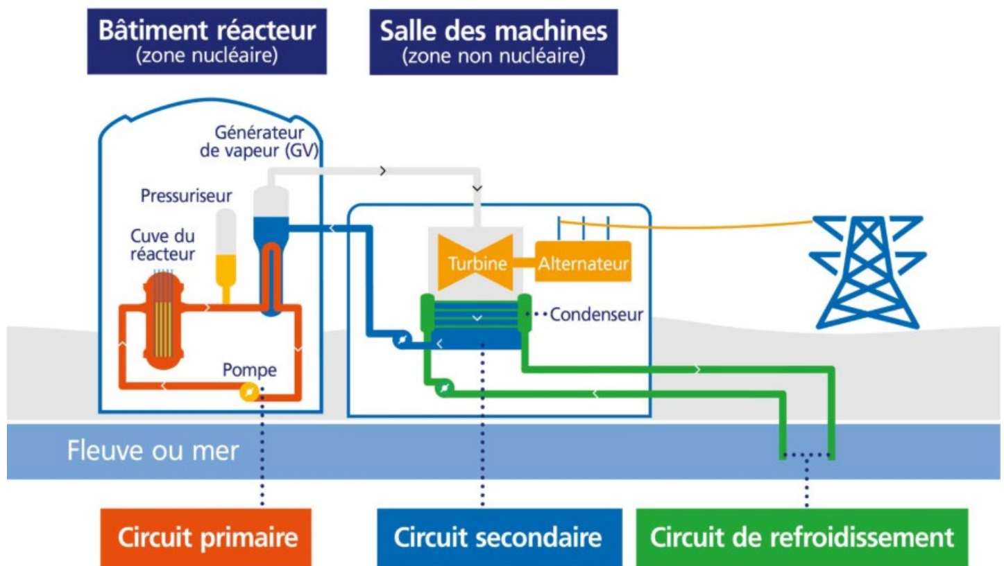
Figure 24. Principes de fonctionnement d'une centrale nucléaire sans aéroréfrigérant
