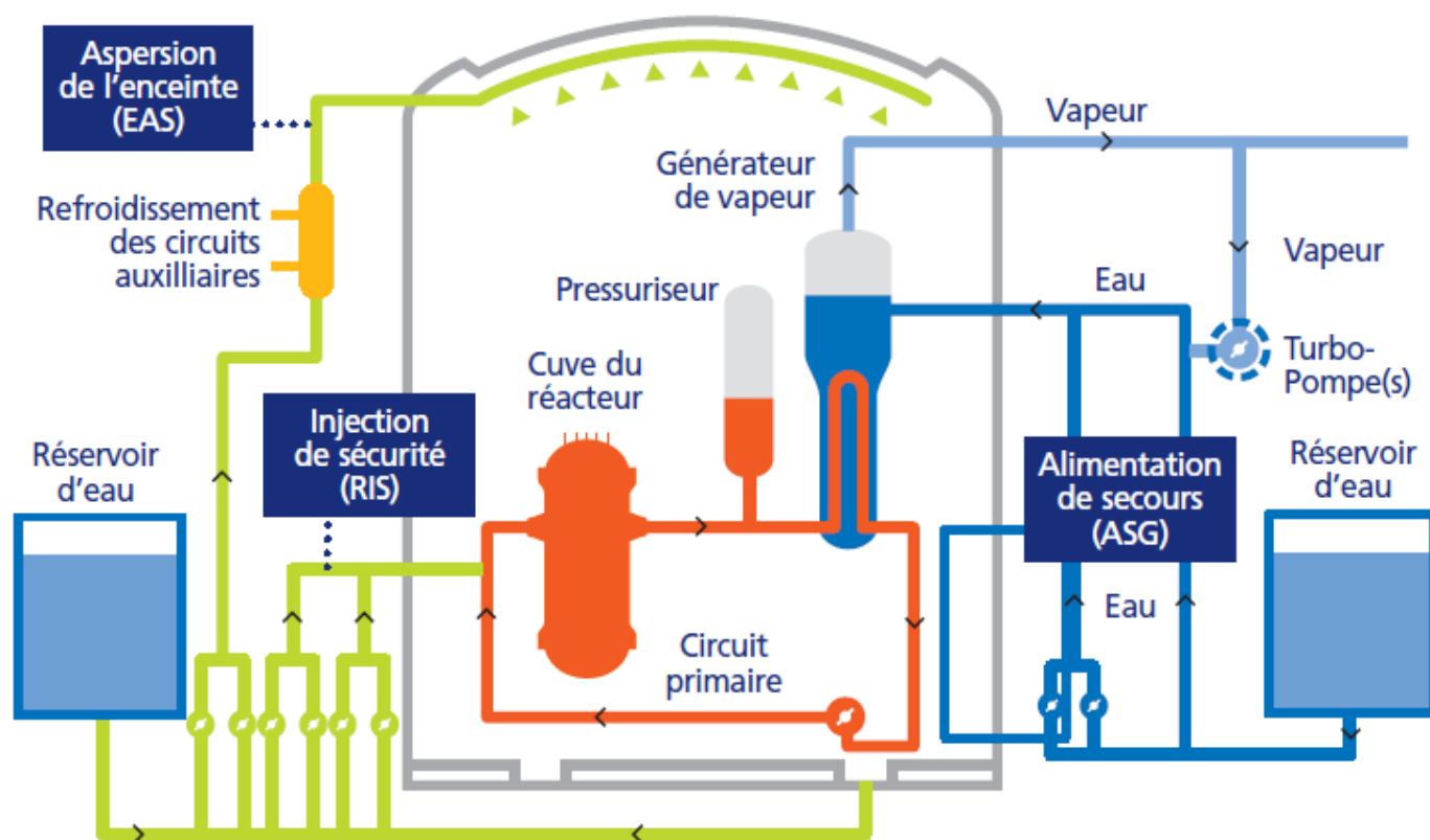
Figure 26. Schéma des systèmes de sauvegarde : 3 principaux circuits (ASG, RIS, EAS)
