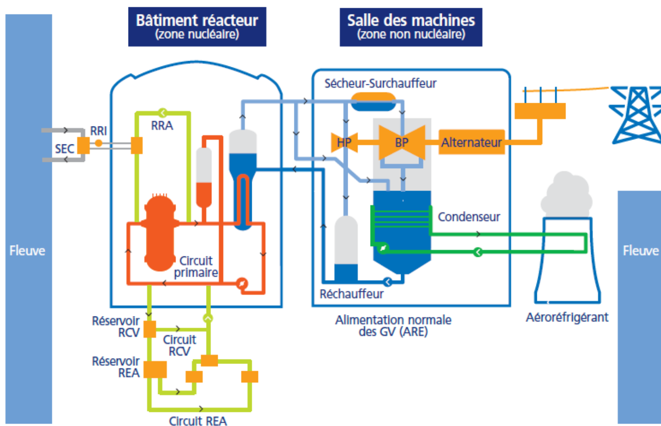
Figure 25. Schéma de réacteur en fonctionnement normal : principaux circuits annexes
