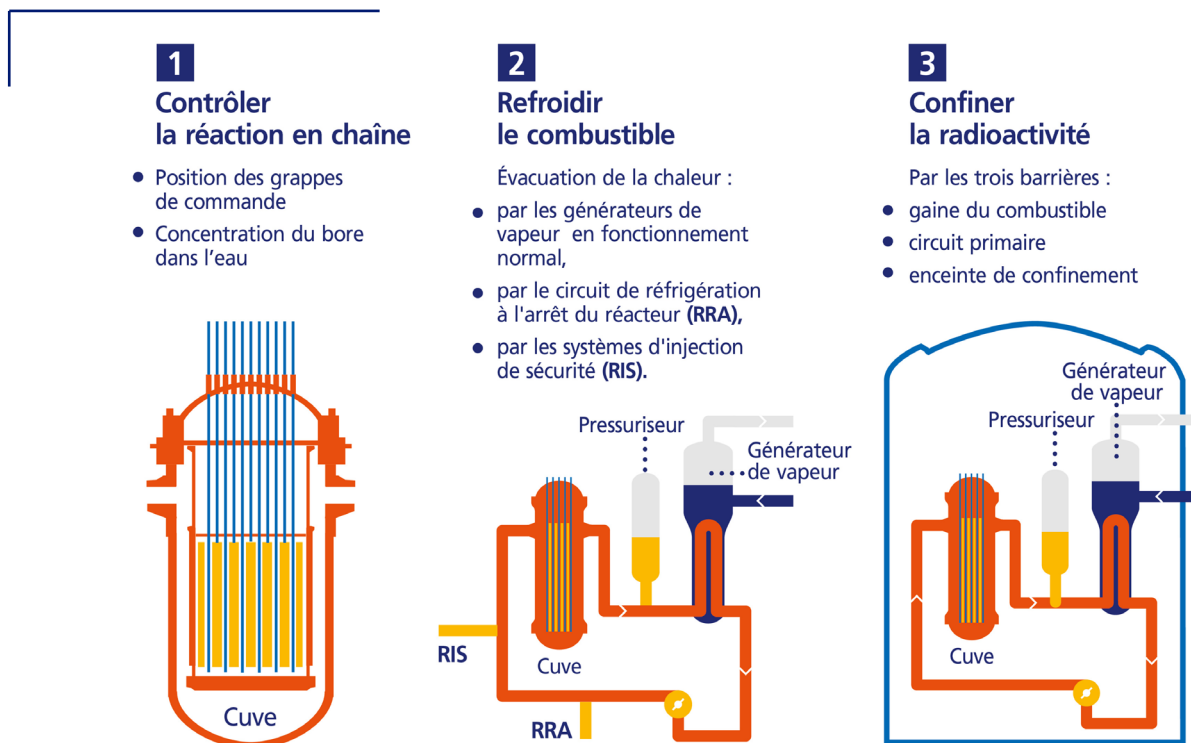
Figure 7. Schéma des trois fonctions de sûreté
