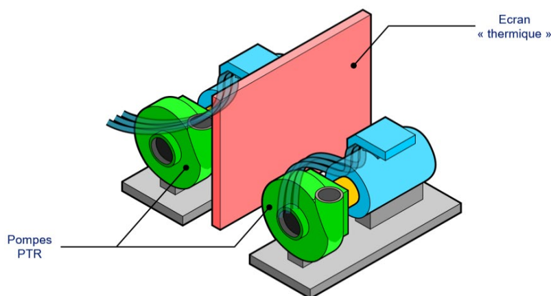
Figure 8. Installation d'un écran thermique entre les pompes du système de refroidissement de la piscine d'entreposage du combustible
