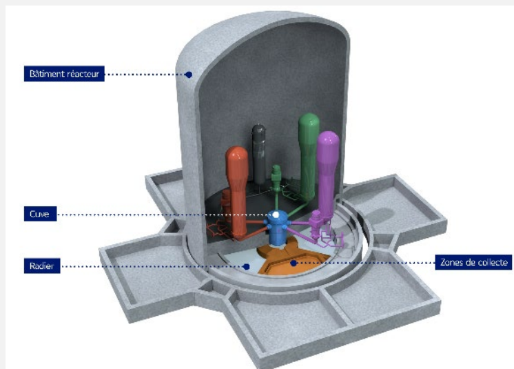
Schéma de principe issu de l'EPR
