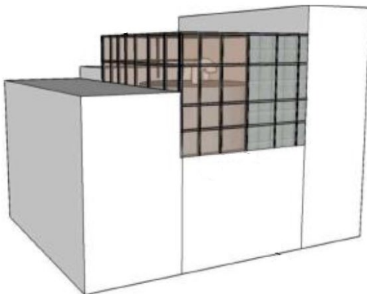
Figure 19. Protection contre la tornade «Noyau Dur» : photo de l'installation actuelle - exemple du réacteur n° 1 de la centrale nucléaire du Tricastin et illustration de la disposition proposée, de type « grilles renforcées », autour de la bâche PTR cylindrique.
