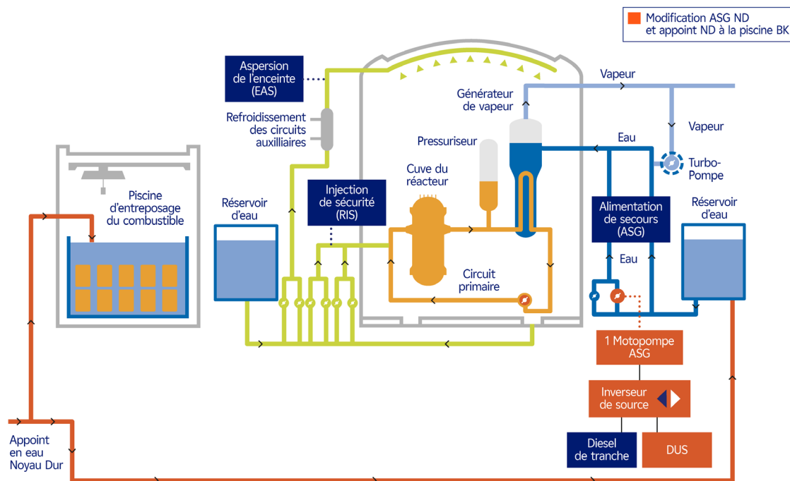
Figure 16. Schéma de principe de la disposition ASG-ND et appoint «Noyau Dur» aux piscines réacteur et combustible
