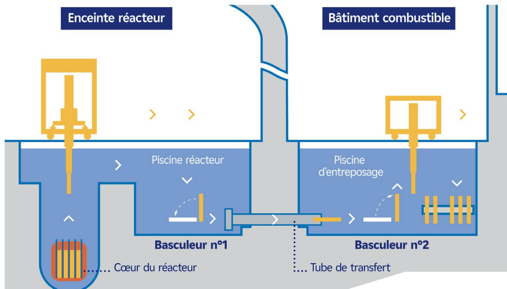
Figure 9. Piscine du bâtiment réacteur et piscine d'entreposage du combustible (illustration du transfert d'un assemblage de combustible du cœur du réacteur vers la piscine d'entreposage)
