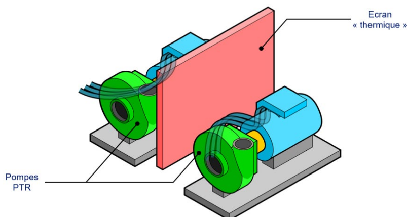
Figure 8. Installation d'un écran thermique entre les pompes du système de refroidissement de la piscine d'entreposage du combustible
