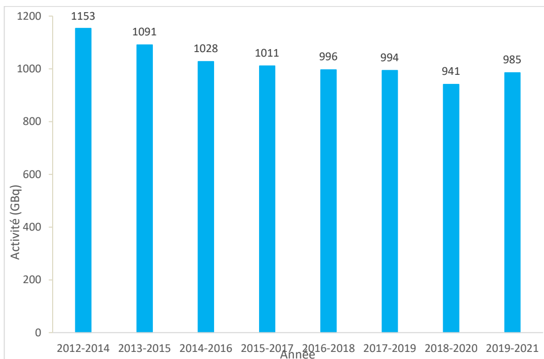
Figure 3 : Activité en tritium rejetée à l'atmosphère, moyenne sur 3 années glissantes sur la période 2012 – 2021, du CNPE du Blayais (GBq/an)
