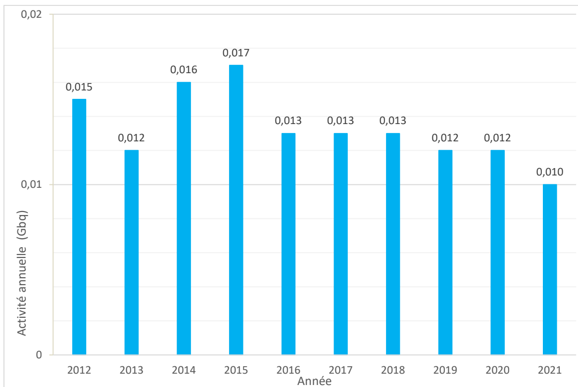
Figure 6 : Activité en iodes rejetée dans les effluents liquides du CNPE du Blayais sur la période 2012 – 2021 (GBq/an)
