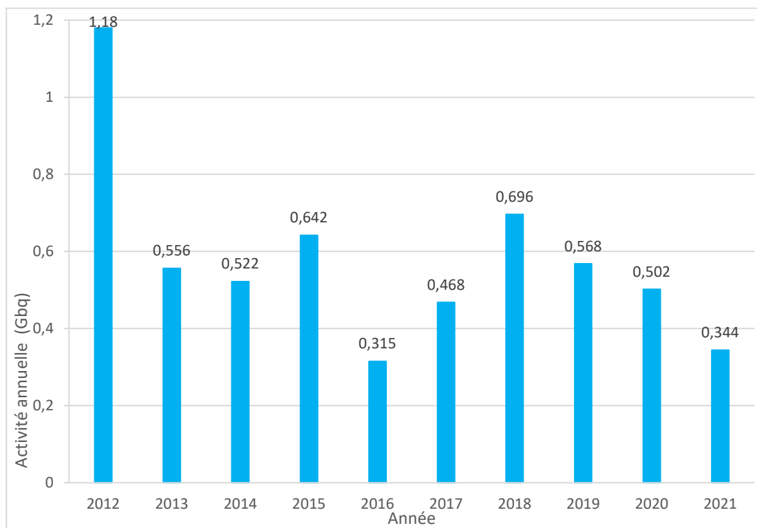
Figure 8 : Activité en autres PF/PA rejetée dans les effluents liquides du CNPE du Blayais sur la période 2012-2021 (GBq/an)
