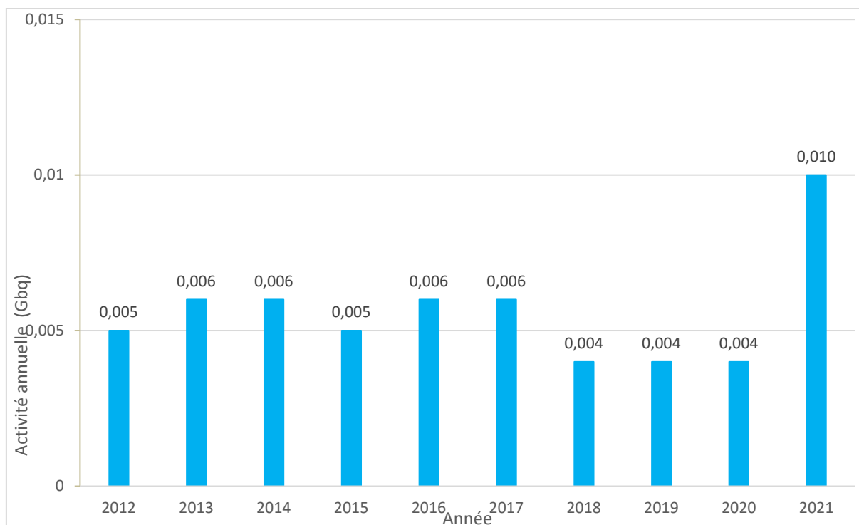
Figure 7 : Activité en autres PF/PA rejetée à l'atmosphère par le CNPE du Blayais sur la période 2012-2021 (GBq/an)
