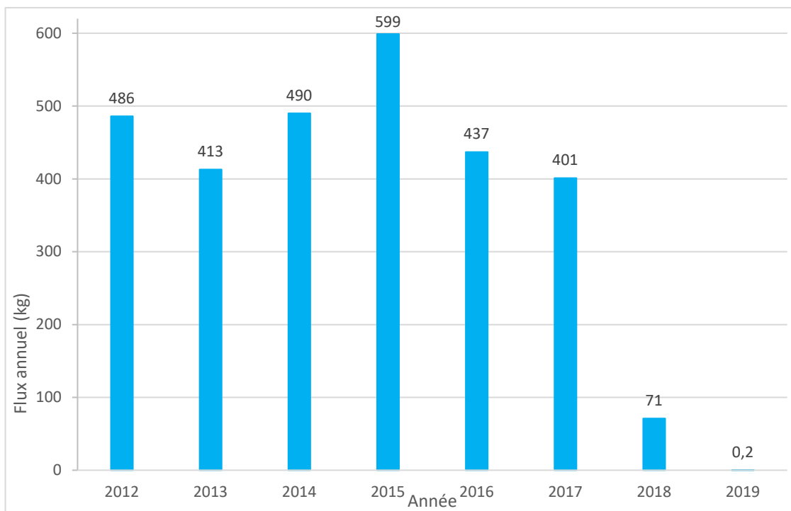
Figure 11 : Rejets annuels de morpholine sur la période 2012-2019 du CNPE du Blayais
