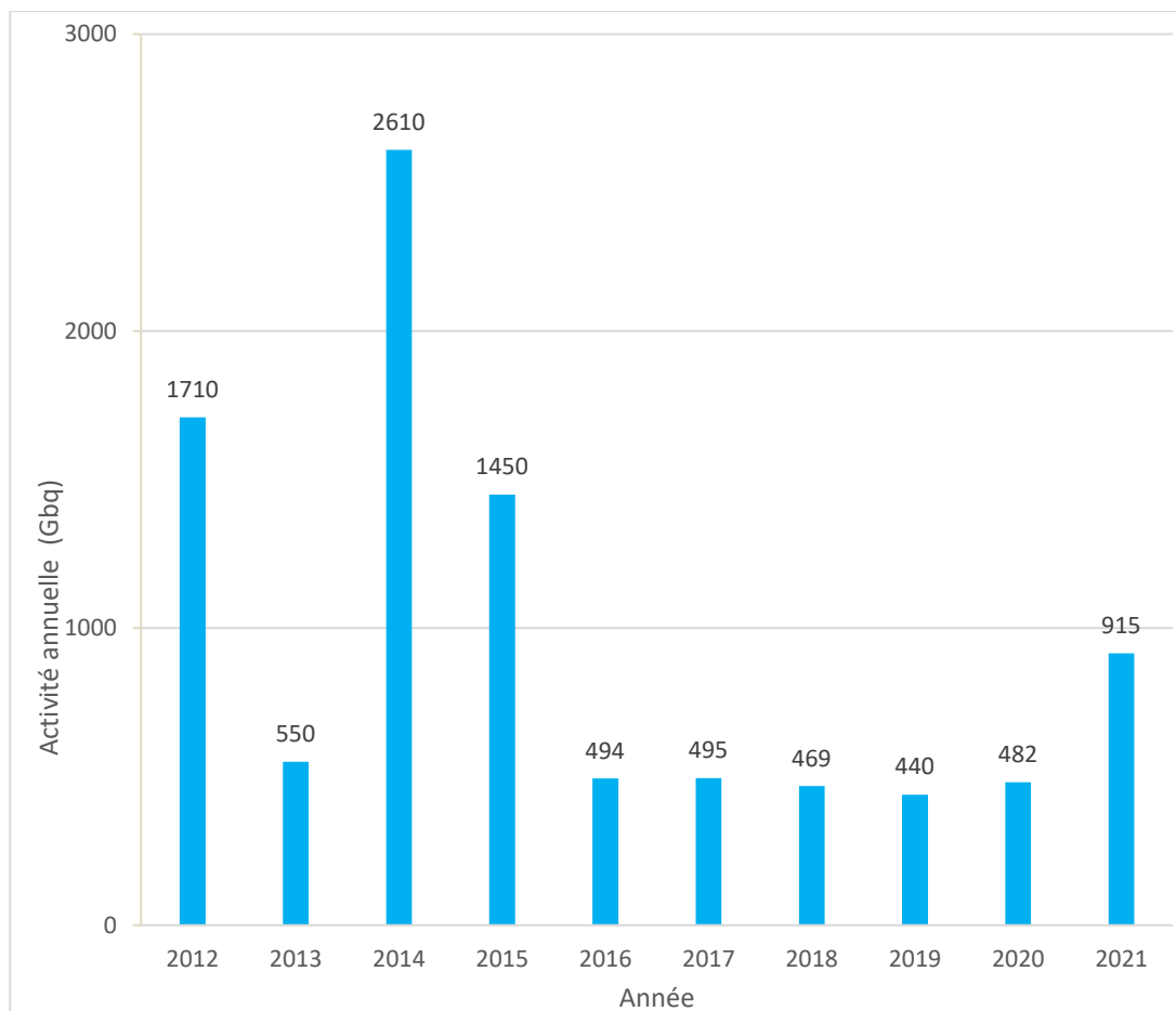
Figure 4 : Activité en gaz rares rejetée à l'atmosphère du CNPE du Blayais sur la période 2012 – 2021 (GBq/an)
