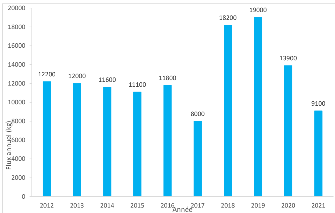
Figure 9 : Rejets annuels d'acide borique sur la période 2012-2021 du CNPE du Blayais
