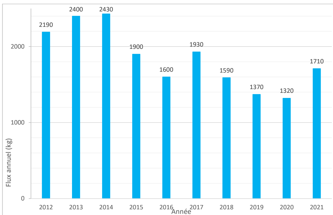
Figure 13 : Rejets annuels d'azote total sur la période 2012– 2021 du CNPE du Blayais
