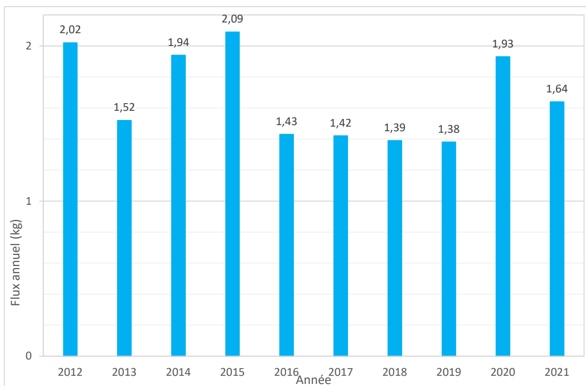
Figure 10 : Rejets annuels d'hydrazine sur la période 2012-2021 du CNPE du Blayais
