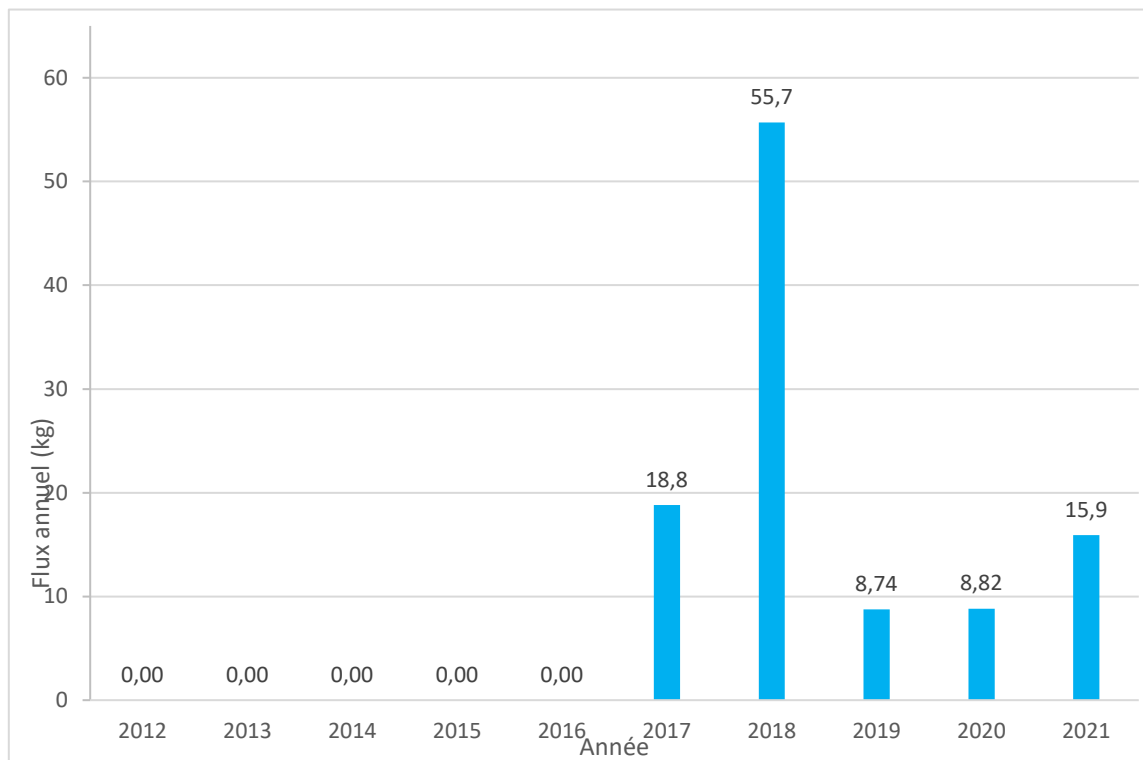
Figure 12 : Rejets annuels d'éthanolamine du CNPE du Blayais sur la période 2012- 2021
