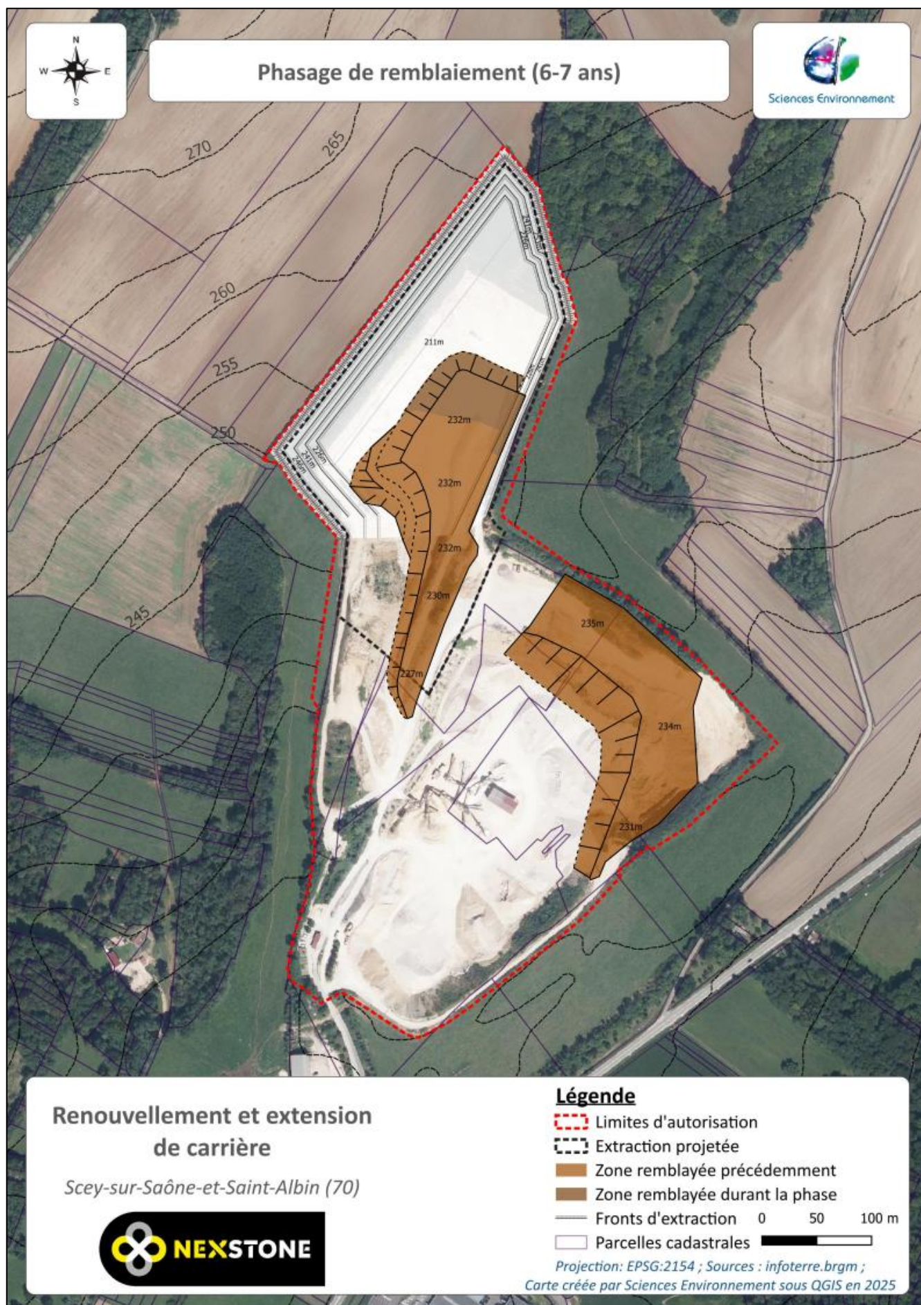
Figure 13 : Plan du phasage de remblaiement – phase 2
