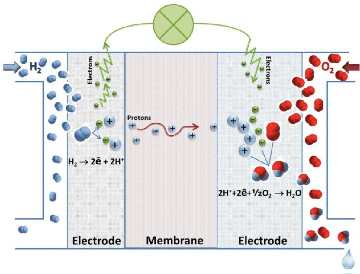
Figure 4 : Fonctionnement d'une pile à combustible à hydrogène (source : H2 mobilité)
