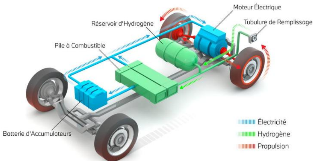
Figure 5 : Fonctionnement d'un véhicule à hydrogène (source : H2 mobilité)
