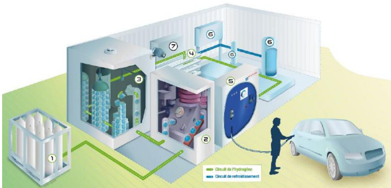
Figure 7 : Fonctionnement d'une station-service à hydrogène
