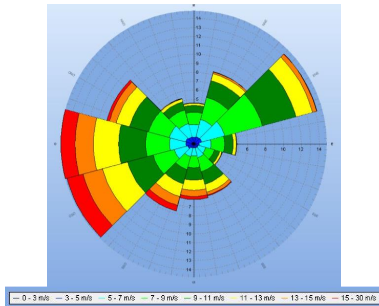
Figure 2 : Rose des énergies à 102 mètres de haut pour une extrapolation long terme sur 15 années (source : Eolise)
