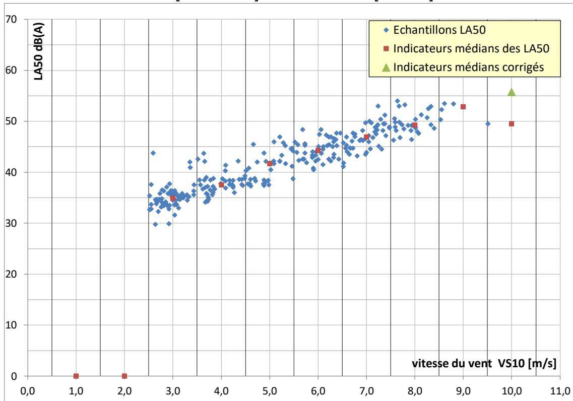
Figure 10 : analyse des bruits résiduels - Les Minimes_M - Secteur secondaire NE [315° - 135°] - Période diurne [7h -22h]
