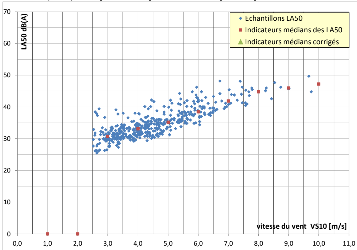
Figure 18 : analyse des bruits résiduels - Quinsac_M - Secteur principal SO [135° - 315°] - Période diurne [7h -22h]
