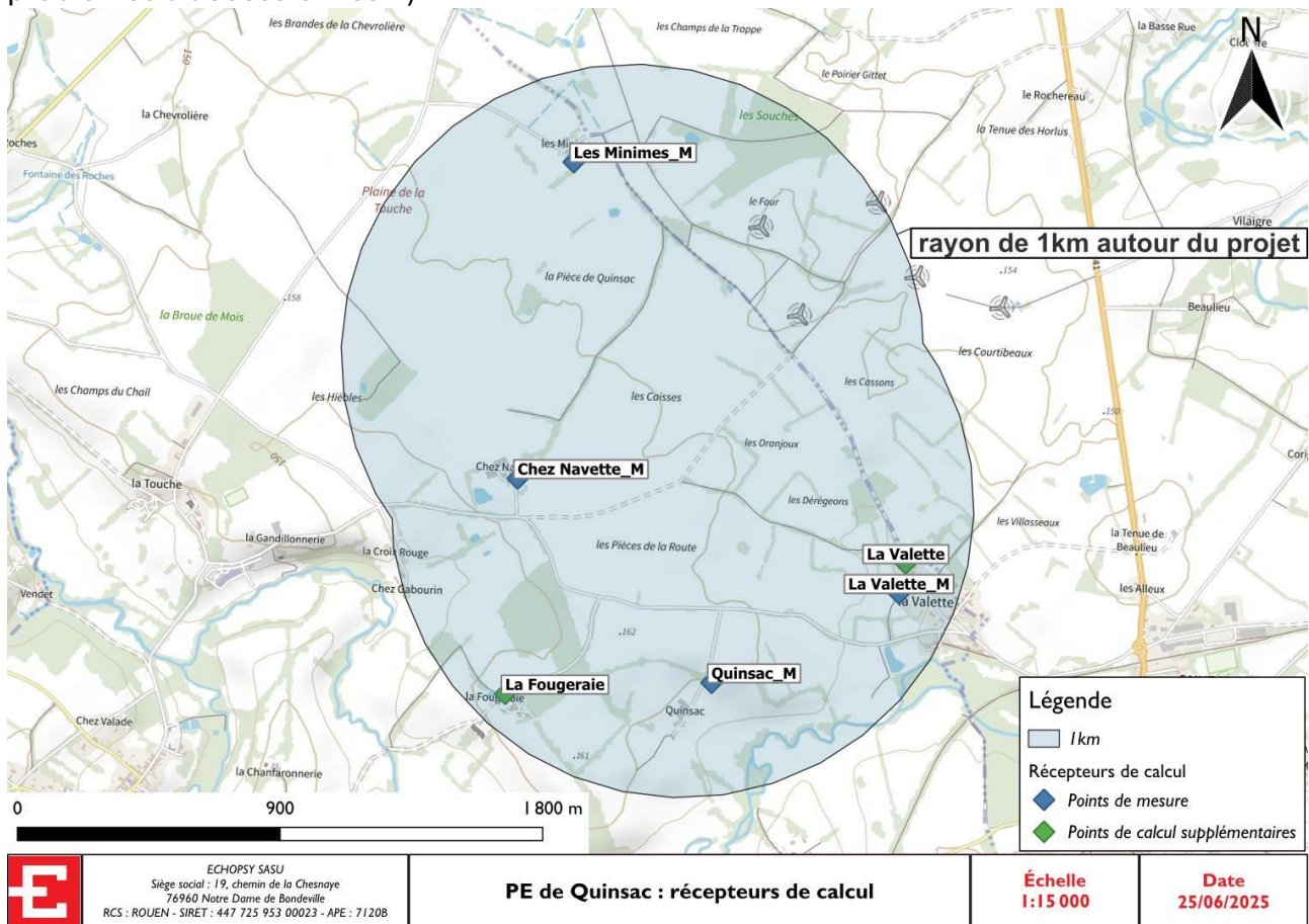
Carte 6 : récepteurs de calculs au complet
