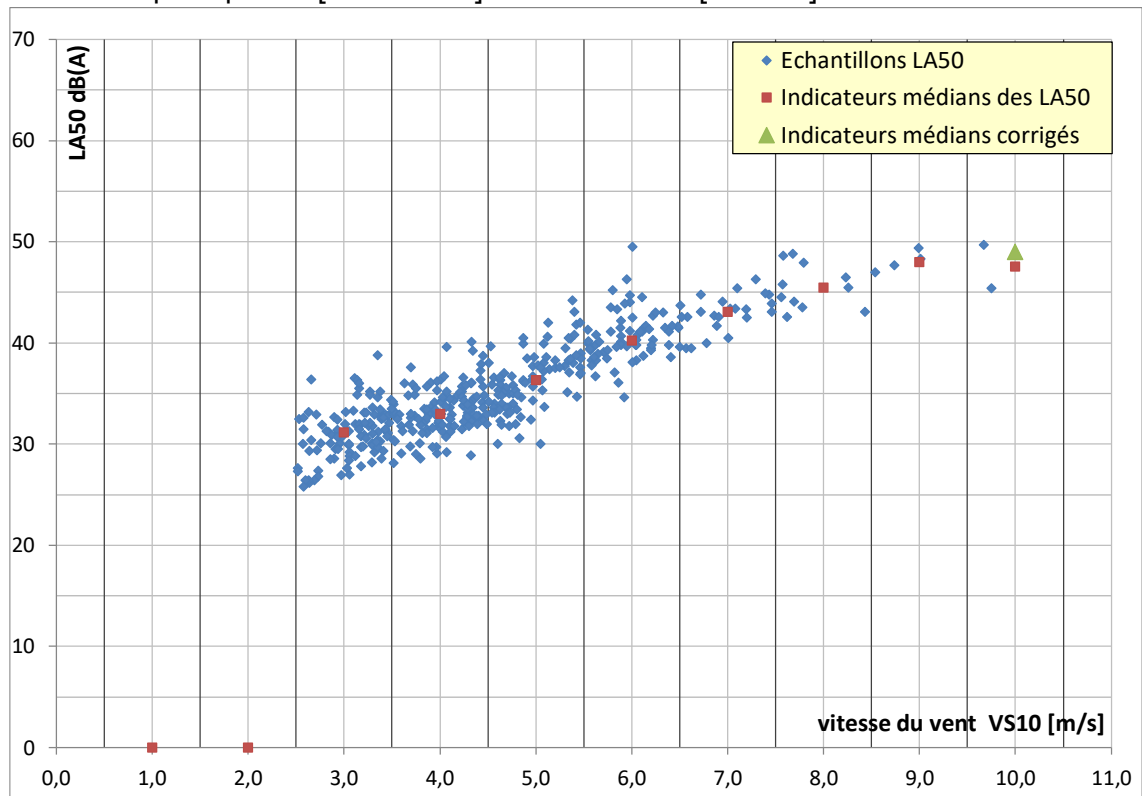
Figure 23 : analyse des bruits résiduels - La Valette_M - Secteur principal SO [135° - 315°] - Période diurne [7h -22h]
