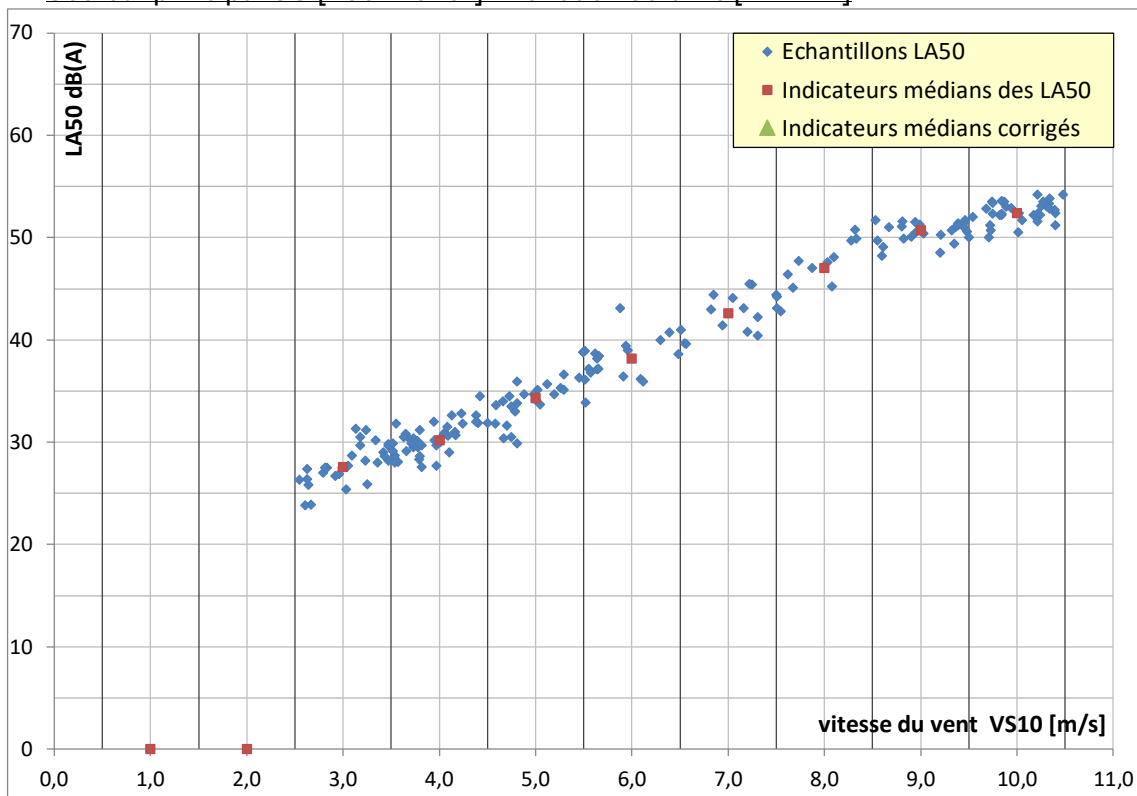
Figure 14 : analyse des bruits résiduels - Chez Navette_M - Secteur principal SO [135° - 315°] - Période nocturne [22h -7h]
