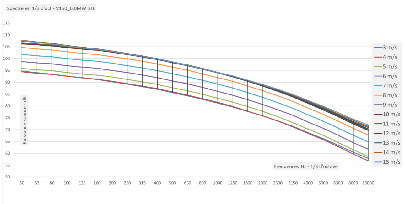
Figure 29 : données acoustique sous forme spectrale – V150_6,0MW
