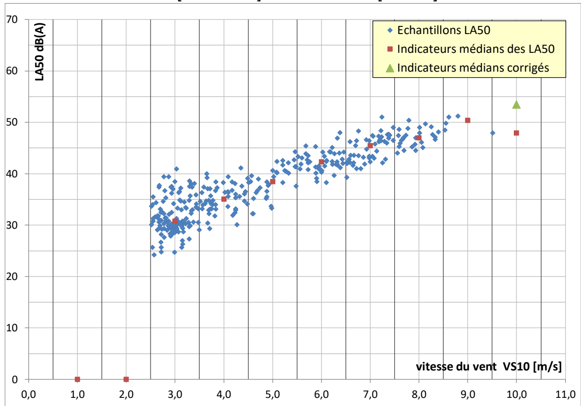
Figure 20 : analyse des bruits résiduels - Quinsac_M - Secteur secondaire NE [315° - 135°] - Période diurne [7h -22h]
