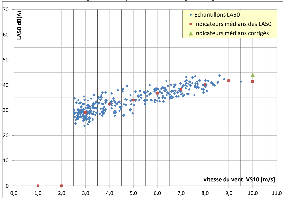
Figure 25 : analyse des bruits résiduels - La Valette_M - Secteur secondaire NE [315° - 135°] - Période diurne [7h -22h]
