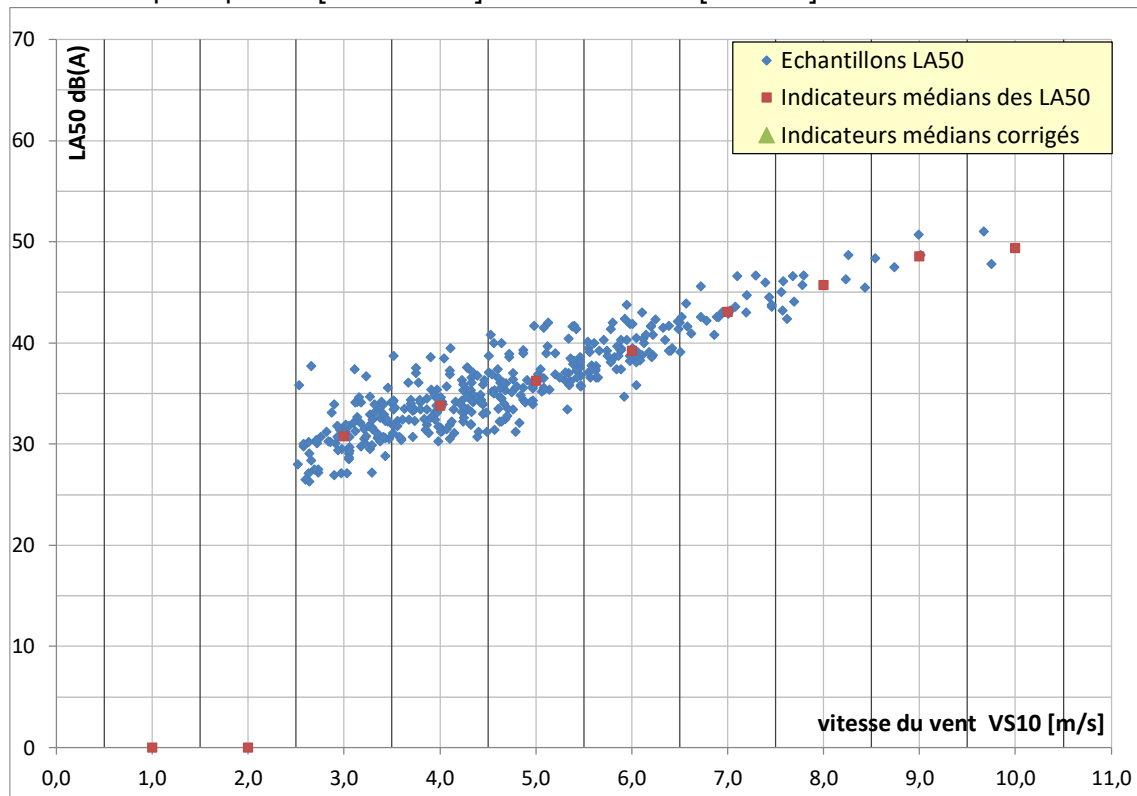
Figure 13 : analyse des bruits résiduels - Chez Navette_M - Secteur principal SO [135° - 315°] - Période diurne [7h -22h]
