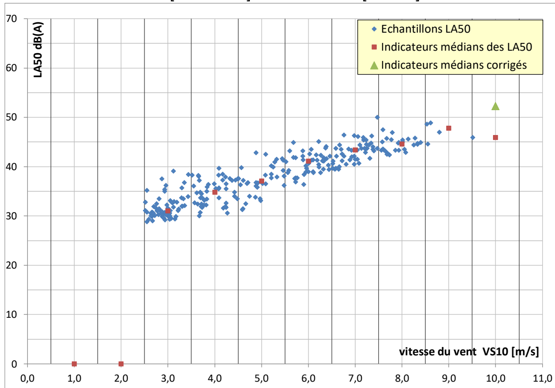
Figure 15 : analyse des bruits résiduels - Chez Navette_M - Secteur secondaire NE [315° - 135°] - Période diurne [7h -22h]
