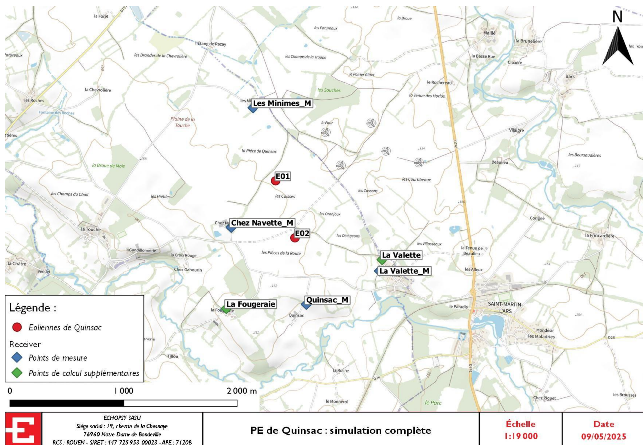
Carte 9 : carte complète de la simulation du projet
