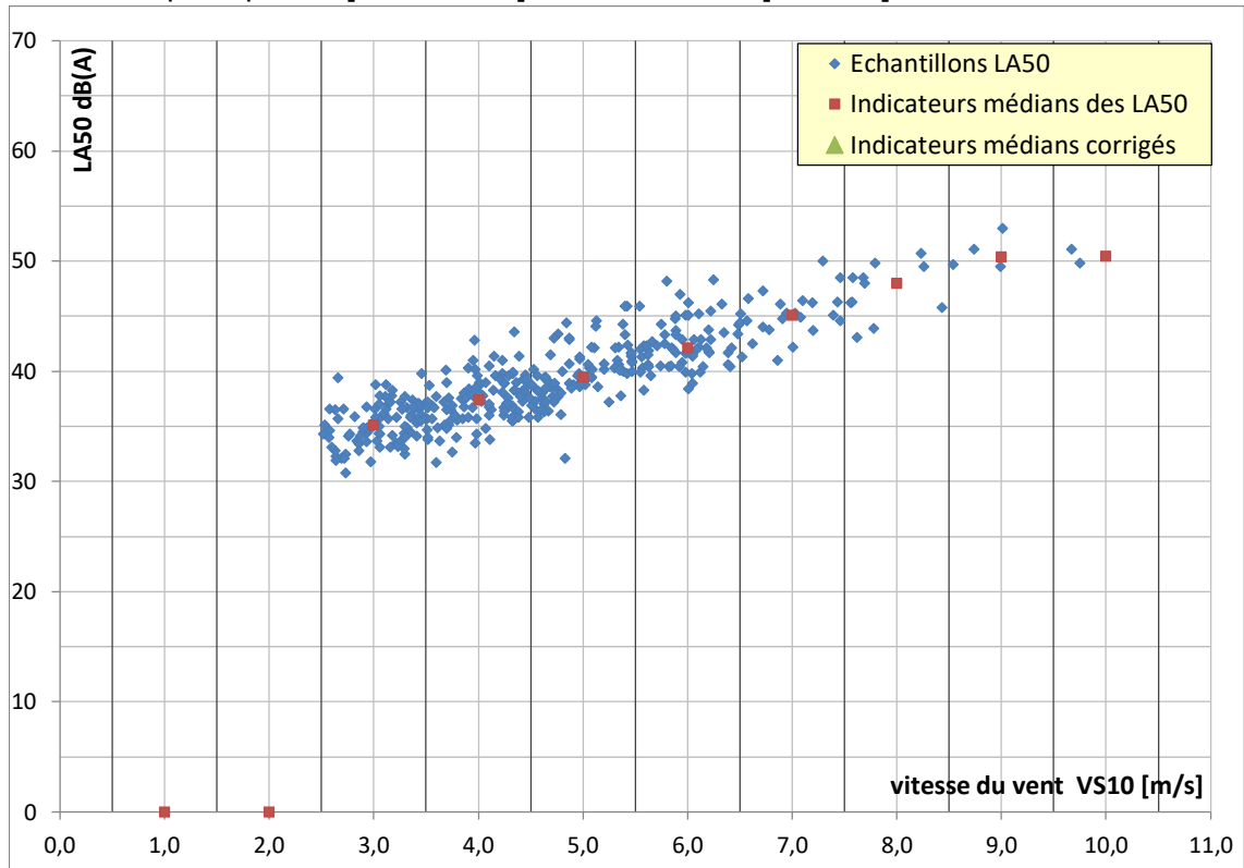
Figure 8 : analyse des bruits résiduels - Les Minimes_M - Secteur principal SO [135° - 315°] - Période diurne [7h -22h]
