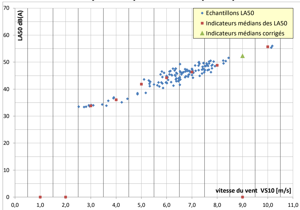
Figure 11 : analyse des bruits résiduels - Les Minimes_M - Secteur secondaire NE [315° - 135°] - Période nocturne [22h - 7h]
