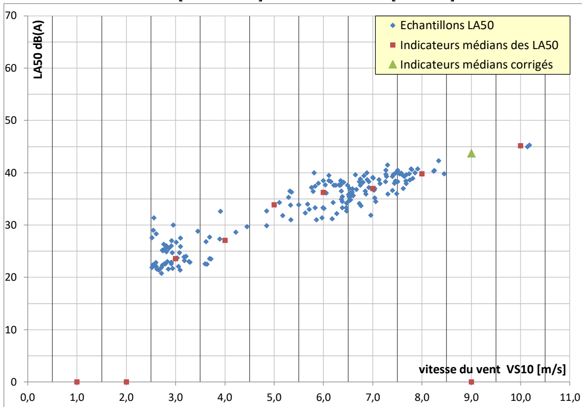
Figure 26 : analyse des bruits résiduels - La Valette_M - Secteur secondaire NE [315° - 135°] - Période nocturne [22h - 7h]
