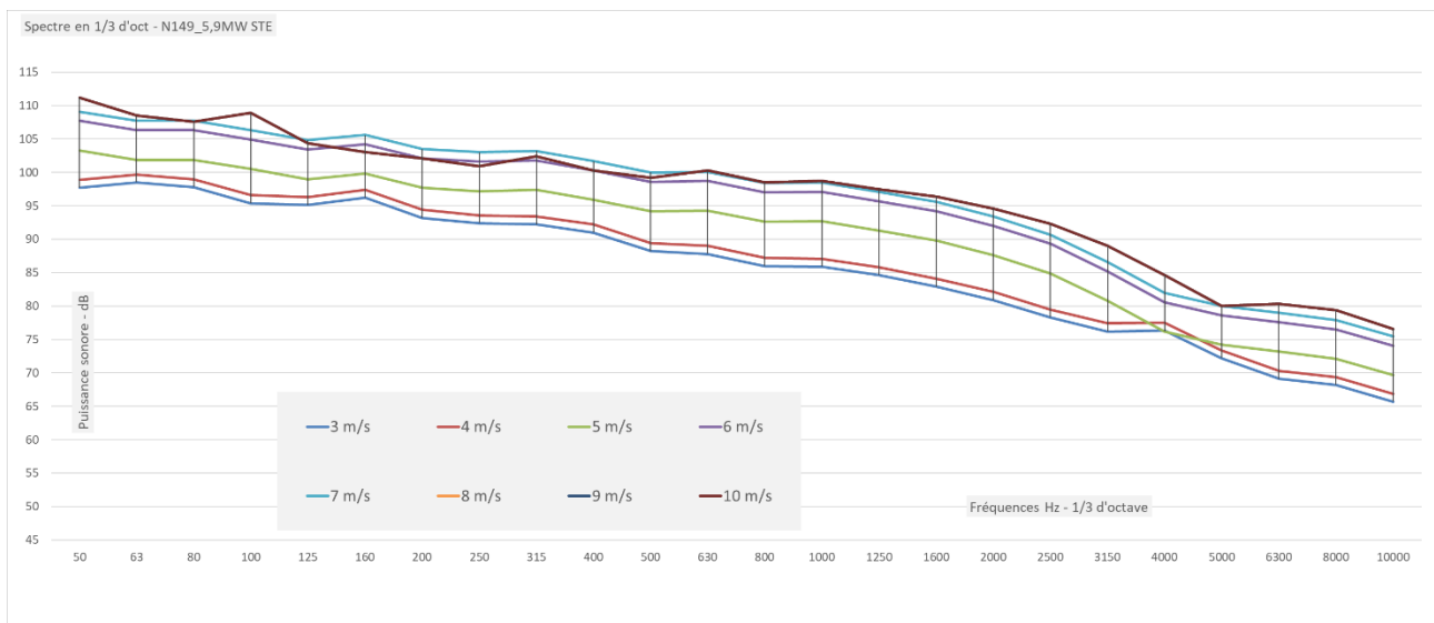
Figure 28 : données acoustique sous forme spectrale – N149_5,9MW
