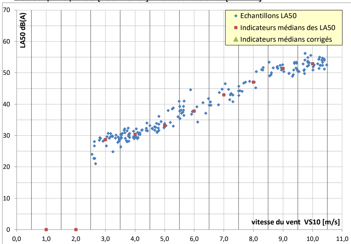
Figure 24 : analyse des bruits résiduels - La Valette_M - Secteur principal SO [135° - 315°] - Période nocturne [22h -7h]
