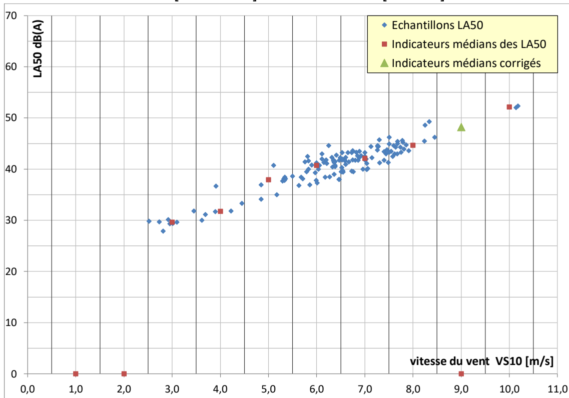
Figure 16 : analyse des bruits résiduels - Chez Navette_M - Secteur secondaire NE [315° - 135°] - Période nocturne [22h - 7h]
