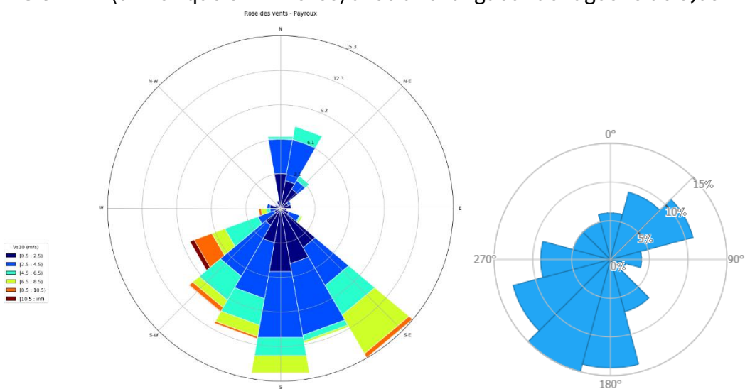
Figure 6 : rose des vents campagne de mesure (à gauche) - rappel de la rose des vents annuelle (à droite)
