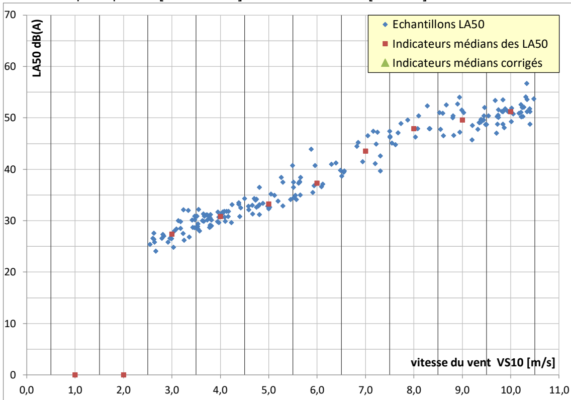
Figure 19 : analyse des bruits résiduels - Quinsac_M - Secteur principal SO [135° - 315°] - Période nocturne [22h -7h]
