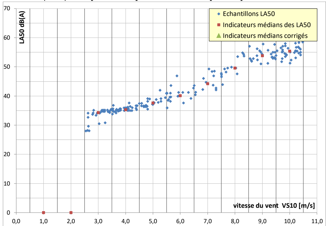
Figure 9 : analyse des bruits résiduels - Les Minimes_M - Secteur principal SO [135° - 315°] - Période nocturne [22h -7h]
