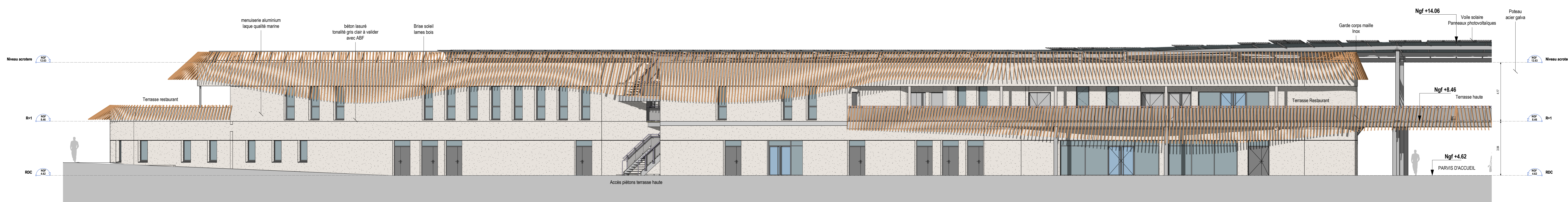
Façade Nord boomerang Zone B 1 : 100
