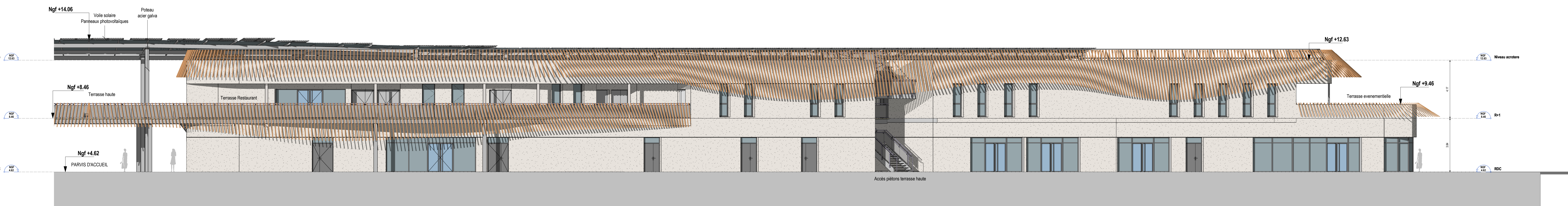
Façade Nord boomerang Zone A 1 : 100
