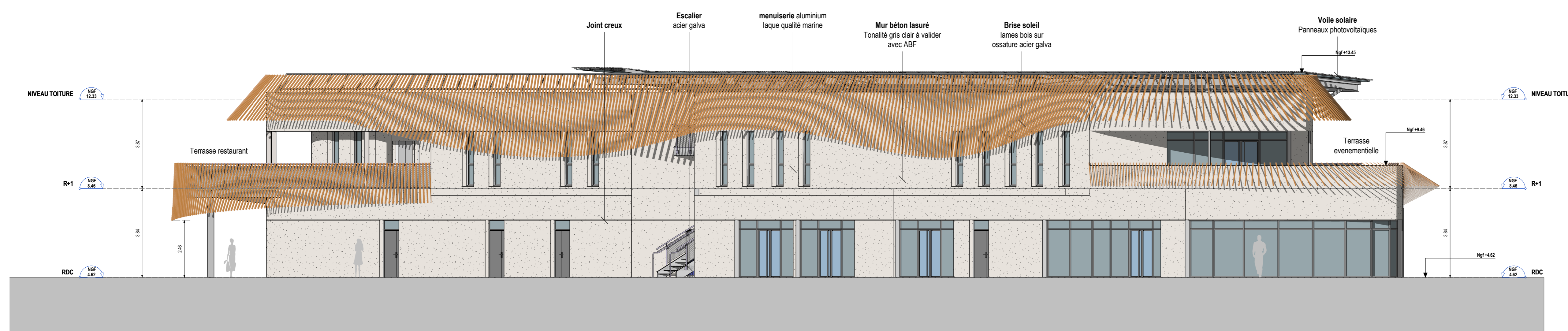
Façade Ouest boomerang 1 : 100
