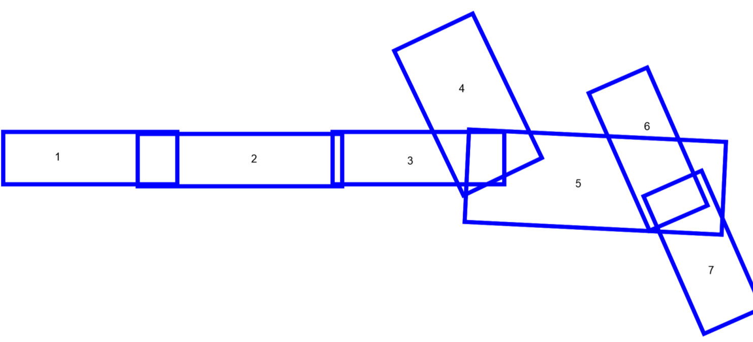
Réseau : Réseau de Collecte de Eschau Axe : Profil P4 - P10 Echelle X : 1/384 Echelle Z : 1/384 Plan Comp : 140.2
