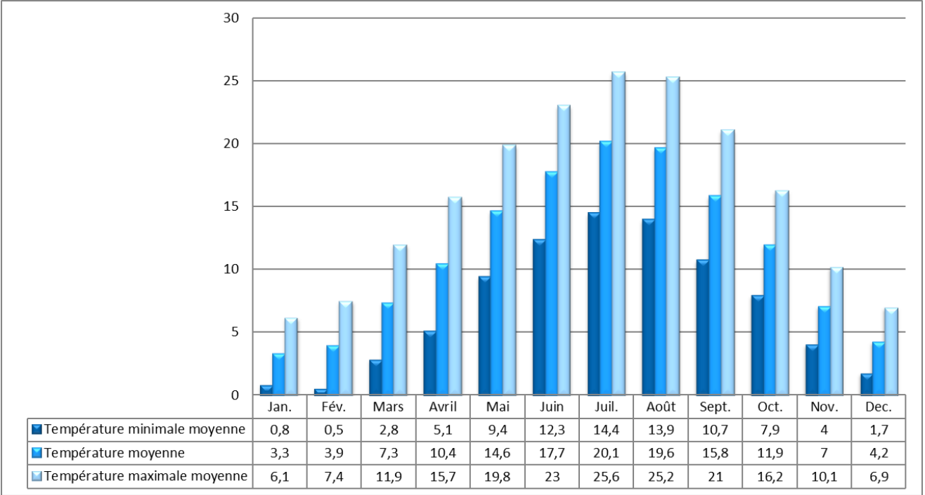
Figure 1 : Illustration des températures de 1981 à 2018 – Station de Saint-Dizier (source : Infoclimat.fr, 2020)
