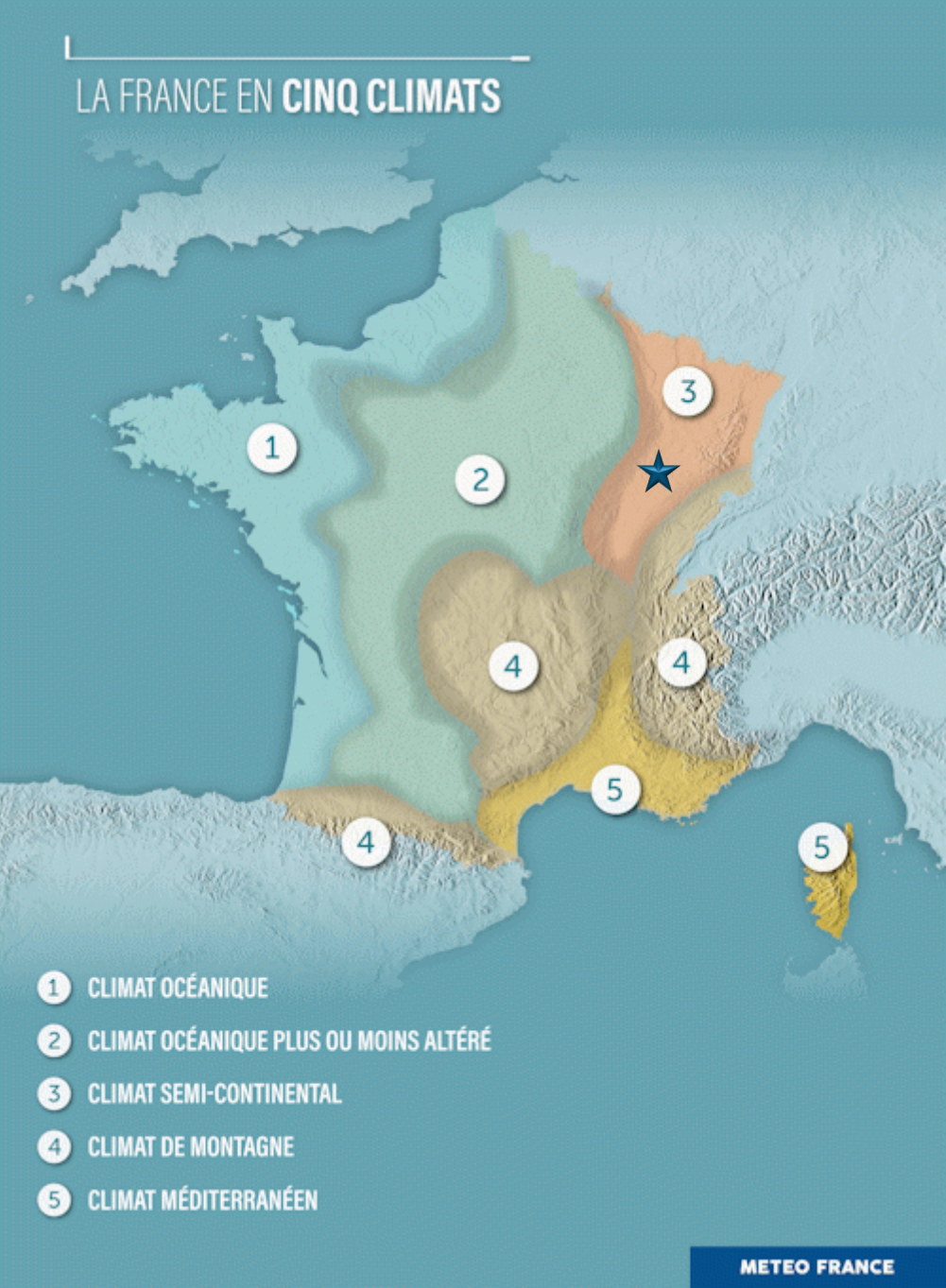
Carte 4 : Climats de France métropolitaine – Etoile bleue : Zone d’implantation potentielle (source : Météo France, 2023)
