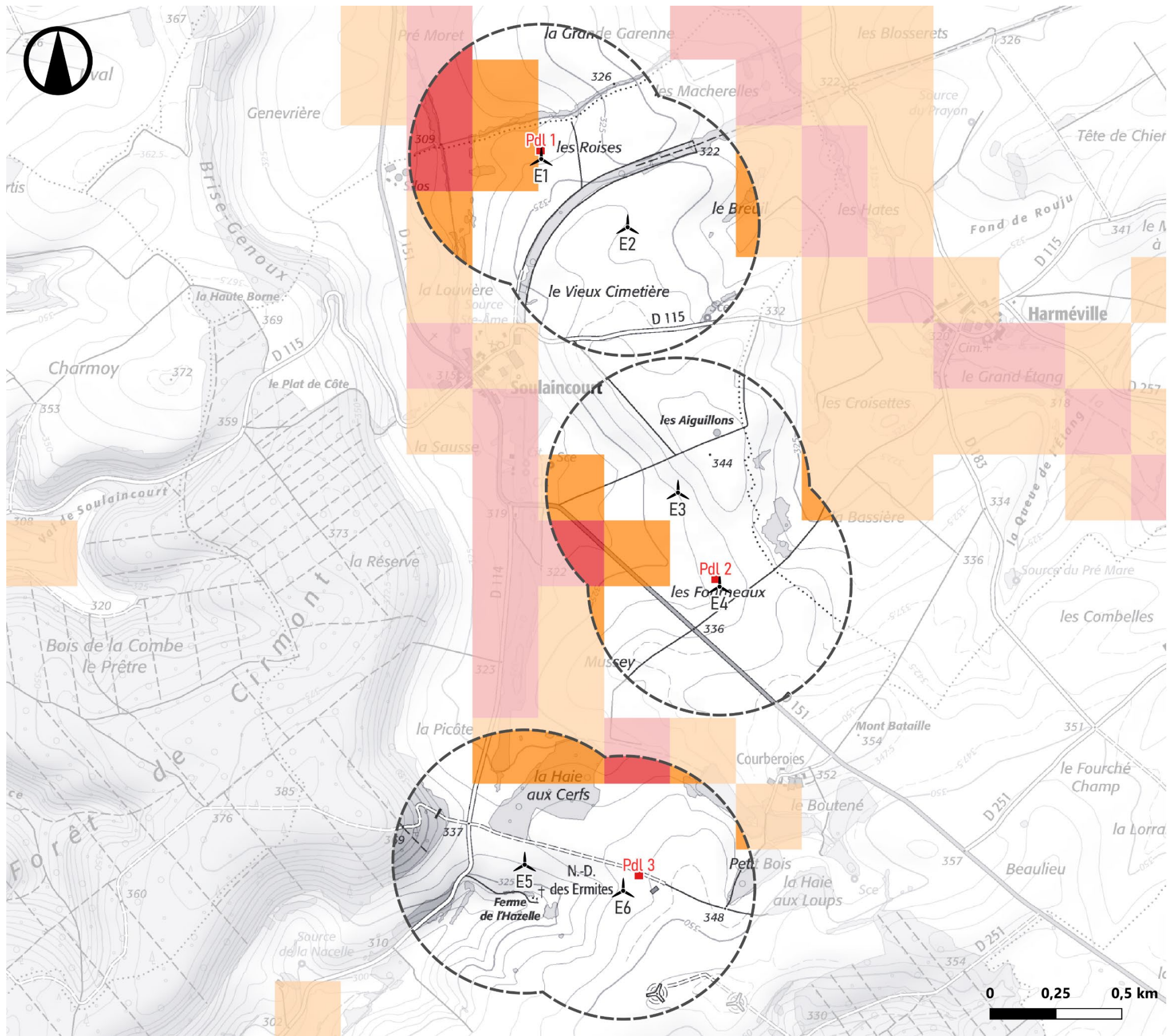
Carte 6 : Risques naturels majeurs au niveau du périmètre d'étude de dangers : sensibilité au phénomène de remontée de nappe
