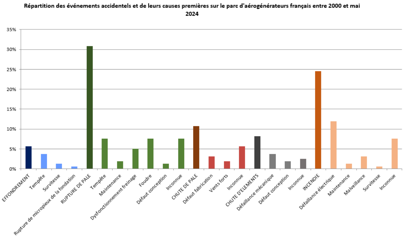
Figure 9 : Répartition des événements accidentels et de leurs causes premières sur le parc éolien français entre 2000 et 2024 (source : SER/FEE/INERIS, 2024)
