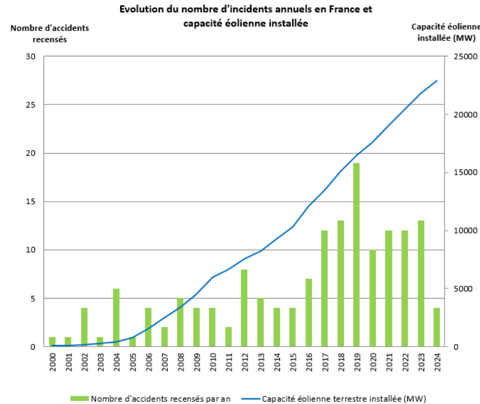
Figure 12 : Évolution du nombre d'incidents annuels en France et nombre d'éoliennes installées (INERIS/SER/FEE, 2024)
