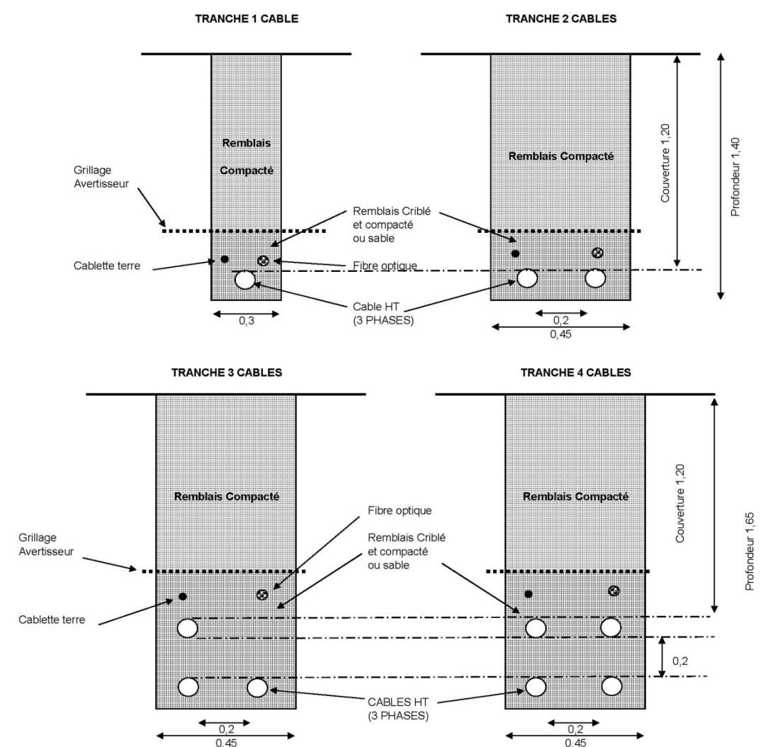
Figure 8 : Vue en coupe des tranchées selon le nombre de câbles passés
