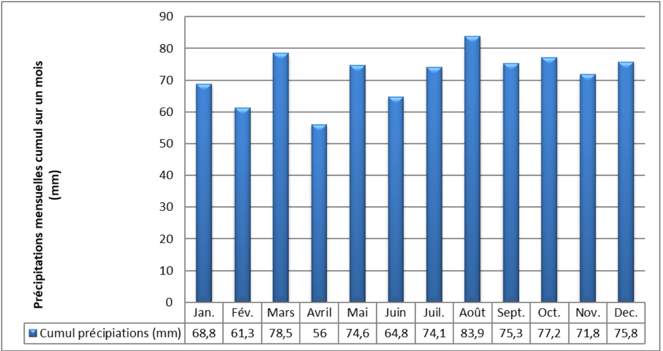
Figure 2 : Illustration des précipitations de 1981 à 2018 – Station de Saint-Dizier (source : Infoclimat, 2020)
