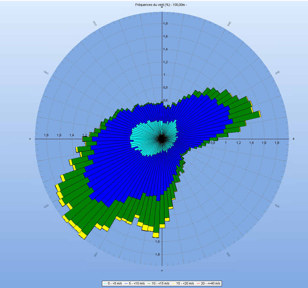
Figure 4 : Rose des vents mesurée au niveau de disponible au niveau du point de données réanalysées ERA5 le plus proche (QEnergy, 2025)
