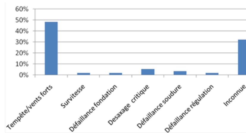
Figure 10 : Répartition des événements accidentels dans le monde entre 2000 et 2024 (source : SER/FEE/INERIS, 2024)
