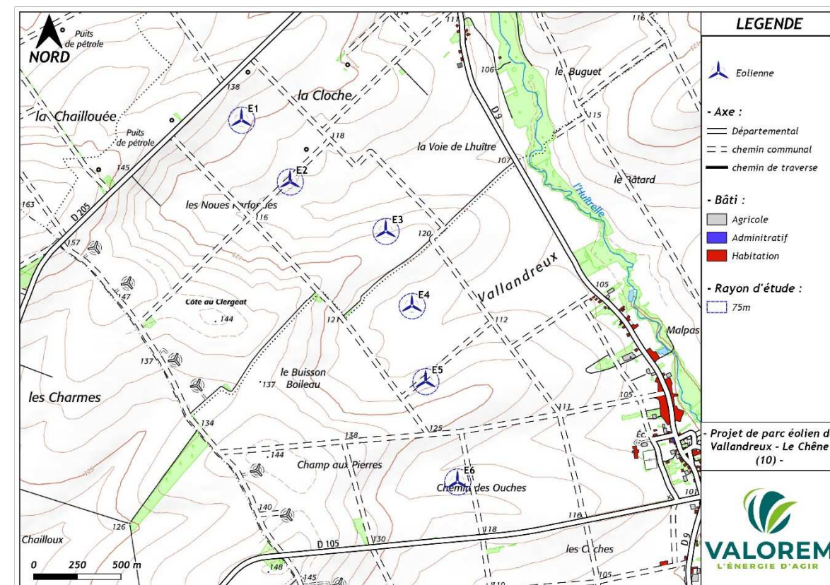
Zones d'effet des phénomènes « Chute de glace »
