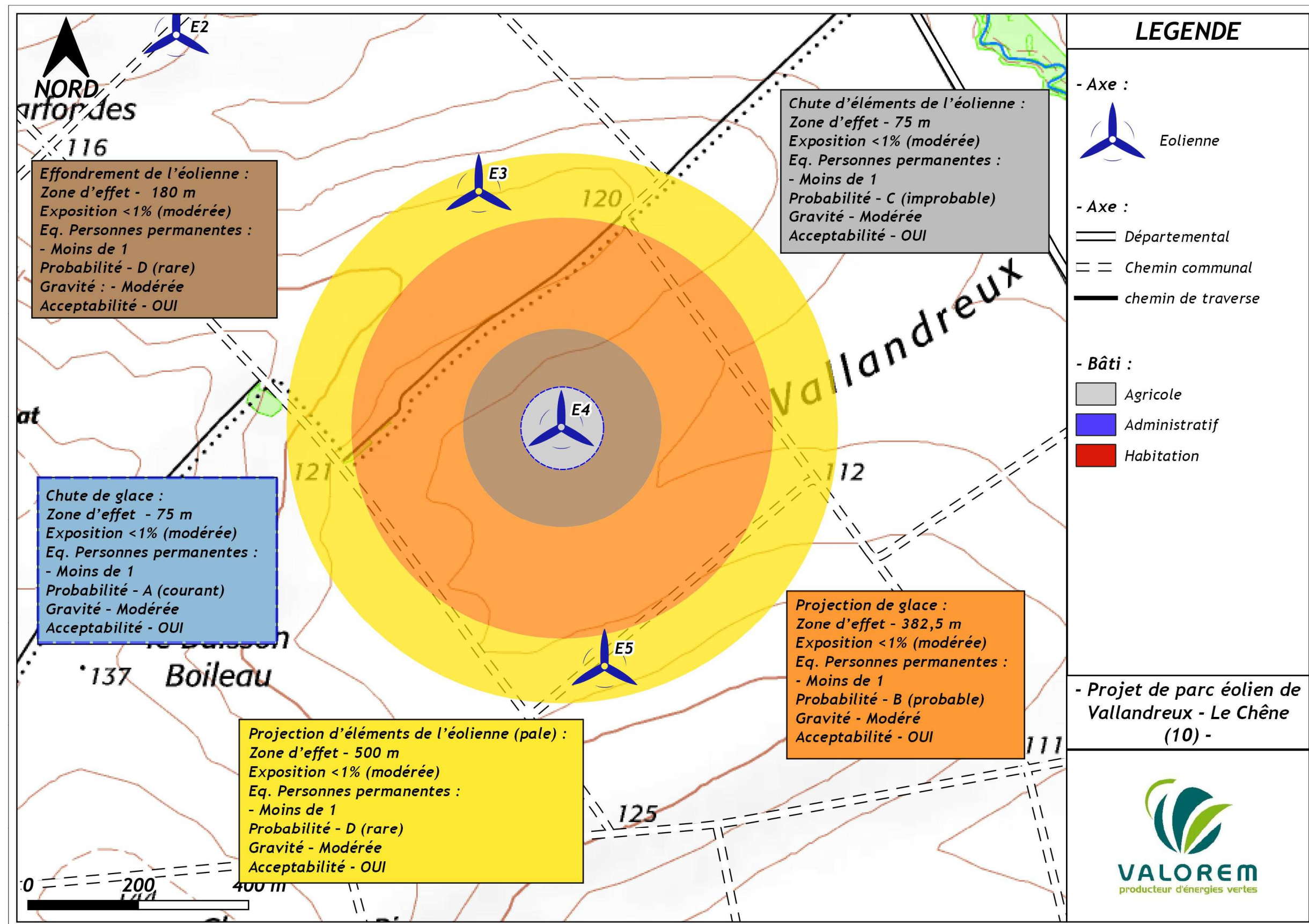
Synthèse des zones d'effet - éolienne E4
