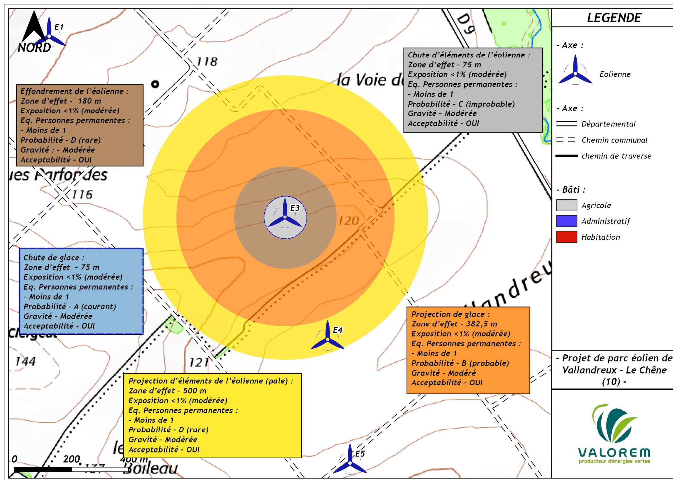
Synthèse des zones d'effet - éolienne E3
