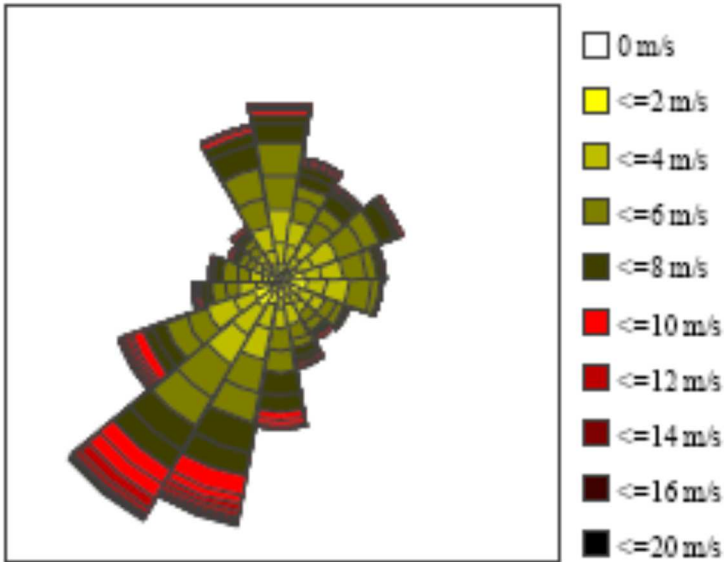
Rose des vents du site.
