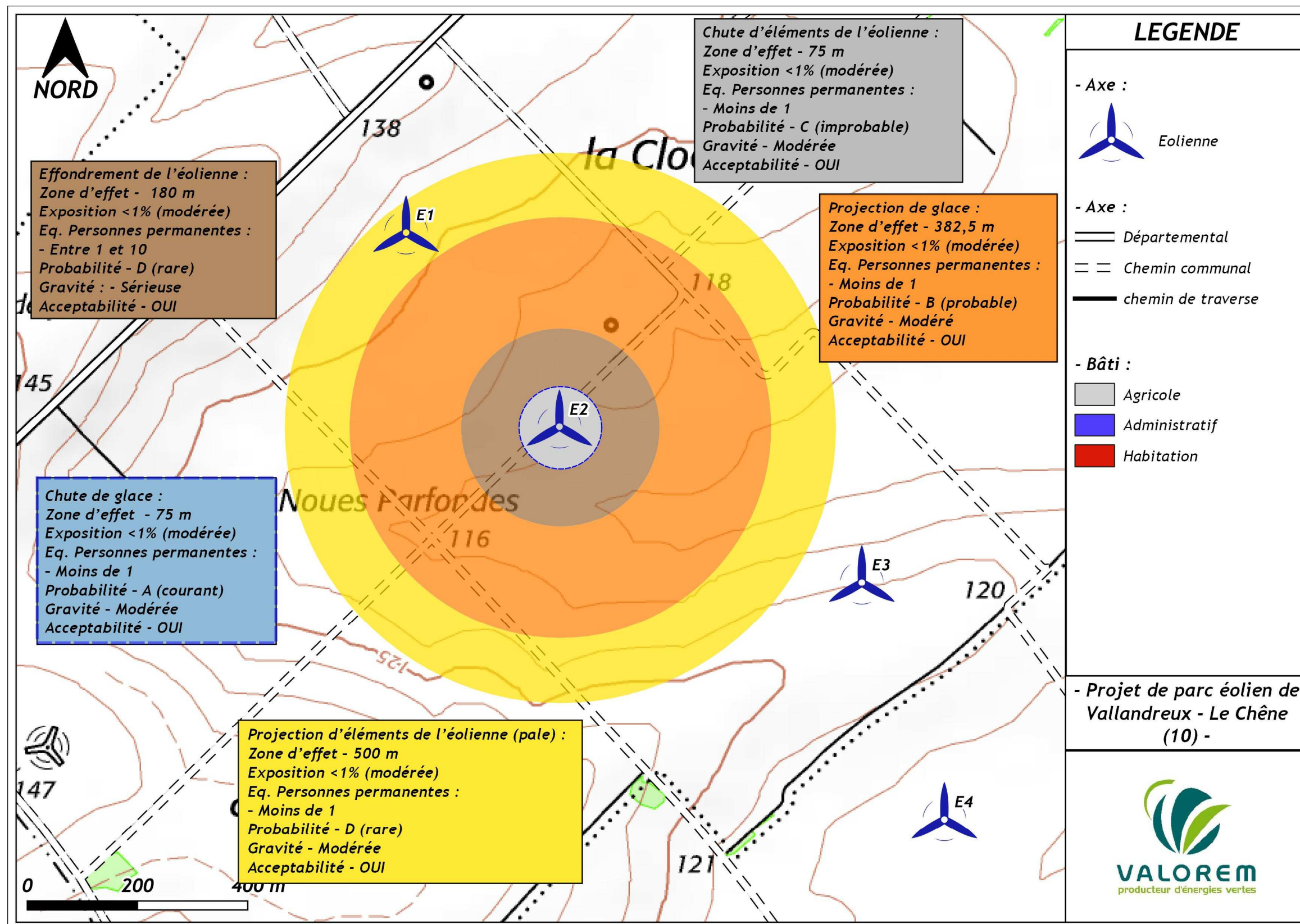
Synthèse des zones d'effet - éolienne E2
