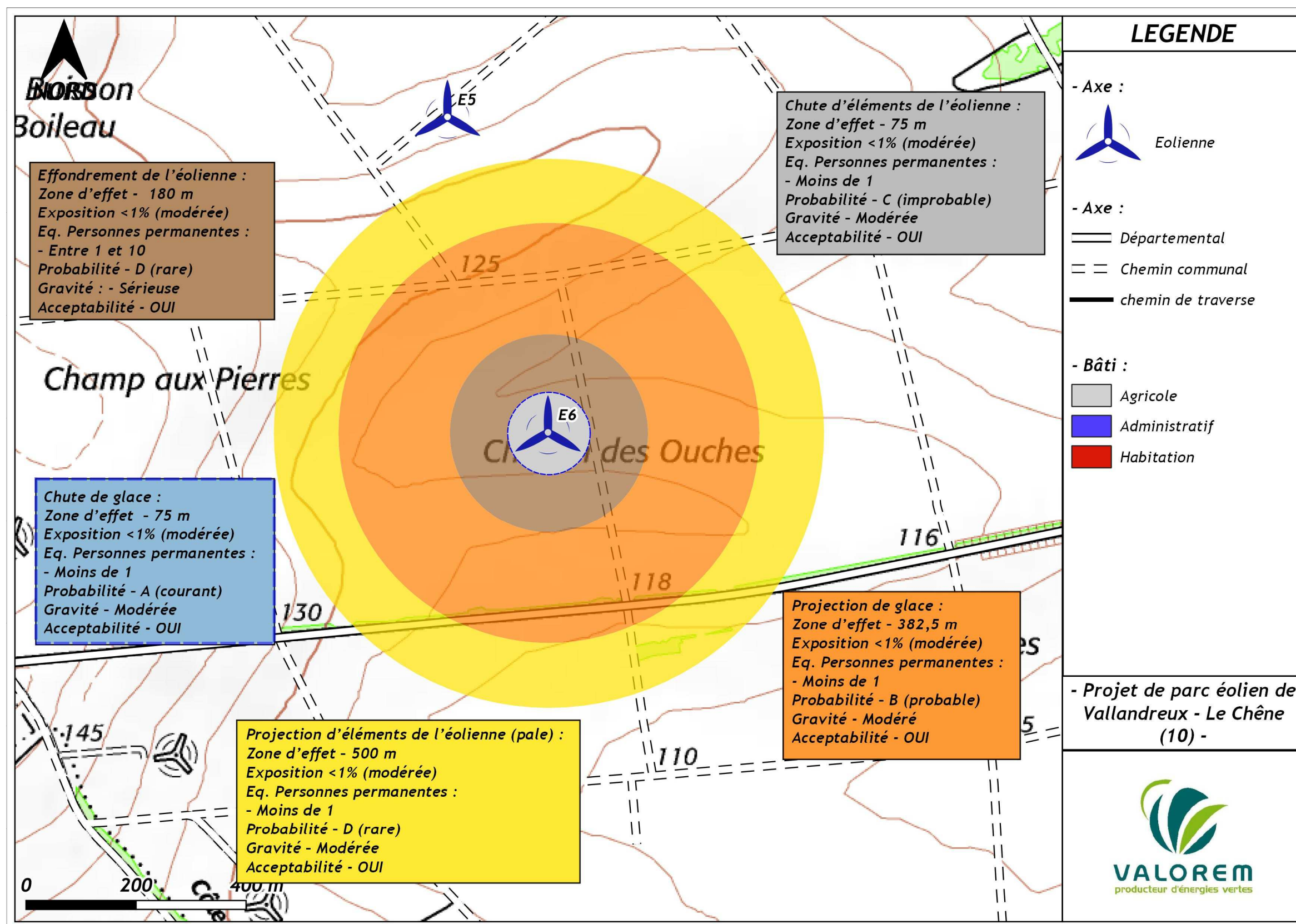
Synthèse des zones d'effet - éolienne E6
