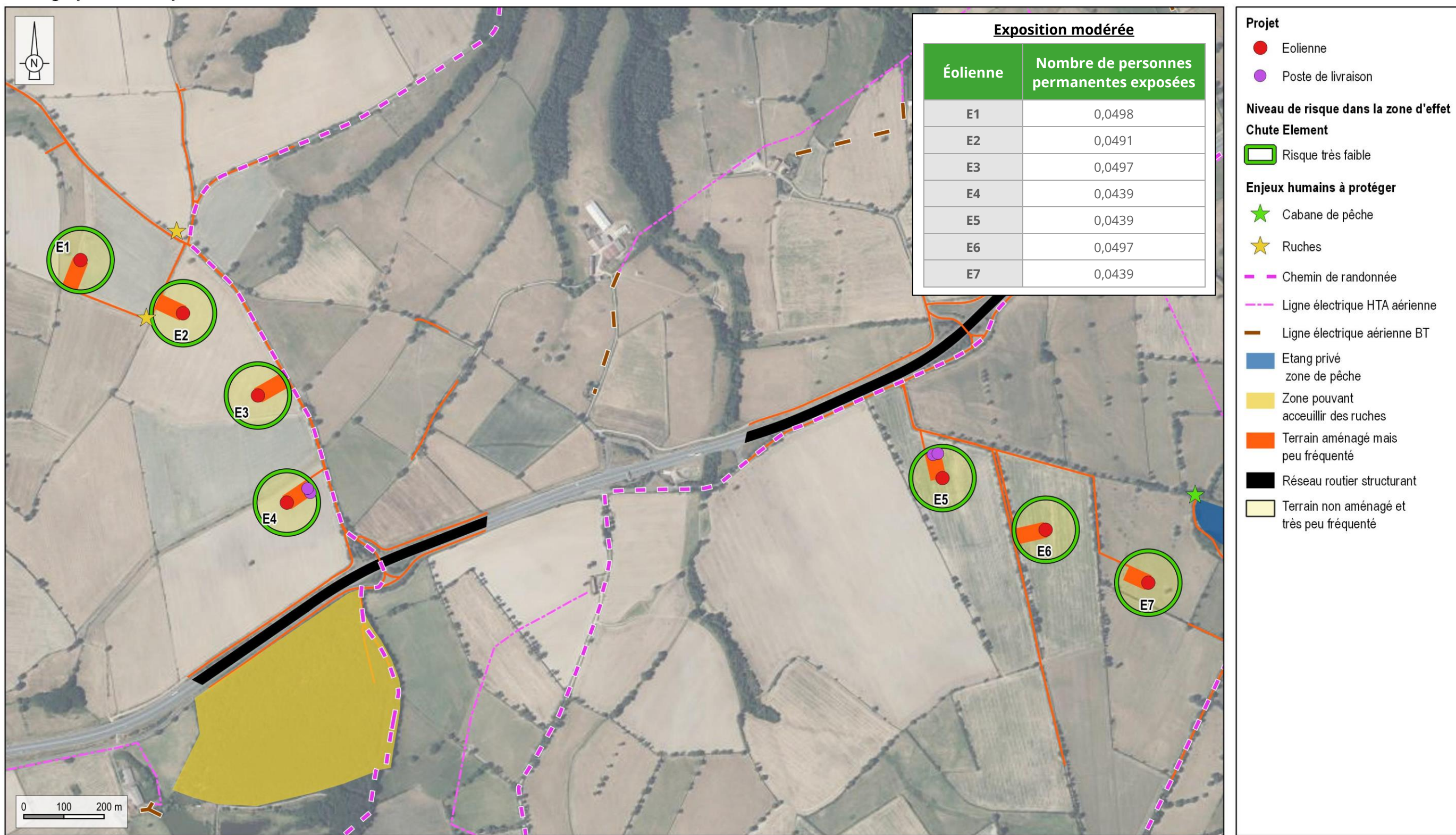
Carte 21 : Cartographie des risques – Scénario de chute d'éléments de l'éolienne
