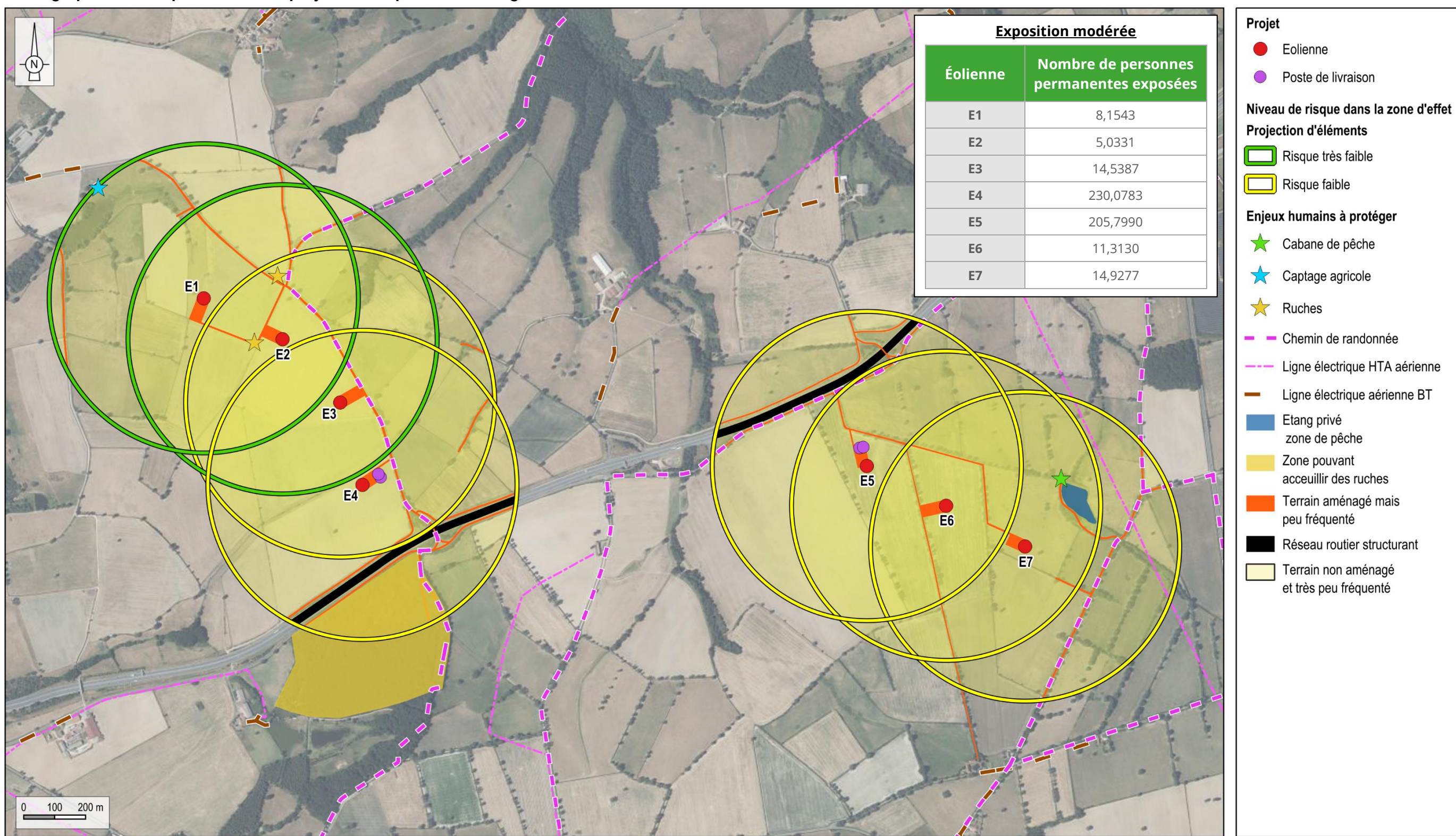
Carte 22 : Cartographie des risques – Scénario de projection de pales ou de fragments de pales
