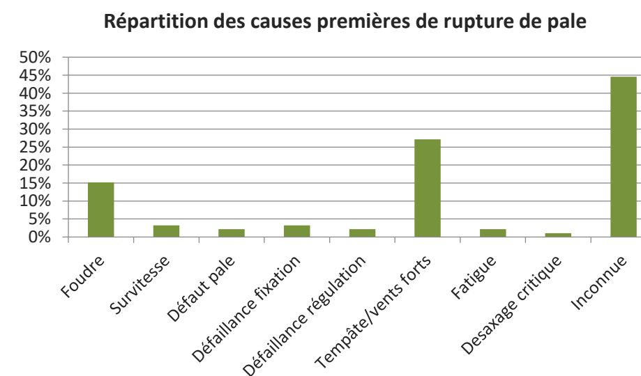
Figure 9 : Répartition des causes premières de rupture de pale dans les accidents à l'international entre 2000 et 2011
