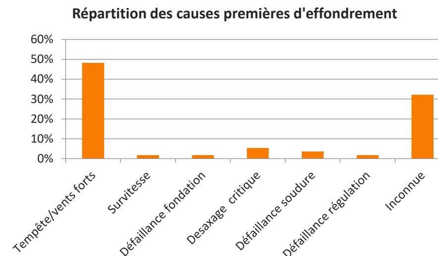
Figure 8 : Répartition des causes premières d'effondrement dans les accidents à l'international entre 2000 et 2011
