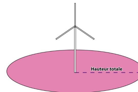
Figure 12 : Zone d'effet du phénomène d'effondrement de l'éolienne
