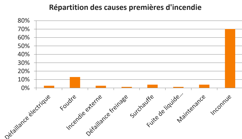
Figure 10 : Répartition des causes premières d'incendie dans les accidents à l'international entre 2000 et 2011
