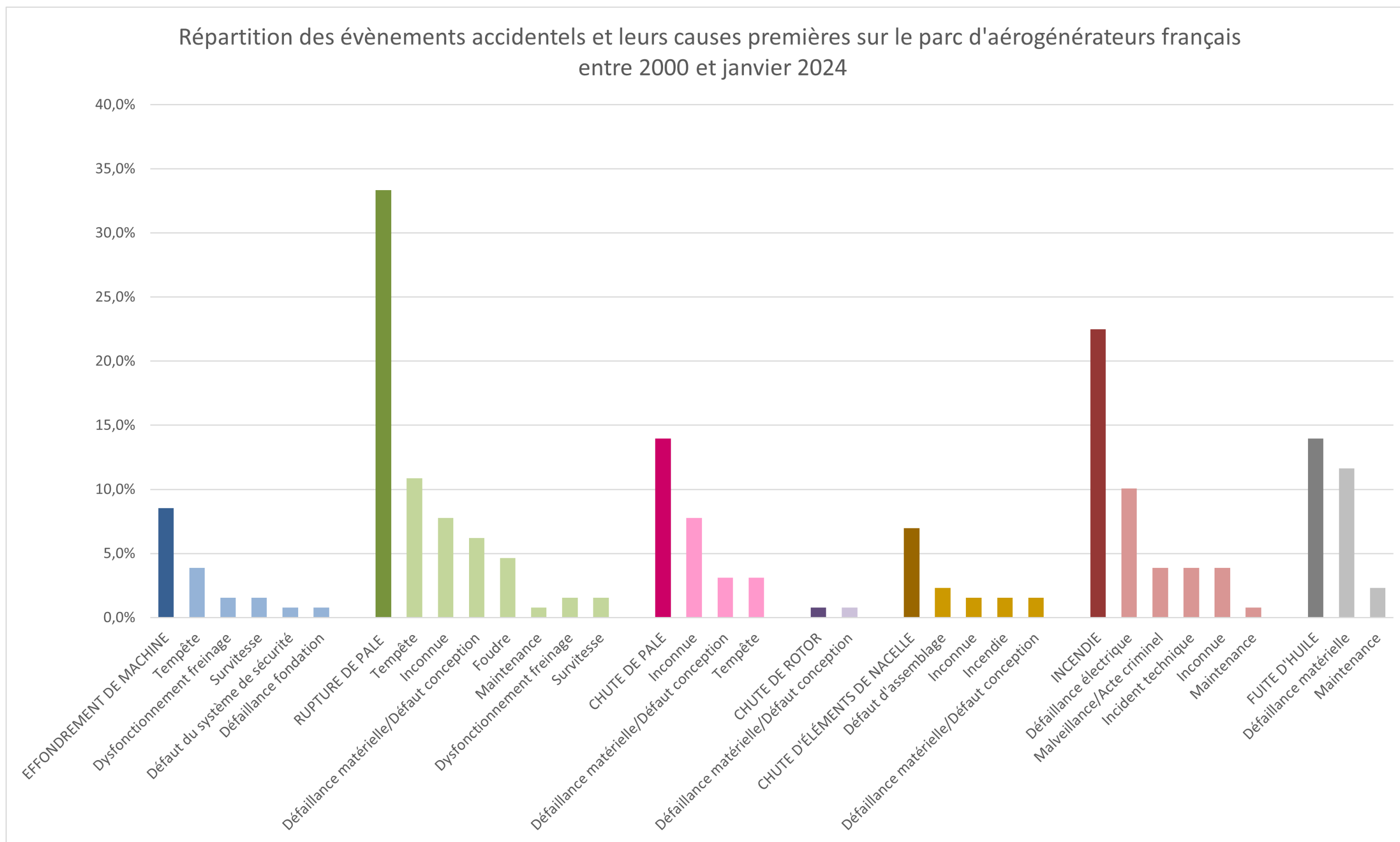
Figure 6 : Répartition des accidents et de leurs causes premières sur le parc éolien français entre 2000 et janvier 2024
