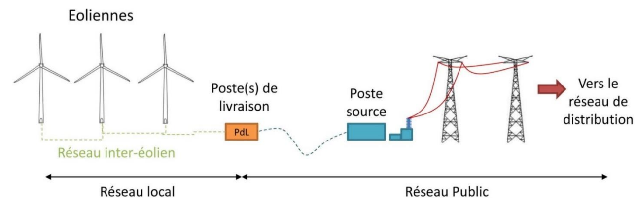
Figure 5 : Raccordement électrique des installations (source : INERIS/SER/FEE, 2012)
