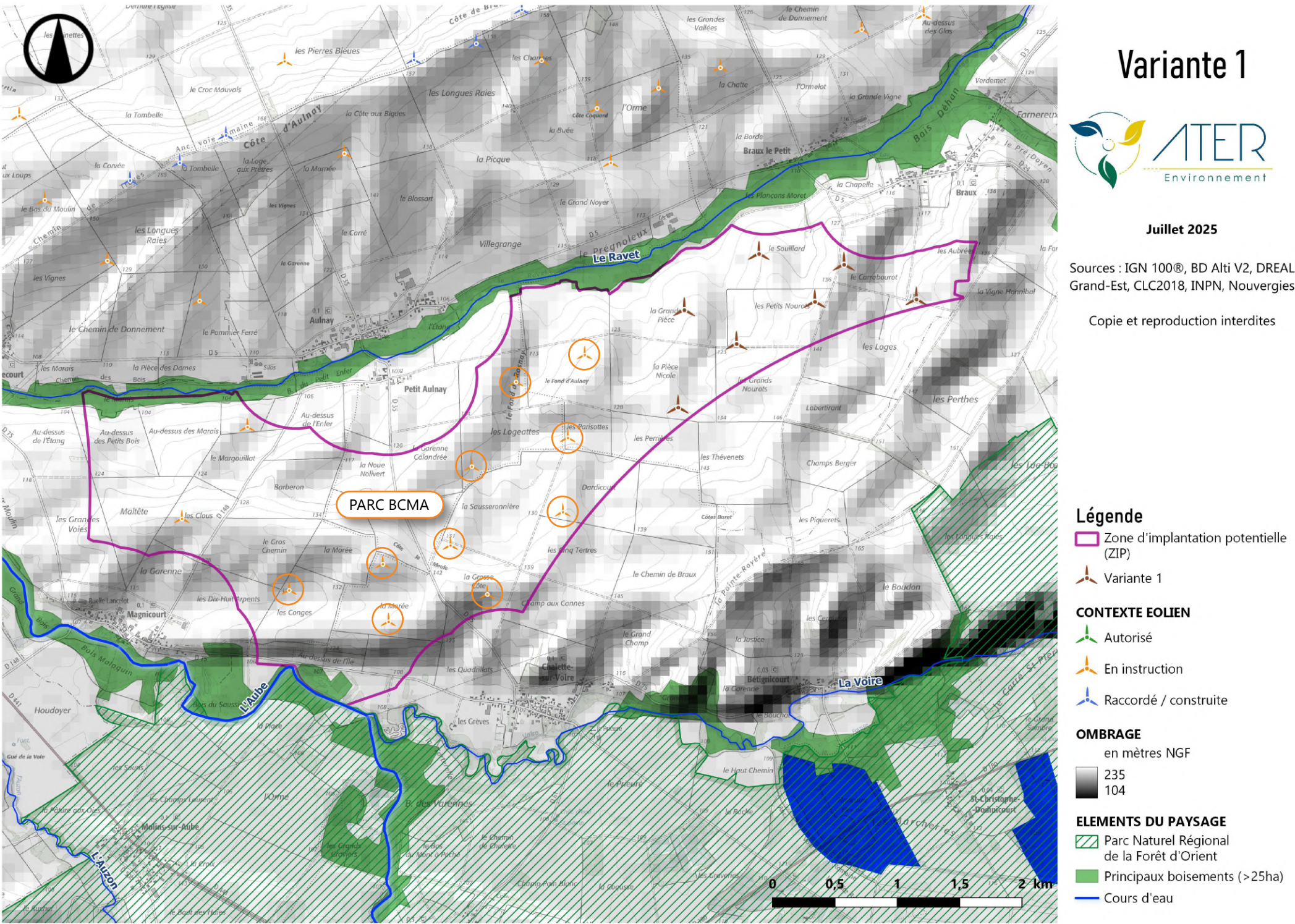
Fig. 141 : Plan d'implantation de la variante 1
