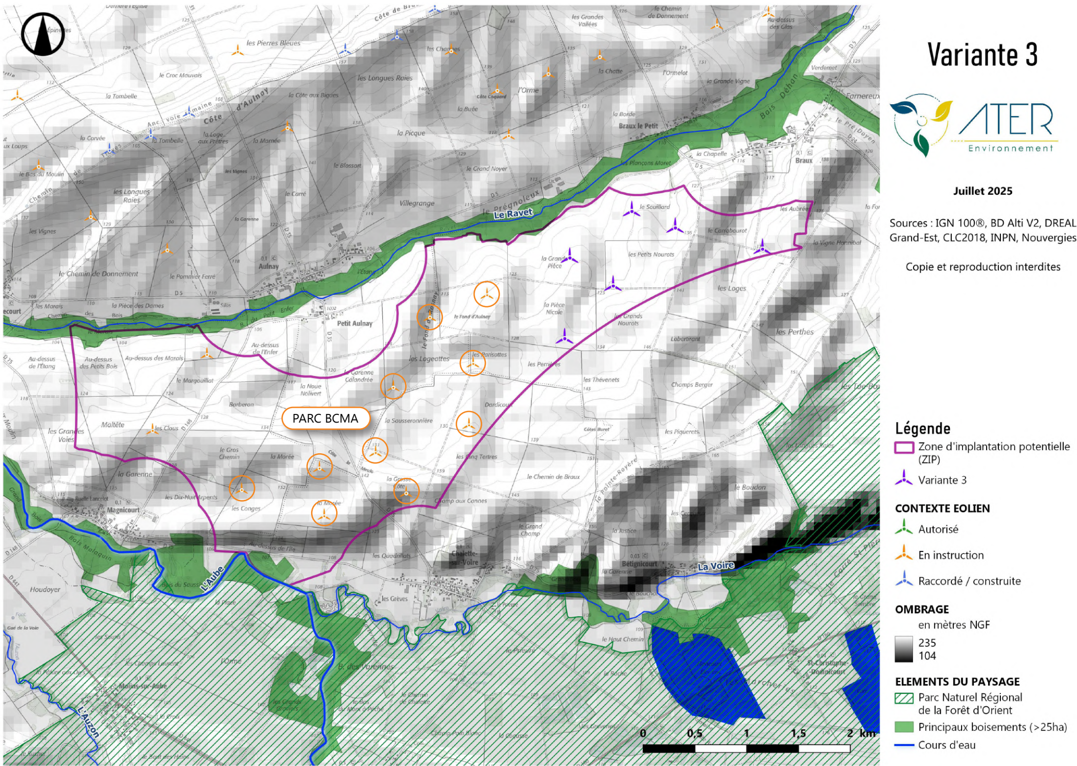
Fig. 143 : Plan d'implantation de la variante 3
