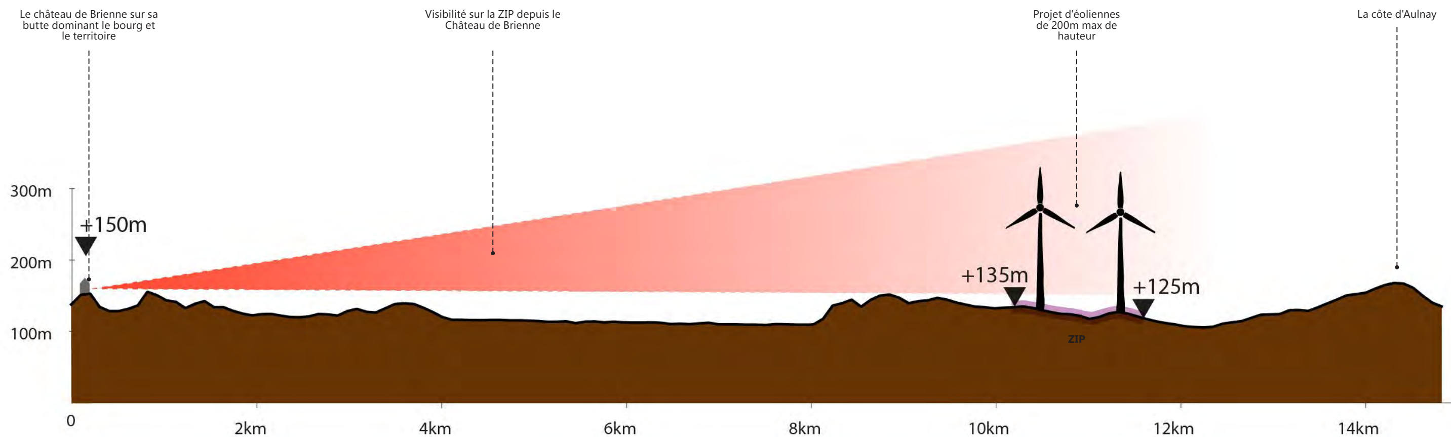
Fig. 103 : Coupe topographique allant du Château de Brienne à la Butte d'Aulnay en passant par la zone d'implantation potentielle. Elle présente une exagération verticale d'un facteur 10. Depuis son implantation en hauteur, le château bénéficie de vues lointaines sur la ZIP. Le bas des futures éoliennes sera caché par le relief tandis que le mat et la partie haute seront visibles.
