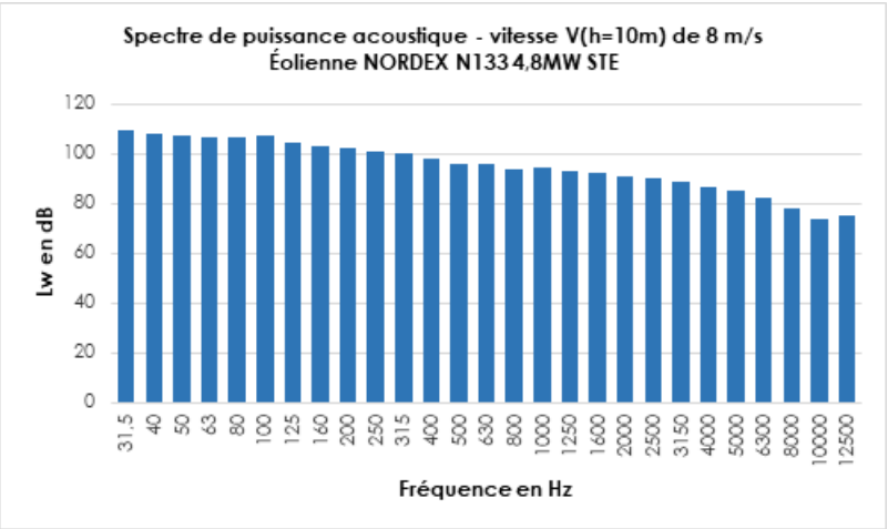
Figure 16. Graphe des niveaux de puissance acoustique d'une NORDEX N133 4,8MW STE par bande de tiers d'octave à la vitesse de 8 m/s
