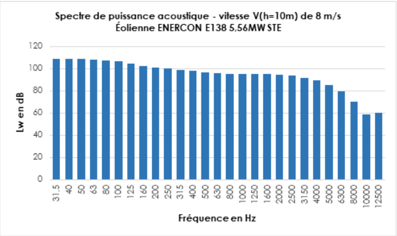
Figure 18. Graphe des niveaux de puissance acoustique d'une ENERCON E138 5,56MW STE par bande de tiers d'octave à la vitesse de 8 m/s
