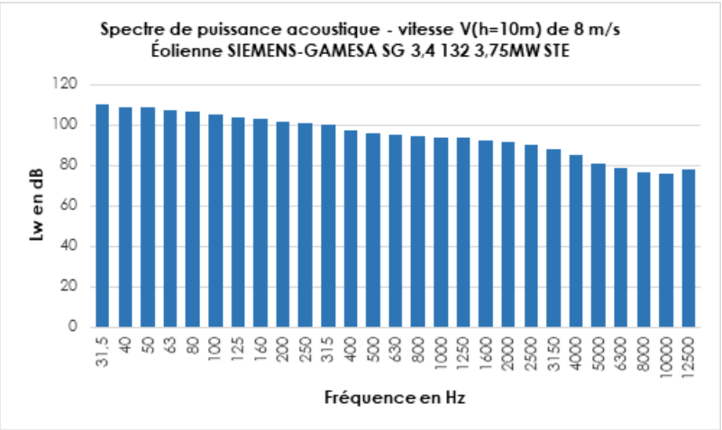
Figure 20. Graphe des niveaux de puissance acoustique d'une SIEMENS-GAMESA SG 3,4 132 3,75MW STE par bande de tiers d'octave à la vitesse de 8 m/s
