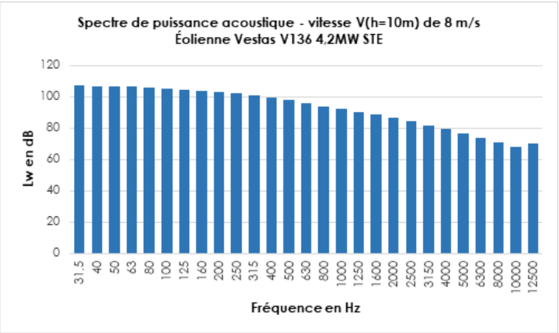
Figure 13. Graphe des niveaux de puissance acoustique d'une VESTAS V136 4,2MW STE par bande de tiers d'octave à la vitesse de 8 m/s
