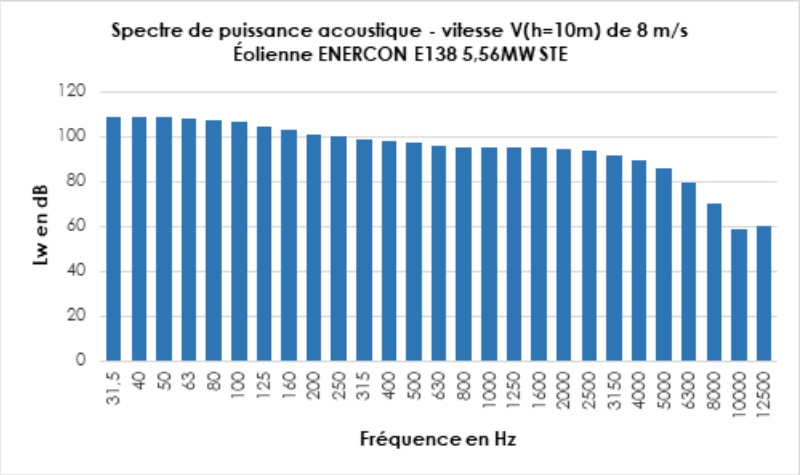
Figure 19. Graphe des niveaux de puissance acoustique d'une ENERCON E138 5,56MW STE par bande de tiers d'octave à la vitesse de 8 m/s
