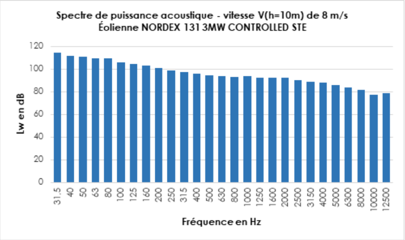
Figure 17. Graphe des niveaux de puissance acoustique d'une NORDEX N131 3,6MW STE par bande de tiers d'octave à la vitesse de 8 m/s
