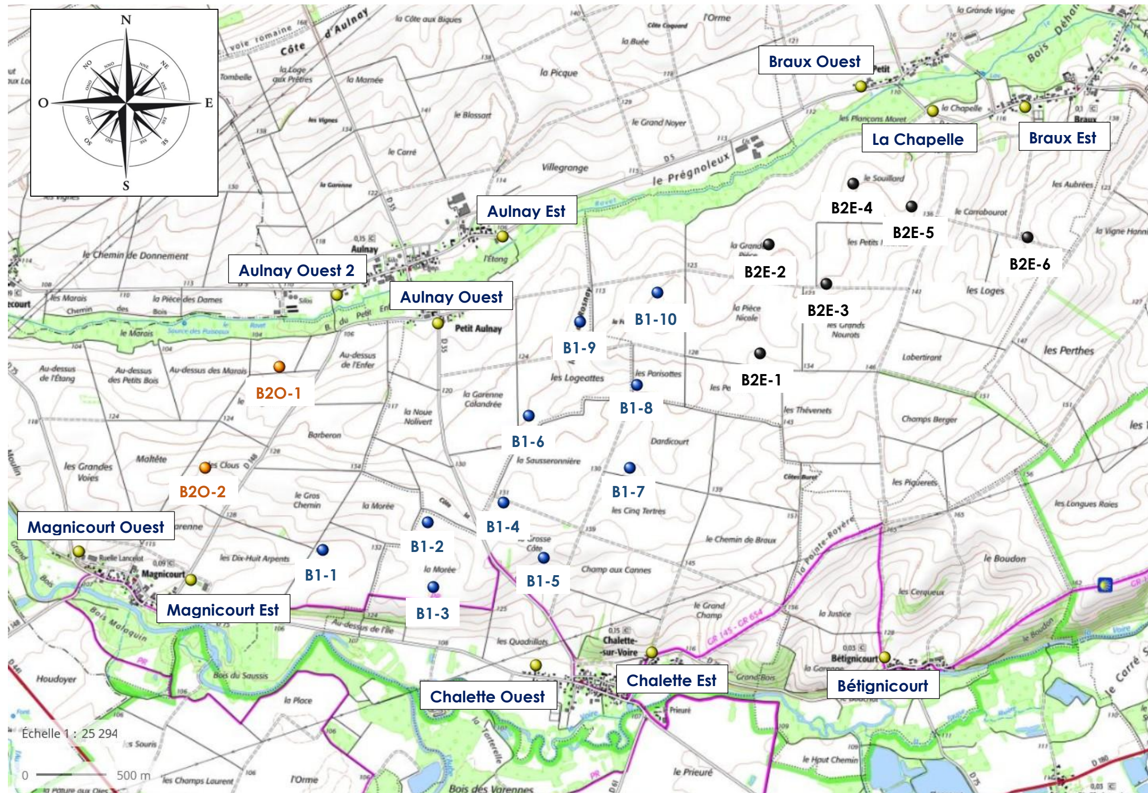
Figure 25. Implantation des points de contrôle et des éoliennes
