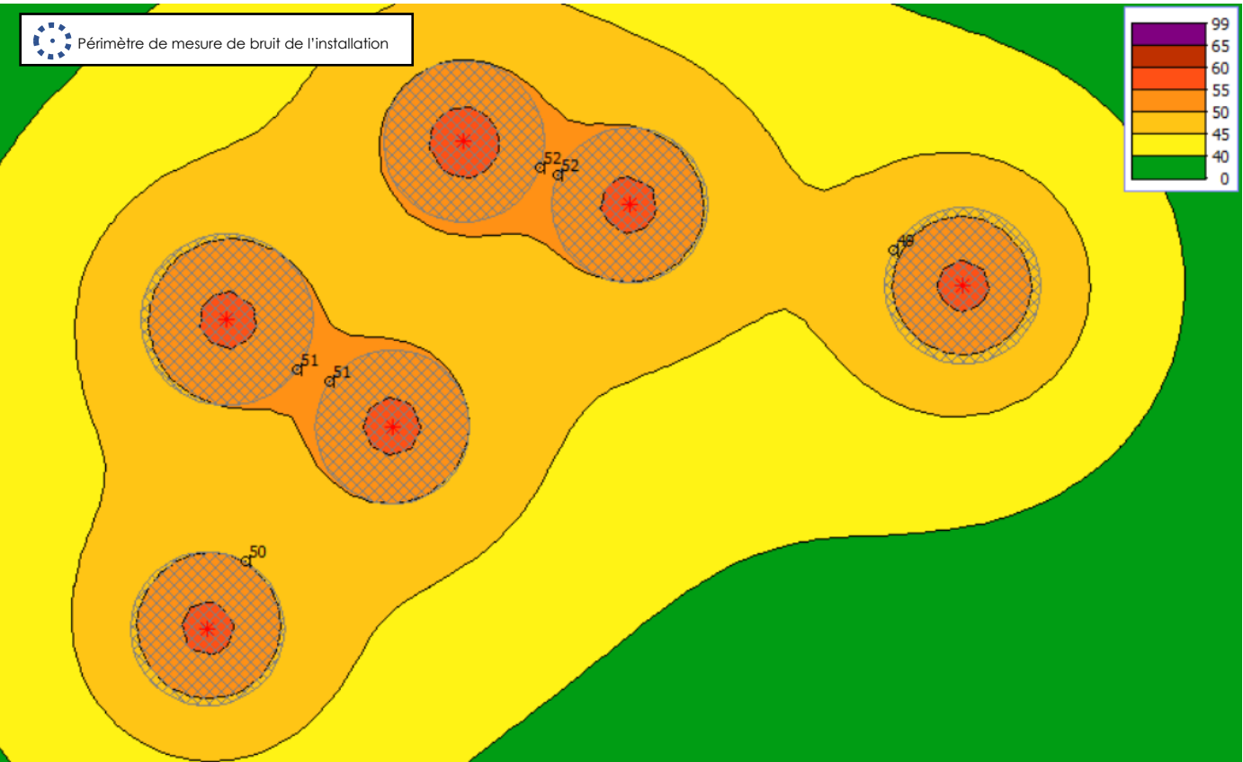
Figure 11. Cartographie sonore – Projet des Nourots – ENERCON E160 5,56MW STE
