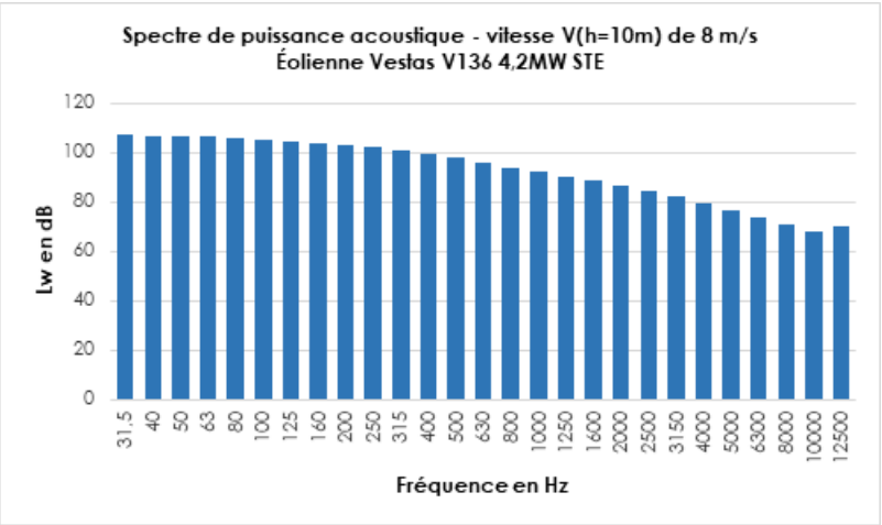
Figure 14. Graphe des niveaux de puissance acoustique d'une VESTAS V136 4,2MW STE par bande de tiers d'octave à la vitesse de 8 m/s
