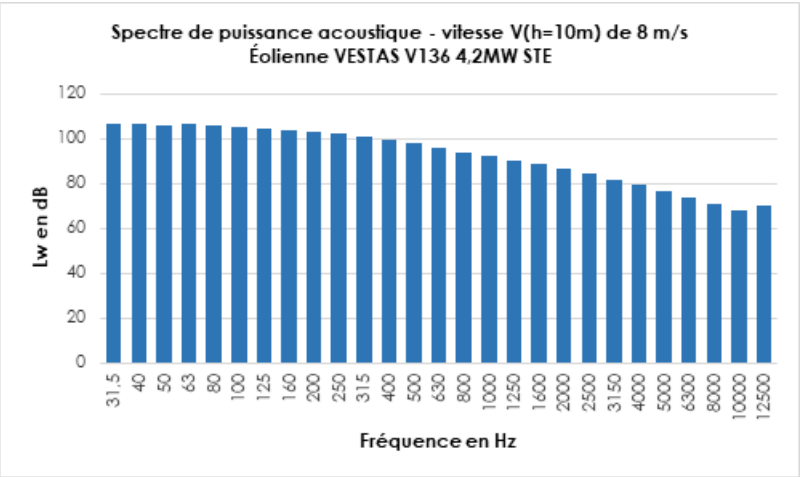
Figure 12. Graphe des niveaux de puissance acoustique d'une VESTAS V136 4,2MW STE par bande de tiers d'octave à la vitesse de 8 m/s
