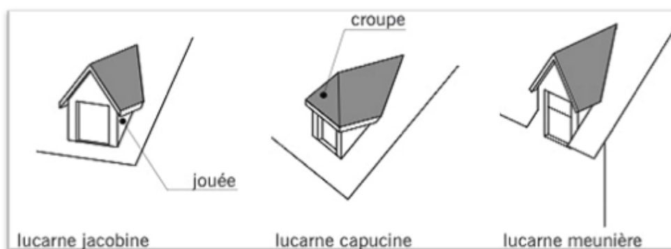
Figure 38 : Types de lucarnes autorisées. Construire en Bresse – CAUE Saône et Loire
